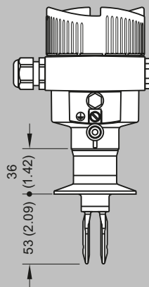
Flange
