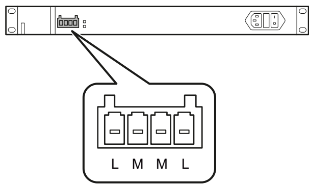
图 6-5 PS598-1 电源单元上插座 X2 的位置
