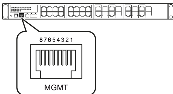
图 6-14 SCALANCE XR524-8C 上带外接口的位置。SCALANCE XR526-8C 与此类似。
