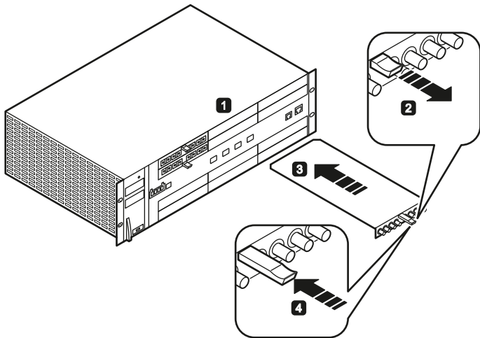
图 5-3 将媒介模块插入 SCALANCE XR552-12M。使用 SCALANCE XR528-6M 时与此类似。
