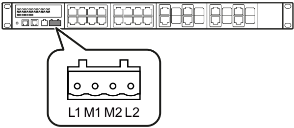
图 6-1 SCALANCE XR524-8C 端子块的位置。SCALANCE XR526-8C 与此类似。
