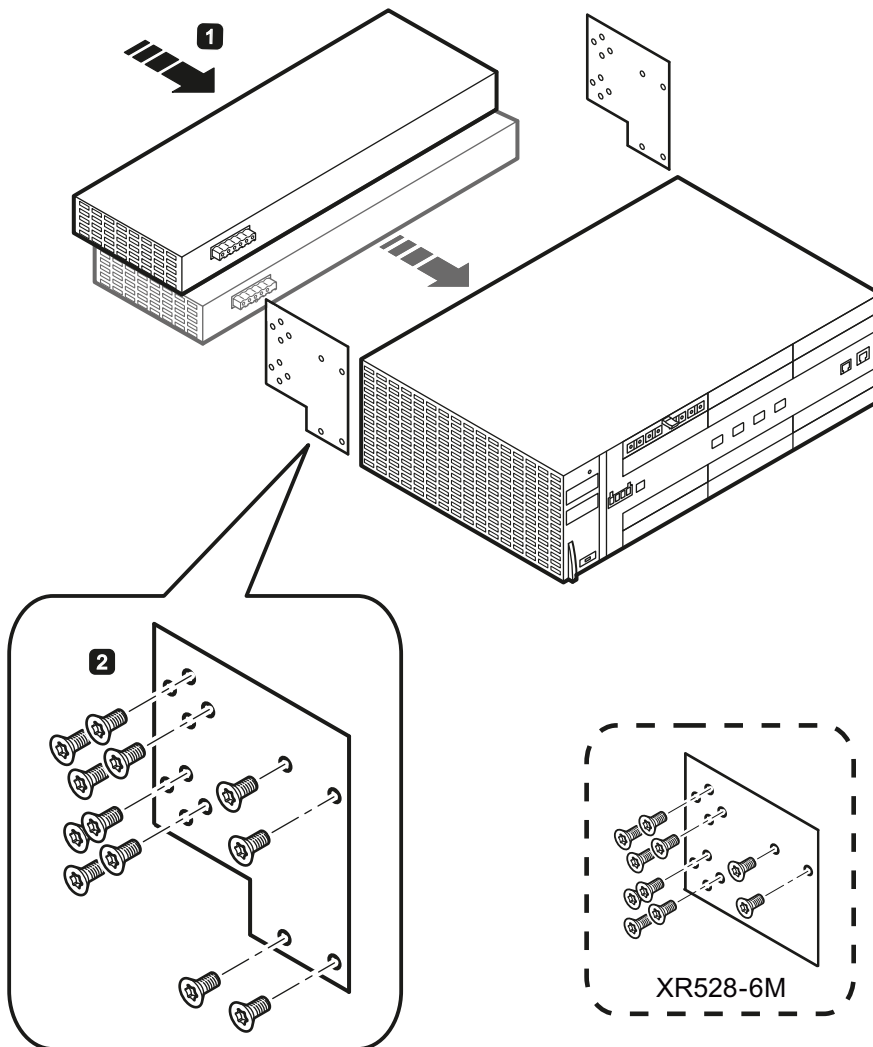
图 5-5 为 SCALANCE XR552-12M 安装后面板。使用 SCALANCE XR528-6M 时与此类似。 在工业以太网交换机的后面板上，提供有插座，最多可直接连接两个 PS598-1 电源单元。 PS598-1 电源单元的背面有相应的插头。
