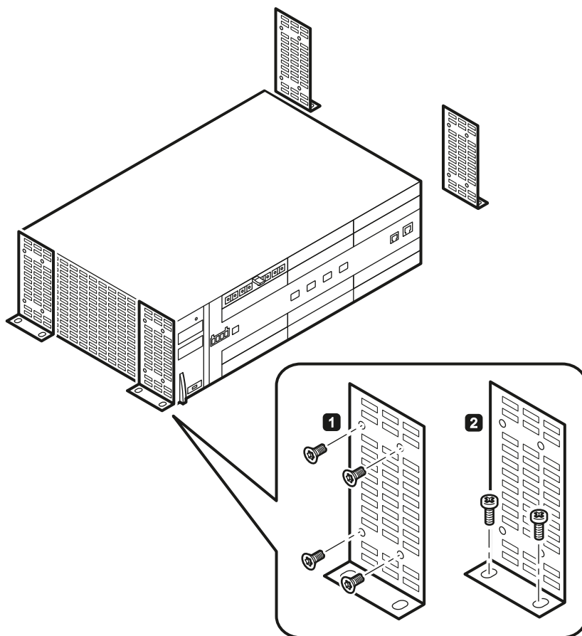
图 5-2 将安装支架安装到 SCALANCE XR552-12M 上。SCALANCE XR524-8C、SCALANCE XR526-8C 和 SCALANCE XR528-6M 的安装方式相同。
