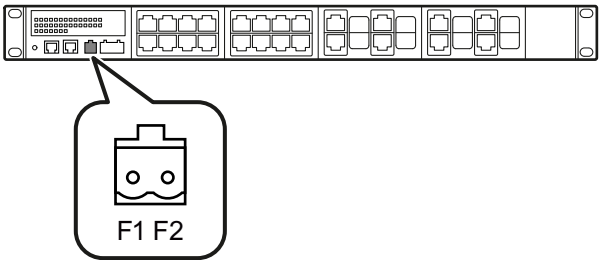
图 6-10 SCALANCE XR524-8C 上信号触点的位置。SCALANCE XR526-8C 与此类似。
