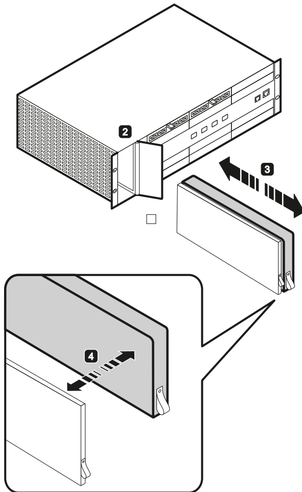
图 8-2 更换 SCALANCE XR552-12M 的风扇。使用 SCALANCE XR528-6M 时与此类似。
