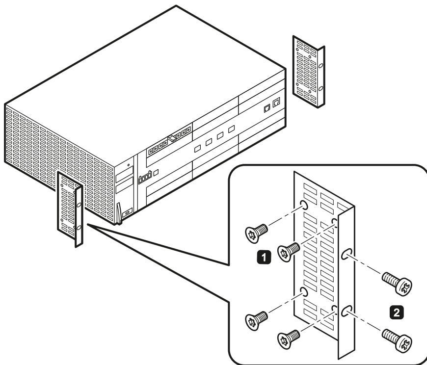
图 5-1 为 SCALANCE XR552-12M 安装 19" 机架。SCALANCE XR524-8C、SCALANCE XR526-8C 和 SCALANCE XR528-6M 的安装方式相同。
