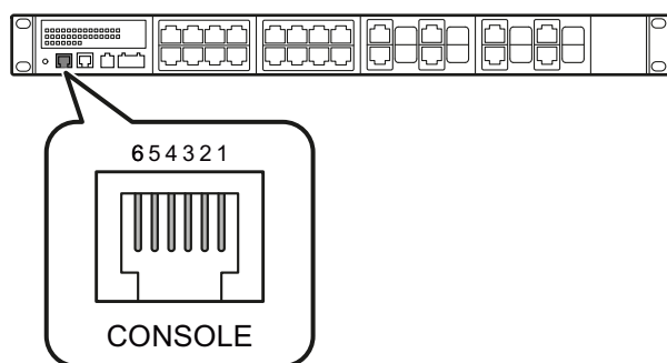
图 6-12 SCALANCE XR524-8C 上 RJ-11 插孔的位置。SCALANCE XR526-8C 与此类似。
