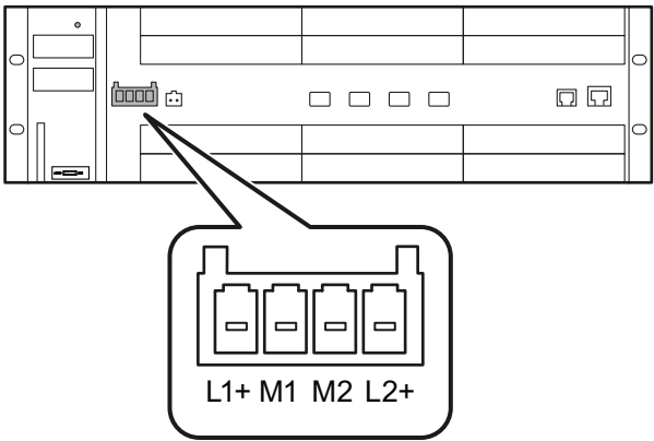
图 6-2 SCALANCE XR552-12M 上端子块的位置。SCALANCE XR528-6M 与此类似。
