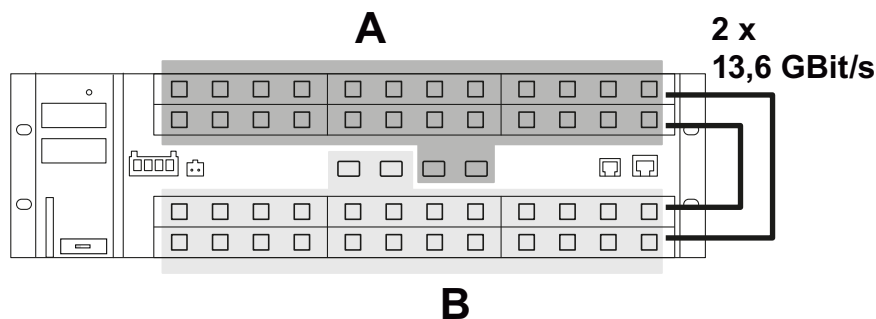
图 6-16 SCALANCE XR552-12M 的块架构
