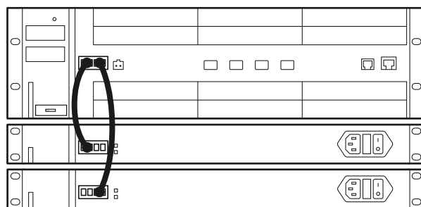
图 6-8 将两个电源单元连接至 SCALANCE XR552-12M。使用 SCALANCE XR528-6M 时与此类似。
