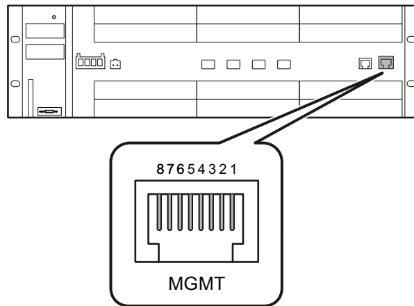
图 6-15 SCALANCE XR552-12M 上带外接口的位置。SCALANCE XR528-6M 上的位置与此类似。
