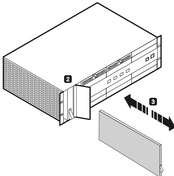
图 8-4 更换 SCALANCE XR552-12M 的滤垫。使用 SCALANCE XR528-6M 时与此类似。
