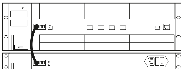
图 6-7 将电源单元连接至 SCALANCE XR552-12M。使用 SCALANCE XR528-6M 时与此类似。
