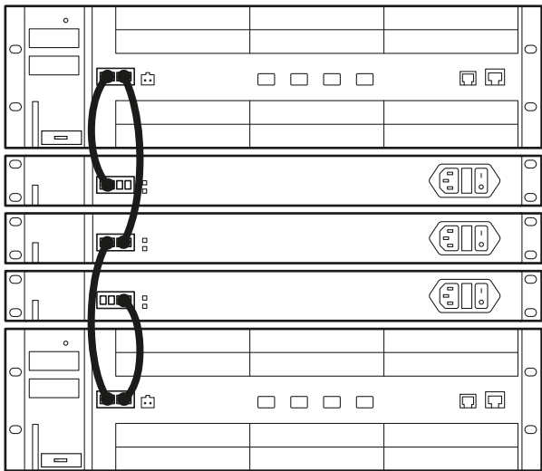
图 6-9 将三个电源单元连接至 SCALANCE XR552-12M。使用 SCALANCE XR528-6M 时与此类似。
