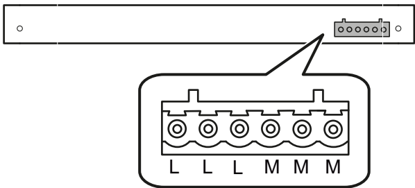
图 6-6 PS598-1 电源单元上插头 X3 的位置
