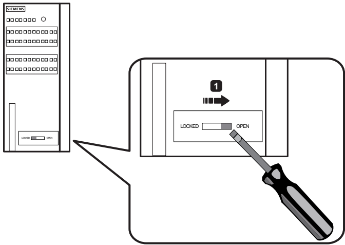
图 8-3 打开 SCALANCE XR552-12M 的机壳。使用 SCALANCE XR528-6M 时与此类似。 2. 打开机壳门 ②。
