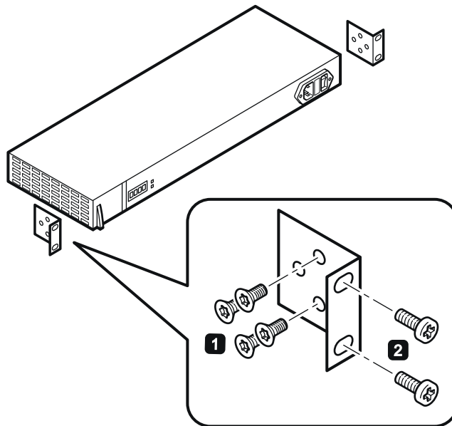
图 5-4 将电源单元安装到 19" 机架上
