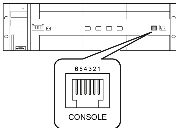
图 6-13 SCALANCE XR552-12M 上 RJ-11 插孔的位置。SCALANCE XR528-6M 与此类似。
