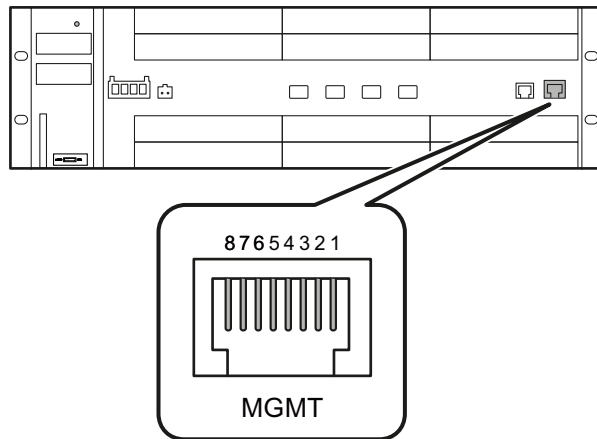
图 6-15 SCALANCE XR552-12M 上带外接口的位置。SCALANCE XR528-6M 与此类似。
