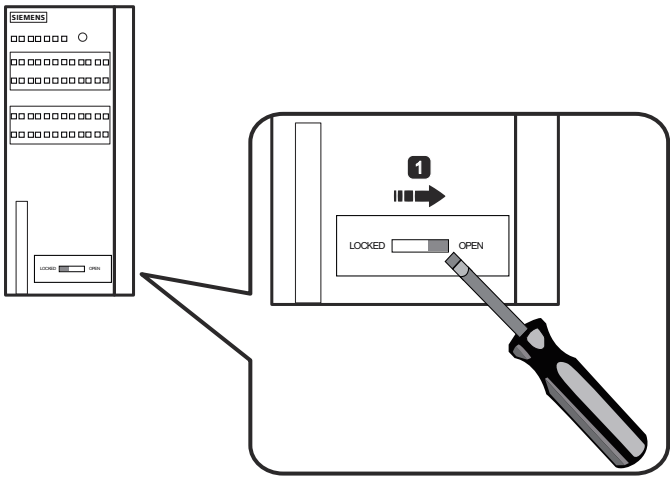
图 7-3 打开 SCALANCE XR552-12M 的机壳。使用 SCALANCE XR528-6M 时与此类似。 2. 打开机壳门 ②。
