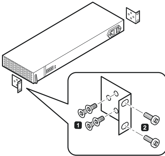
图 5-4 将电源单元安装到 19" 机架上
