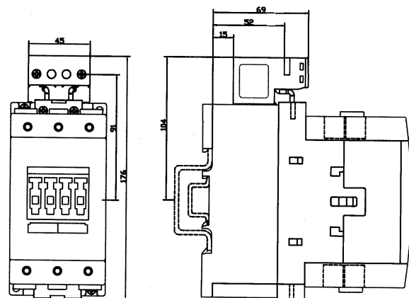
Fig. 3-126: 3RT10 4.-1X.40-0LA2
