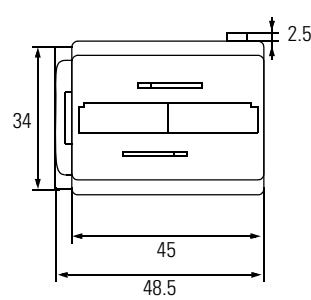
3RA1924-1A
