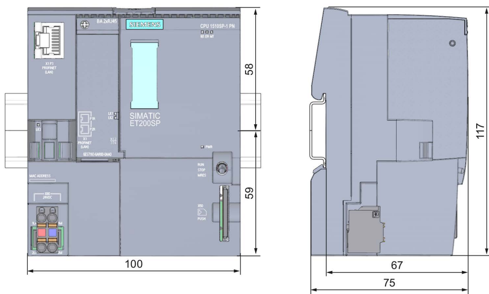
Bild A-1 Maßbild 1510SP-1 PN
