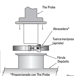
Férula sanitaria 4"
