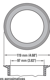
Férula sanitaria 4"
