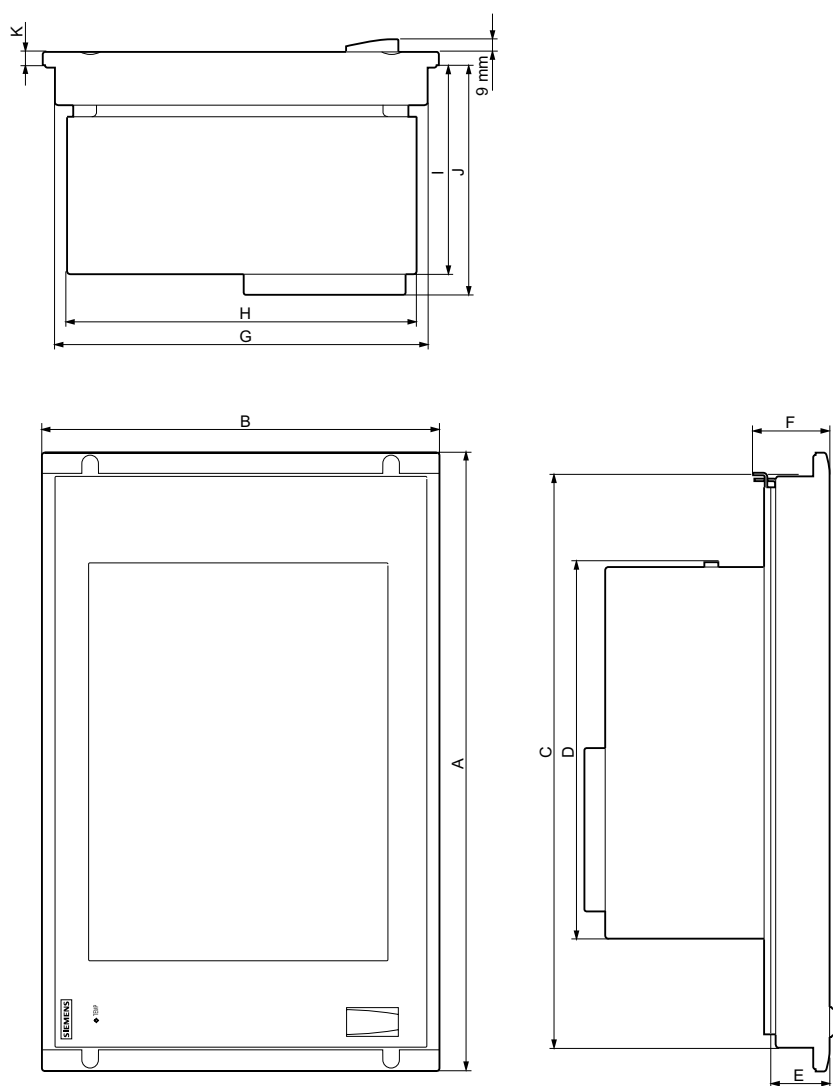
图 16-1 Panel PC 677B 尺寸图
