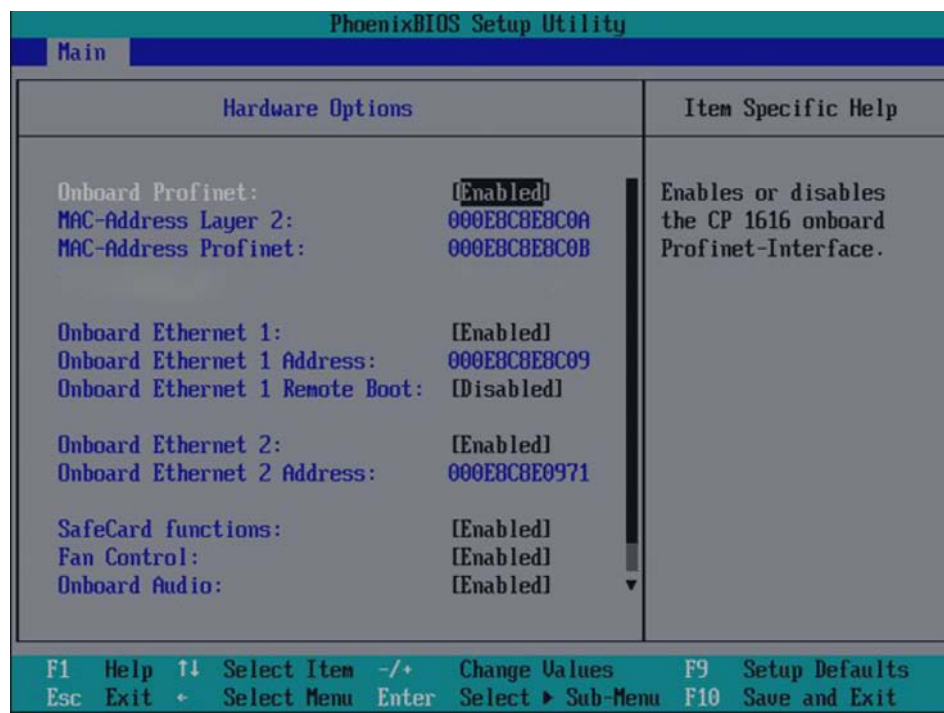
图 17-14 PROFINET 的“Hardware Options（硬件选项）”域
