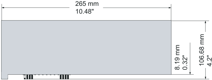
图 16-4 PCI 模块的最大尺寸
