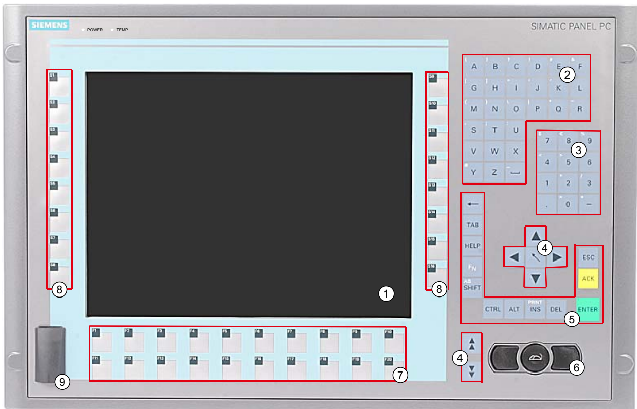
图 10-1 12" 按键式面板实例
