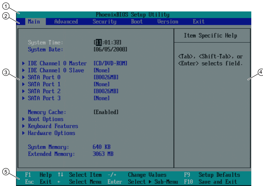
图 17-5 SETUP 主菜单（实例）
