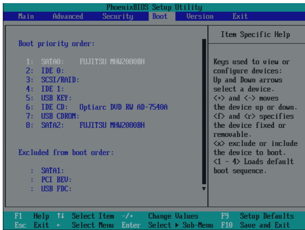
图 17-21 Boot（引导）菜单
