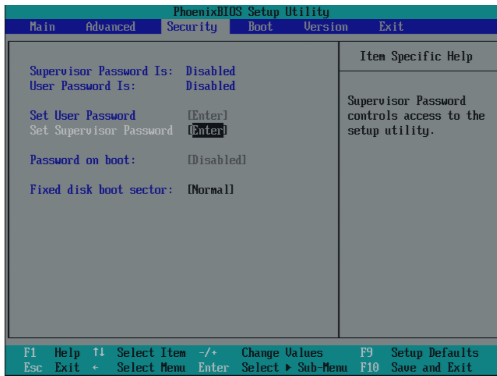
图 17-20 Security（安全性）菜单
