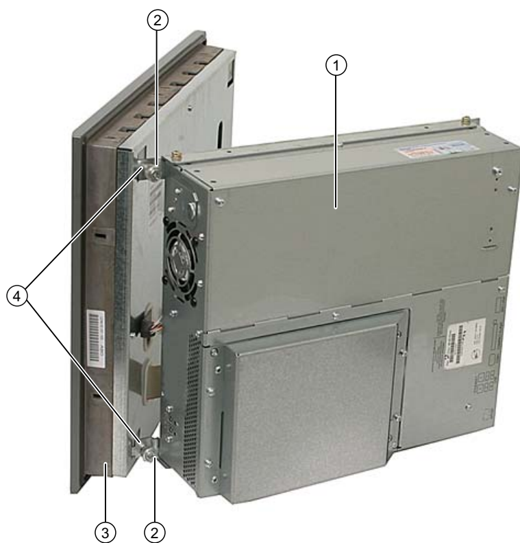
图 12-1 将控制单元与计算机单元分离
