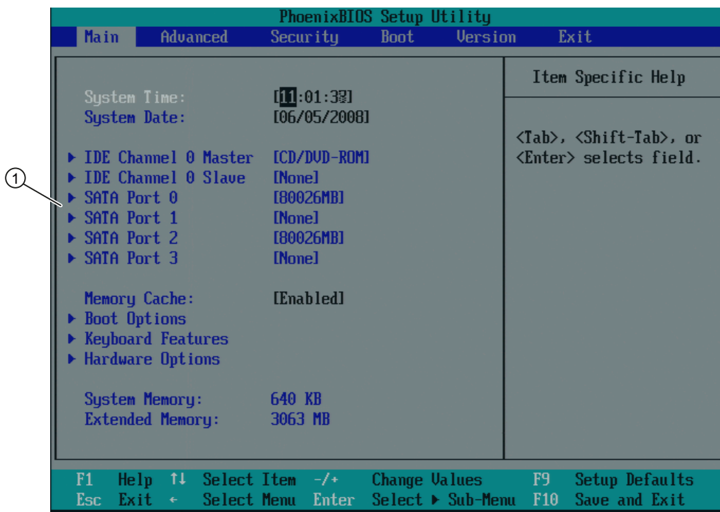
图 17-6 Main (主) 菜单 (实例)
