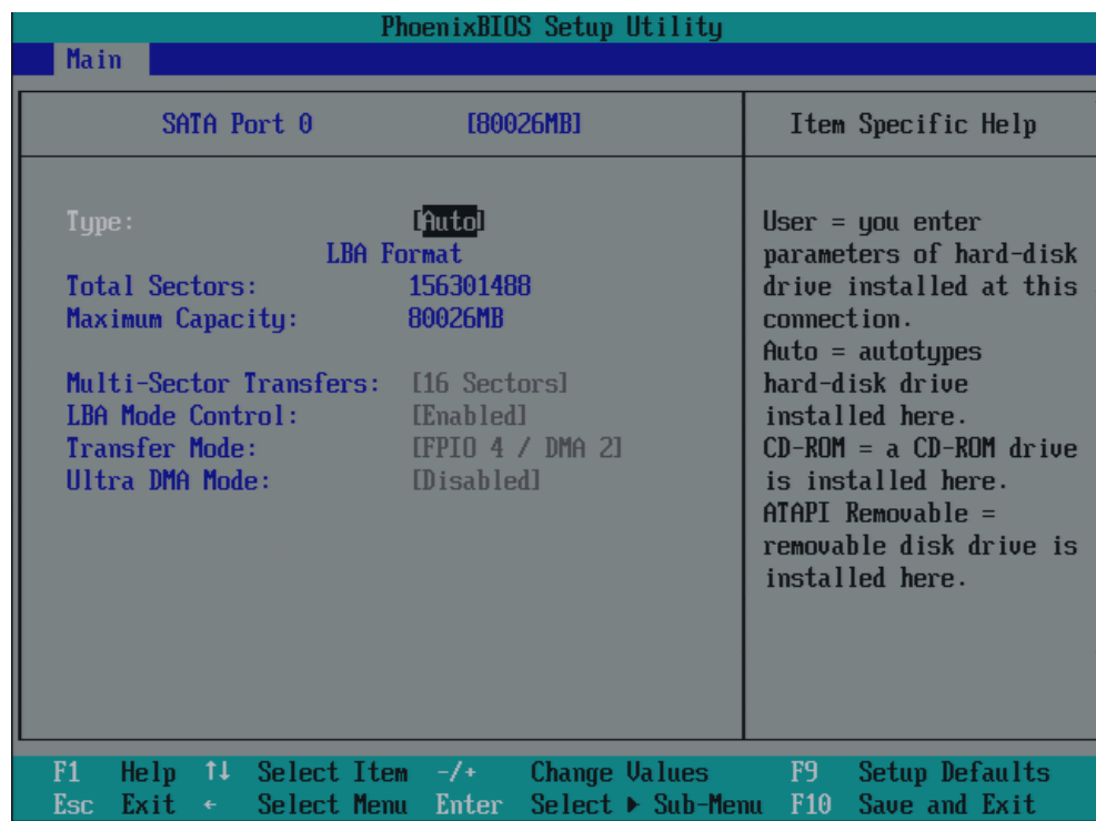
图 17-8 SATA Port 0 (SATA 端口 0) (实例)
