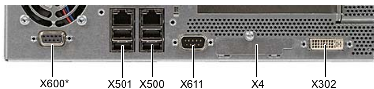
图 17-2 端口上的连接器针脚分配
