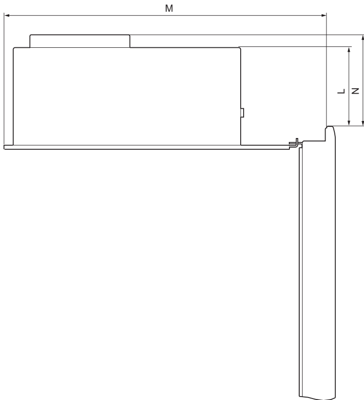
图 16-2 Panel PC 677B 尺寸图，从控制单元旋下计算机单元
