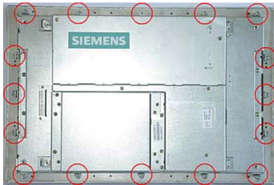
图 5-5 卡件的位置
