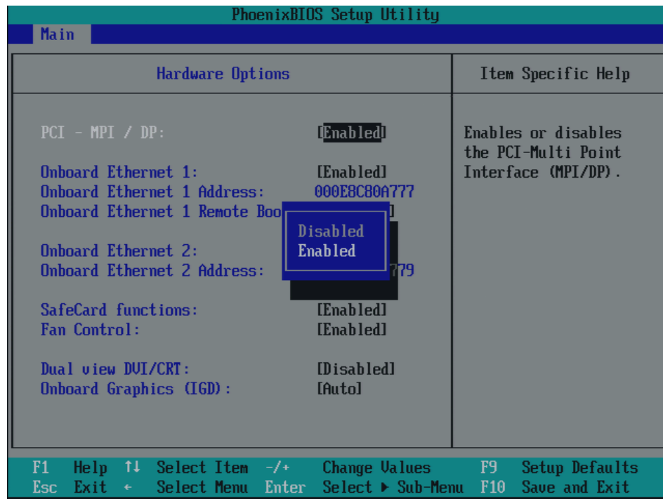
图 17-13 “Hardware Options（硬件选项）”域
