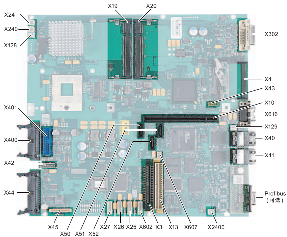
图 17-1 母板上的接口
