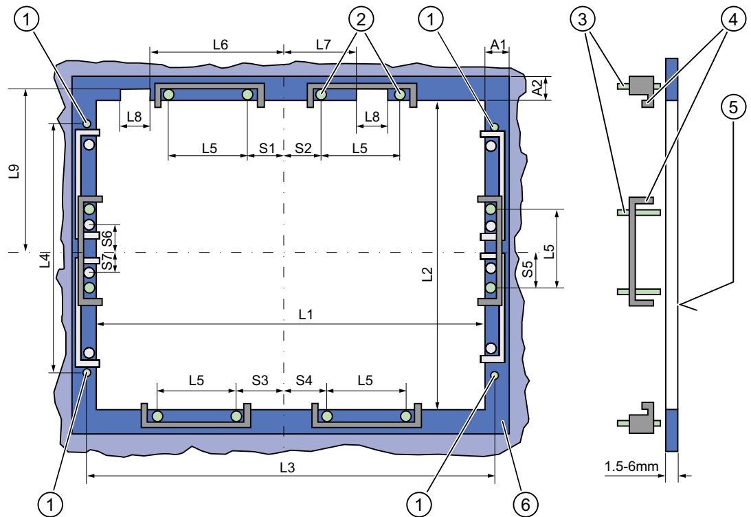
图 4-2 螺钉的钻孔和卡件螺钉的压点
