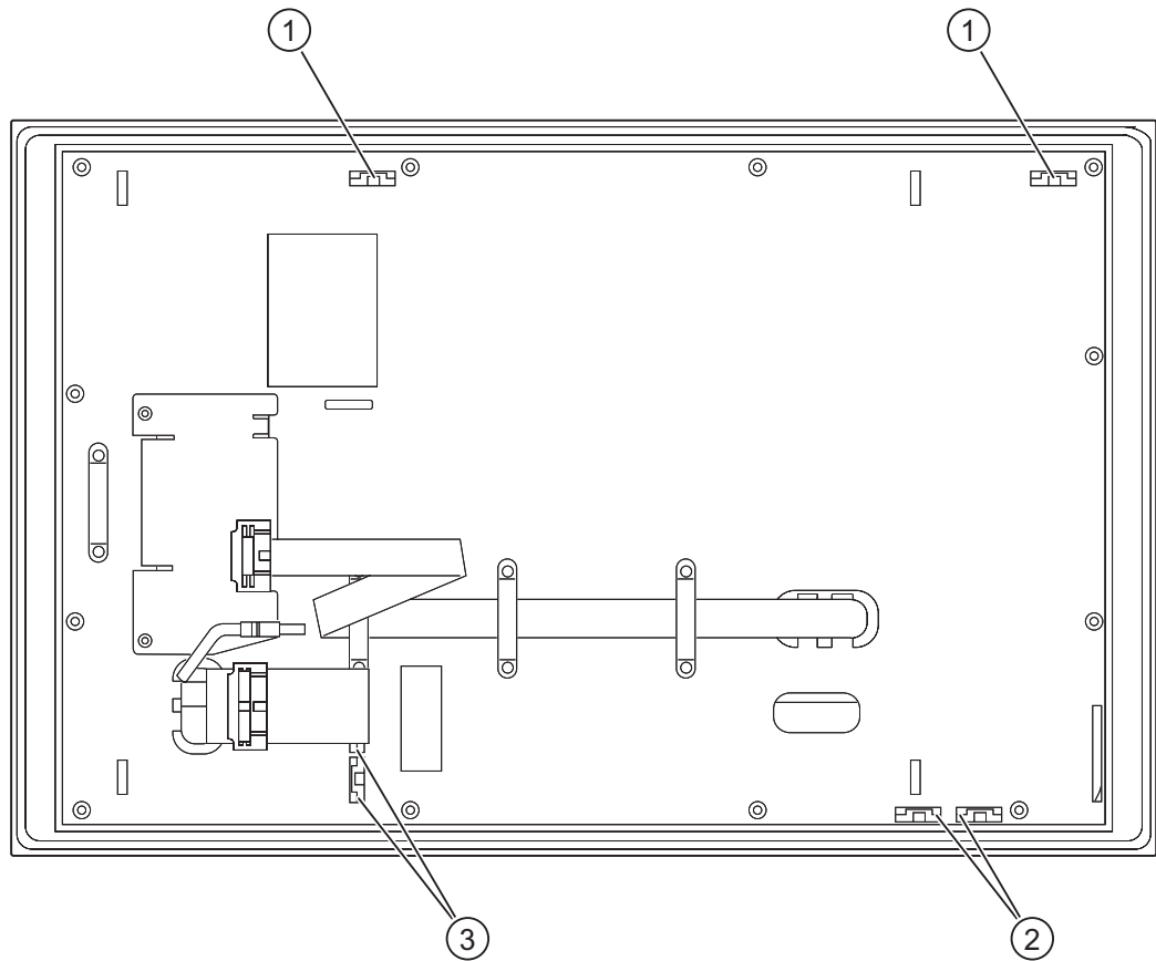
图 10-7 12" 触摸屏前面板实例中带有连接和标签条插槽的控制单元后侧。
