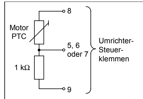
Bild 3-8 Schaltung für Motor-Überhitzungsschutz mit PTC
