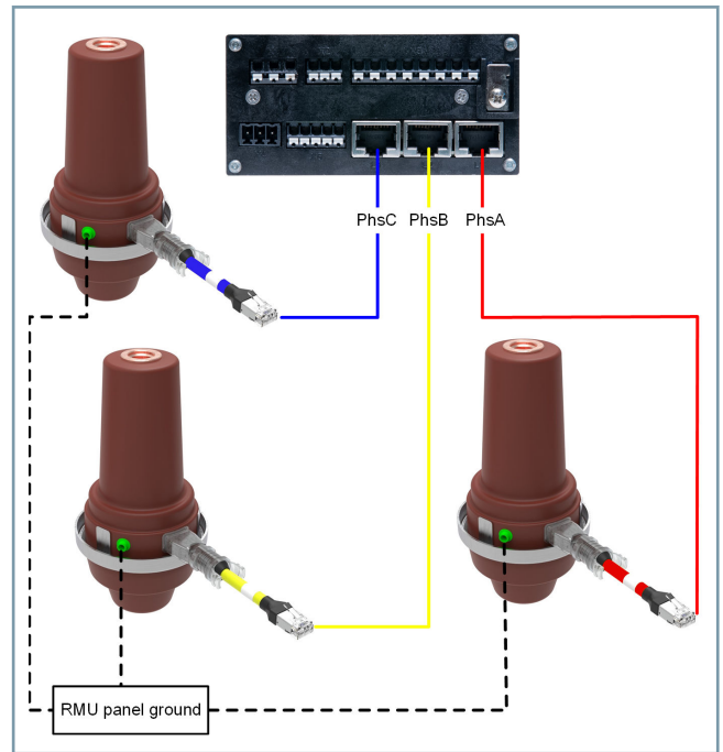
[dw_sicam-sib_sensor-conn, 2_en_US]
