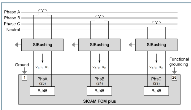
[dw_sicam-sib_sel-curr-temp, 2_en_US]
