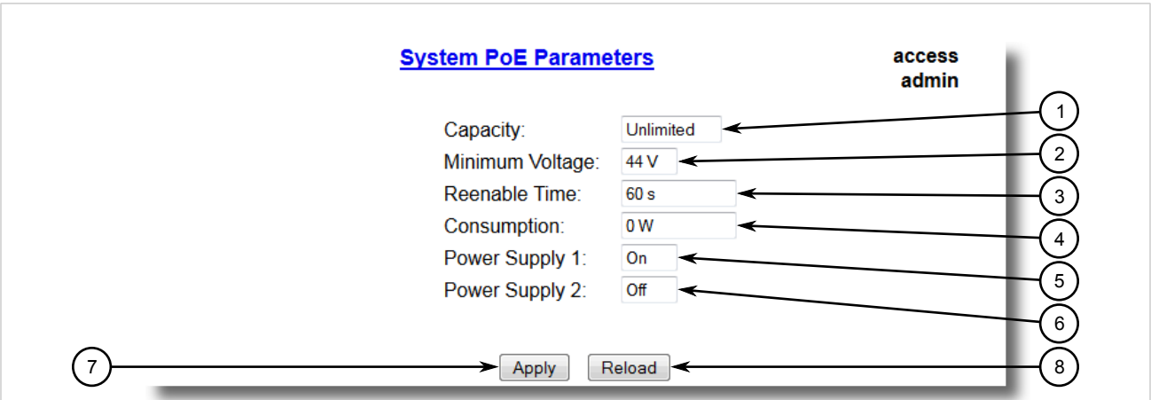
Figure 31 : Formulaire System PoE Parameters
