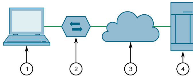
Figure 174 : Topologie générale de IEEE 802.1x
