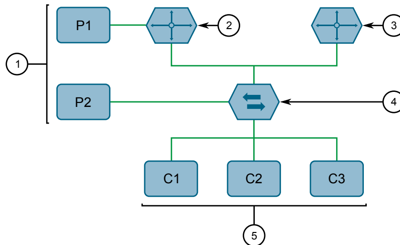
Figure 157 : Exemple - Fonctionnement combiné du routeur et du commutateur IGM
