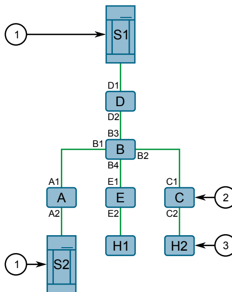
Figure 161 : Exemple - Établir une appartenance à un groupe avec GMRP
