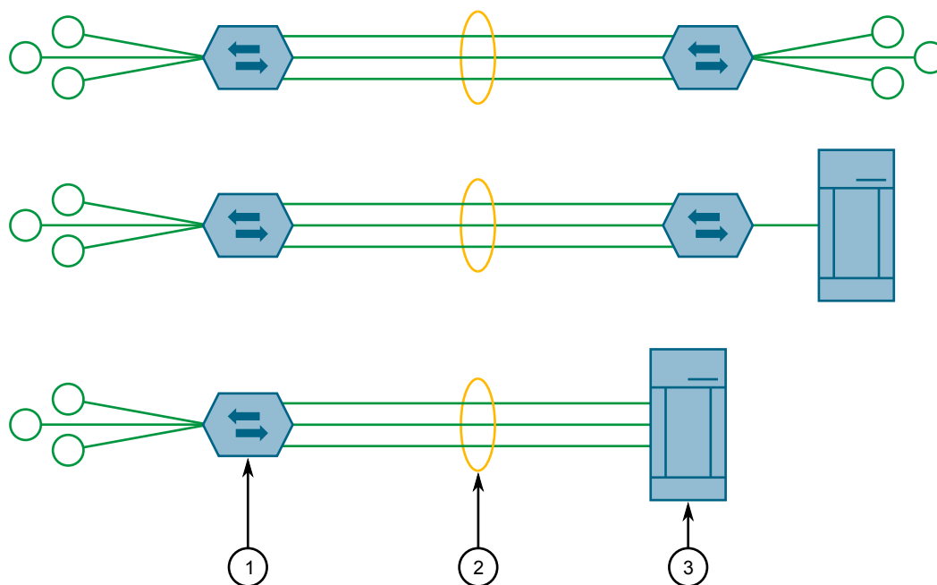
Figure 180 : Exemples d'agrégation de liaisons
