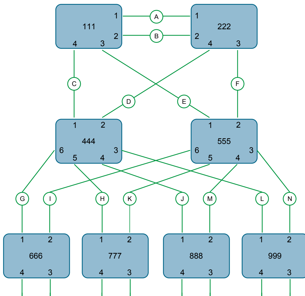
Figure 97 : Exemple - configuration de câblage structuré
