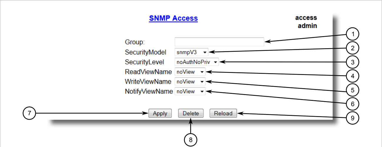
Figure 146 : Formulaire SNMP Access
