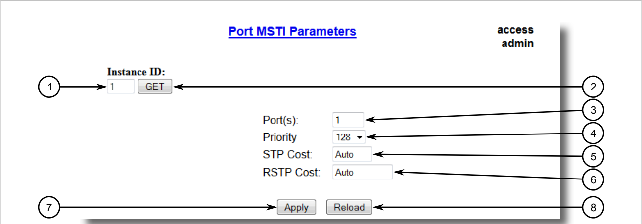
Figure 111 : Formulaire Port MSTI Parameters
