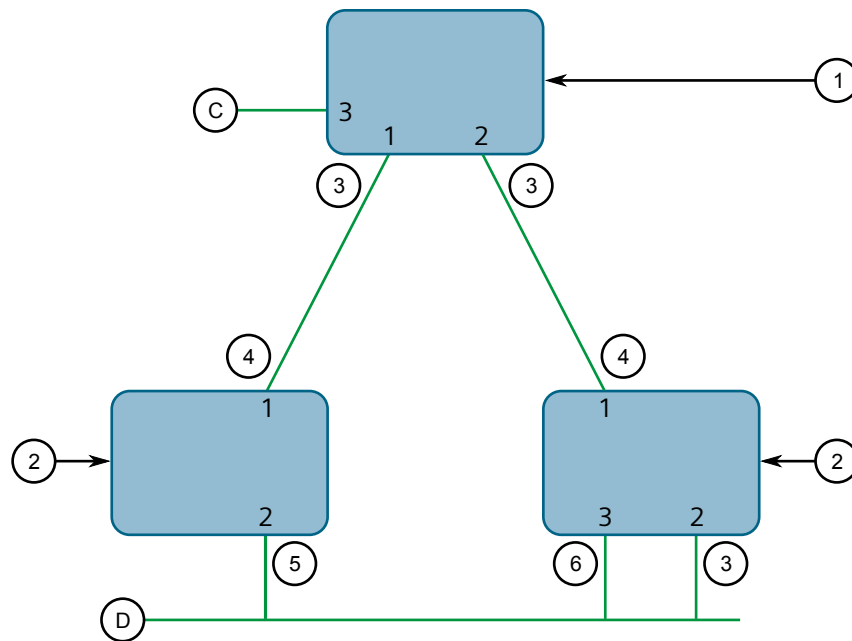
Figure 96 : Rôles de pont et port
