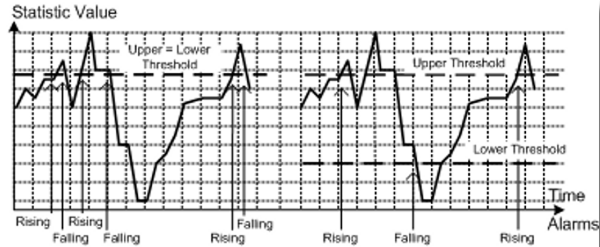
Figure 57 : Le processus d'alarme
