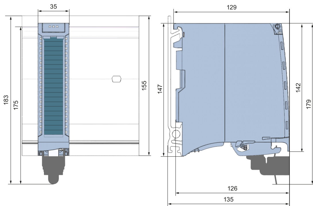
Figura A-1 Croquis acotado del módulo AI 8xU/I/RTD/TC ST
