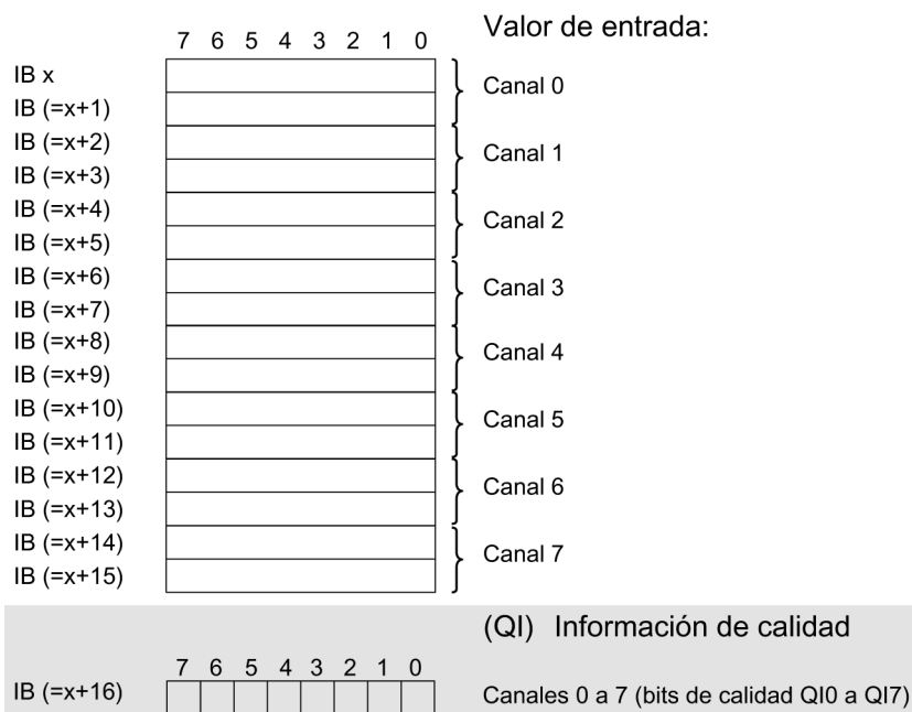
Figura 4-4 Área de direcciones en la configuración como AI 8xU/I/RTD/TC ST de 1 x 8 canales con información de calidad
