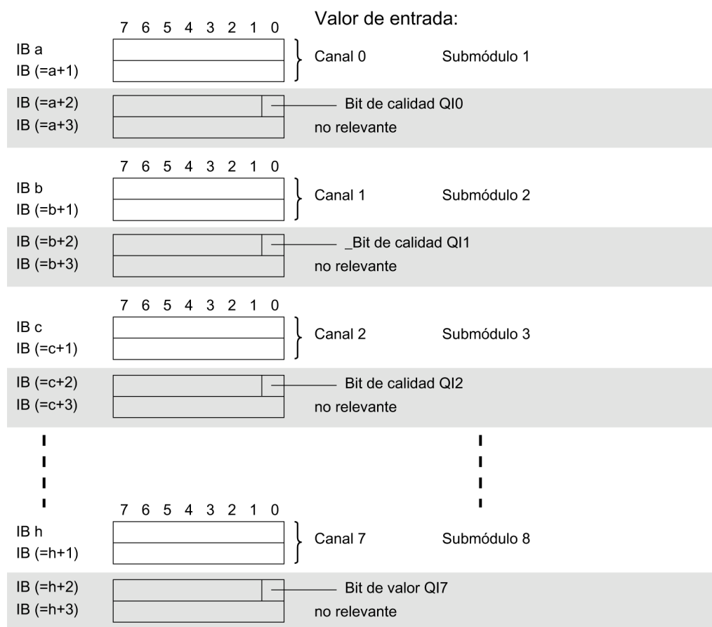
Figura 4-5 Área de direcciones en la configuración como AI 8xU/I/RTD/TC ST S QI de 8 x 1 canales con información de calidad
