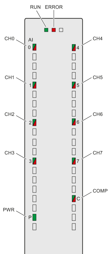
Figura 5-1 LED del módulo AI 8xU/I/RTD/TC ST
