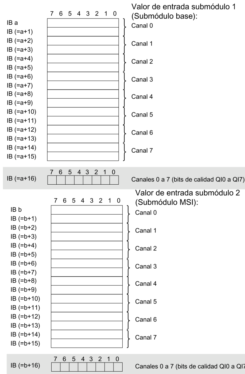
Figura 4-6 Área de direcciones en la configuración como AI 8xU/I/RTD/TC ST MSI de 1 x 8 canales con información de calidad
