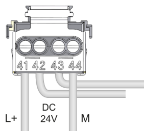
Figura 3-1 Conexión del módulo de alimentación
