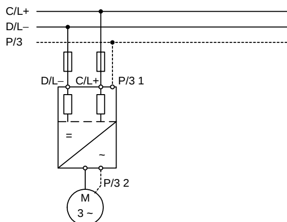
Bild 7-3 DC-Sammelschienen
