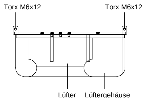
Bild 11-1 Lüfterbaugruppe
