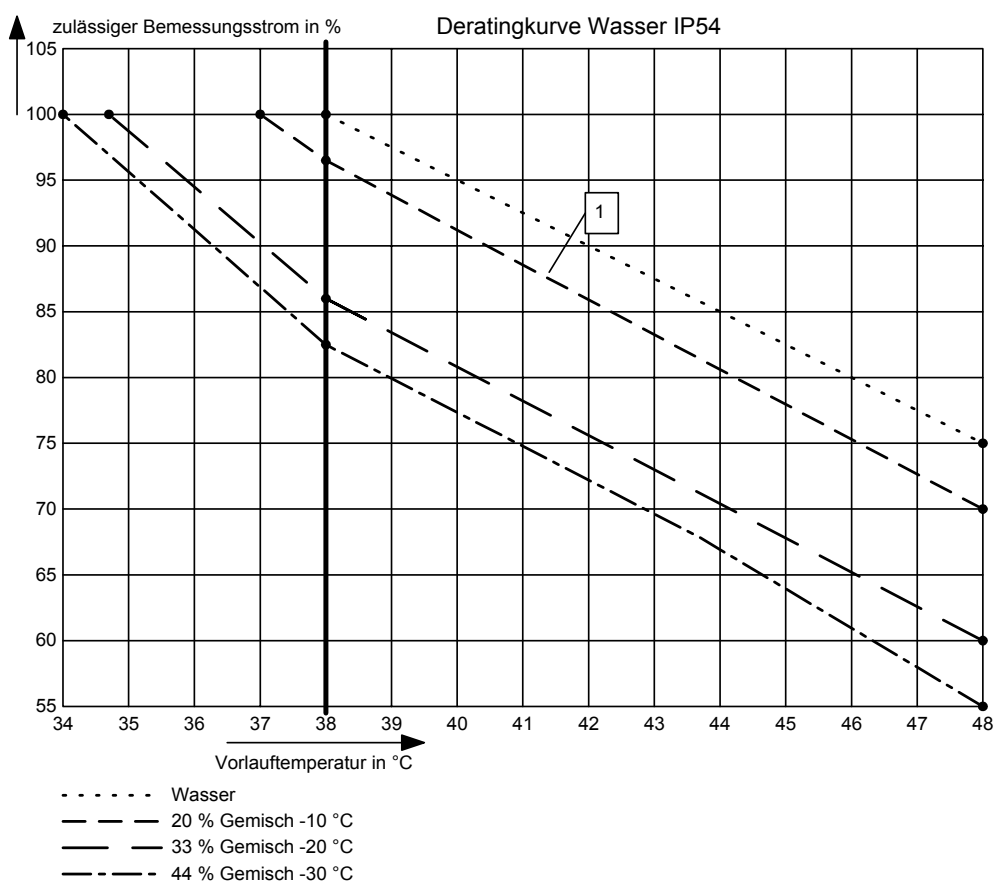
Bild 13-5 Reduktionskurve 2 für den Einbau in IP54 Schränke
