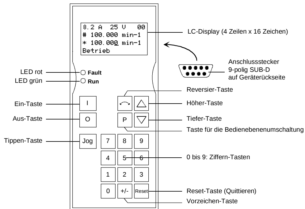
Bild 8-15 Ansicht OP1S
