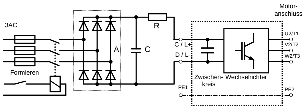
Bild 12-1 Formierschaltung
