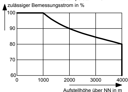
Bild 13-1 Derating-Kurven
