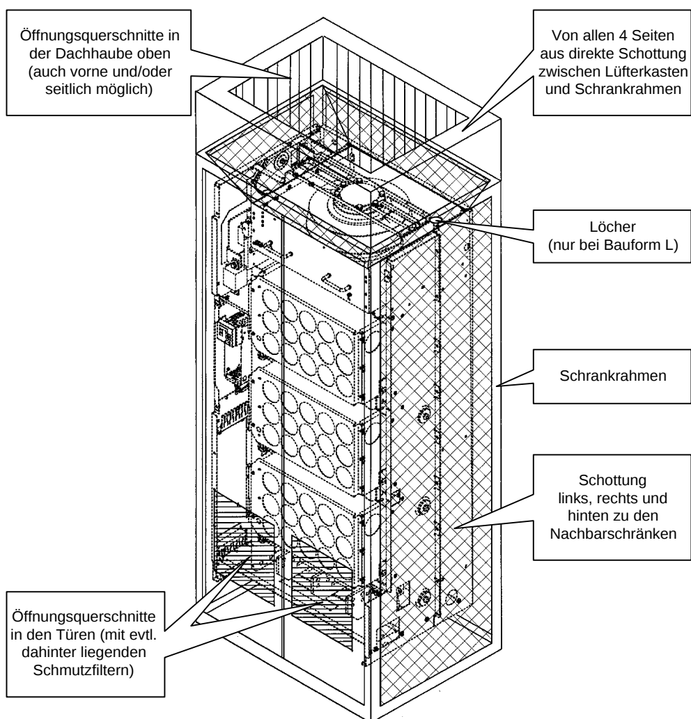
Bild 5-8 Schottungsmaßnahmen
