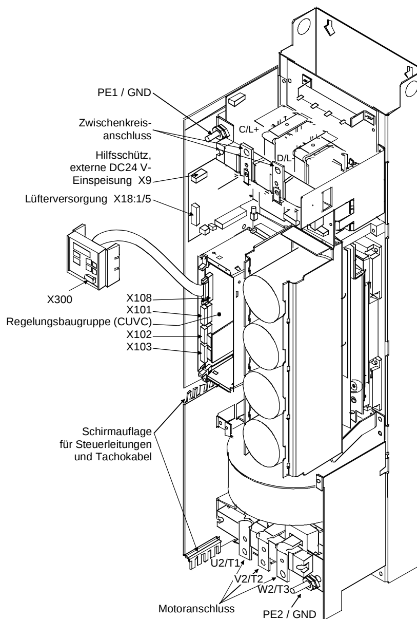
Bild 7-1 Anschlussübersicht Bauform E und F
