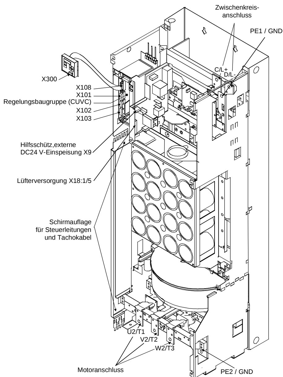
Bild 7-2 Anschlussübersicht Bauform G
