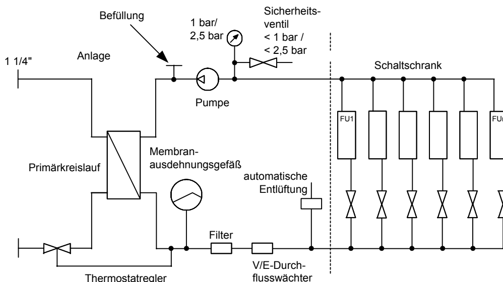
Bild 13-3 Wasser-Wasser-Wärmetauscher
