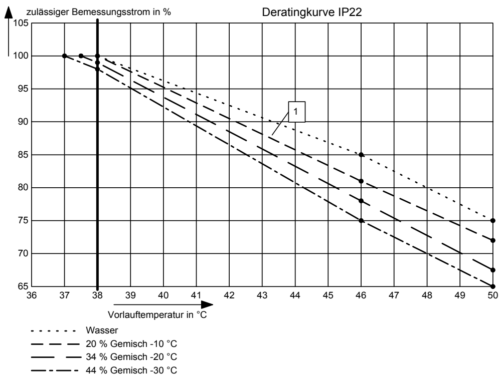
Bild 13-4 Reduktionskurve für den Einbau in IP22 Schränke
