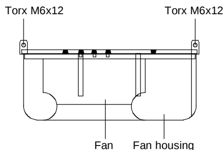
Fig. 11-1 Fan assembly
