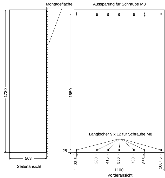
Bild 5-5 Maßbild Bauform L
