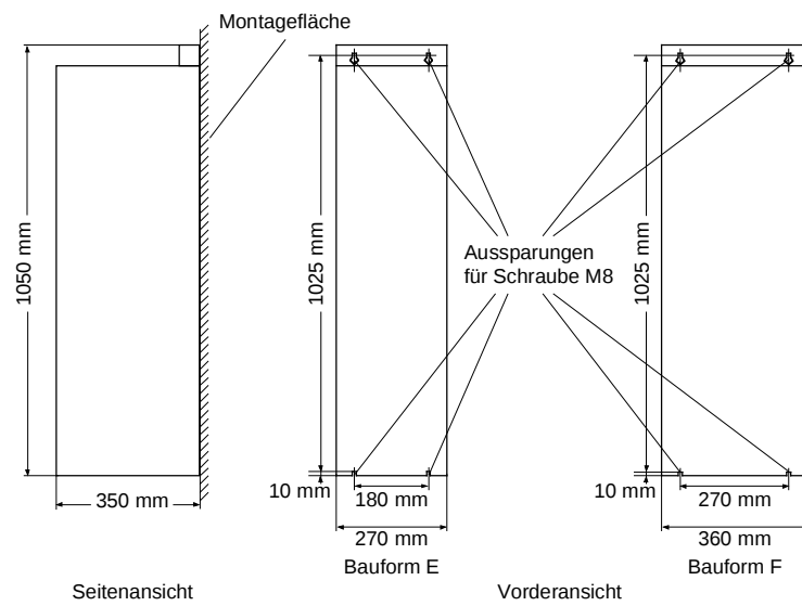
Bild 5-2 Maßbild Bauformen E, F
