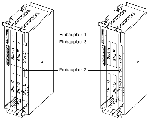
Bild 5-9 Lage der Slots für Kompakt- und Einbaugeräte
