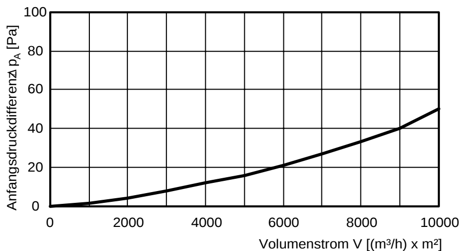
Bild 5-7 Datenblatt der Filtermatte
