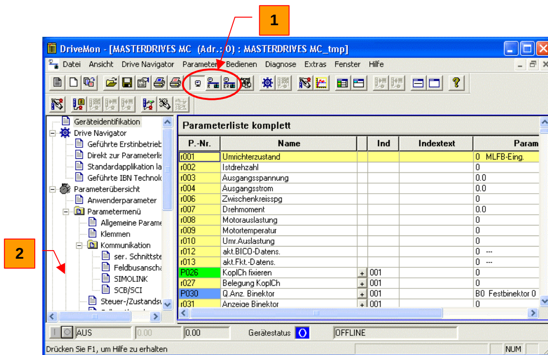
Bild 8-9 Antriebsfenster/Parameterliste
