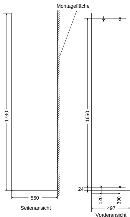
Bild 5-6 Maßbild Drosselchassis
