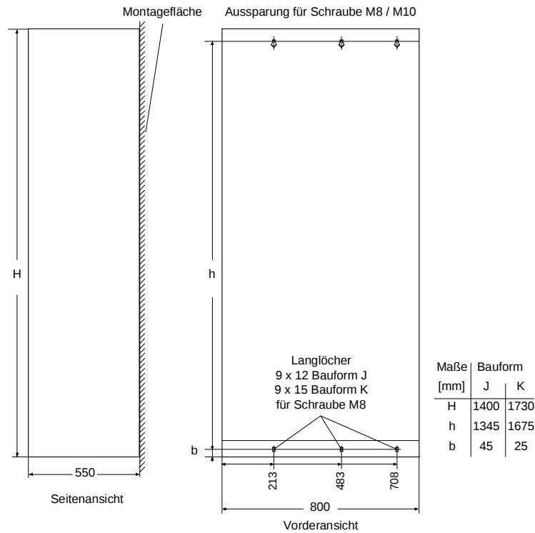
Bild 5-4 Maßbild Bauform J, K
