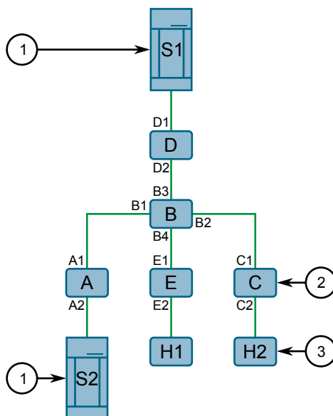
Figure 153 : Exemple - Établir une appartenance à un groupe avec GMRP
