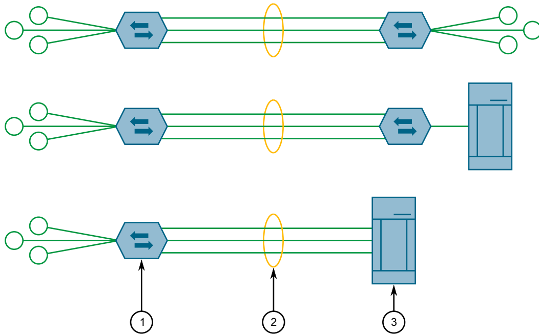
Figure 163 : Exemples d'agrégation de liaisons
