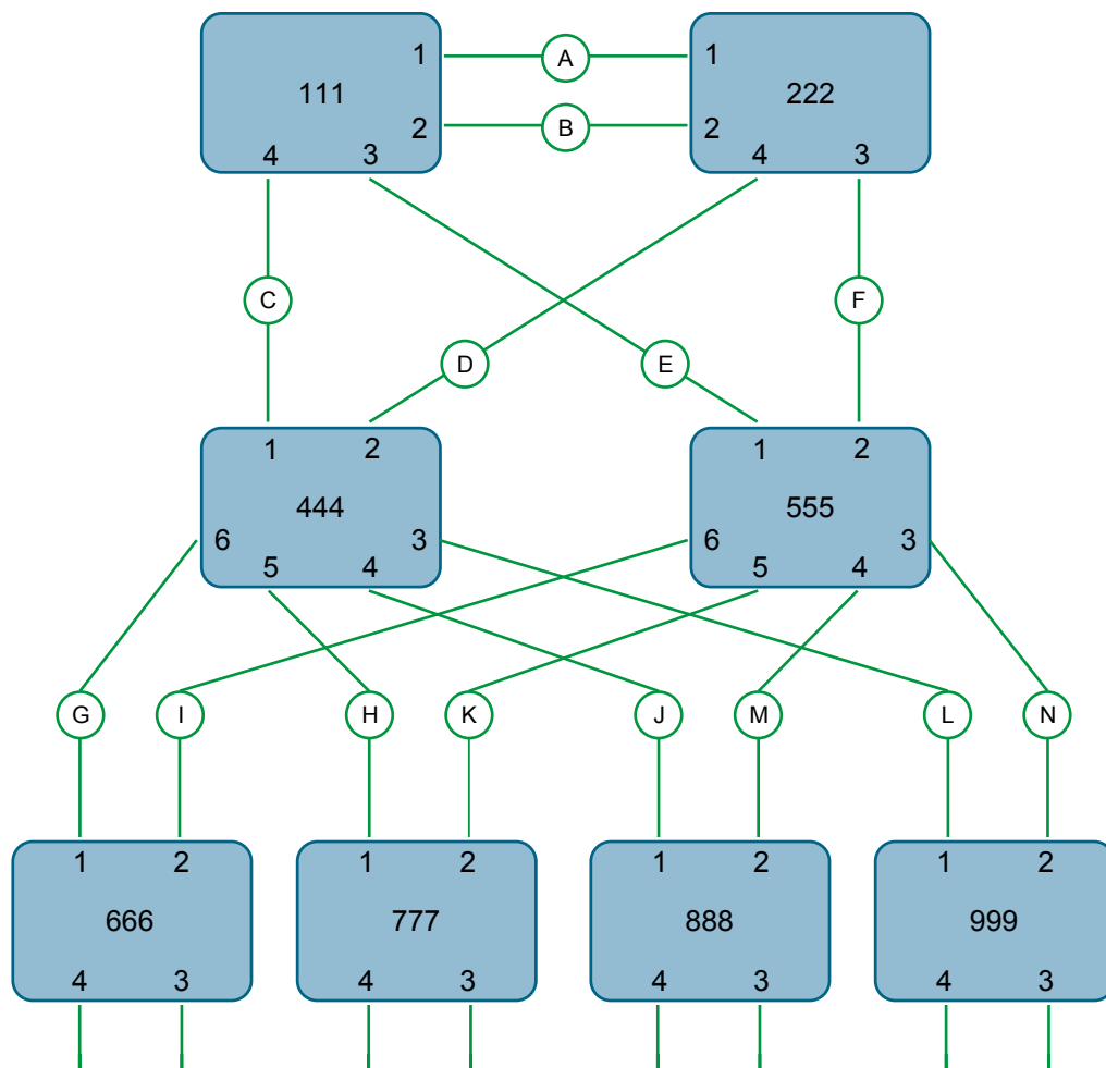
Figure 88 : Exemple - configuration de câblage structuré
