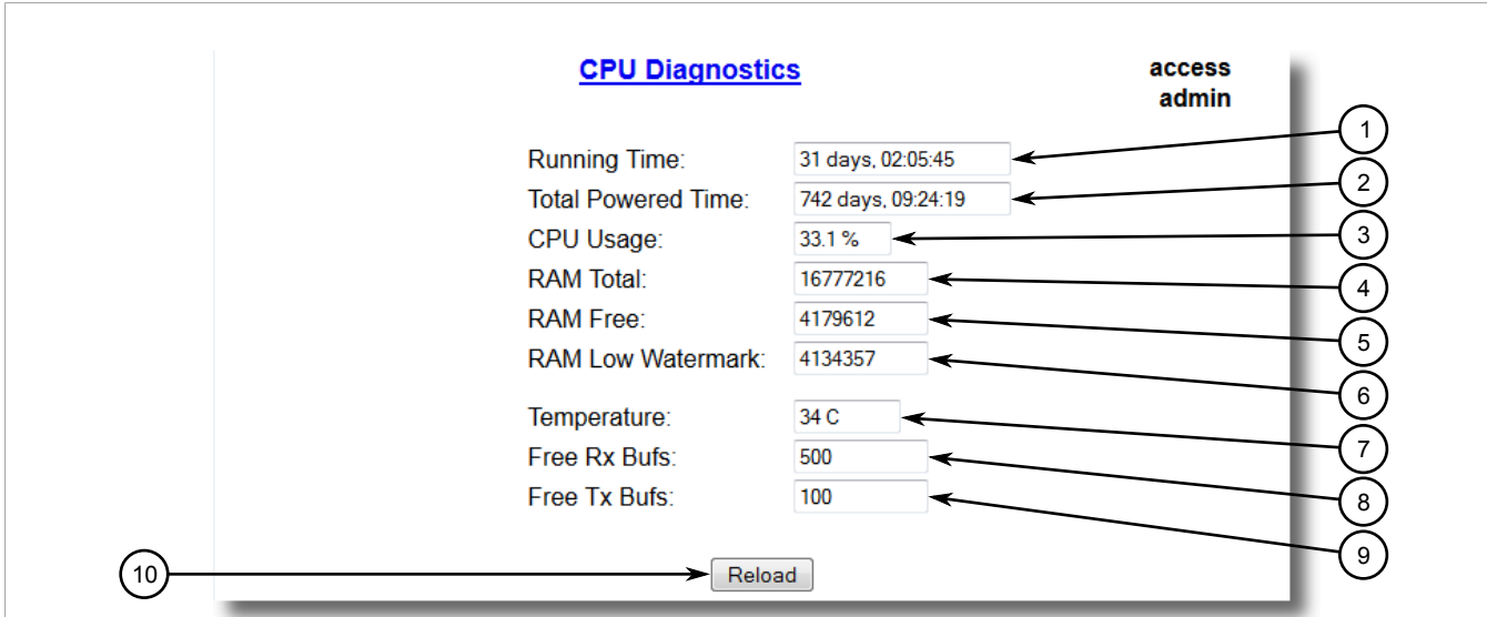
Figure 9 : Formulaire CPU Diagnostics
