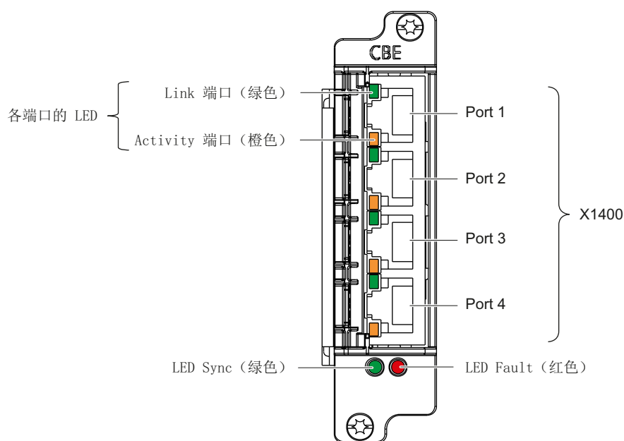
图 9-23 以太网通讯板 CBE30-2
