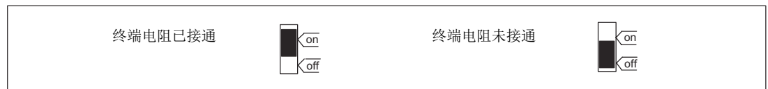
图 7-10 终端电阻接通或断开
