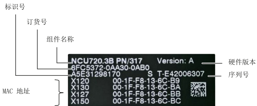
图 3-3 PROFINET/以太网接口的 MAC 地址
