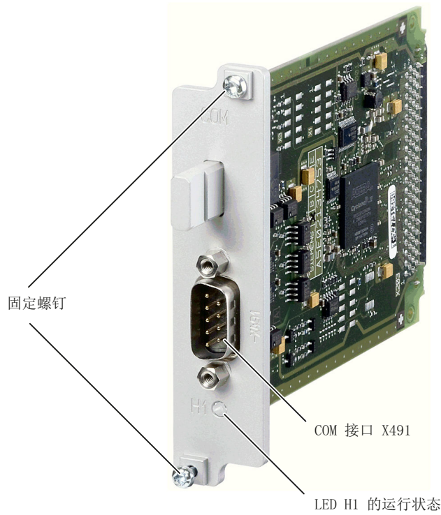
图 9-20 COM01.3 RS 232C (V.24) 模块
