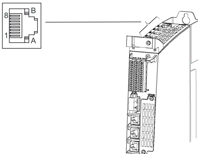
图 7-4 DRIVE-CLiQ 接口
