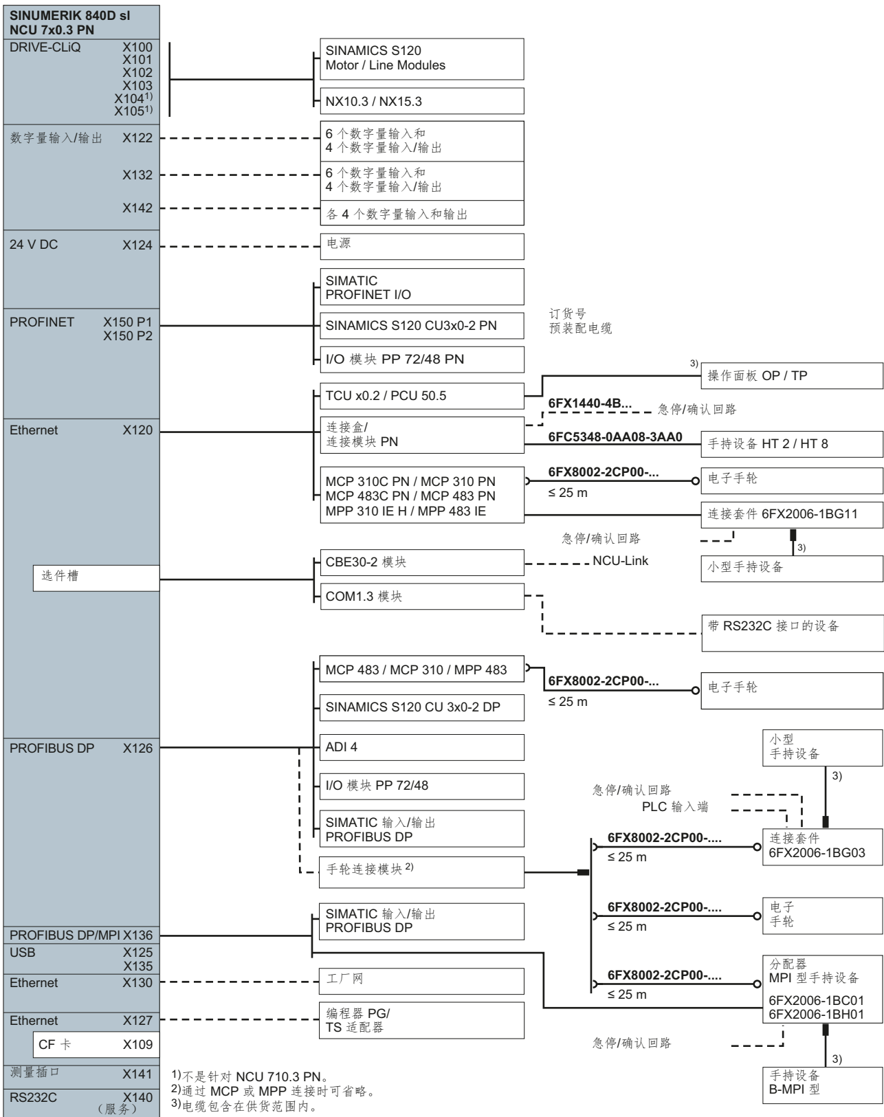
图 7-1 NCU 的接线方式
