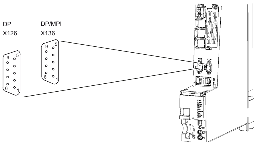
图 7-9 PROFIBUS DP/MPI 接口
