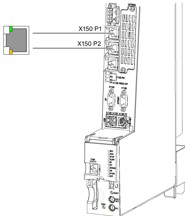
图 7-6 PROFINET 接口
