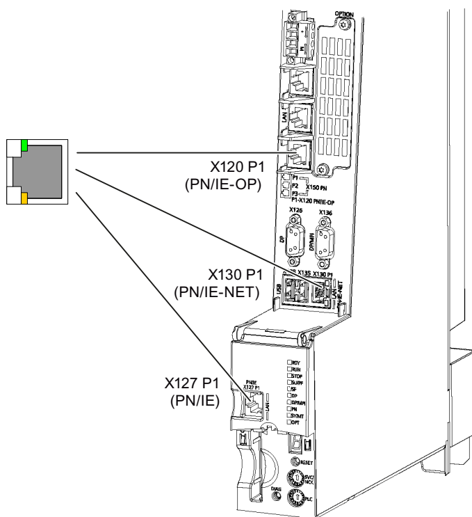
图 7-5 以太网接口
