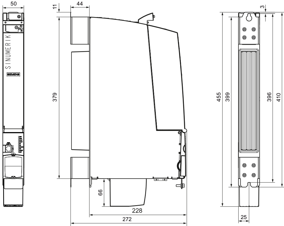
图 5-1 NCU 720.3 PN 和 NCU 730.3 PN 的尺寸图；单位为 mm
