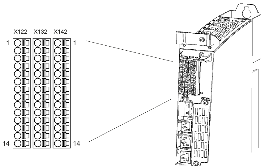
图 7-11 数字量输入/输出端（接口 X122、X132 和 X142）
