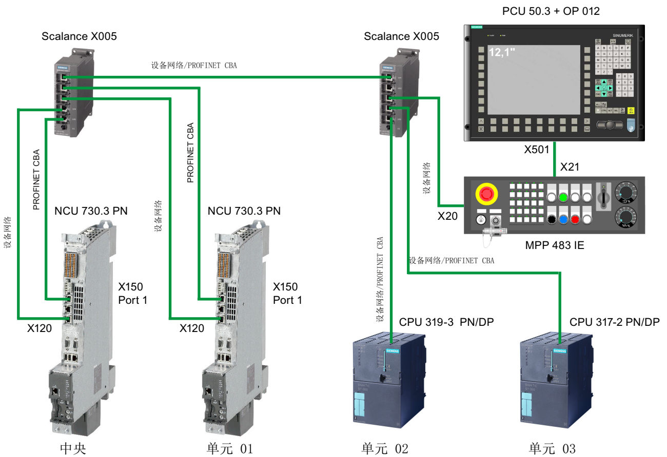
图 7-8 PROFINET CBA 的配置示例
