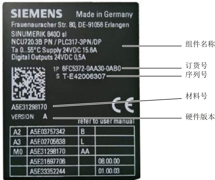
图 3-2 铭牌
