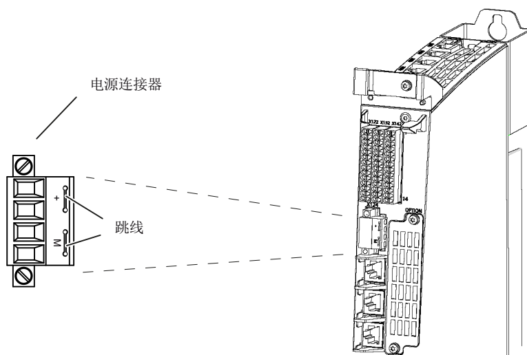
图 7-3 电源接口
