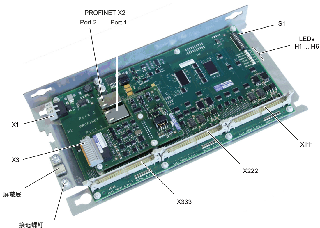
图 9-13 输入/输出模块 PP 72/48D 2/2A PN
