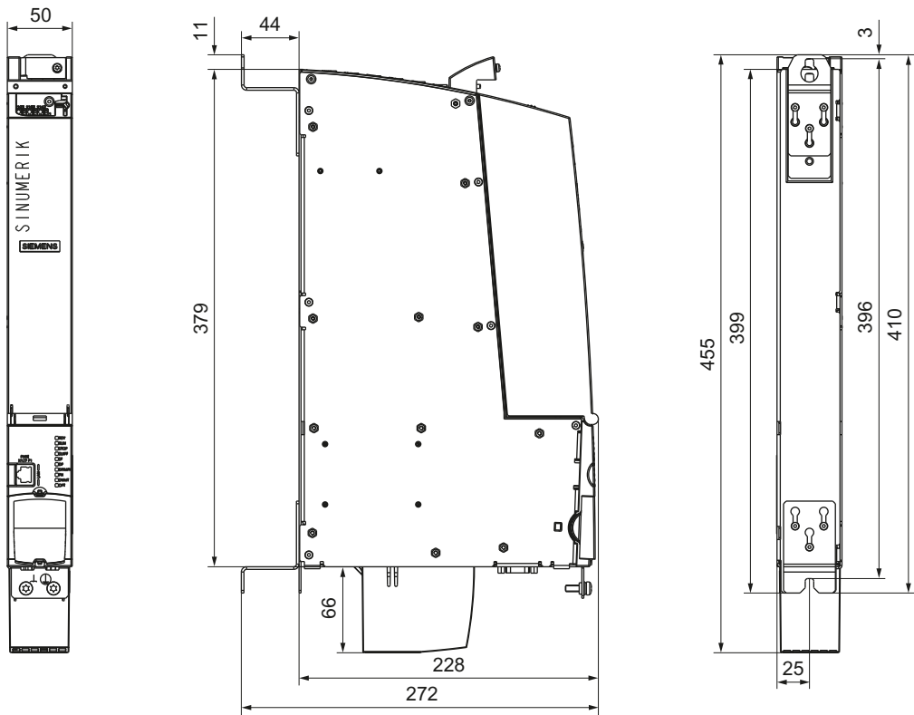
图 5-2 NCU 710.3 PN, NCU 710.3B PN, NCU 720.3B PN 和 NCU 730.3B PN 的尺寸图；单位为 mm
