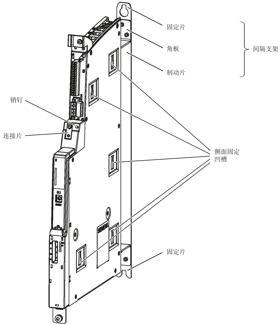
图 9-4 NX 模块的安装辅助装置
