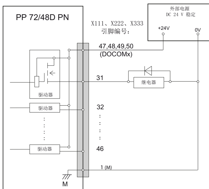
图 9-12 数字量输出端的接线图
