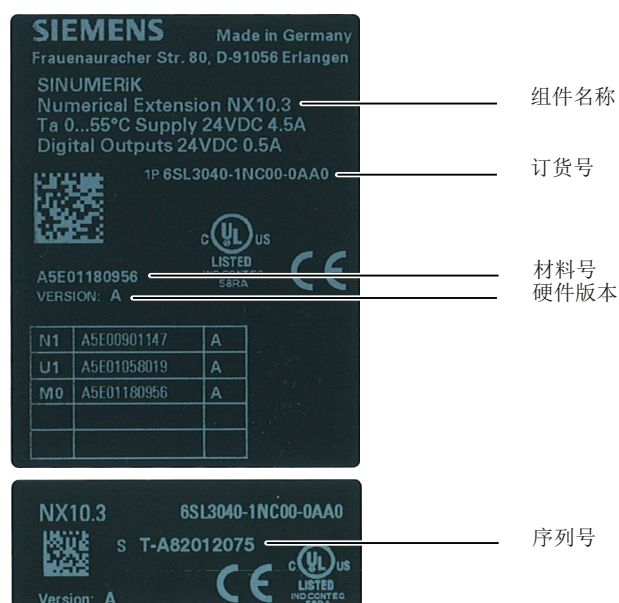
图 9-2 NX10.3（示例）上的铭牌
