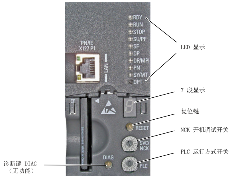
图 3-4 操作和显示单元的位置
