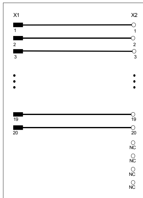
Bild 8-18 Schaltbild SU11
