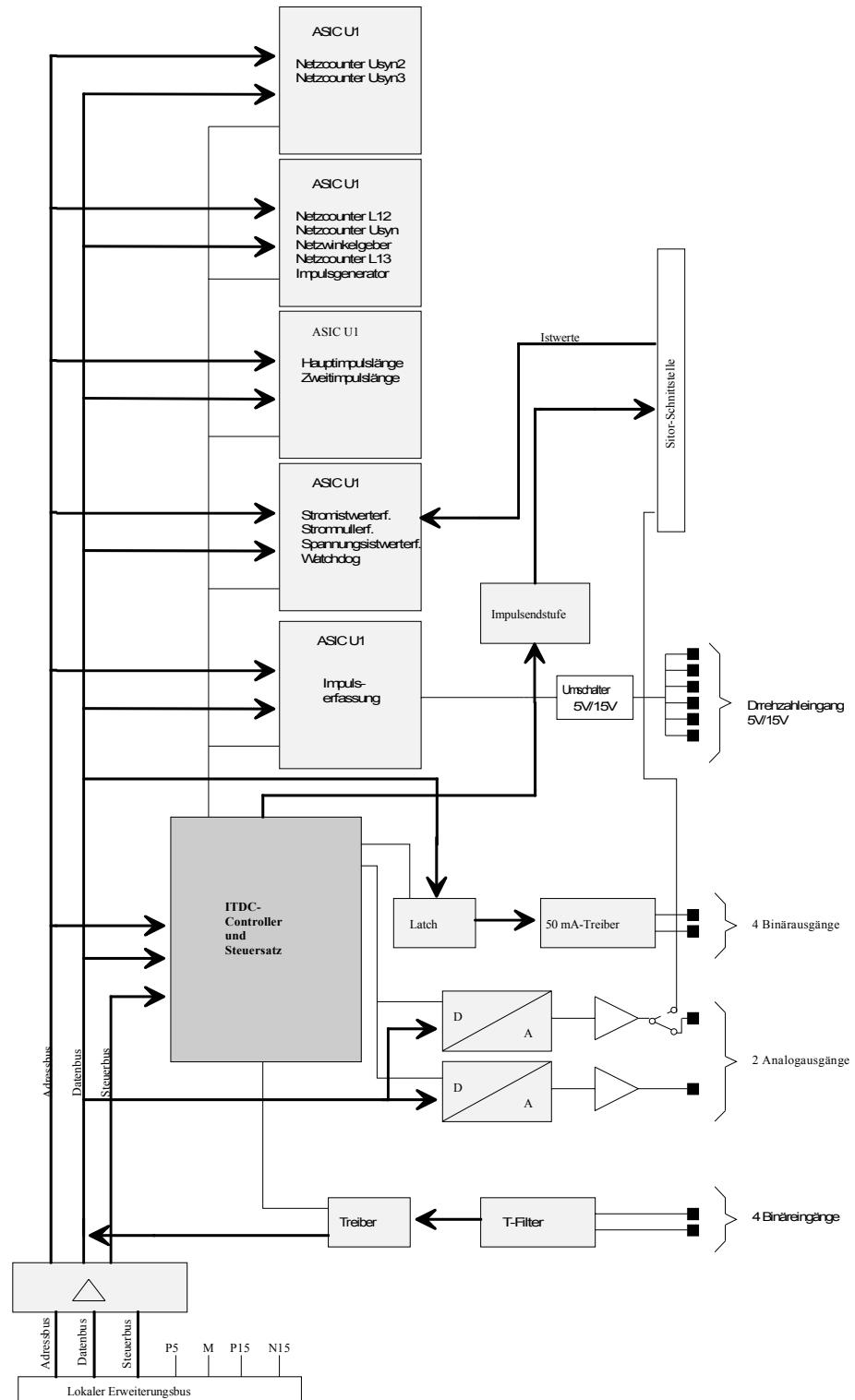
Bild 5-11 Blockschaltbild ITDC
