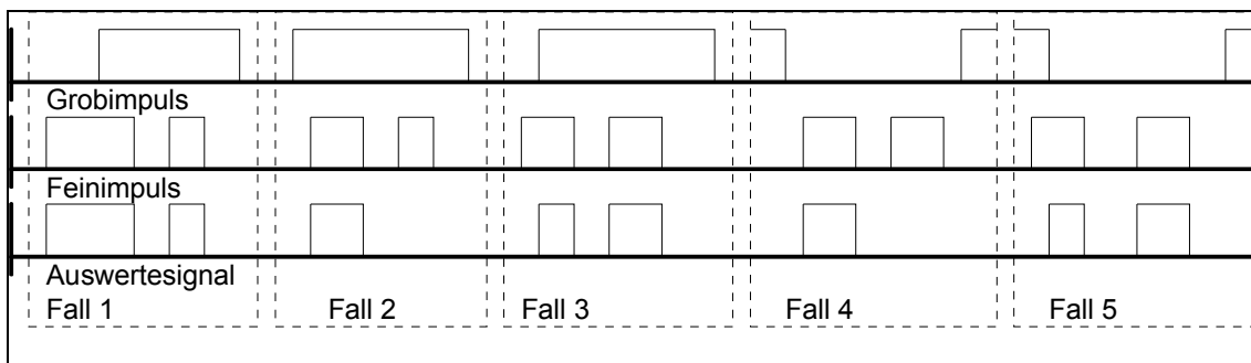
Bild 7-1 Grob- und Feinimpulsauswertung
