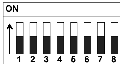
Bild 7-3 Schalter S1
