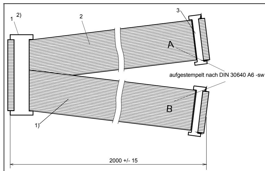
Bild 9-6 Flachleitung SC55
