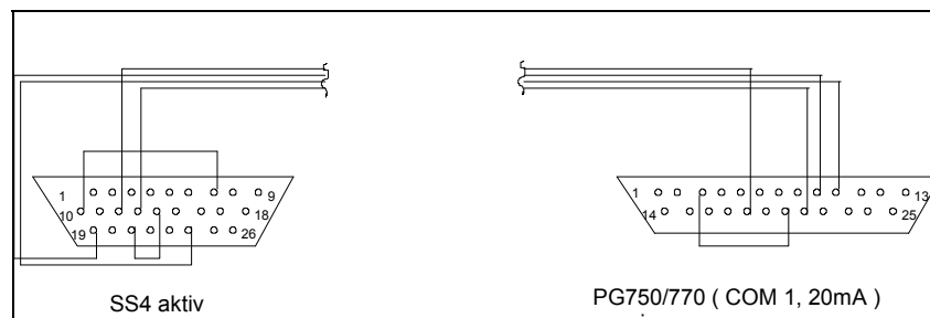
Bild 6-9 SS4 an PG750/770 ( COM1 ) über die 20mA-Schnittstelle (aktiv)
