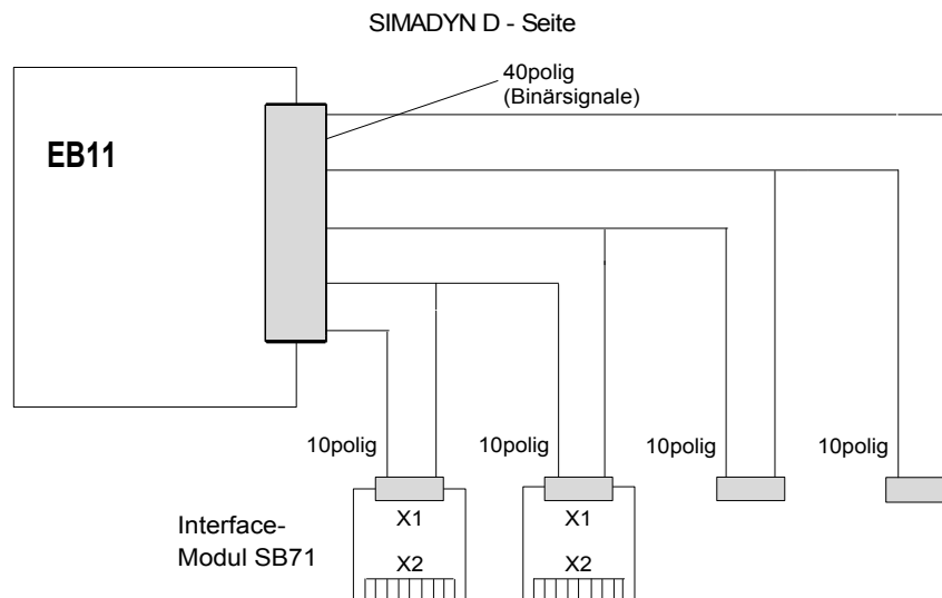
Bild 8-15 Applikationsbeispiel für Interfacemodul SB71 an binäre Ein-, Ausgabebaugruppe EB11
