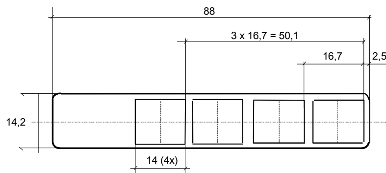
Bild 10-4 Maßbild Beschriftungsstreifen
