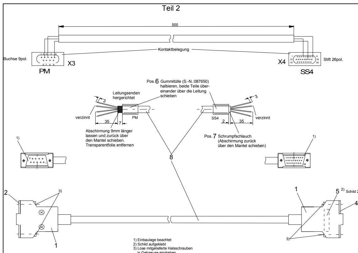
Bild 9-7 Flachleitung SC57
