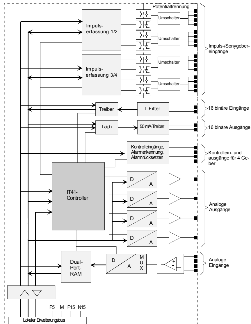
Bild 5-3 Blockschaltbild der IT41
