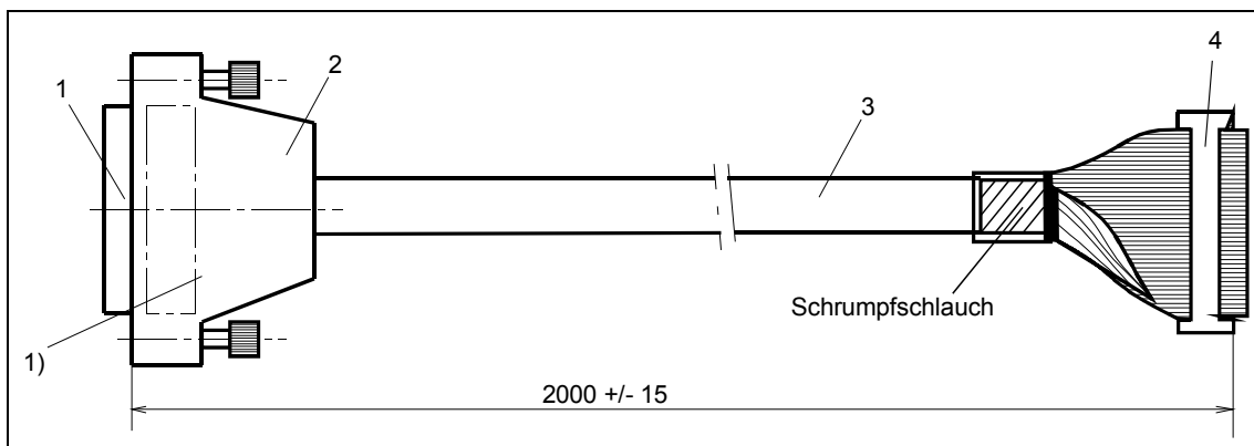
Bild 9-4 Rundleitung SC51
