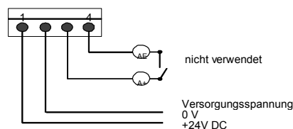
Anschlüsse am Klemmenblock
