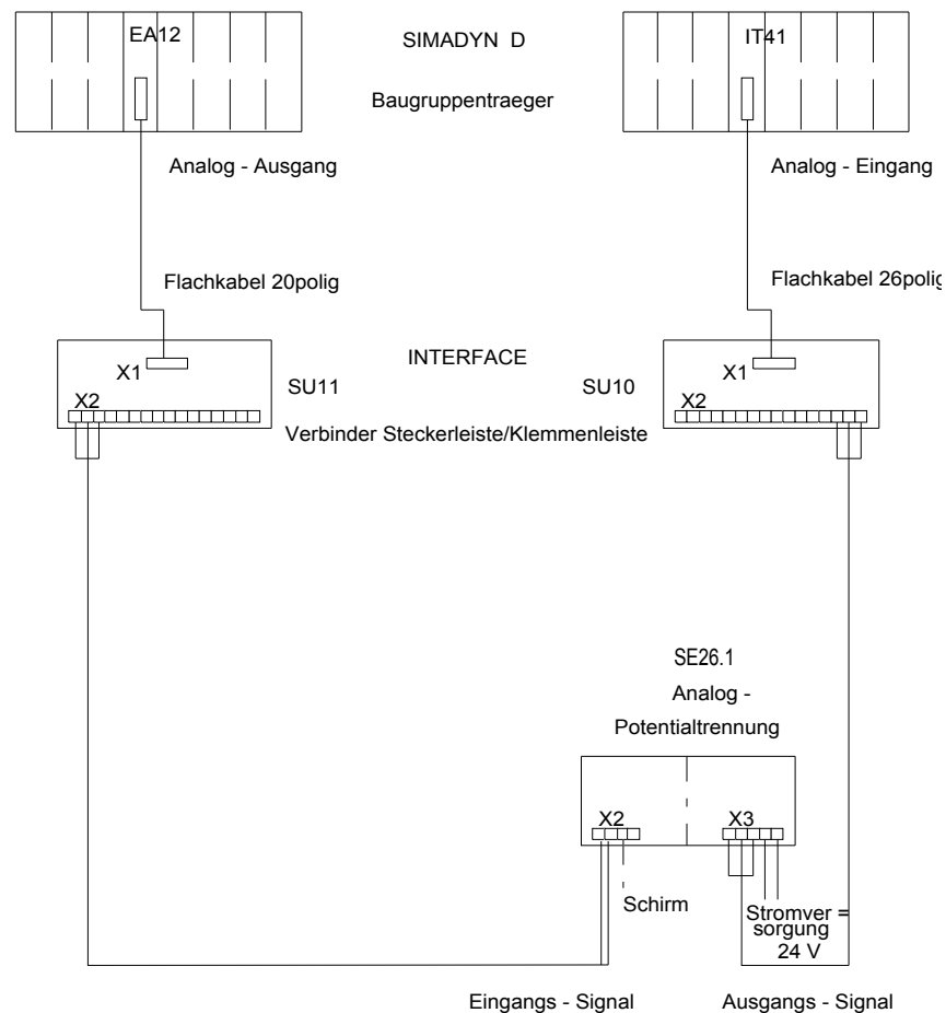
Bild 8-3 Anschlussbeispiel für das Interfacemodul SE26.1
