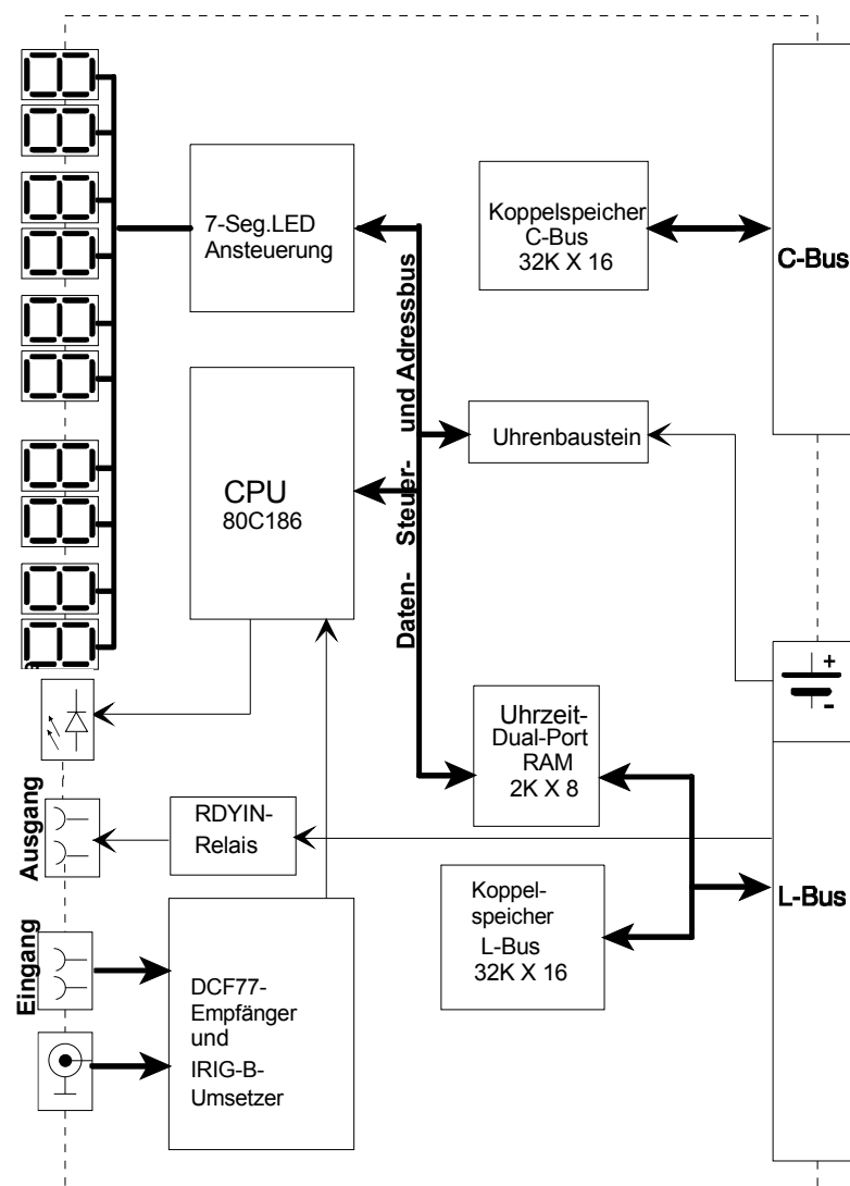
Bild 4-1 Blockschaltbild MM3
