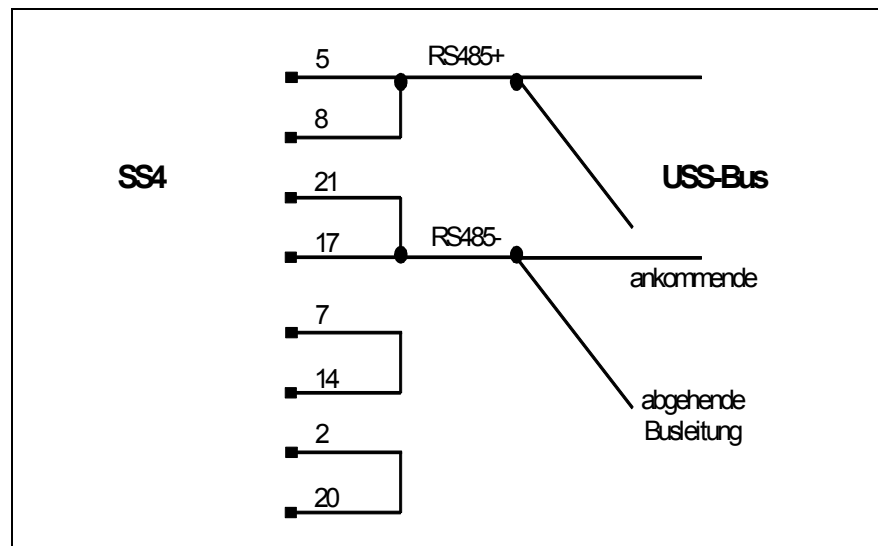
Bild 6-14 SS4-Steckerbelegung ohne Busabschluß (SS4 in der Mitte der Busleitung)
