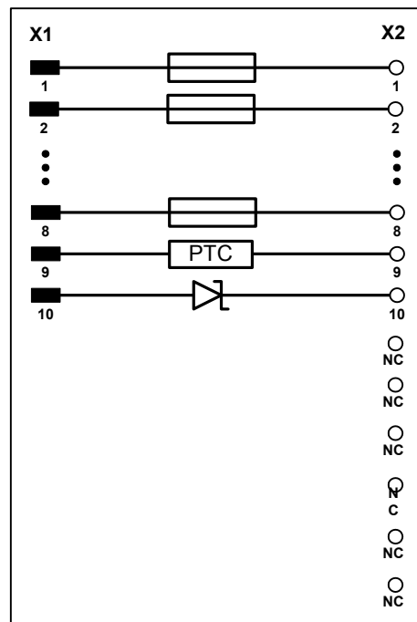
Bild 8-19 Schaltbild SU12
