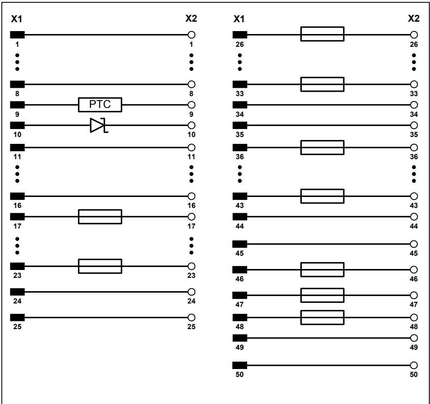
Bild 8-20 Schaltbild SU13
