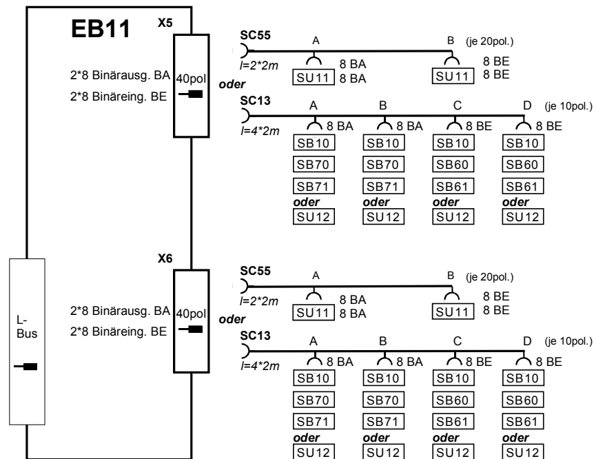
Bild 5-2 Anschlußmöglichkeiten von Leitungen und Interfacemodulen
