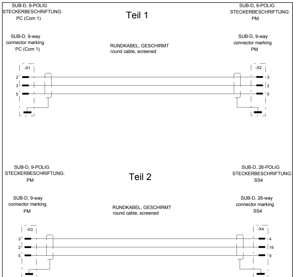
Bild 9-8 Flachleitung SC57
