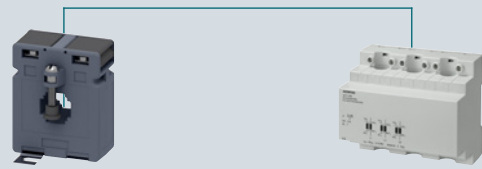
4NC Stromwandler
