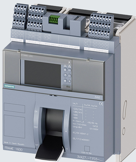
Kompaktleistungsschalter 3VA27
