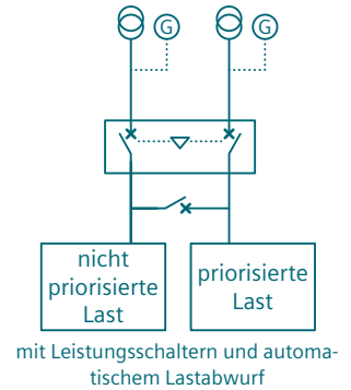
mit Leistungsschaltern
