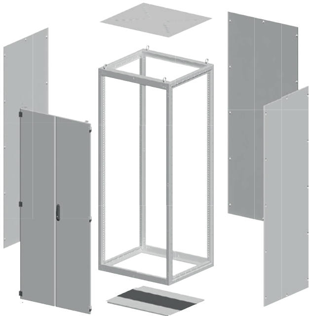
2 Tür, Türhälfte
