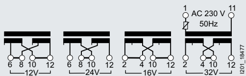
5 TE
