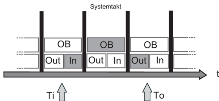
Bild 5-10 Systemtakt
