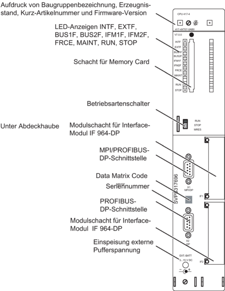
Bild 2-6 Anordnung der Bedien- und Anzeigeelemente der CPU 417-4
