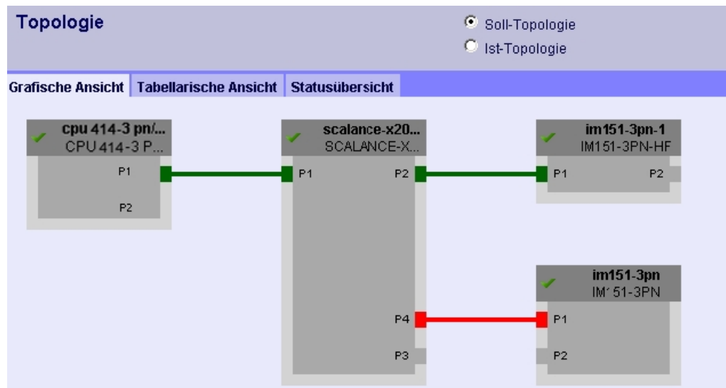
Bild 4-26 "Soll-Topologie" mit vertauschten Ports
