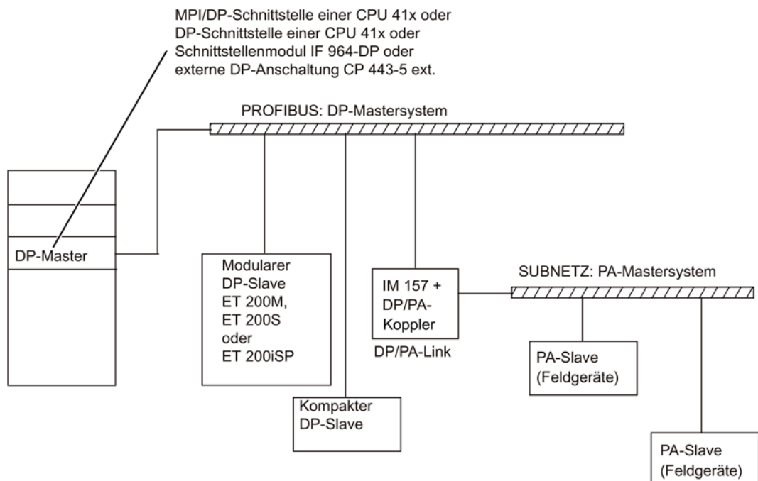
Bild 3-1 Übersicht: Systemstruktur für Anlagenänderungen im laufenden Betrieb
