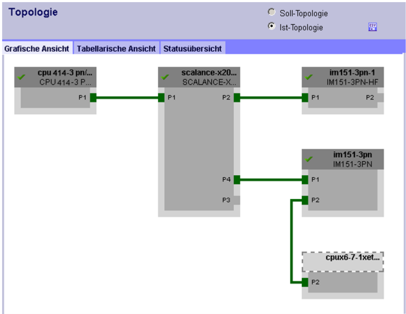
Bild 4-22 "Ist-Topologie" in Ordnung
