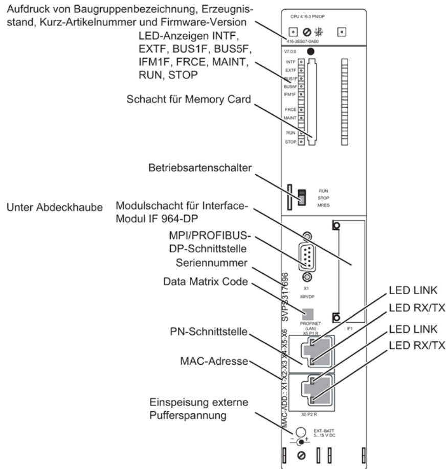
Bild 2-5 Anordnung der Bedien- und Anzeigeelemente der CPU 41x-3 PN/DP
