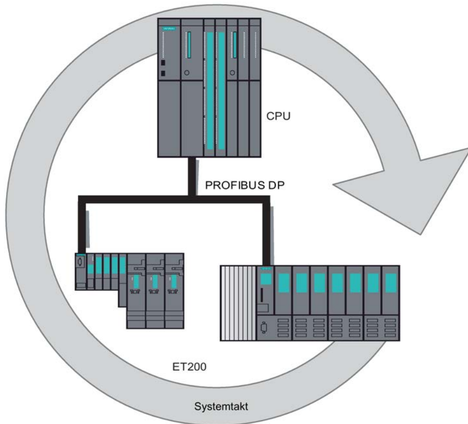
Bild 5-9 Just-In-Time
