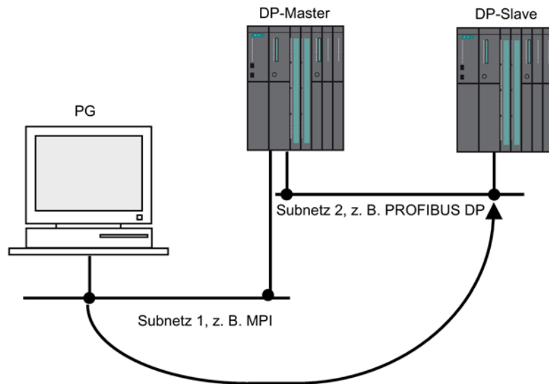
Bild 4-1 S7-Routing
