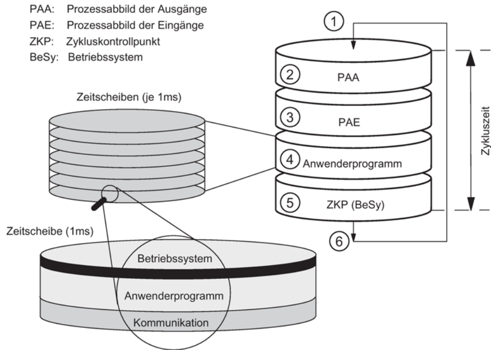
Bild 9-1 Teile und Zusammensetzung der Zykluszeit
