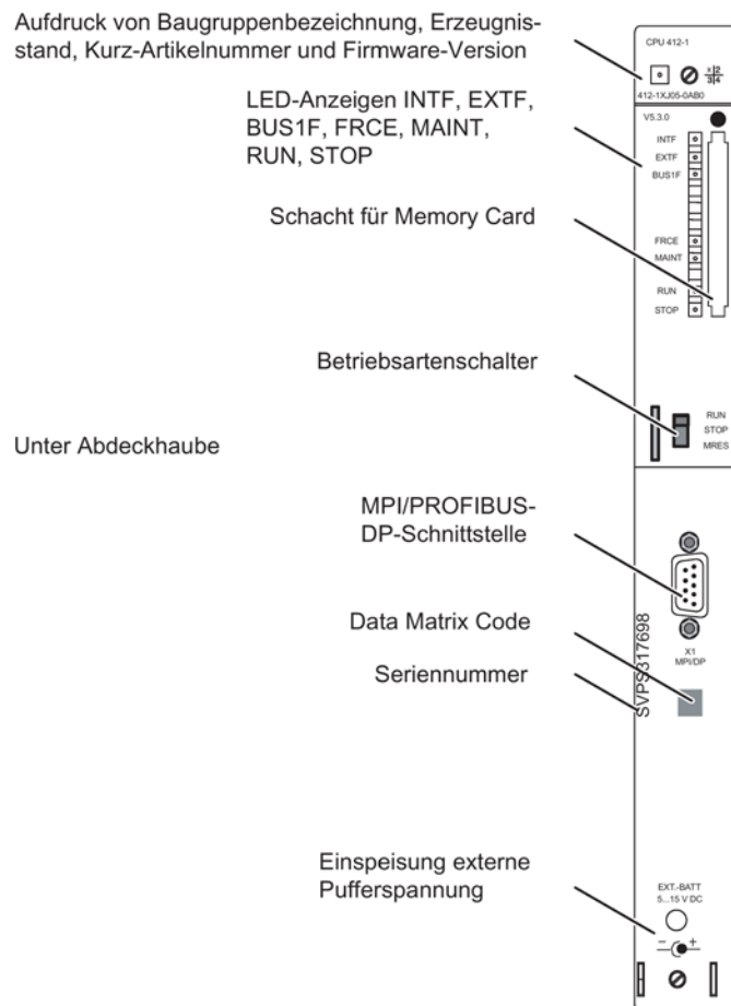
Bild 2-1 Anordnung der Bedien- und Anzeigeelemente der CPU 412-1
