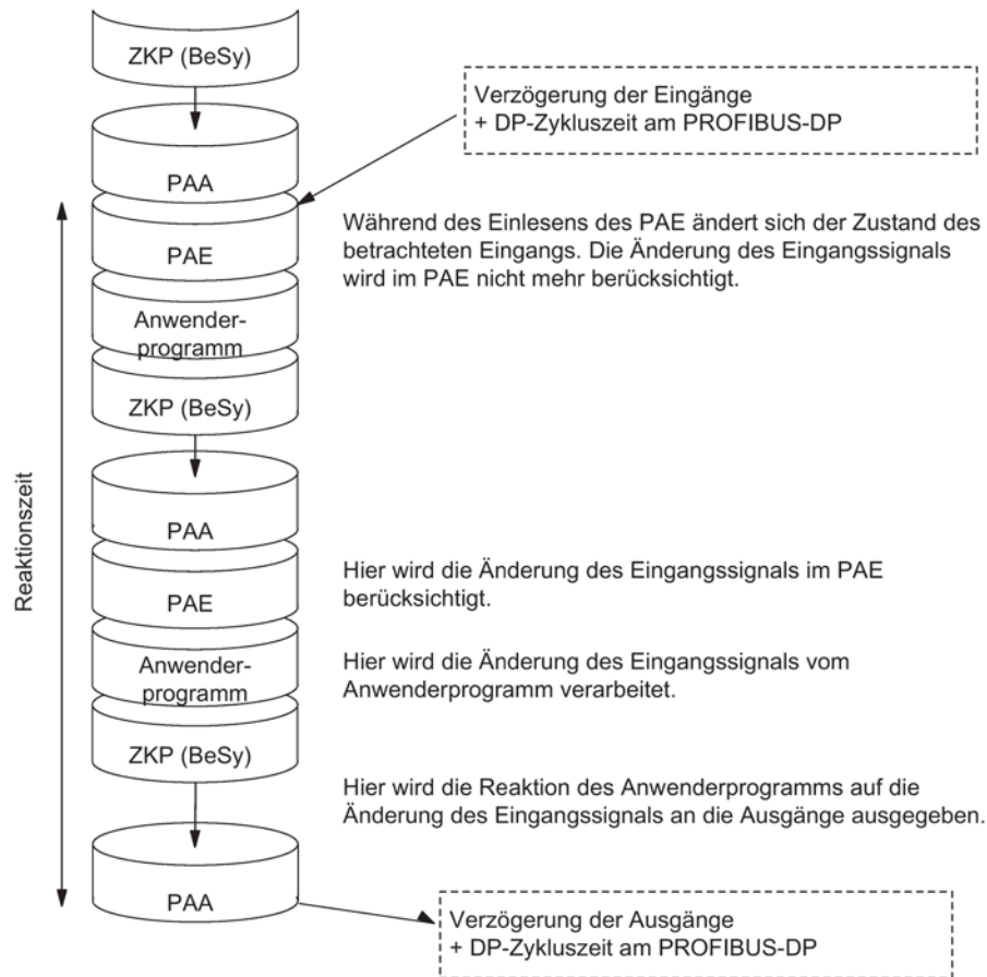
Bild 9-10 Längste Reaktionszeit
