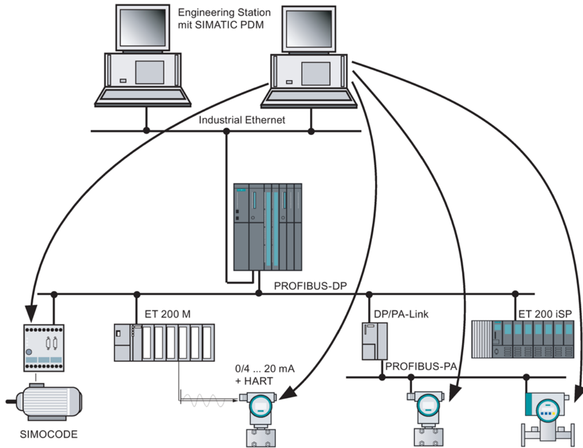
Bild 4-4 Datensatz-Routing
