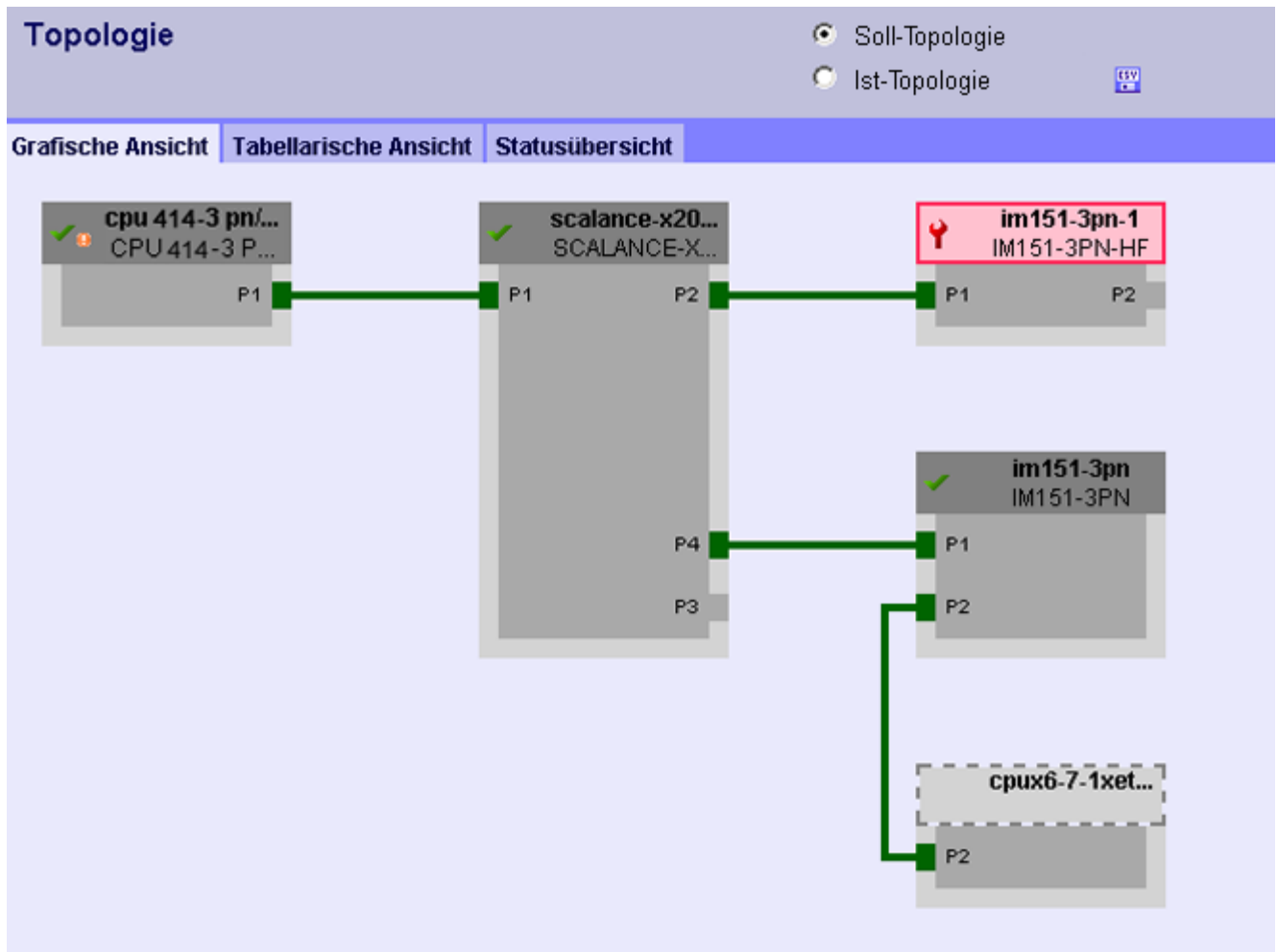
Bild 4-24 "Soll-Topologie" mit ausgefallenem Gerät
