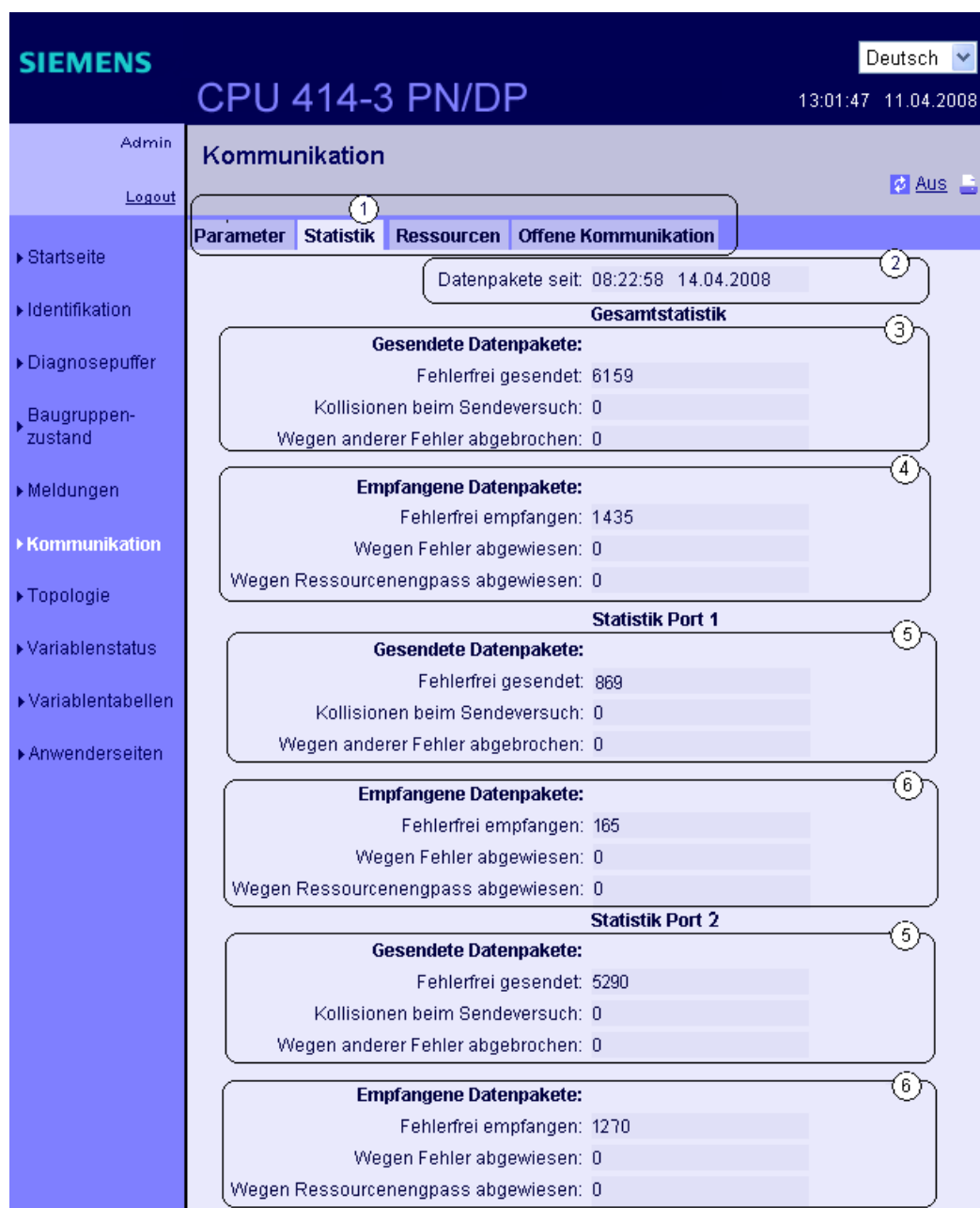
Bild 4-18 Kennzahlen zur Datenübertragung
