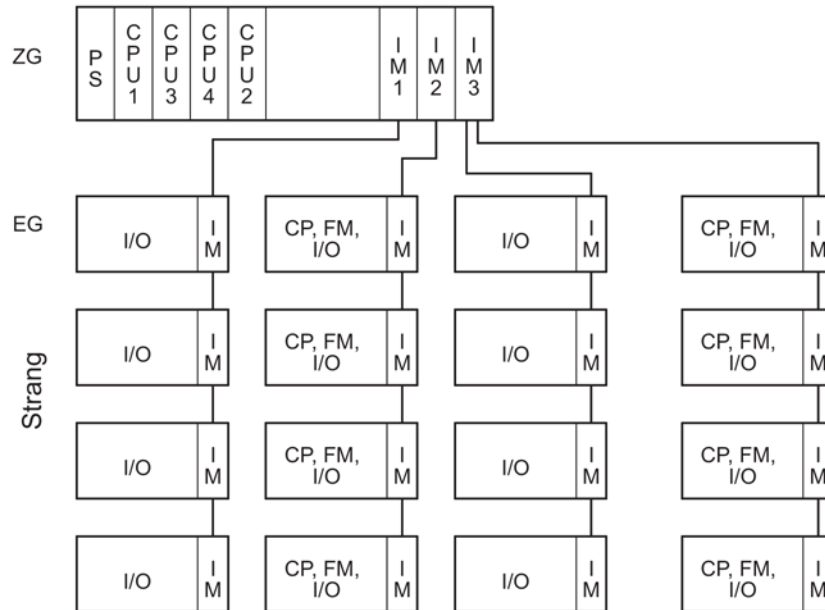
Bild 3-2 Beispiel für Multicomputing
