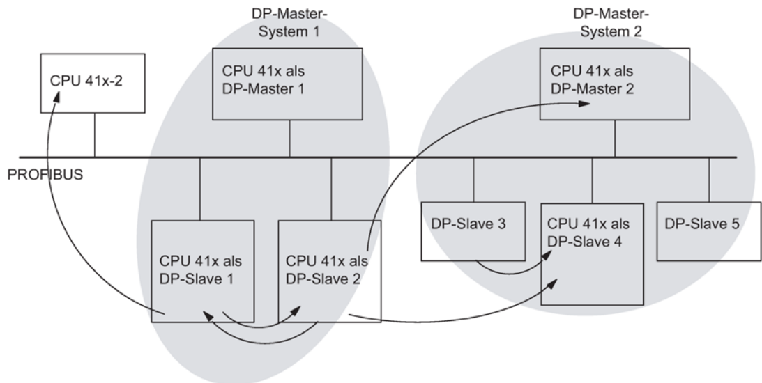
Bild 5-7 Direkter Datenaustausch mit CPUs 41x
