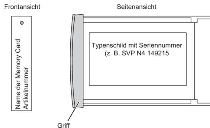
Bild 2-9 Aufbau der Memory Card
