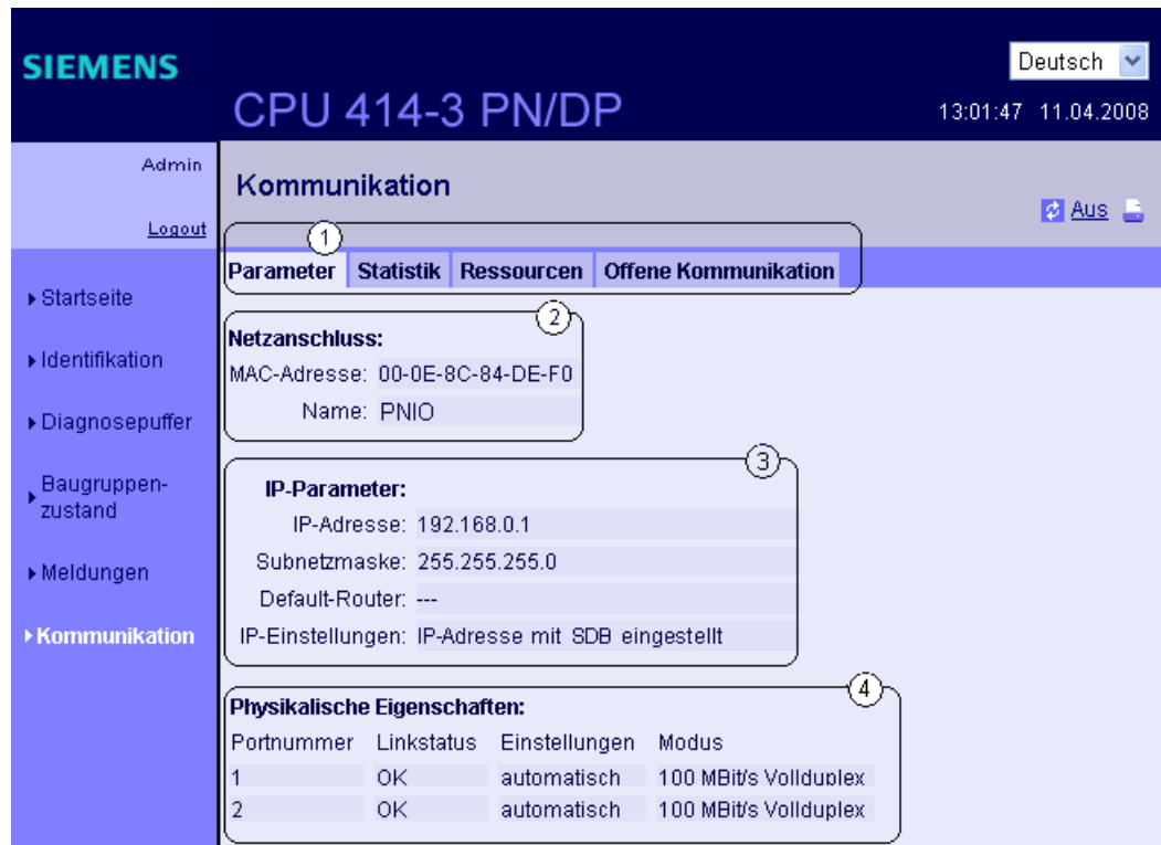
Bild 4-17 Parameter der integrierten PROFINET-Schnittstelle
