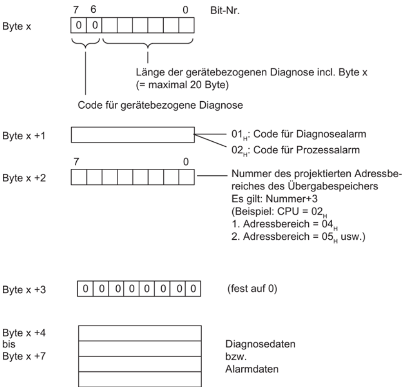
Bild 5-5 Aufbau der gerätebezogenen Diagnose
