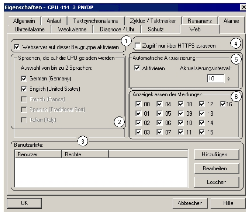
Bild 4-6 Einstellungen in HW-Konfig
