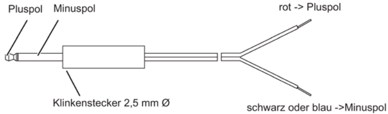
Bild 2-7 Anschlusskabel mit Klinkenstecker
