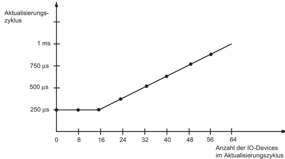
Bild 9-8 Aktualisierungszyklus
