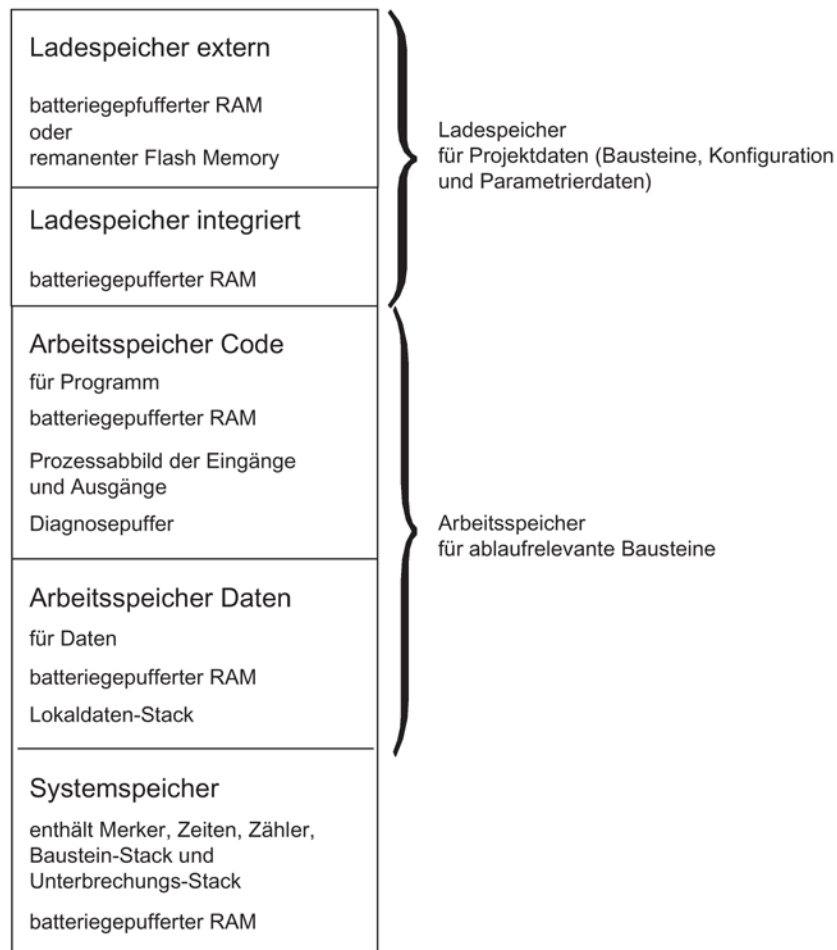
Bild 8-1 Speicherbereiche der S7-400 CPUs
