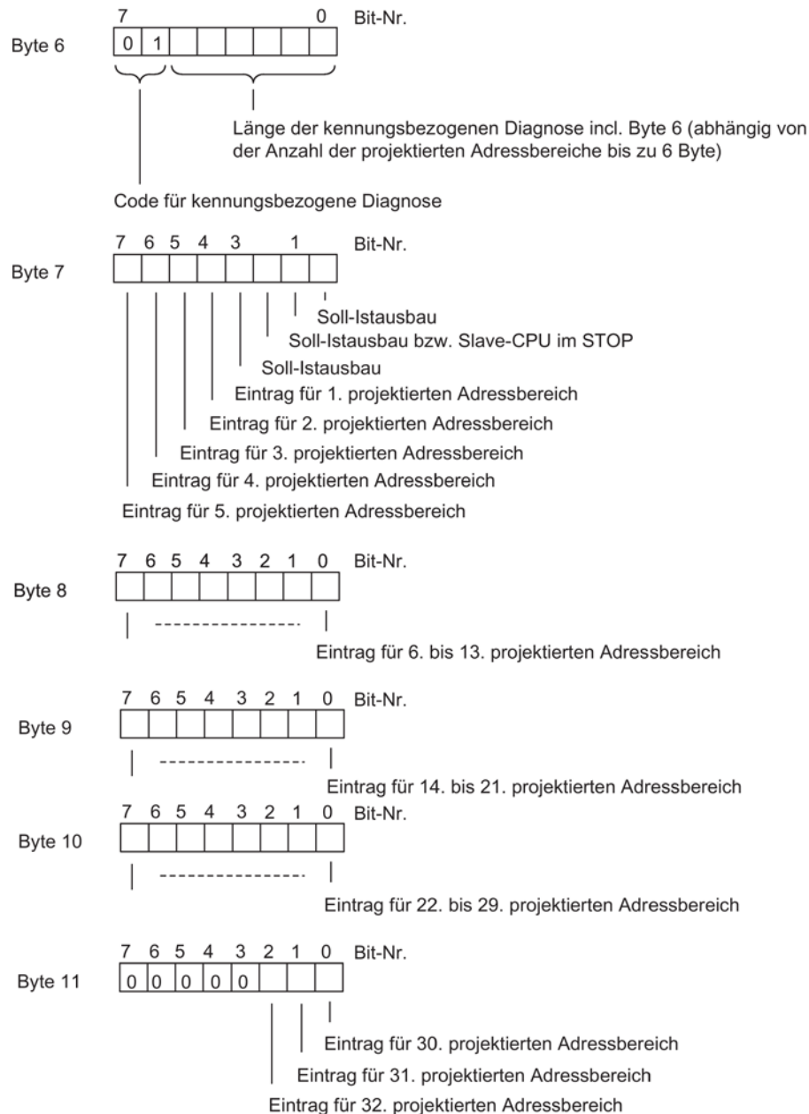
Bild 5-4 Aufbau der kennungsbezogenen Diagnose der CPU 41x
