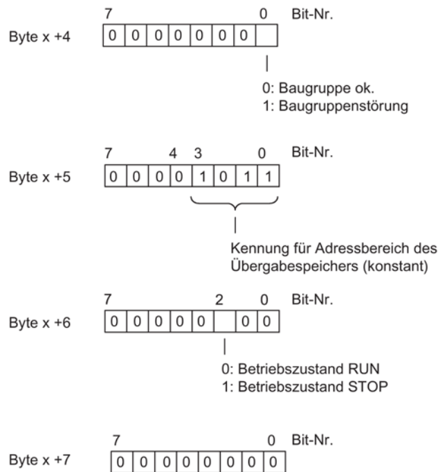
Bild 5-6 Byte x +4 bis x +7 für Diagnose- und Prozessalarm
