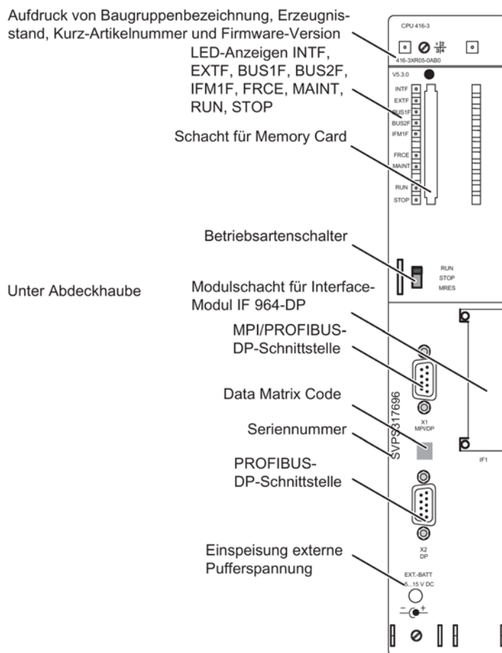
Bild 2-4 Anordnung der Bedien- und Anzeigeelemente der CPU 41x-3
