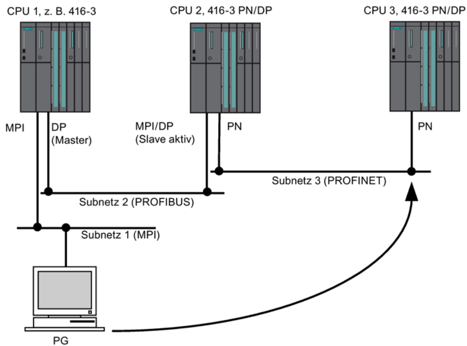
Bild 4-2 S7-Routing-Netzübergänge: MPI-DP-PROFINET
