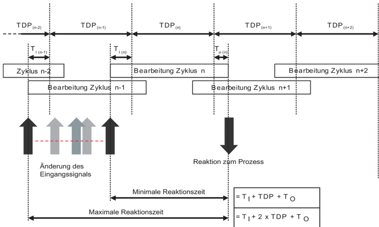
Bild 5-8 Taktsynchrone Datenverarbeitung
