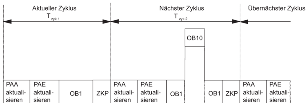
Bild 9-2 Unterschiedliche Zykluszeiten
