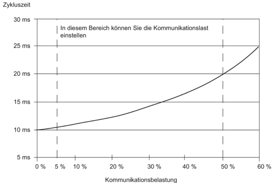
Bild 9-6 Abhängigkeit der Zykluszeit von der Kommunikationslast
