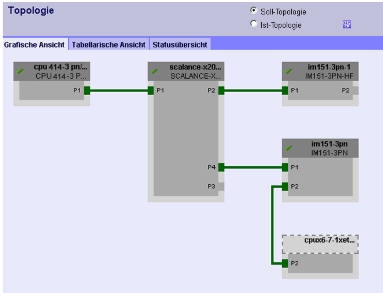
Bild 4-23 "Soll-Topologie" in Ordnung
