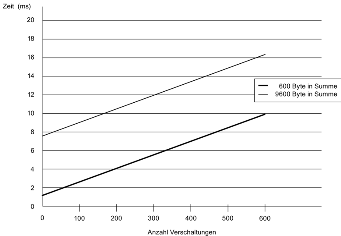
Bild 9-11 Verarbeitungszeit zum Senden und Empfangen
