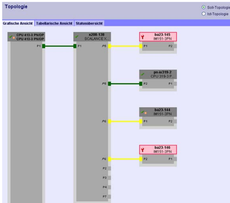
Bild 4-27 "Soll-Topologie" mit Werkzeugwechsel
