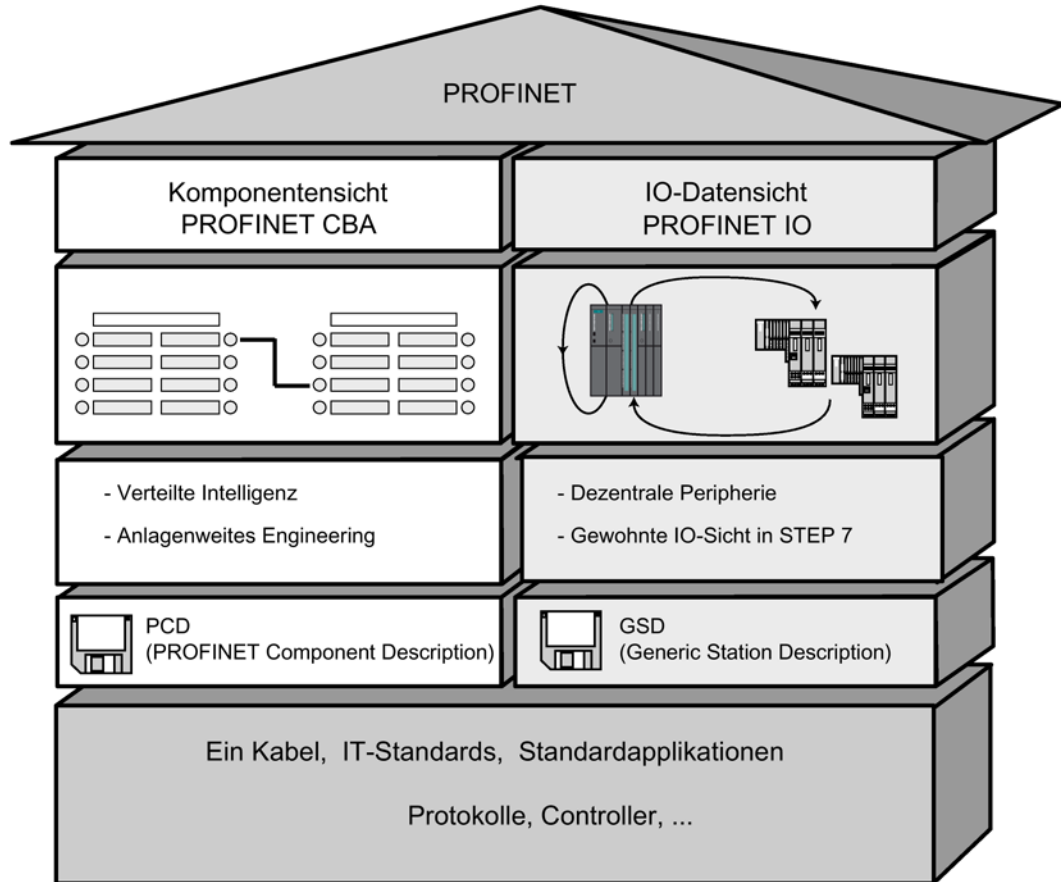
Bild 6-1 PROFINET IO und PROFINET CBA
