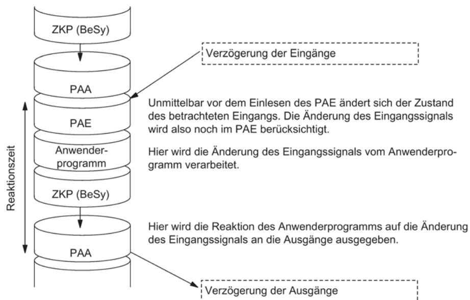
Bild 9-9 Kürzeste Reaktionszeit
