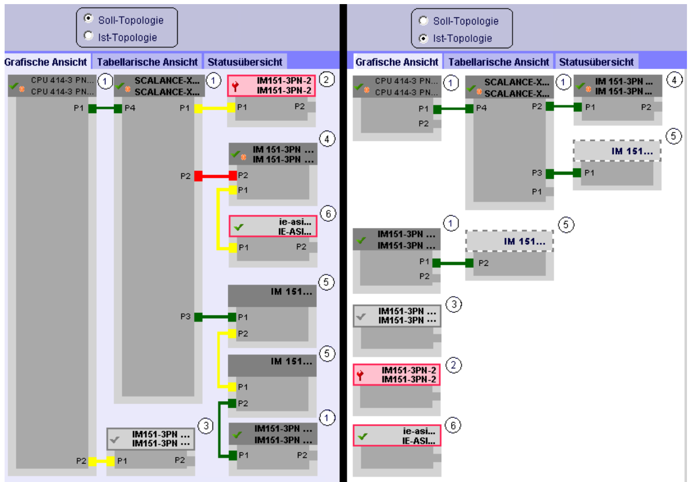
Bild 4-19 Topologie - Grafische Ansicht
