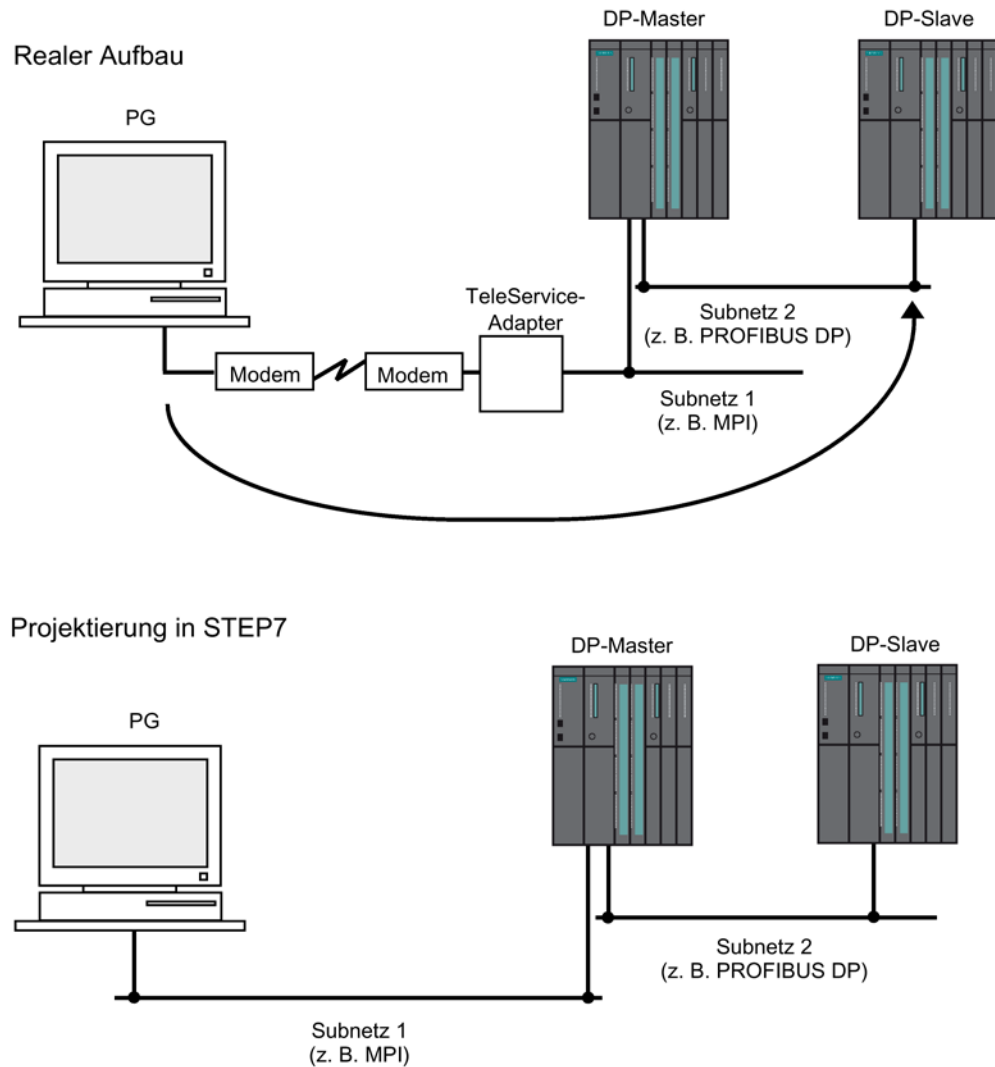
Bild 4-3 S7-Routing: Applikationsbeispiel TeleService
