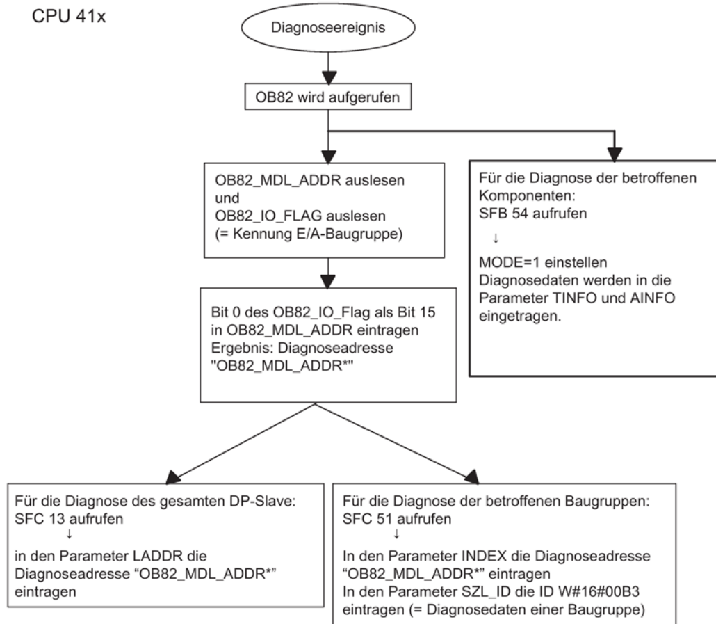
Bild 5-1 Diagnose mit CPU 41x
