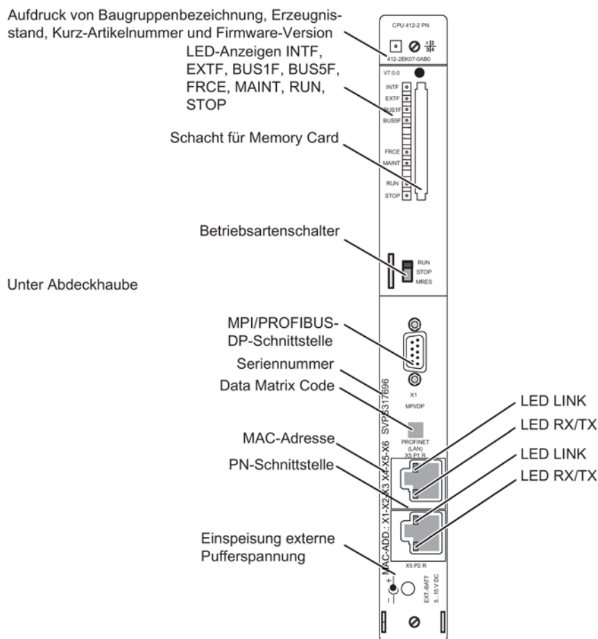
Bild 2-2 Anordnung der Bedien- und Anzeigeelemente der CPU 412-2 PN
