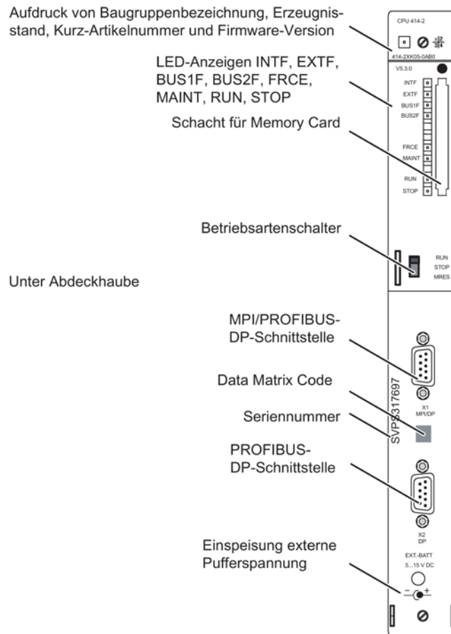
Bild 2-3 Anordnung der Bedien- und Anzeigeelemente der CPU 41x-2
