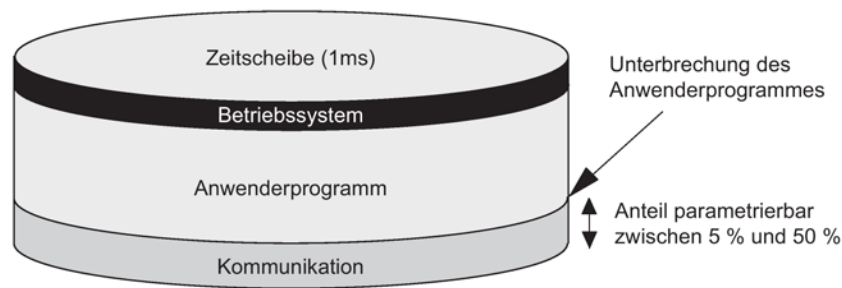
Bild 9-5 Aufteilung einer Zeitscheibe
