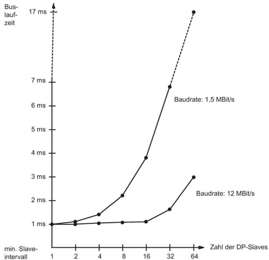
Bild 9-7 DP-Zykluszeiten im PROFIBUS DP-Netz
