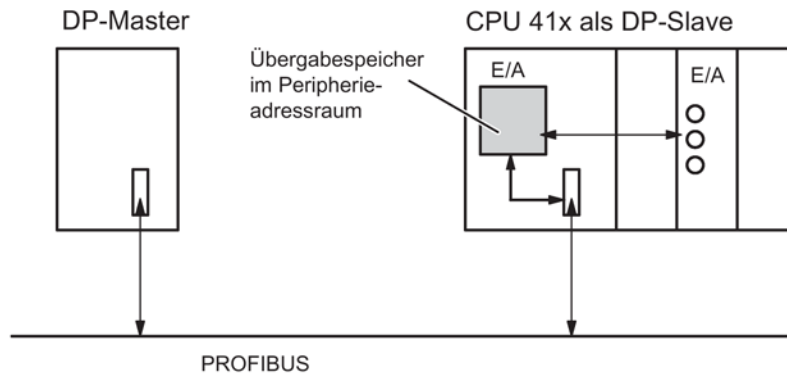
Bild 5-2 Übergabespeicher in der CPU 41x als DP-Slave
