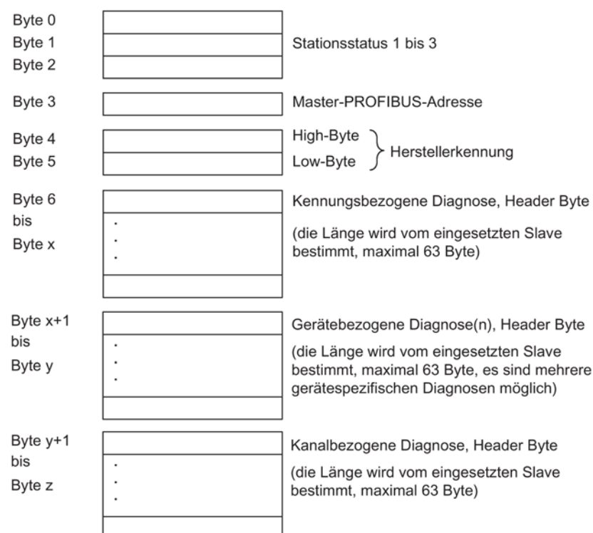
Bild 5-3 Aufbau einer Slave-Diagnose
