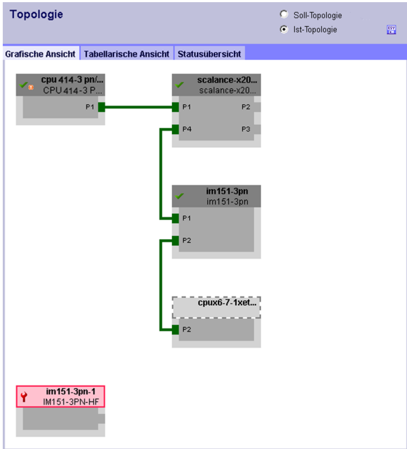
Bild 4-25 "Ist Topologie" mit ausgefallenem Gerät
