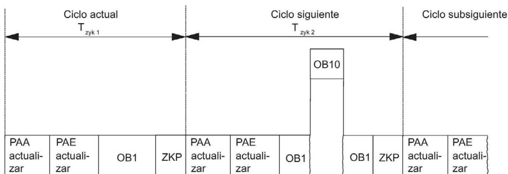
Figura 9-2 Tiempos de ciclo diferentes
