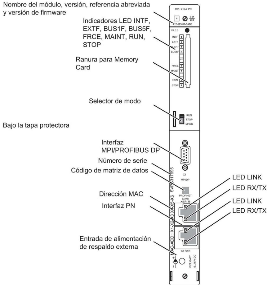
Figura 2-2 Disposición de los elementos de mando e indicadores de la CPU 412-2 PN
