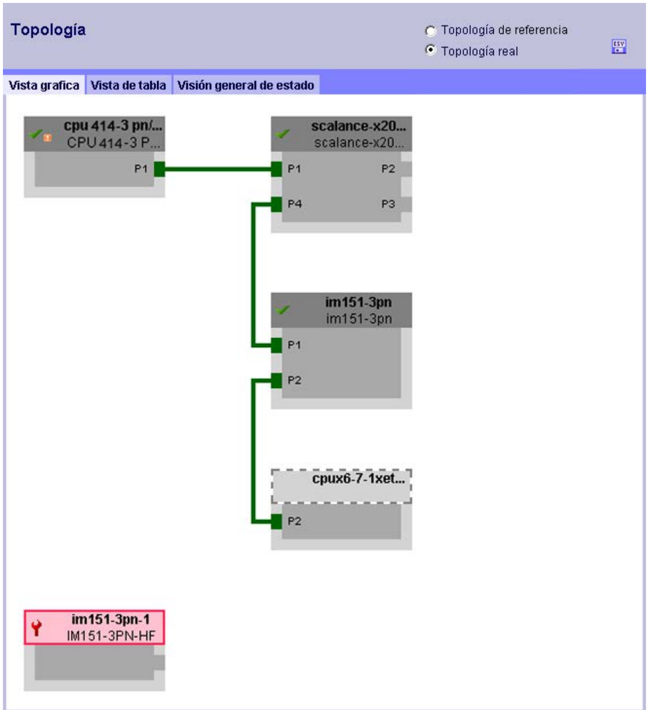
Figura 4-25 "Topología real" con dispositivo que falla
