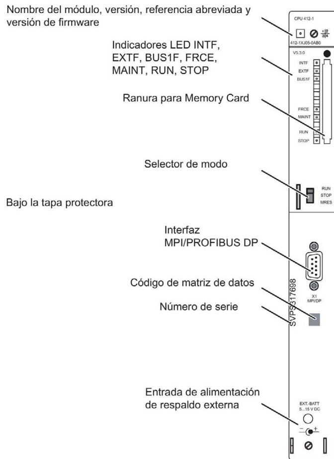
Figura 2-1 Disposición de los elementos de mando e indicadores de la CPU 412-1
