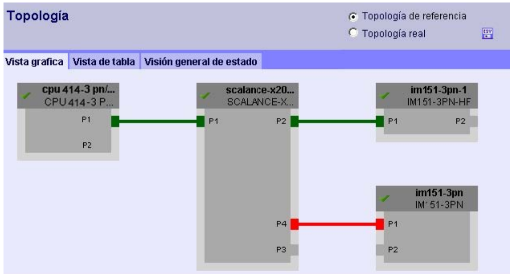
Figura 4-26 "Topología prevista" con puertos intercambiados
