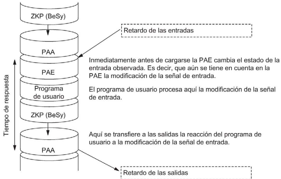
Figura 9-9 Tiempo de respuesta mínimo
