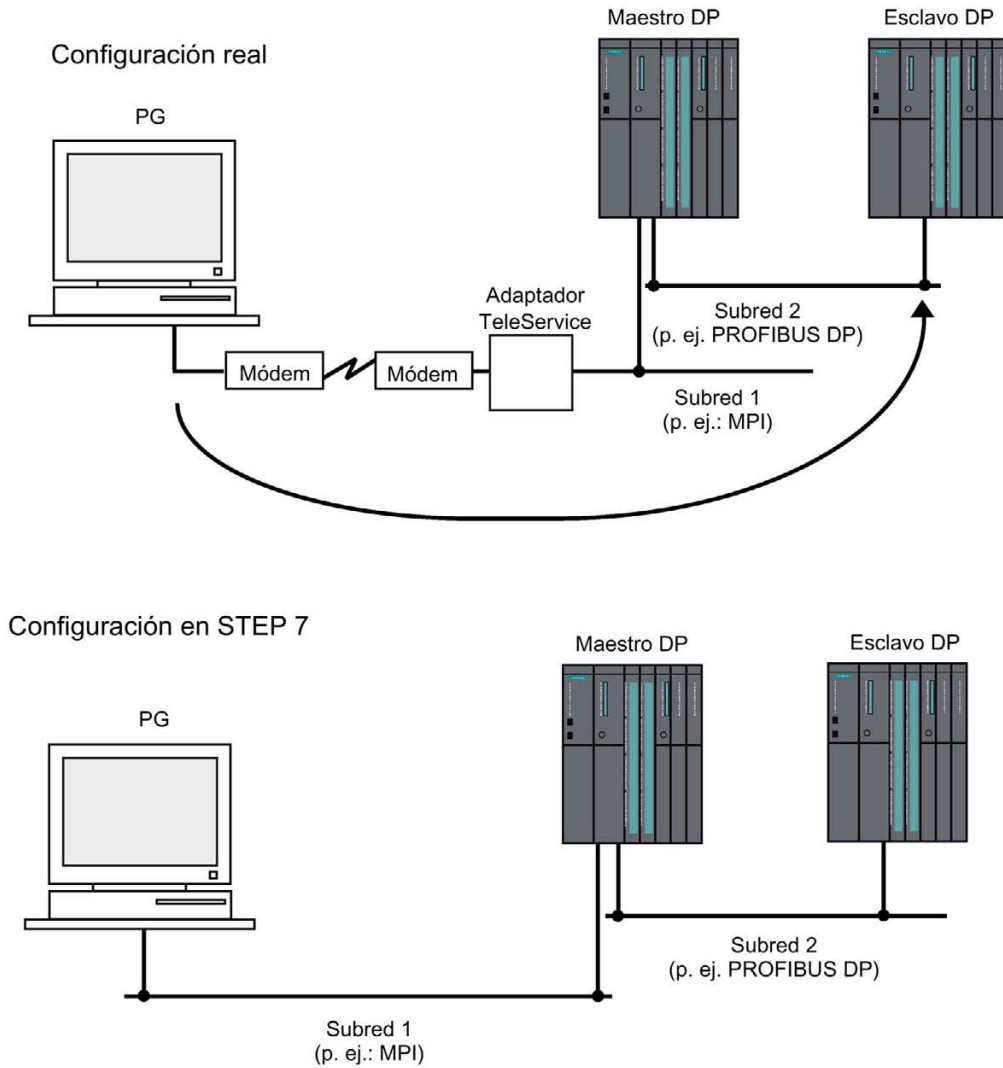
Figura 4-3 S7-Routing: Ejemplo de aplicación TeleService
