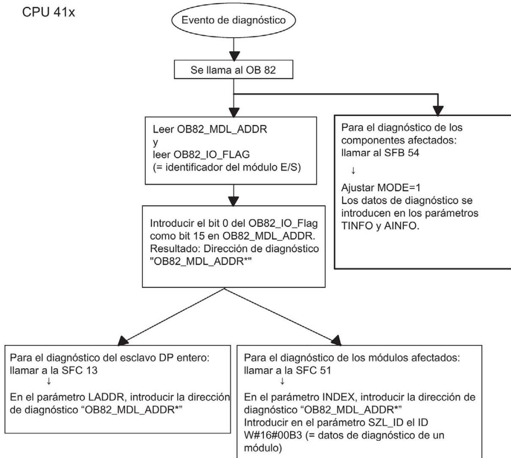
Figura 5-1 Diagnóstico con CPU 41x
