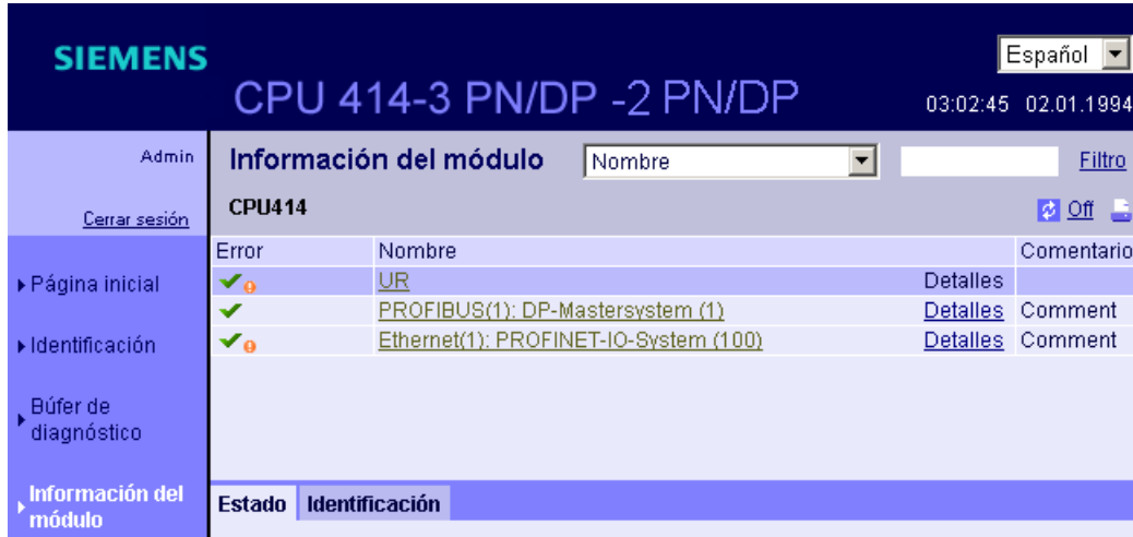
Figura 4-12 Información del módulo
