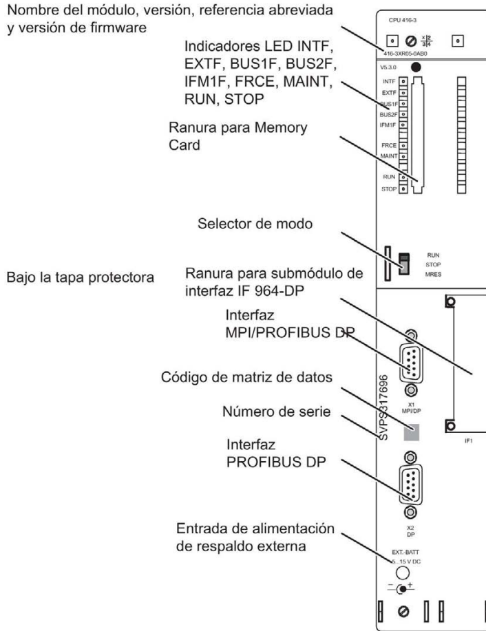
Figura 2-4 Disposición de los elementos de mando e indicadores de la CPU 41x-3
