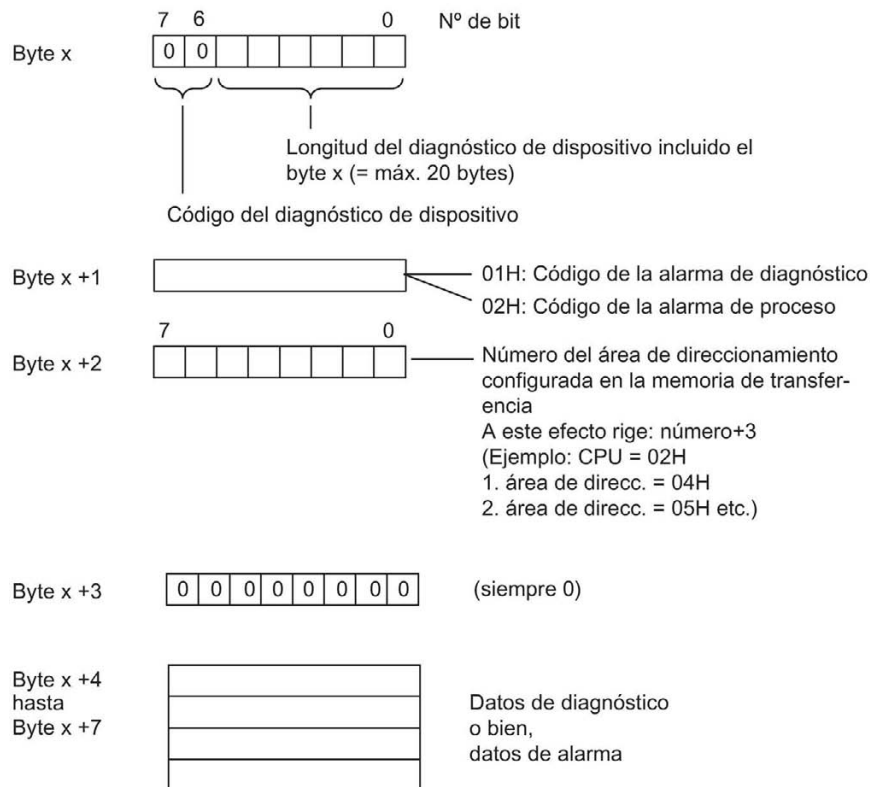
Figura 5-5 Estructura del diagnóstico de equipo
