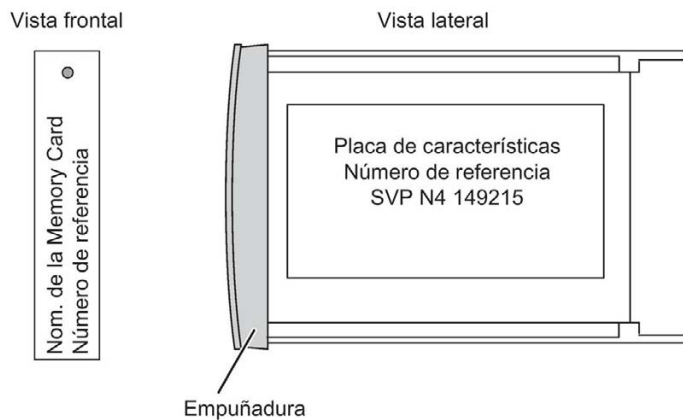
Figura 2-9 Diseño de la Memory Card
