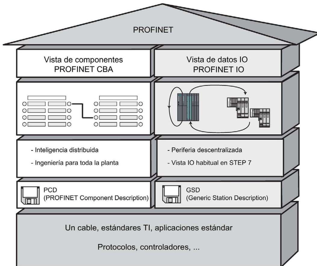
Figura 6-1 PROFINET IO y PROFINET CBA
