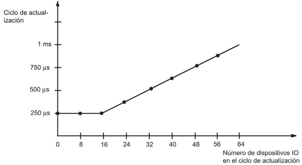
Figura 9-8 Ciclo de actualización
