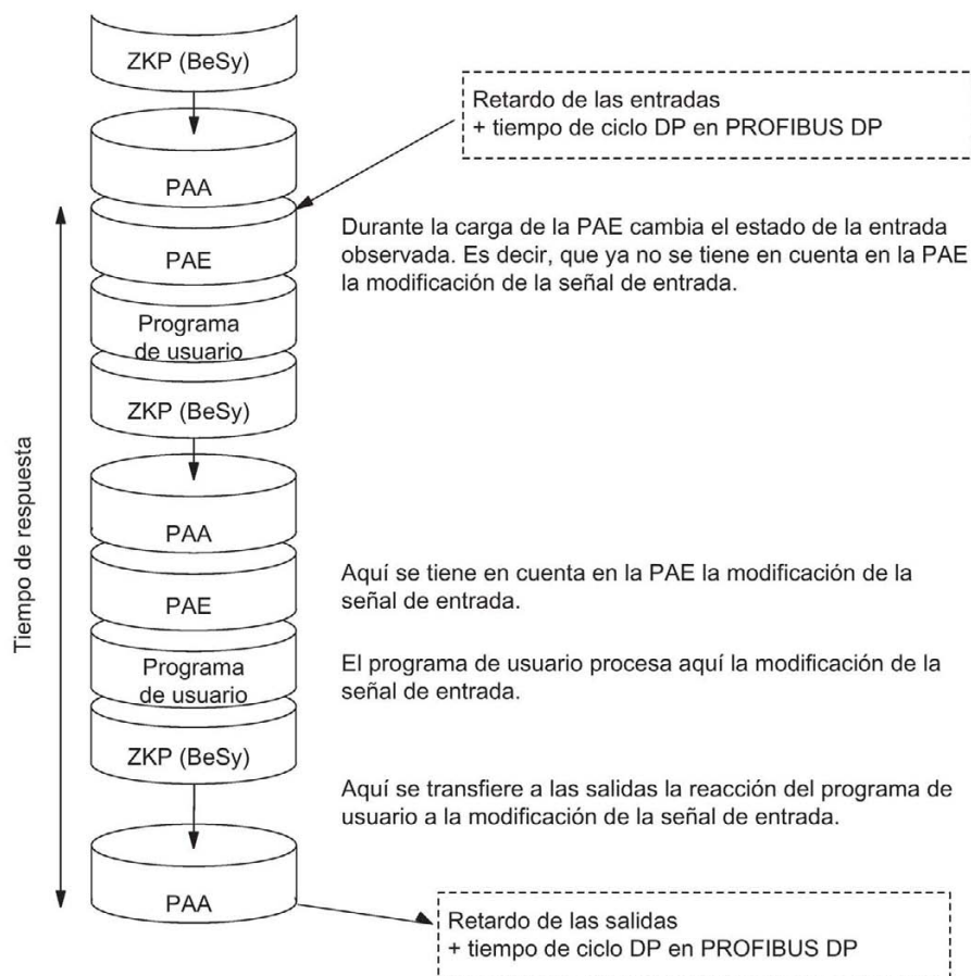
Figura 9-10 Tiempo de respuesta máximo
