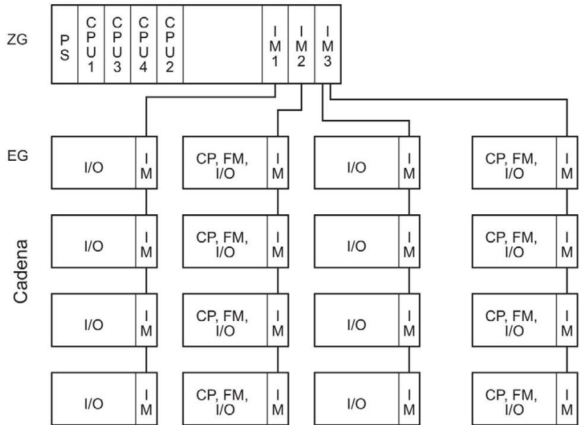
Figura 3-2 Ejemplo de modo multiprocesador
