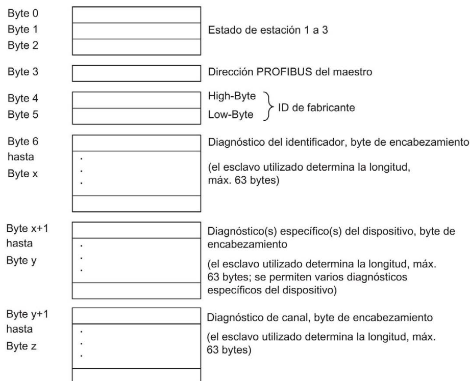
Figura 5-3 Estructura de un diagnóstico de esclavo
