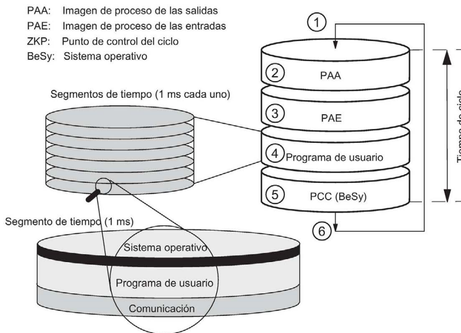
Figura 9-1 Elementos y composición del tiempo de ciclo
