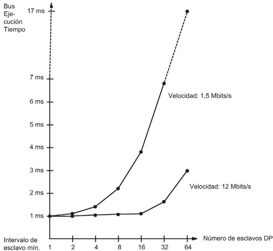
Figura 9-7 Tiempos de ciclo DP en la red PROFIBUS DP
