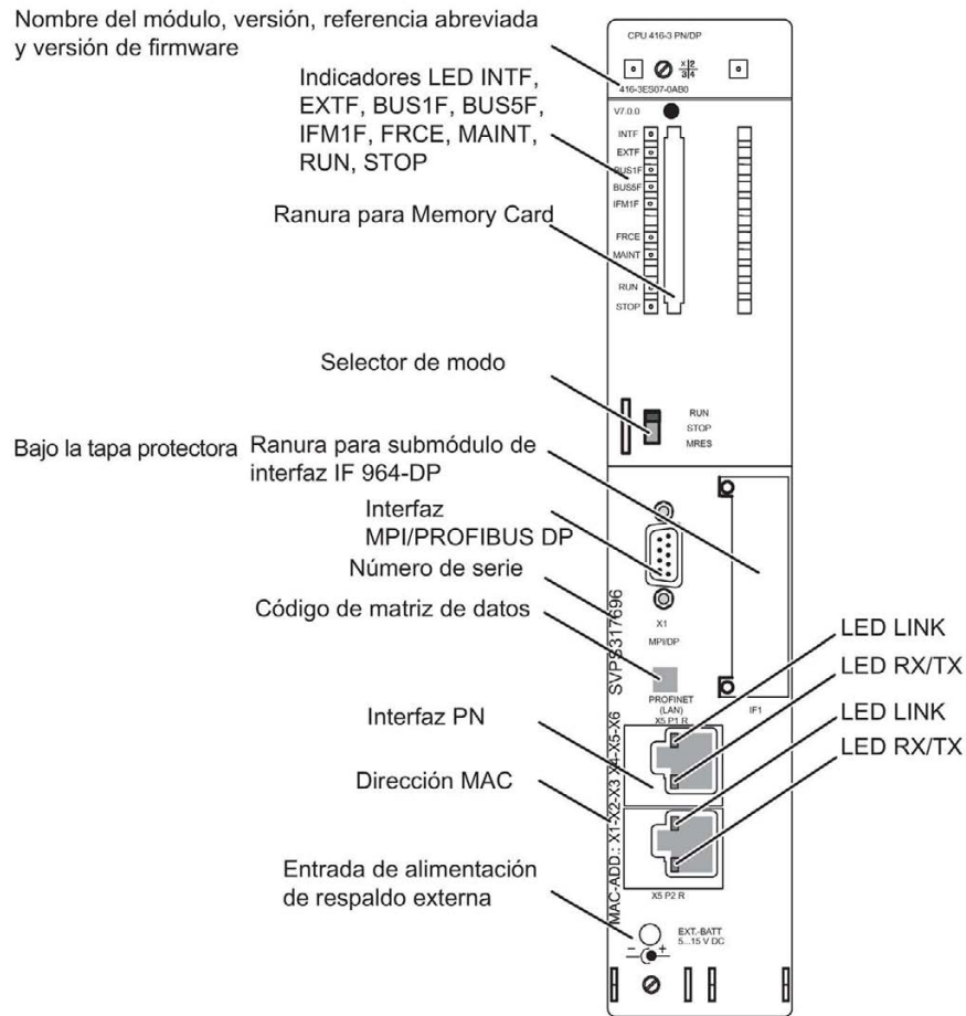
Figura 2-5 Disposición de los elementos de mando e indicadores de la CPU 41x-3 PN/DP
