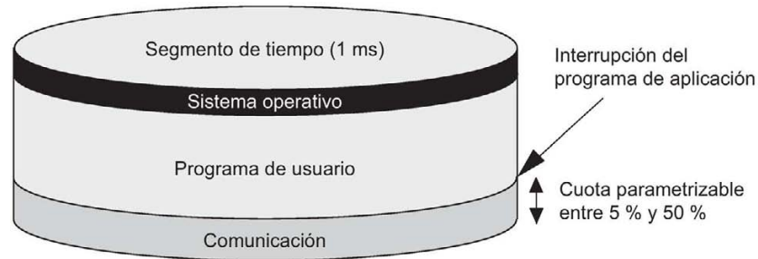
Figura 9-5 Fraccionamiento de un segmento de tiempo
