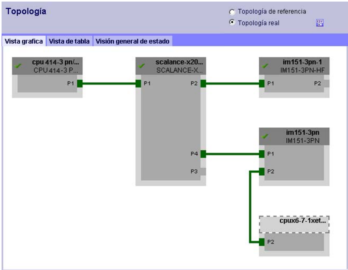
Figura 4-22 "Topología real" correcta
