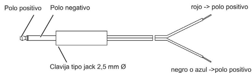
Figura 2-7 Cable de conexión con clavija tipo jack
