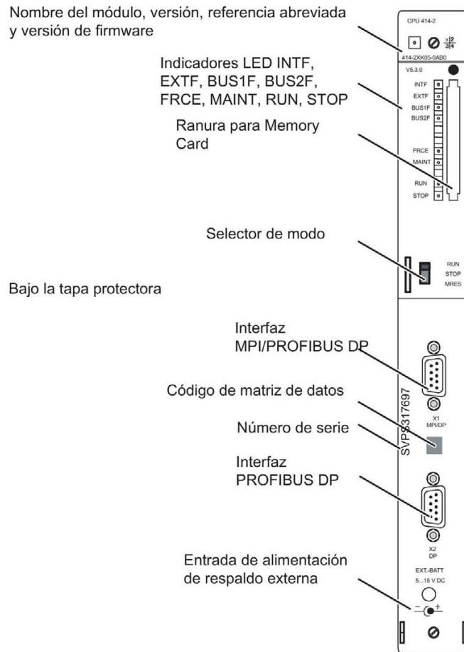
Figura 2-3 Disposición de los elementos de mando e indicadores de la CPU 41x-2
