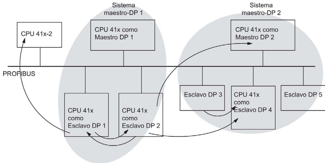
Figura 5-7 Comunicación directa con CPUs 41x
