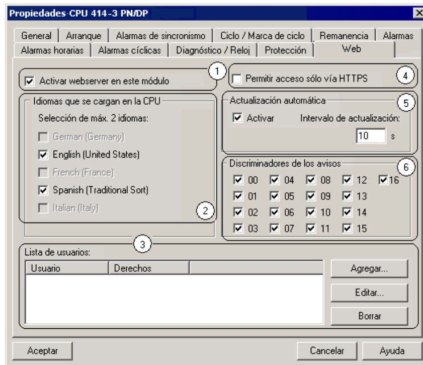
Figura 4-6 Ajustes en HW Config
