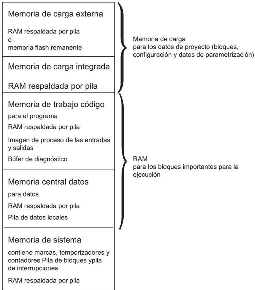
Figura 8-1 Áreas de memoria de las CPU S7-400
