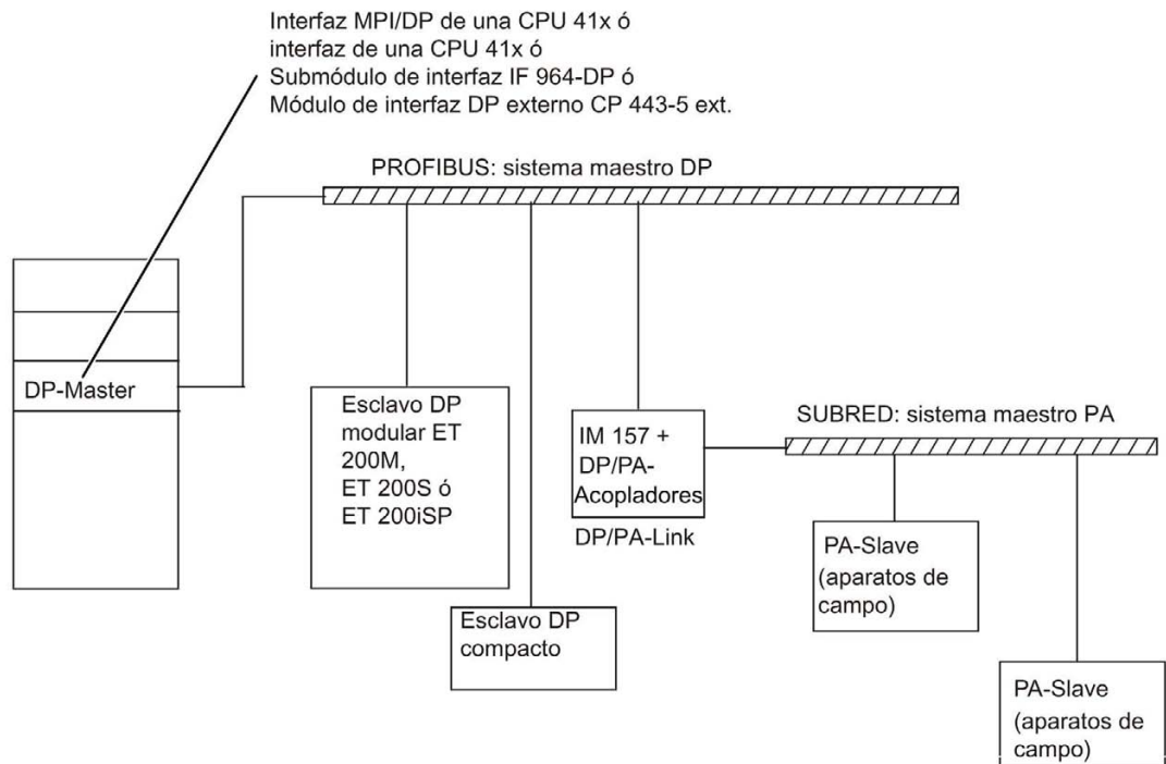
Figura 3-1 Resumen: Estructura del sistema para modificaciones con la instalación en marcha
