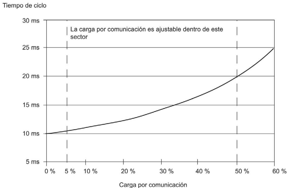
Figura 9-6 Dependencia entre el tiempo de ciclo real y la carga por comunicación
