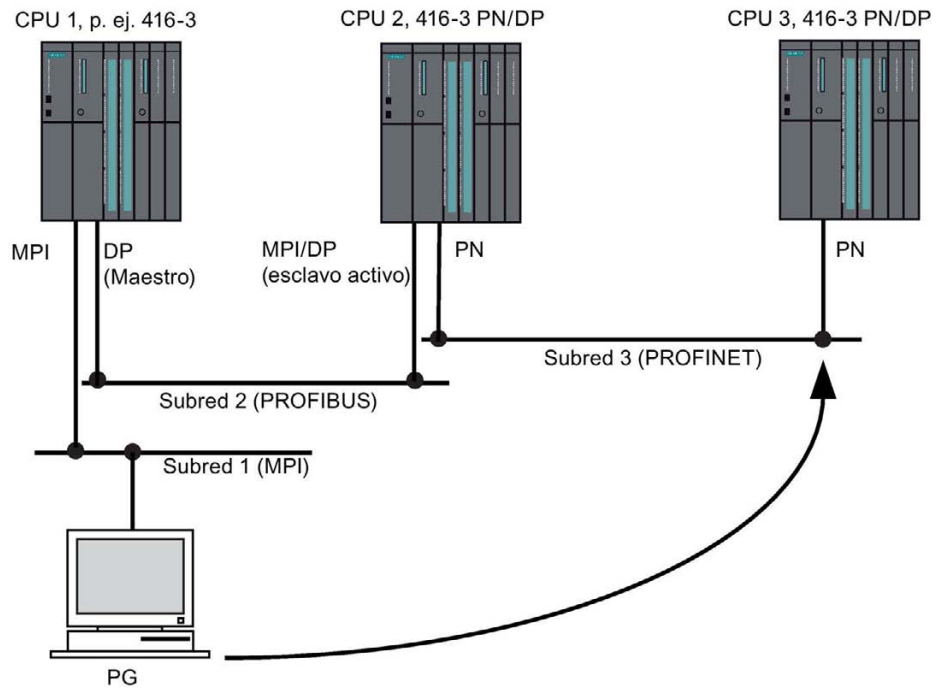
Figura 4-2 Transiciones de red vía S7-Routing: MPI - DP - PROFINET
