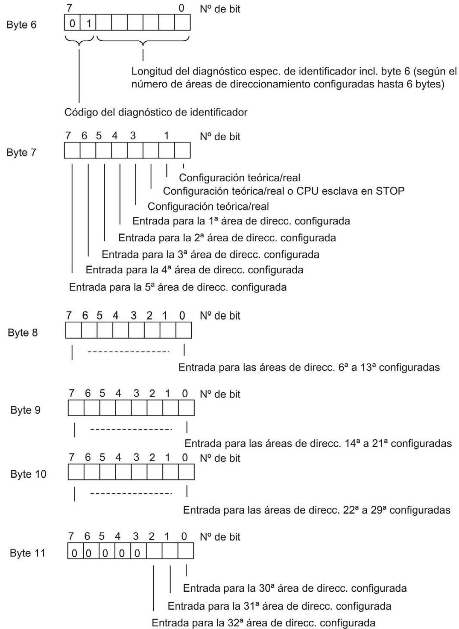
Figura 5-4 Estructura del diagnóstico de código en la CPU 41x
