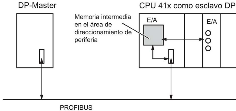
Figura 5-2 Memoria intermedia en la CPU 41x como esclavo DP
