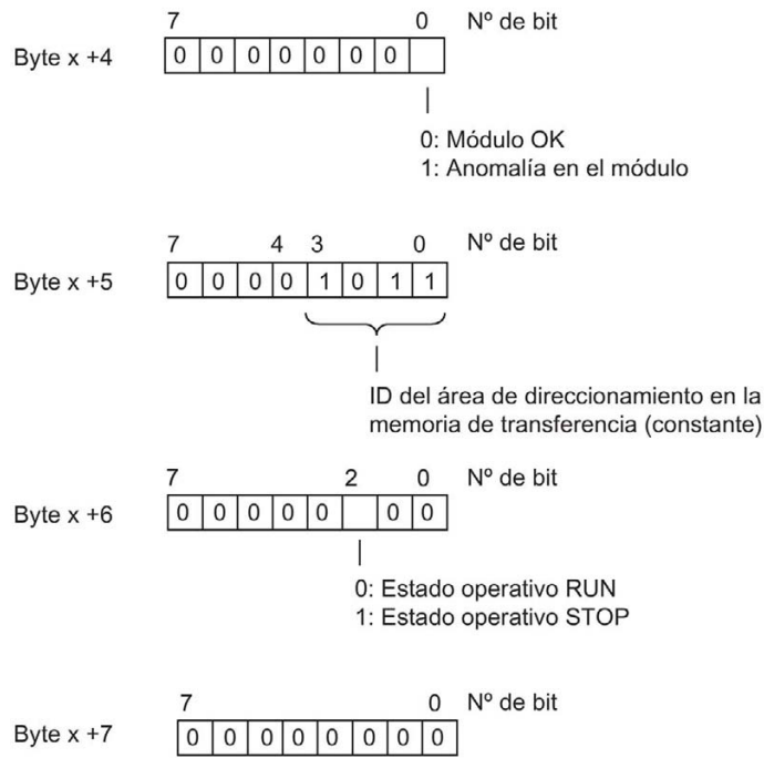
Figura 5-6 Bytes x +4 hasta x +7 alarma de diagnóstico y de proceso
