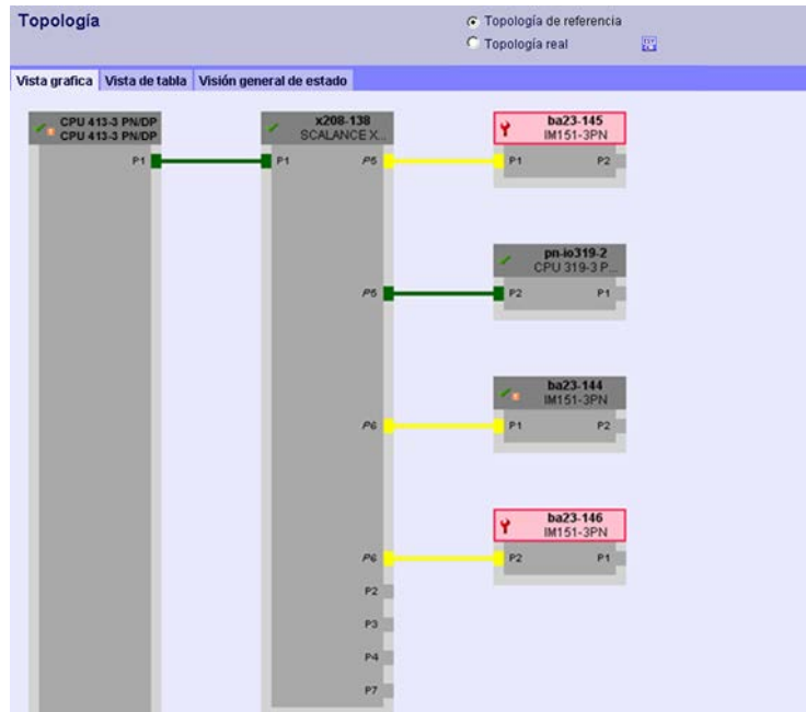
Figura 4-27 "Topología prevista" con cambio de herramienta
