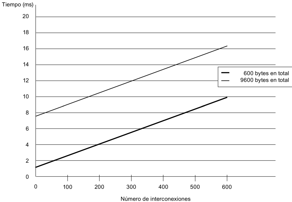
Figura 9-11 Tiempo de procesamiento para transmisión y recepción
