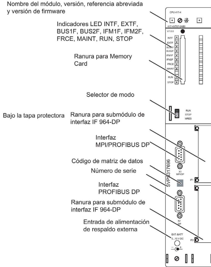
Figura 2-6 Disposición de los elementos de mando e indicadores de la CPU 417-4
