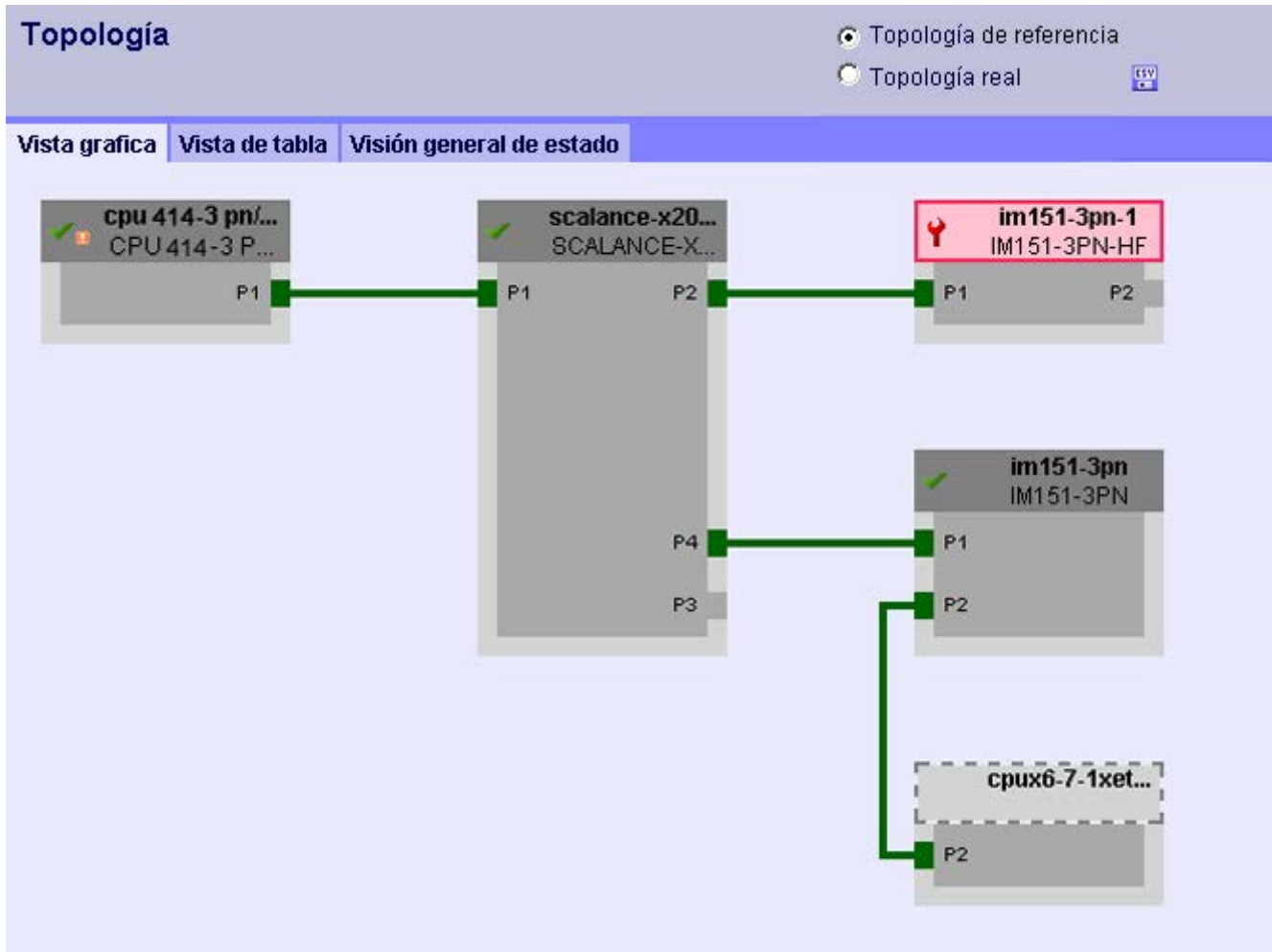
Figura 4-24 "Topología prevista" con dispositivo que falla
