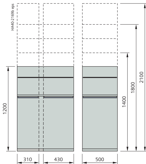
Switchgear height 1200 mm
