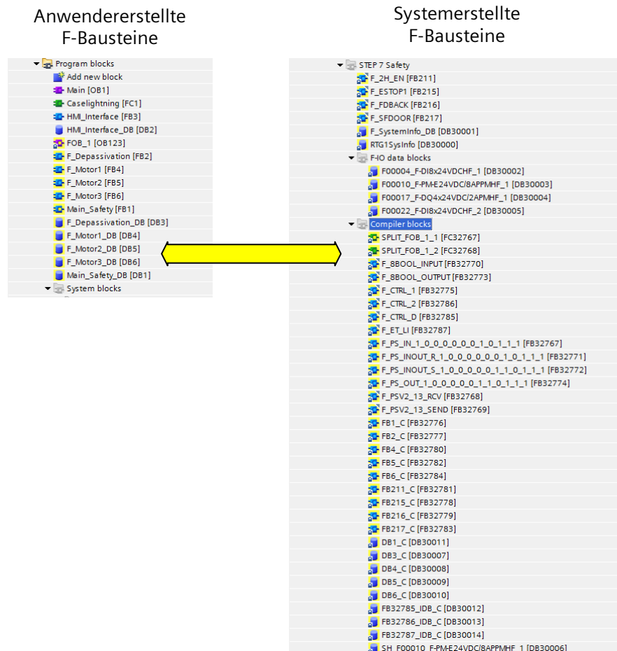
Abbildung 4-1: Absicherungsprogramm
