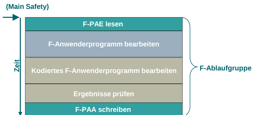
Abbildung 5-1 Ablauf der Bearbeitung des Sicherheitsprogramms
