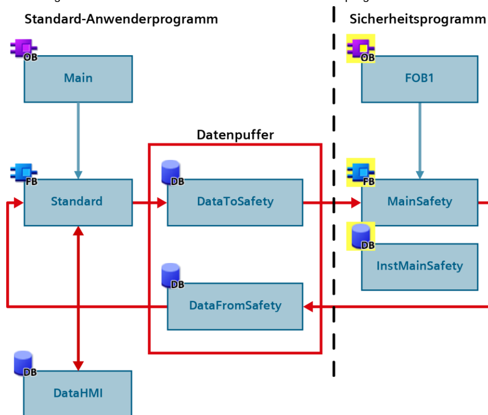
Abbildung 3-3: Datenaustausch zwischen HMI und Sicherheitsprogramm
