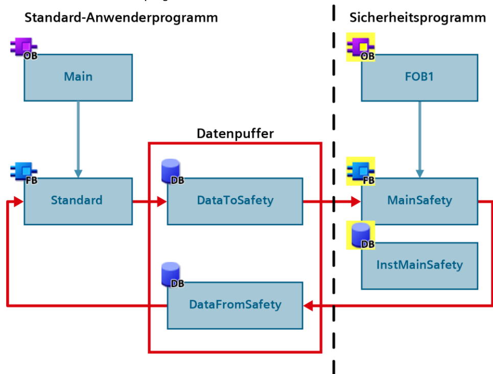
Abbildung 3-4: Datenaustausch zwischen Standard-Anwenderprogramm und Sicherheitsprogramm
