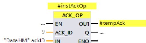
Abbildung 3-5: Systembaustein "ACK_OP"
