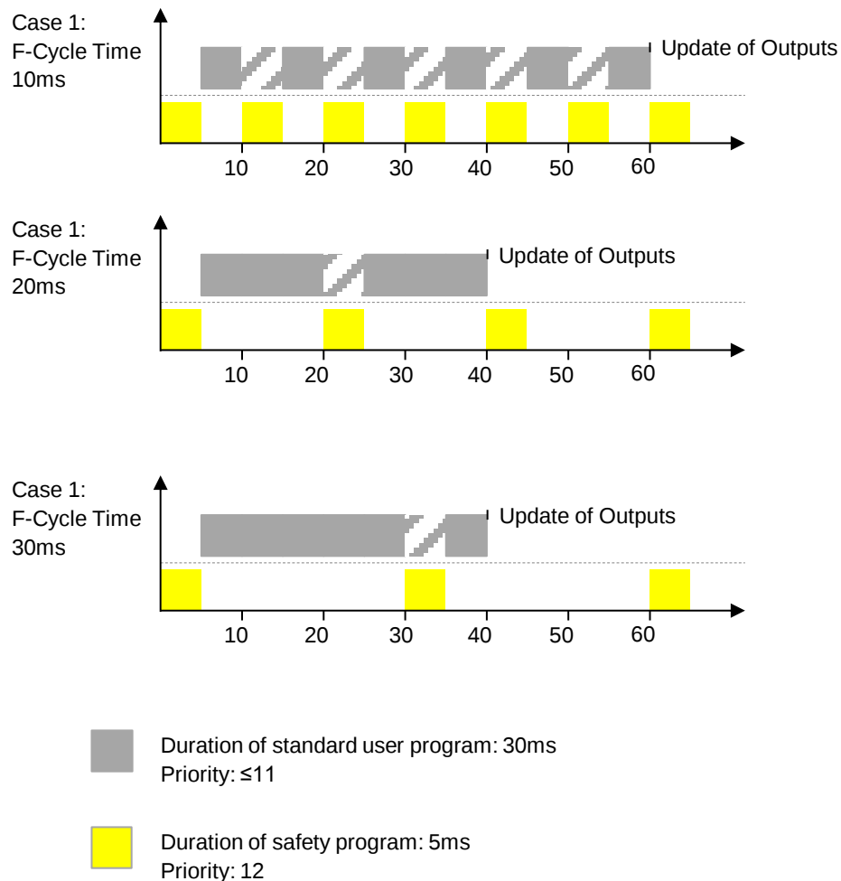
Abbildung 2-2:: Einfluss der Zykluszeit des Sicherheitsprogramms auf das Standard-Anwenderprogramm
