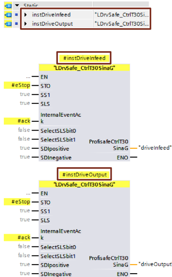
Abbildung 4-4: Multiinstanzen
