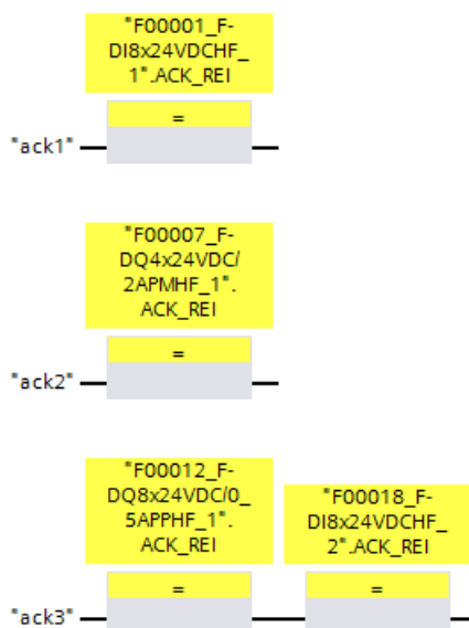
Abbildung 3-12: Separate Wiedereingliederung von Modulen
