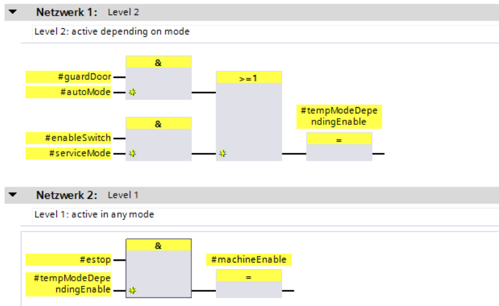
Abbildung 3-2: Betriebsarten programmieren
