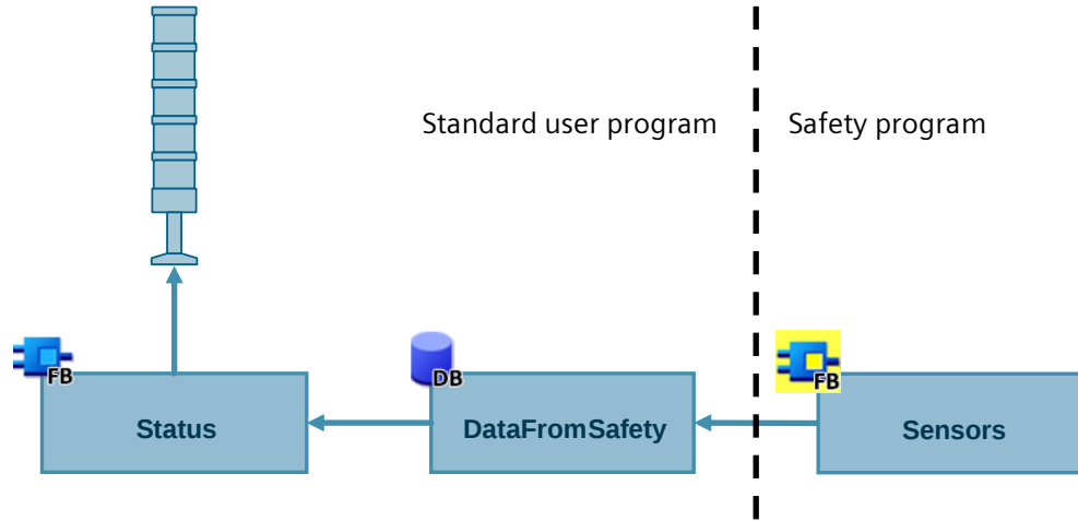
Abbildung 3-2: Diagnose- und Meldeinformationen aus dem Sicherheitsprogramm lesen
