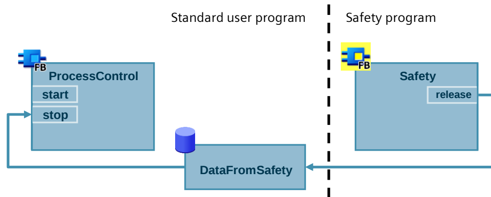
Abbildung 3-6: Prozesssteuerung mit dem Freigabesignal verriegeln
