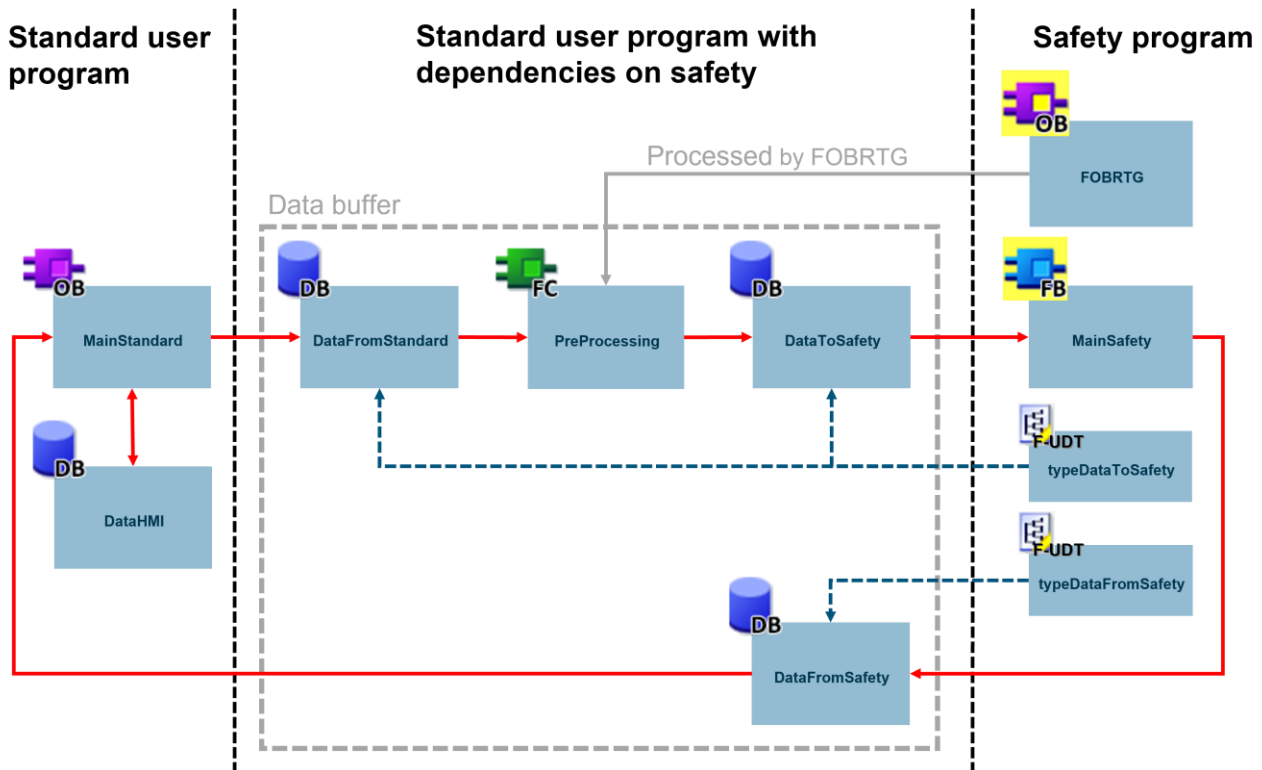
Abbildung 3-6 Prozessübersicht Datenaustausch zwischen Standard und Safety
