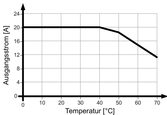
Bild 4-17 6EP1336-3BA10 Einbaulage (3)
