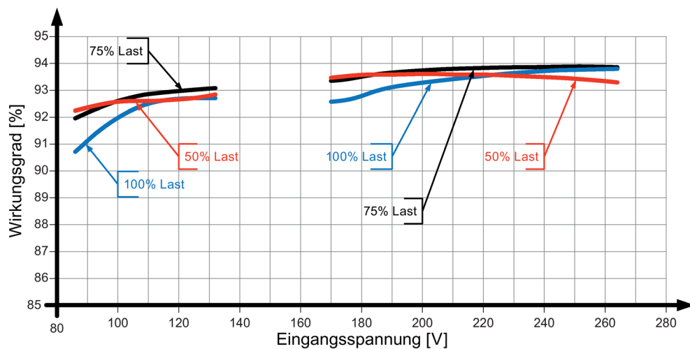
Bild 6-13 Wirkungsgrad 6EP3334-8SB00-0AY0
