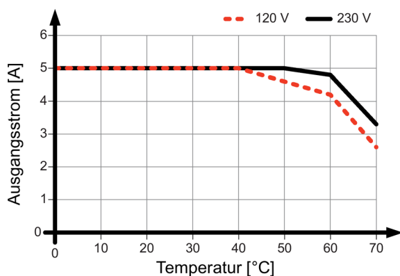
Bild 4-5 6EP3333-8SB00-0AY0 Einbaulage (1)
