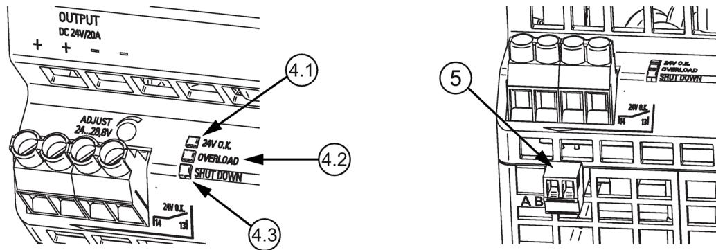
Bild 2-7 Betriebsanzeige und Meldekontakt für 6EP1336-3BA10
