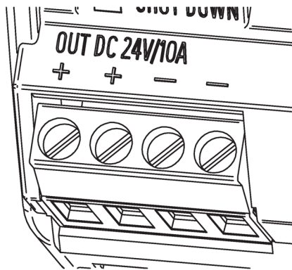
Bild 5-3 Ausgangsanschluss (Beispiel 6EP3334-8SB00-0AY0)
