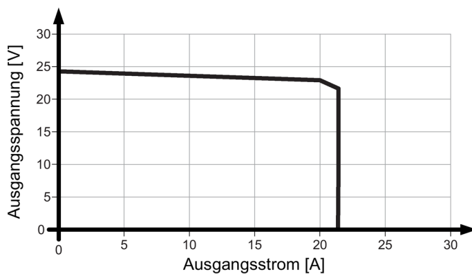
Bild 6-8 Ausgangskennlinie 6EP1336-3BA10 Parallelbetrieb
