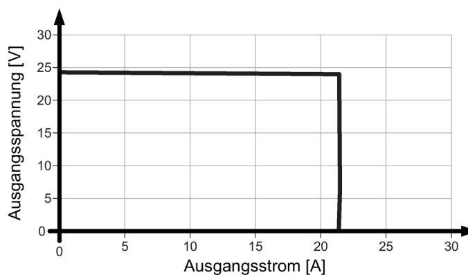
Bild 6-5 Ausgangskennlinie 6EP1336-3BA10 Einzelbetrieb
