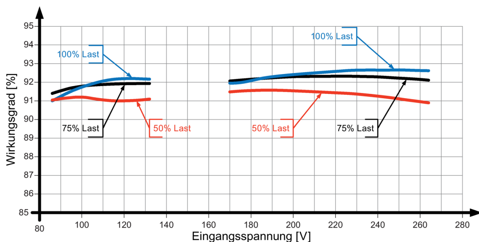
Bild 6-12 Wirkungsgrad 6EP3333-8SB00-0AY0
