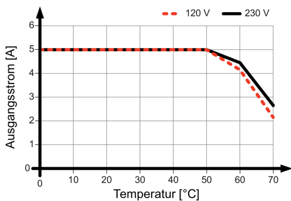
Bild 4-9 6EP3333-8SB00-0AY0 Einbaulage (5)
