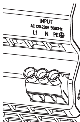
Bild 5-2 Netzanschluss für 6EP1336-3BA10
