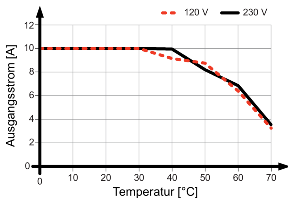
Bild 4-10 6EP3334-8SB00-0AY0 Einbaulage (1)
