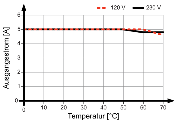
Bild 4-7 6EP3333-8SB00-0AY0 Einbaulage (3)
