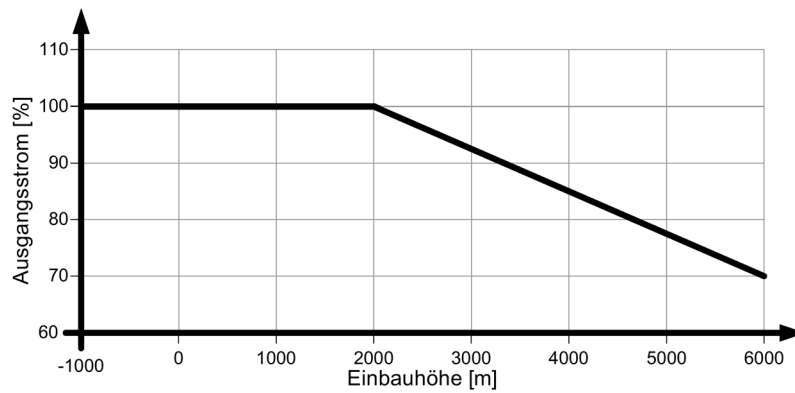
Bild 4-4 Einbauhöhenderating
