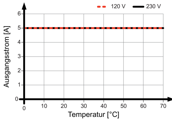
Bild 4-1 6EP3333-8SB00-0AY0 Standardeinbaulage
