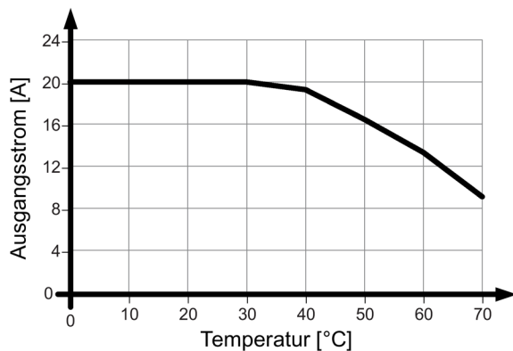
Bild 4-15 6EP1336-3BA10 Einbaulage (1)
