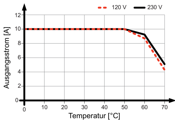
Bild 4-12 6EP3334-8SB00-0AY0 Einbaulage (3)
