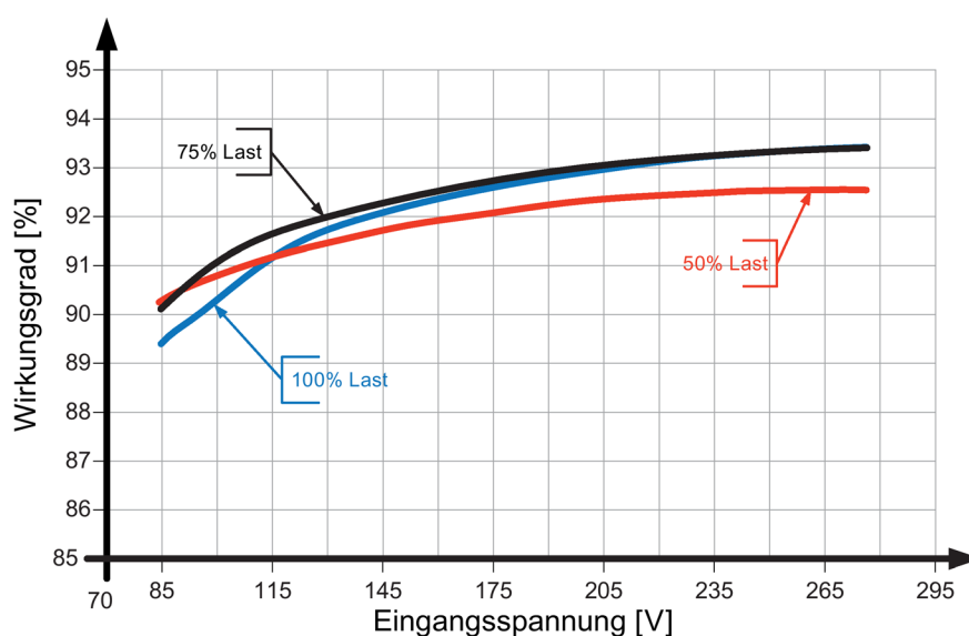
Bild 6-14 Wirkungsgrad 6EP1336-3BA10
