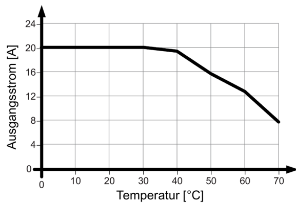
Bild 4-19 6EP1336-3BA10 Einbaulage (5)
