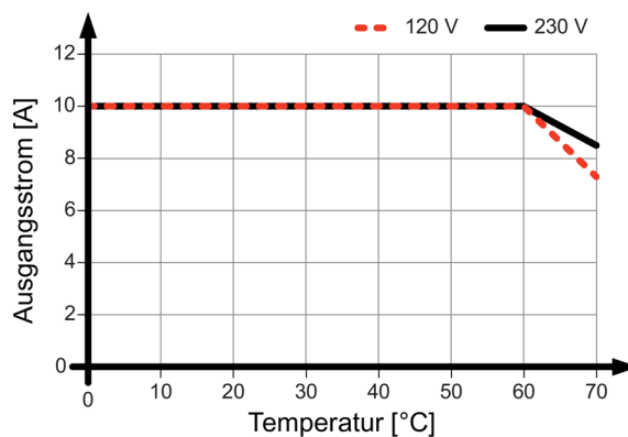
Bild 4-2 6EP3334-8SB00-0AY0 Standardeinbaulage
