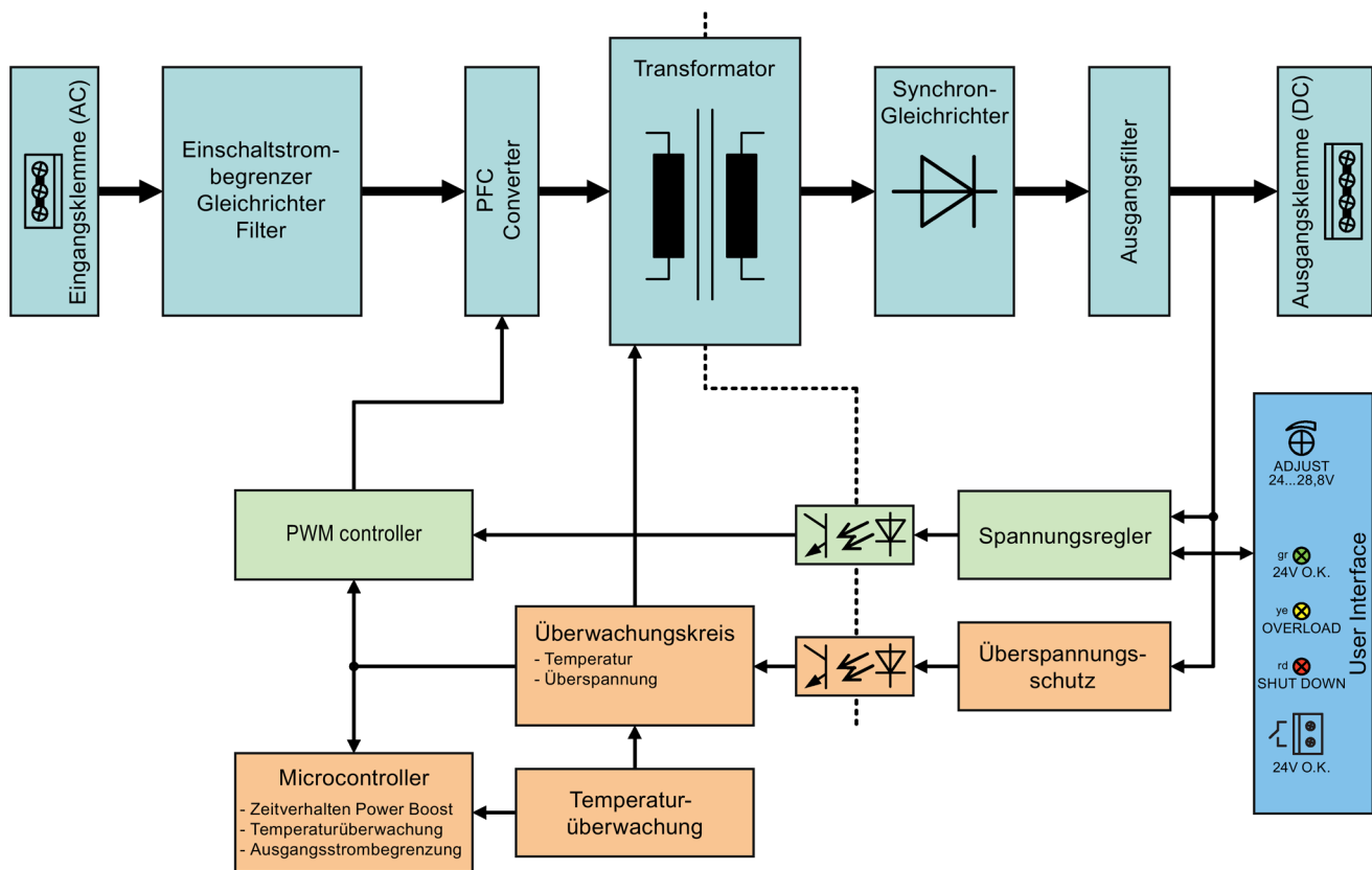
Bild 2-11 Blockdiagramm für 6EP1336-3BA10
