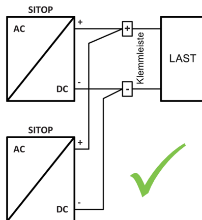
Bild 9-1 Parallelschaltung
