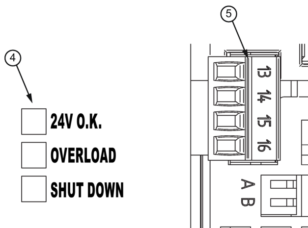
Bild 2-6 Betriebsanzeige und Meldekontakt für 6EP3333-8SB00-0AY0 und 6EP3334-8SB00-0AY0
