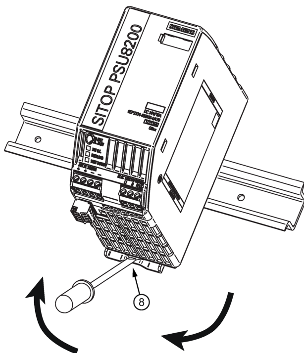
Bild 3-1 Montage/Demontage (Beispiel: 6EP3334-8SB00-0AY0)
