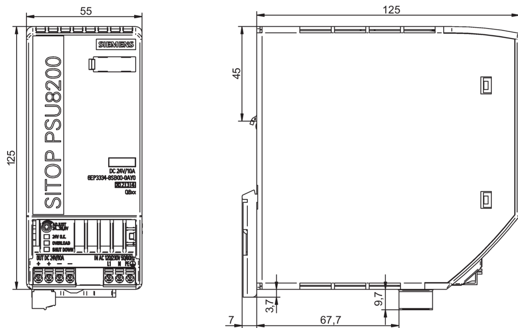
Bild 2-13 Maßzeichnung 6EP3334-8SB00-0AY0
