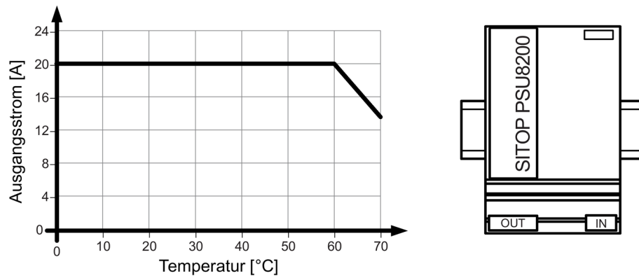
Bild 4-3 6EP1336-3BA10 Standardeinbaulage
