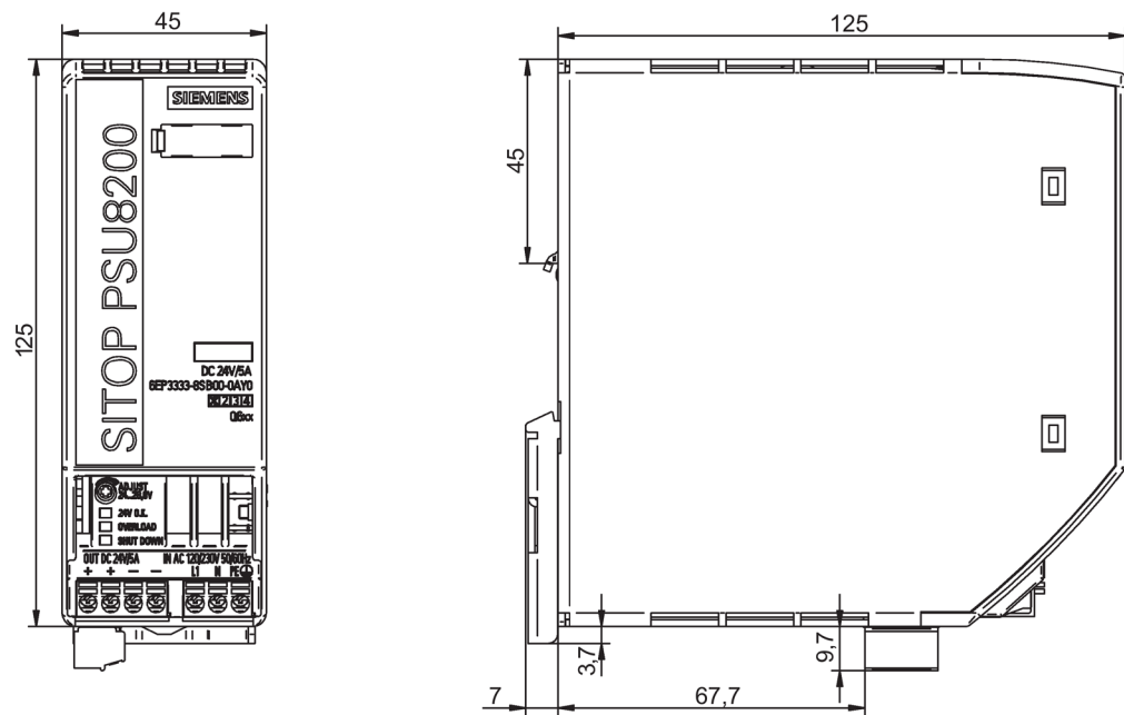
Bild 2-12 Maßzeichnung 6EP3333-8SB00-0AY0
