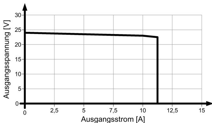
Bild 6-7 Ausgangskennlinie 6EP3334-8SB00-0AY0 Parallelbetrieb
