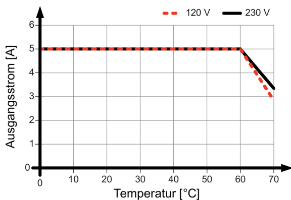
Bild 4-6 6EP3333-8SB00-0AY0 Einbaulage (2)
