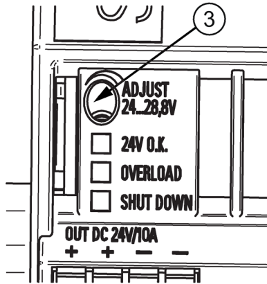
Bild 2-5 Potenziometer (Beispiel: 6EP3334-8SB00-0AY0)
