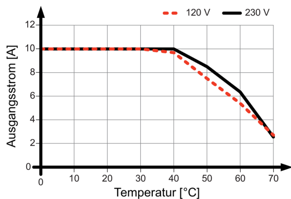
Bild 4-14 6EP3334-8SB00-0AY0 Einbaulage (5)
