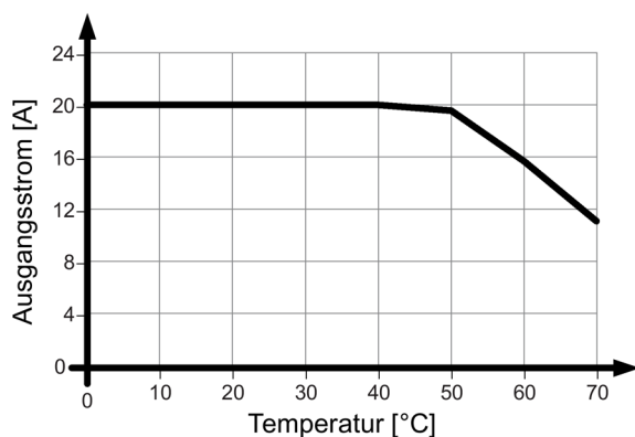
Bild 4-16 6EP1336-3BA10 Einbaulage (2)
