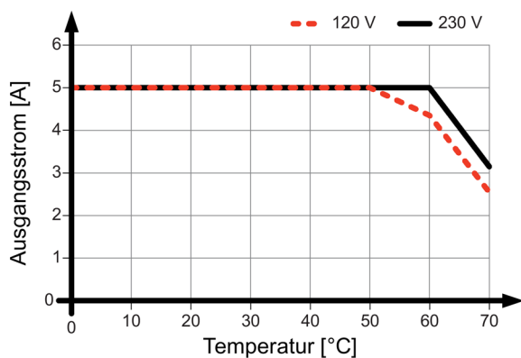
Bild 4-8 6EP3333-8SB00-0AY0 Einbaulage (4)
