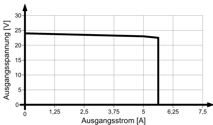
Bild 6-6 Ausgangskennlinie 6EP3333-8SB00-0AY0 Parallelbetrieb
