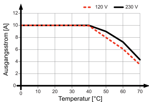
Bild 4-13 6EP3334-8SB00-0AY0 Einbaulage (4)
