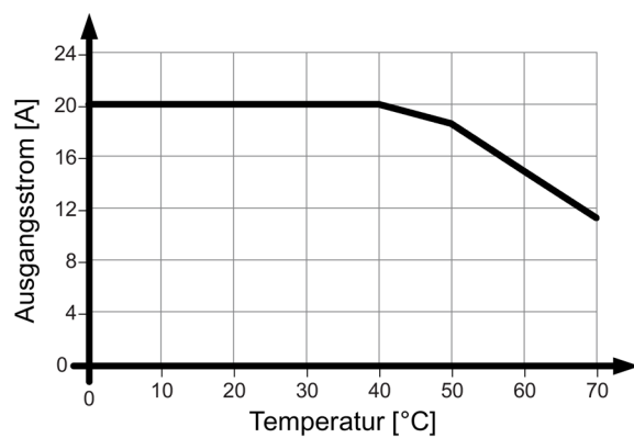
Bild 4-18 6EP1336-3BA10 Einbaulage (4)
