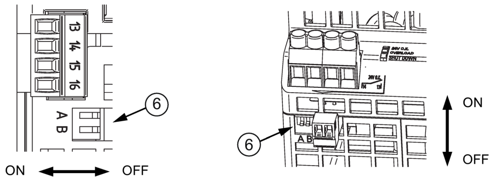
Bild 2-8 Wahlschalter
