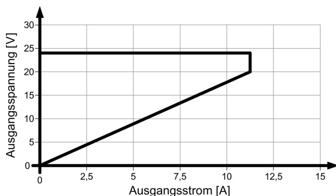
Bild 6-10 Ausgangskennlinie 6EP3334-8SB00-0AY0 Speichernde Abschaltung
