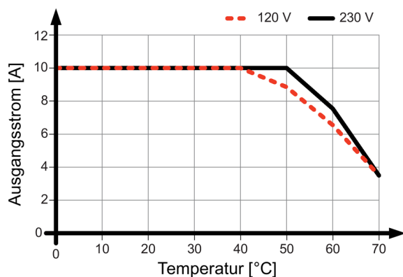
Bild 4-11 6EP3334-8SB00-0AY0 Einbaulage (2)
