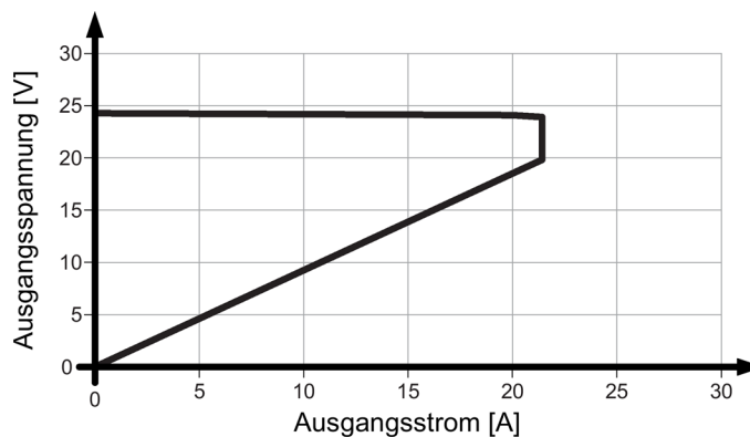
Bild 6-11 Ausgangskennlinie 6EP1336-3BA10 Speichernde Abschaltung
