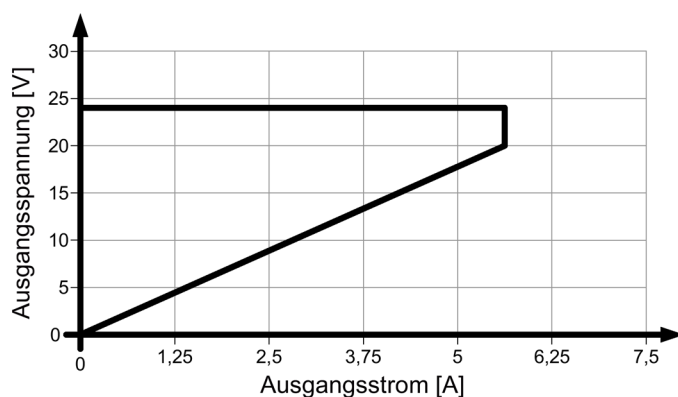
Bild 6-9 Ausgangskennlinie 6EP3333-8SB00-0AY0 Speichernde Abschaltung
