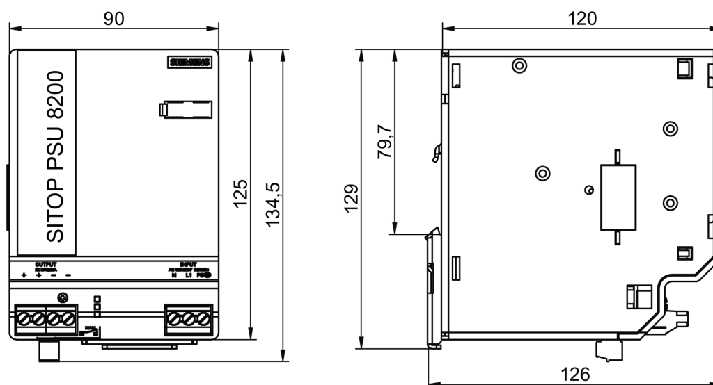
Bild 2-14 Maßzeichnung 6EP1336-3BA10
