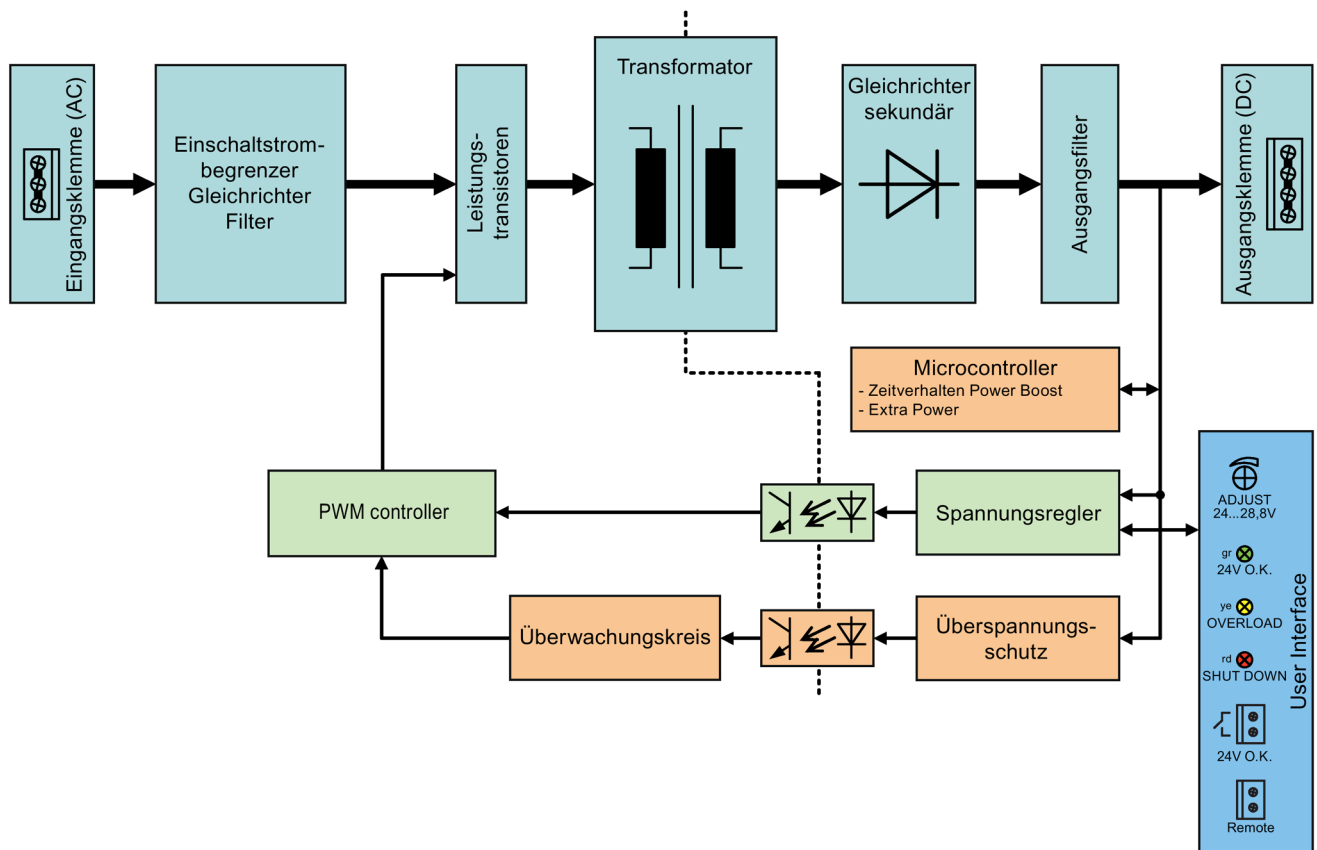
Bild 2-10 Blockdiagramm für 6EP3333-8SB00-0AY0 und 6EP3334-8SB00-0AY0
