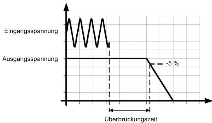
Bild 6-1 Netzausfallüberbrückung
