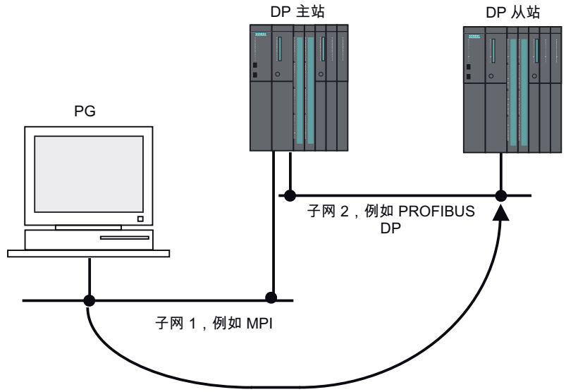
图 4-1 S7 路由
