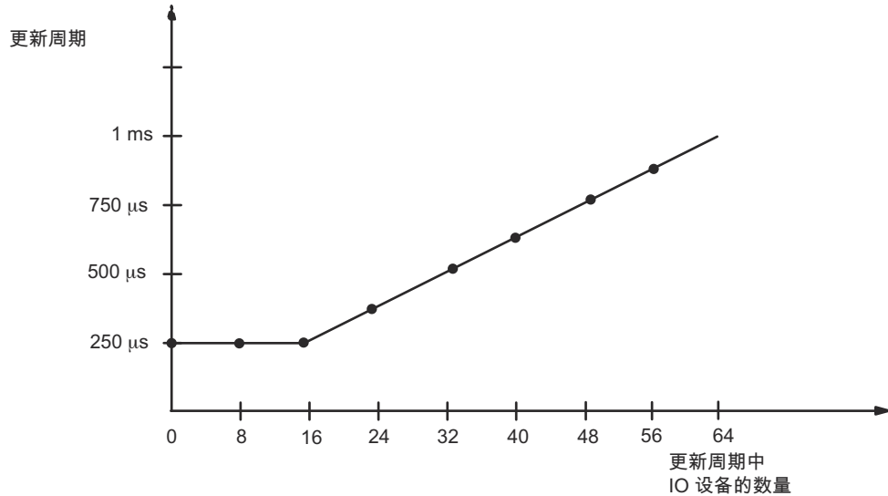
图 9-8 更新周期
