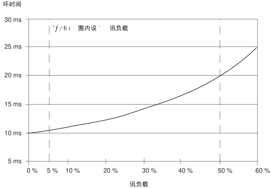
图 9-6 周期时间与通信负载的相关性
