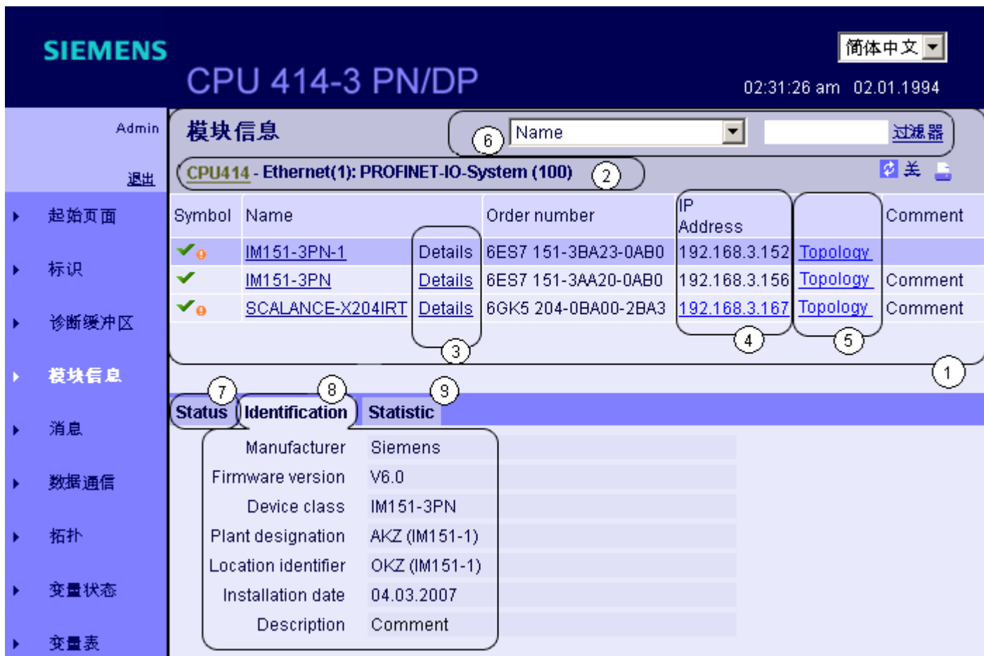
图 4-13 模块状态
