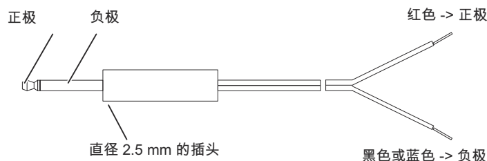
图 2-7 带插头的电缆
