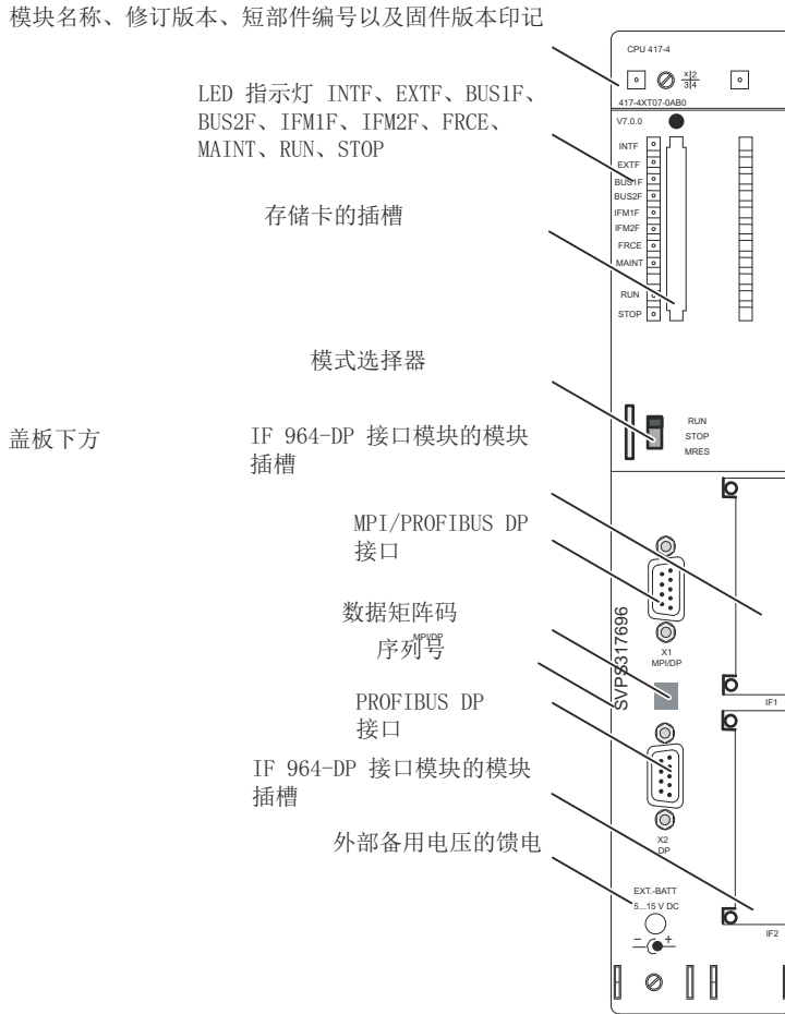
图 2-6 CPU 417-4 上控制和显示元件的排列
