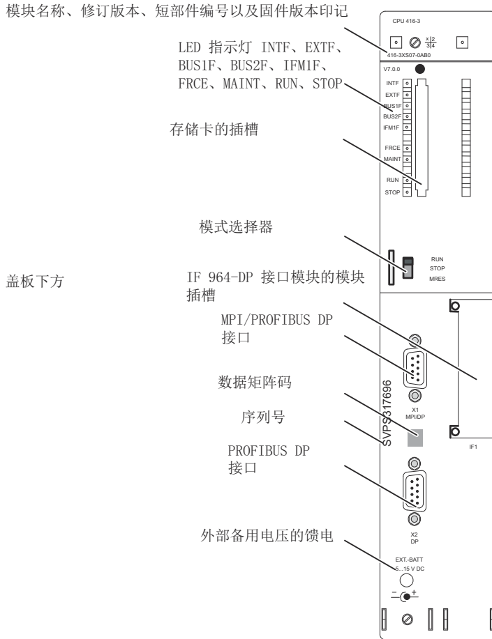
图 2-4 CPU 41x-3 上控制和显示元件的排列
