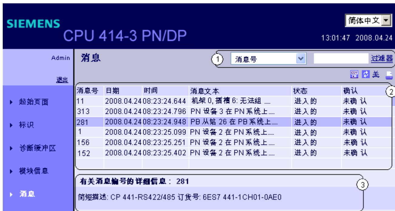
图 4-16 消息
