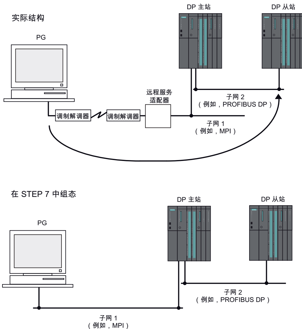
图 4-3 S7 路由: TeleService 应用示例
