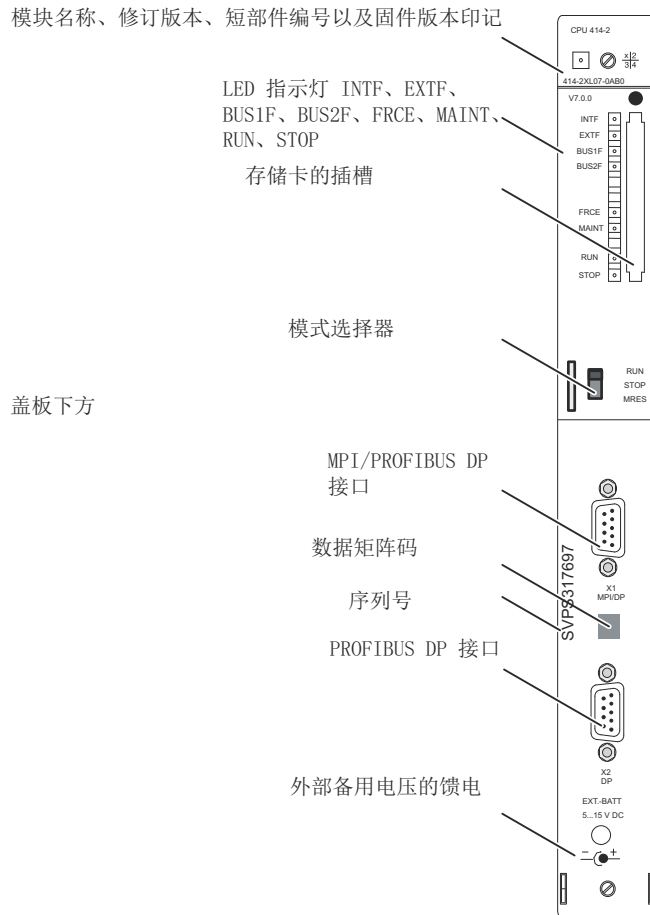
图 2-3 CPU 41x-2 上控制和显示元件的排列
