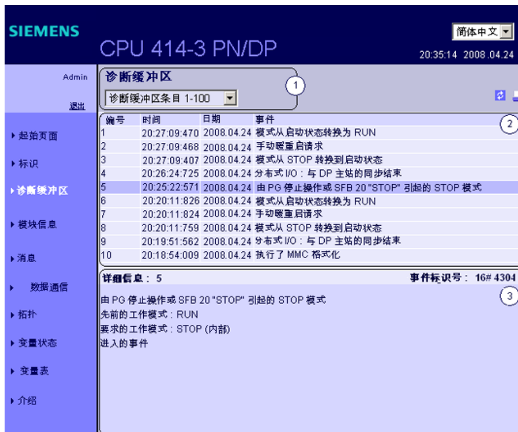
图 4-11 诊断缓冲区
