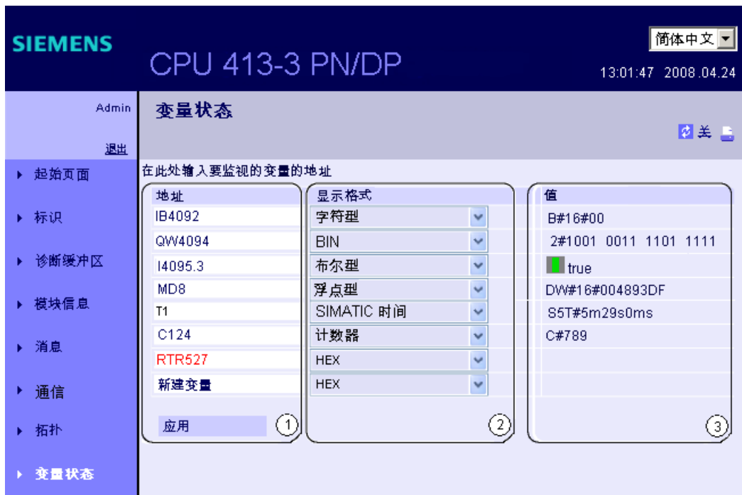
图 4-28 变量状态
