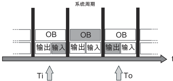
图 5-10 系统周期
