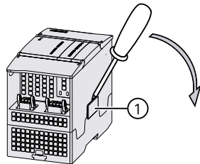
① 总线盖
