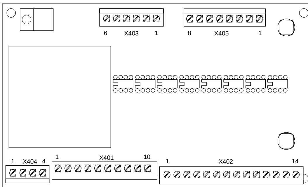
Bild 5-3 Klemmenleistenanordnung auf der DTI-Baugruppe 6SE7090-0XX84-3DB0
