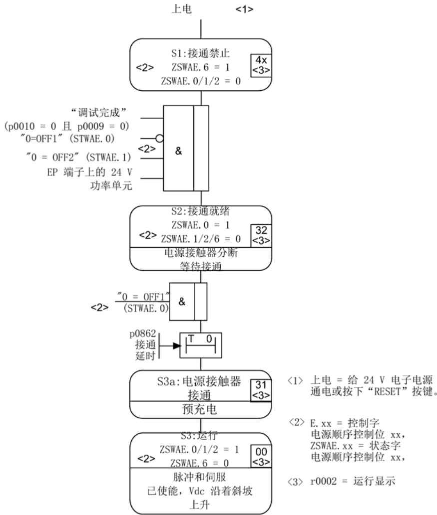
图 2-9 基本型电源的启动过程
