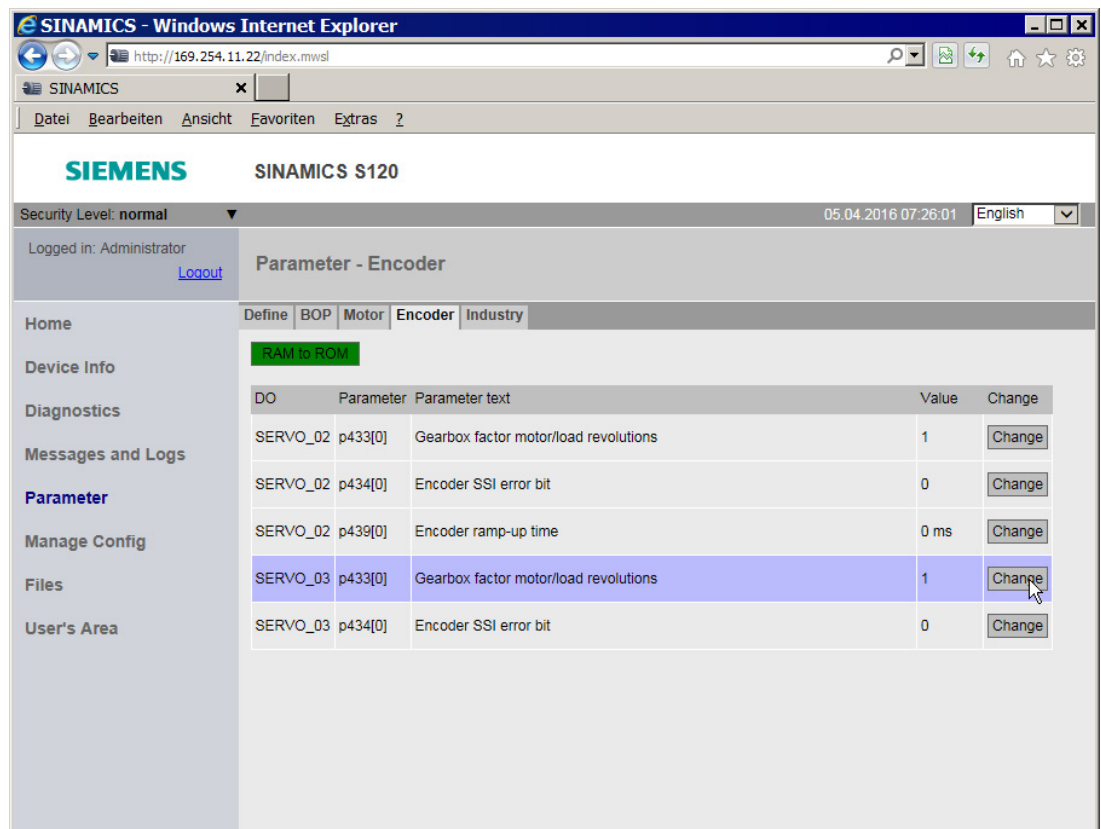
图 7-42 修改驱动参数
