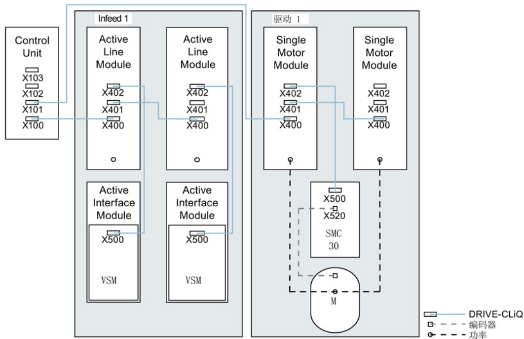
图 A-3 由并联的装机装柜型功率单元组成的驱动组
