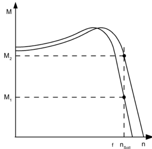
图 6-5 转差补偿
