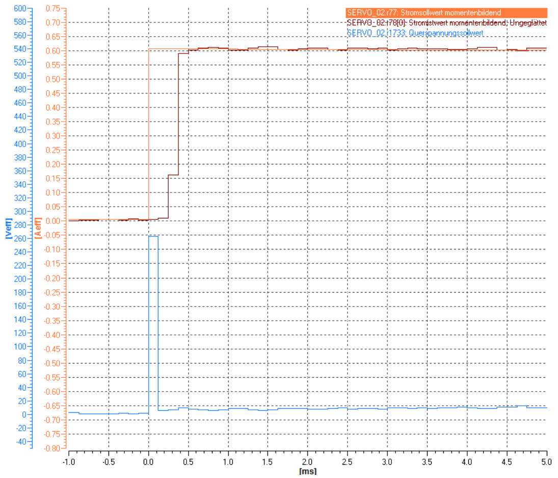
图 4-30 电压前馈控制 p1703 正常
