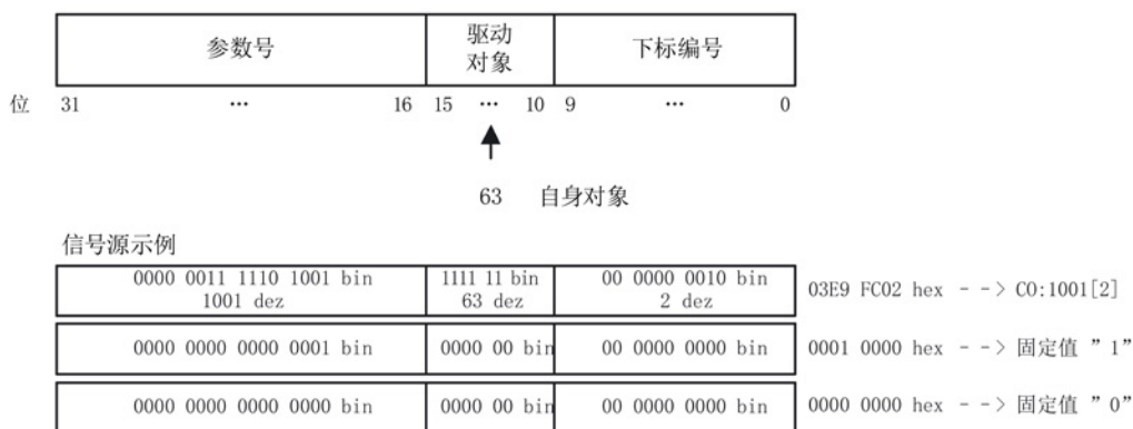
图 13-11 二进制/模拟量互联输出参数的内部编码
