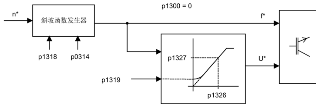
图 4-13 V/f 控制的结构
