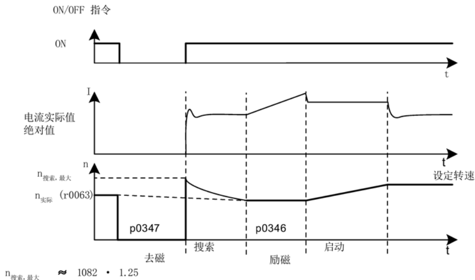
图 5-24 示例：捕捉重启，用于无编码器异步电机
