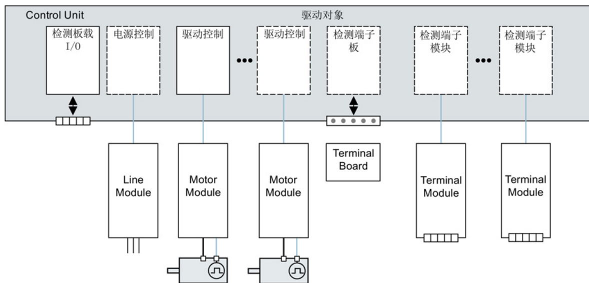
图 13-3 驱动对象 - Drive Objects
