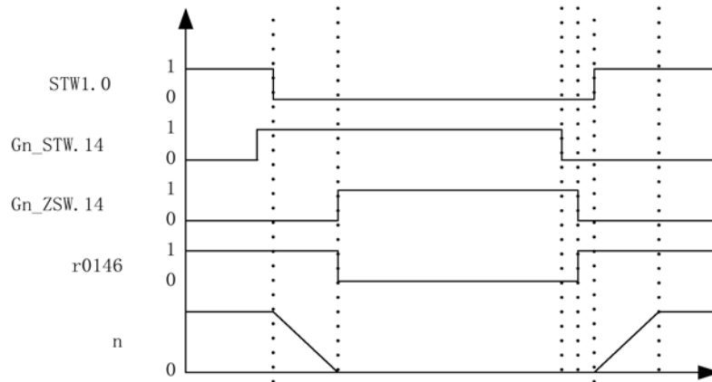
图 7-12 驻留编码器的时序图
