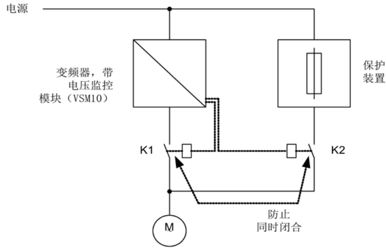
图 5-28 线路示例：带同步、不带重叠的旁路
