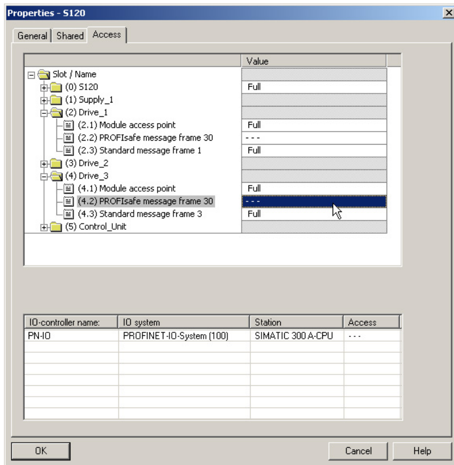
图 11-42 使能 A-CPU 的 Safety 报文
