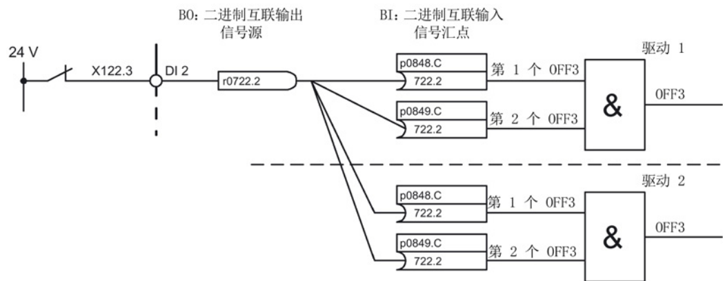
图 13-13 “OFF3”互联到多个驱动（示例）
