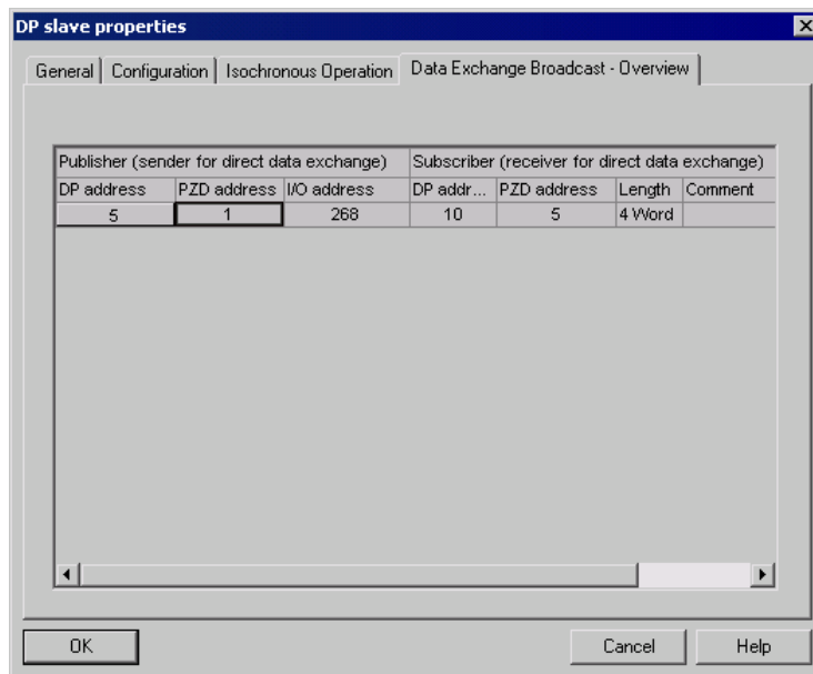
图 11-25 “从站-从站”通讯一览
