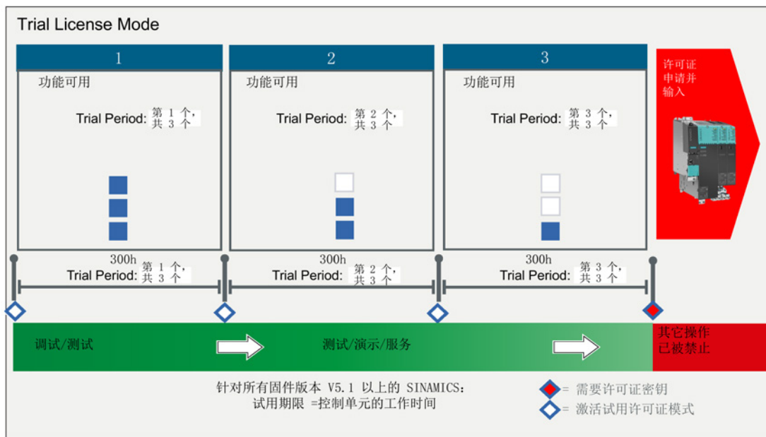
图 13-5 示意图：试用许可证模式
