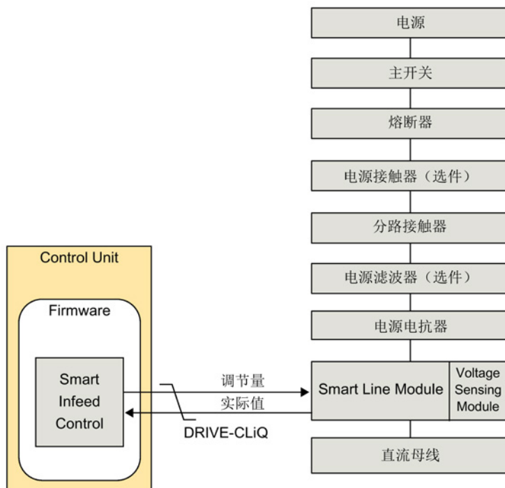
图 2-5 装机装柜型非调节型电源的结构框图
