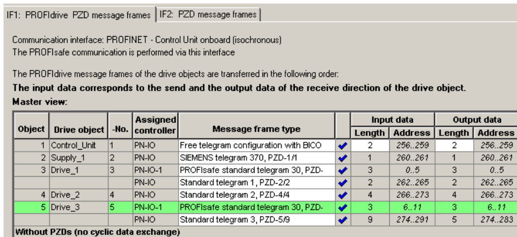
图 11-40 报文已通过 HW-Config 调整
