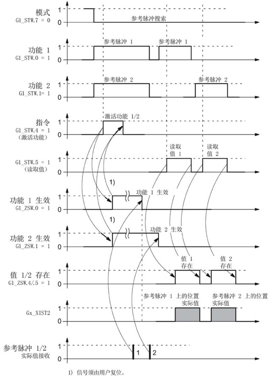
图 11-4 “参考脉冲搜索”功能的时序图
