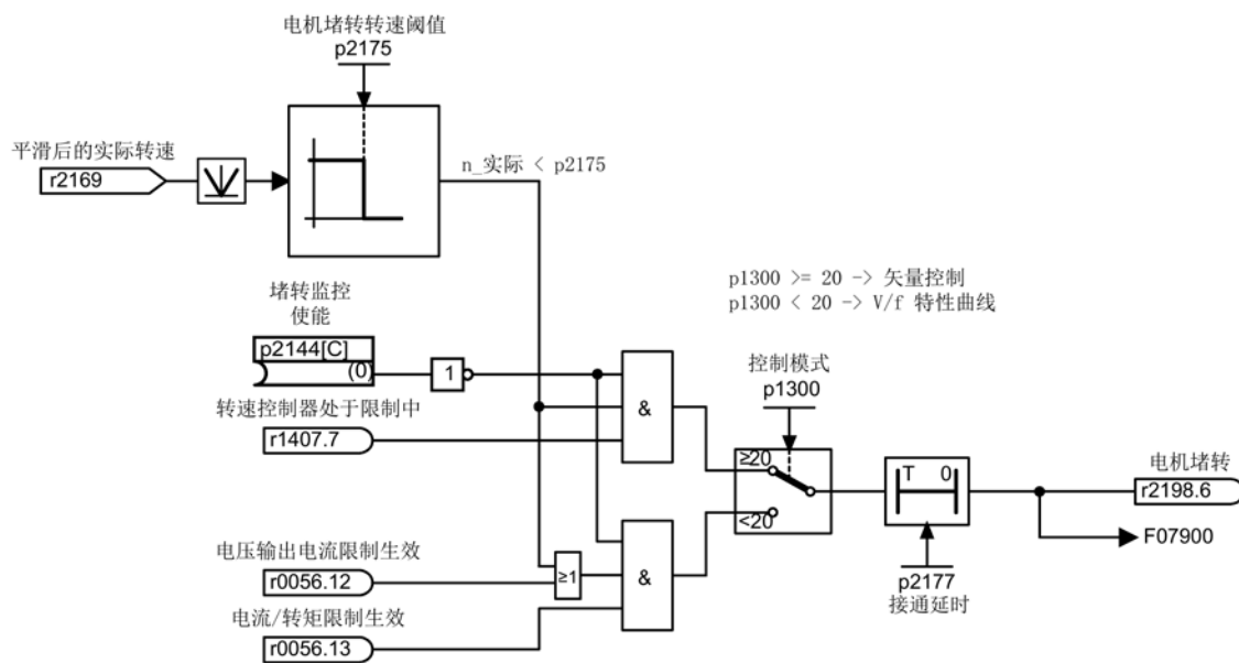
图 9-1 堵转保护
