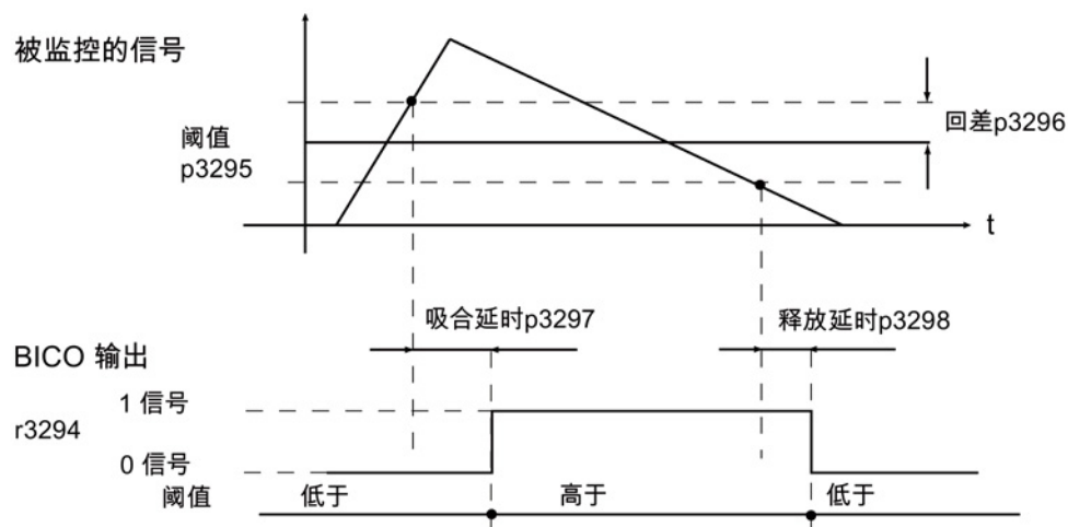
图 4-23 变量报告功能
