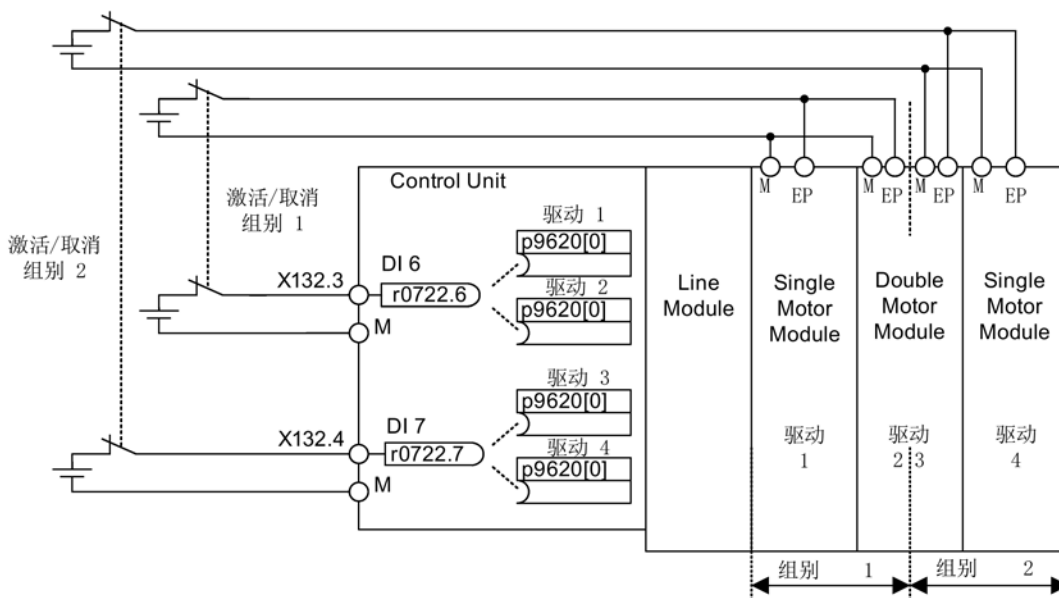
图 10-3 示例：端子分组：以书本型电机模块和 CU320-2 为例
