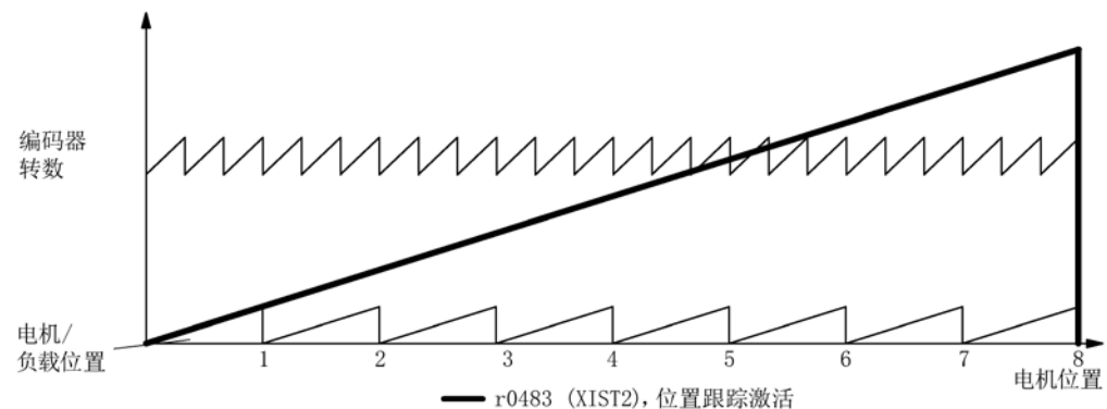
图 7-16 奇数传动比，有位置跟踪(p0412 = 8)
