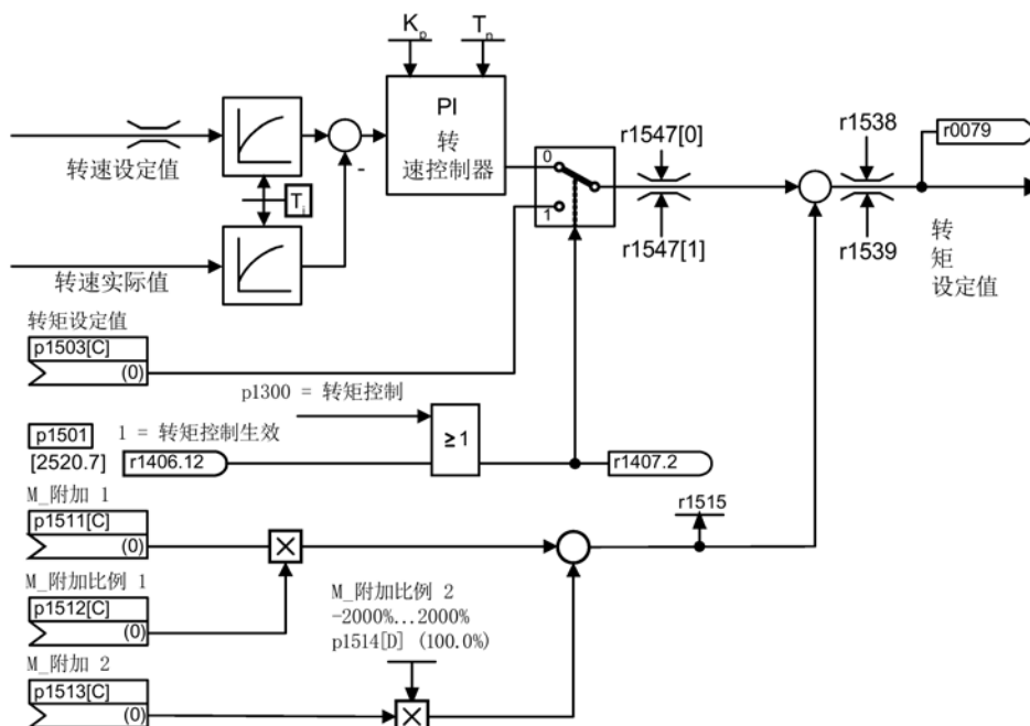
图 5-13 转速/转矩控制
