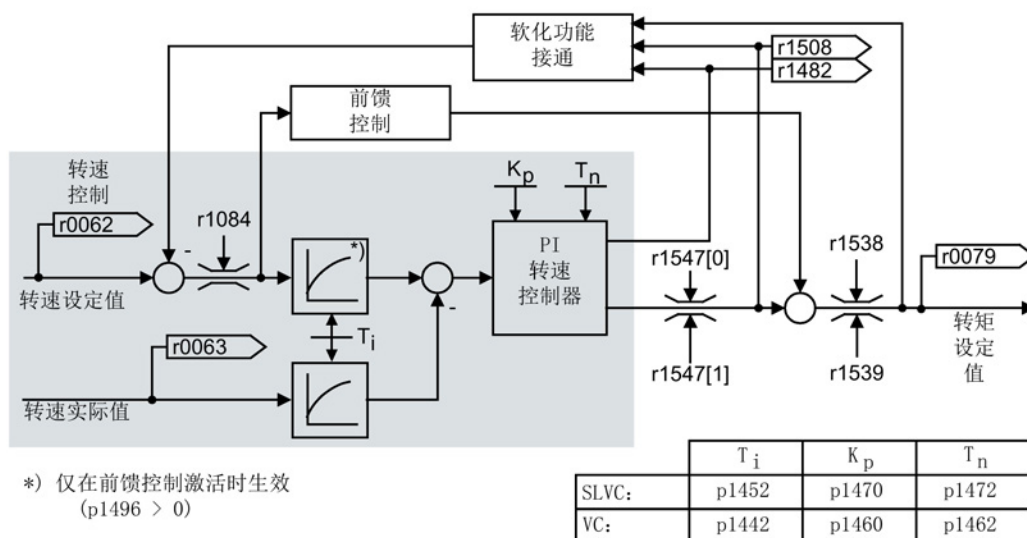
图 5-6 转速控制器
