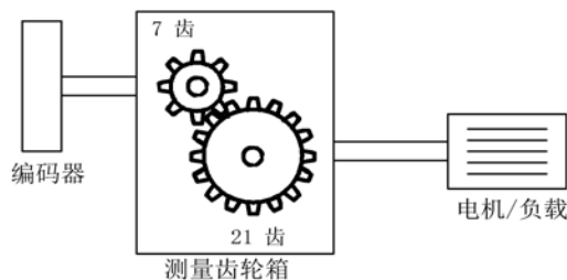
图 7-14 测量齿轮箱
