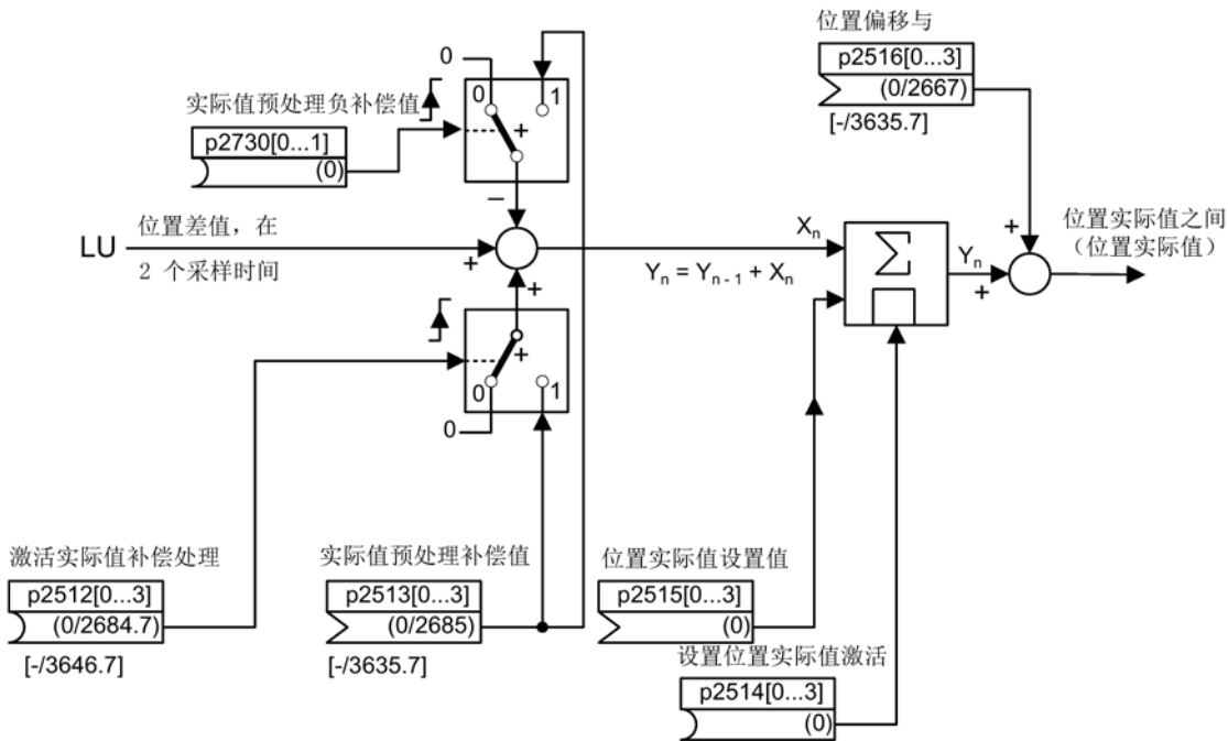
图 8-8 位置实际值处理
