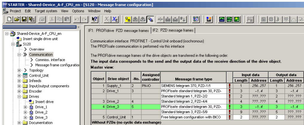
图 11-39 显示报文状态
