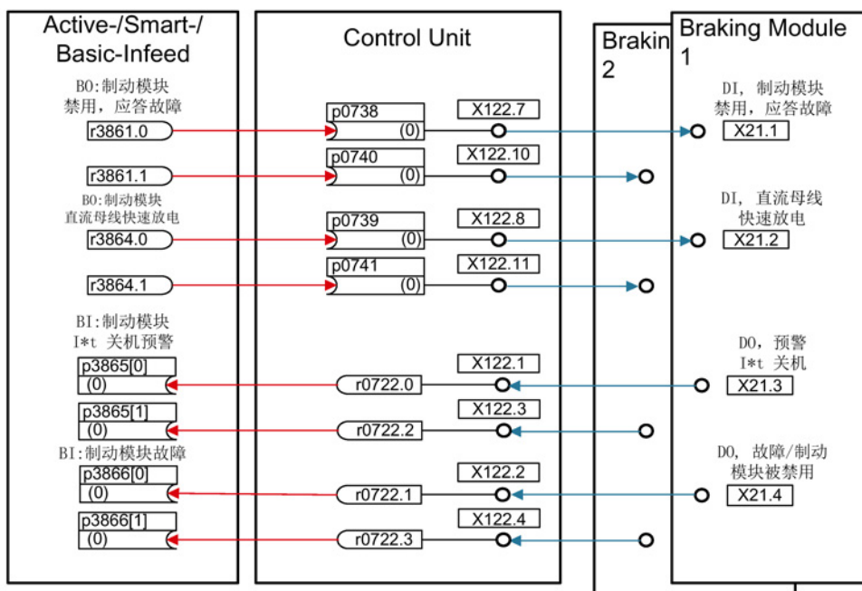
图 8-5 示例：控制 2 个书本型制动模块
