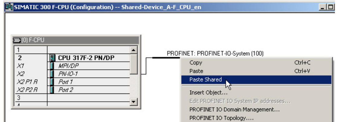
图 11-43 PROFI-safe 控制系统配置
