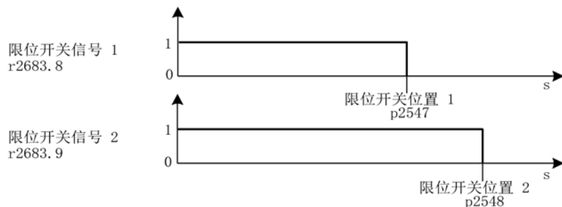
图 8-12 限位开关
