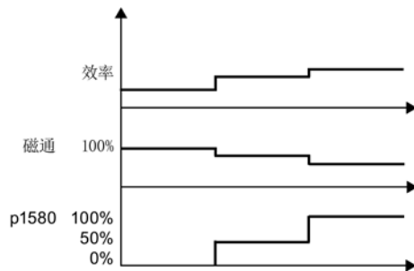
图 5-22 简单效率优化
