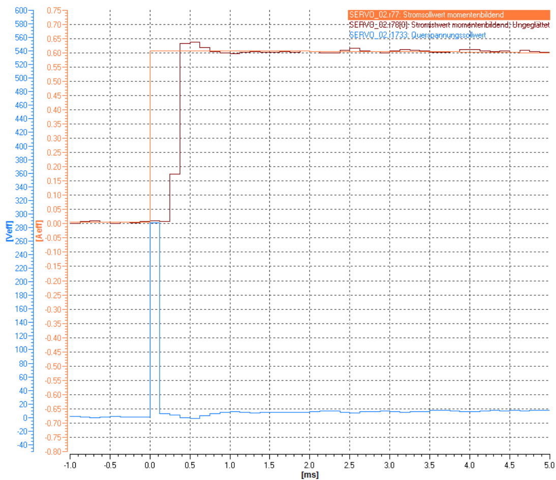
图 4-31 电压前馈控制 p1703 太大
