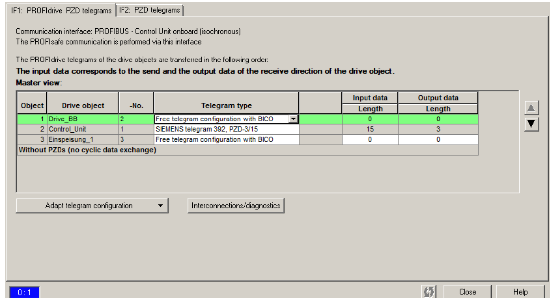
图 11-1 PZD 报文
