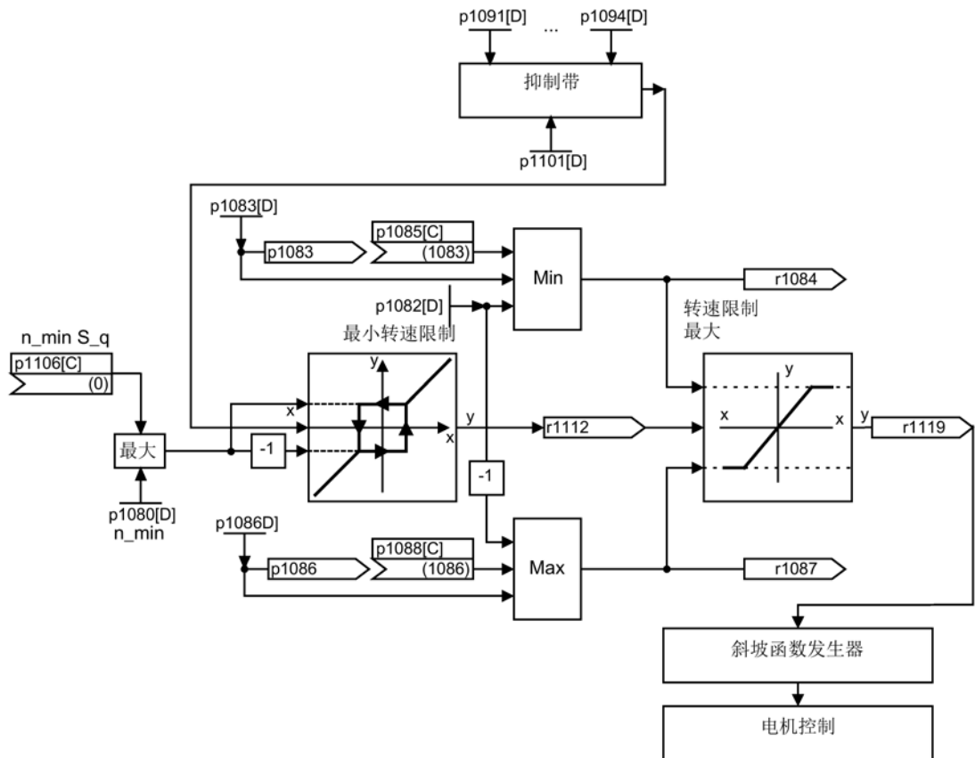
图 3-7 回避带，设定值限制，最小转速
