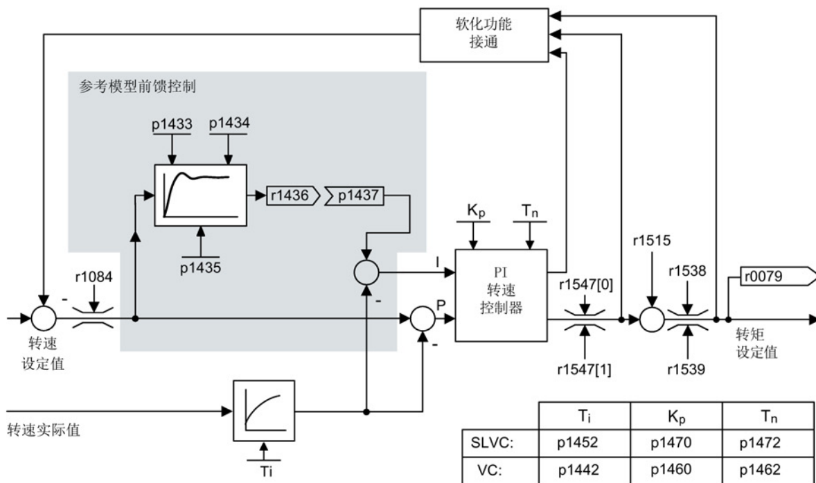
图 5-10 参考模型
