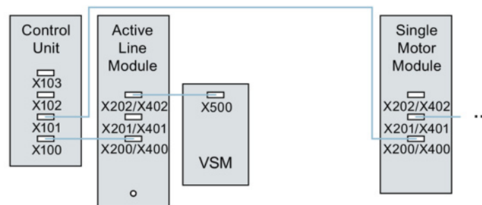
图 13-26 书本型和装机装柜型组件带有 VSM 的拓扑示例
