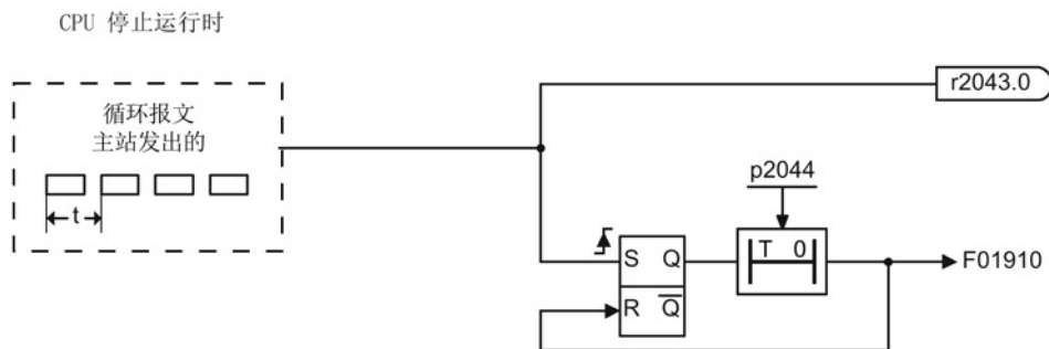
图 11-16 CPU 停止运行时的报文故障监控
