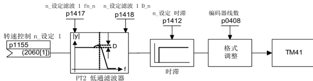
图 7-18 编码器仿真功能图
