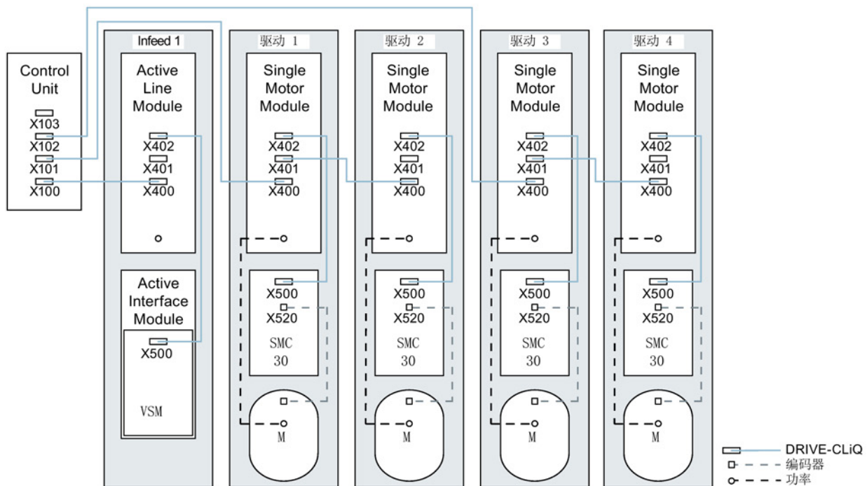
图 A-2 脉冲频率不同的驱动组（装机装柜型）
