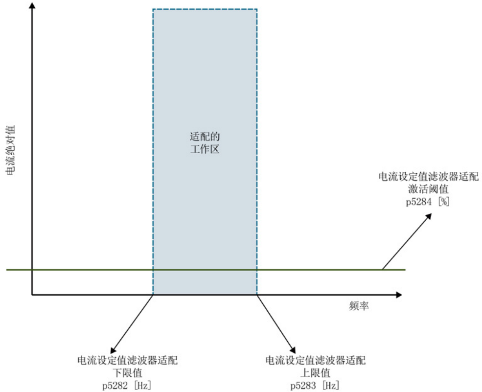
图 4-11 工作原理
