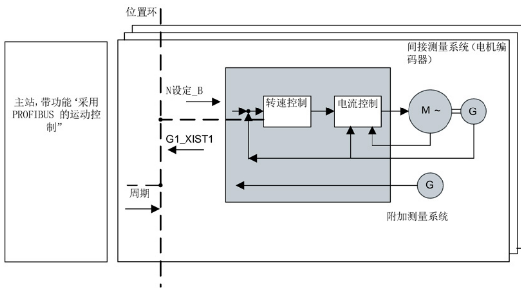
图 11-6 “采用 PROFIBUS 的运动控制”概览（示例：控制器和 3 种设备）
