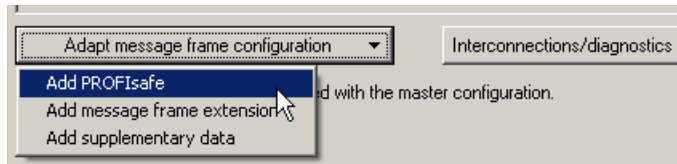
图 11-38 为驱动添加 PROFIsafe 报文
