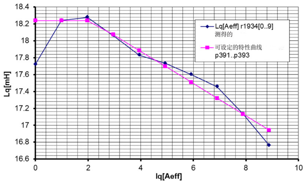
Lq 特性曲线
