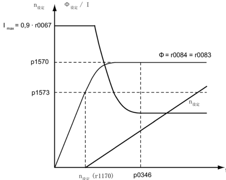
图 5-23 快速励磁的特性曲线
