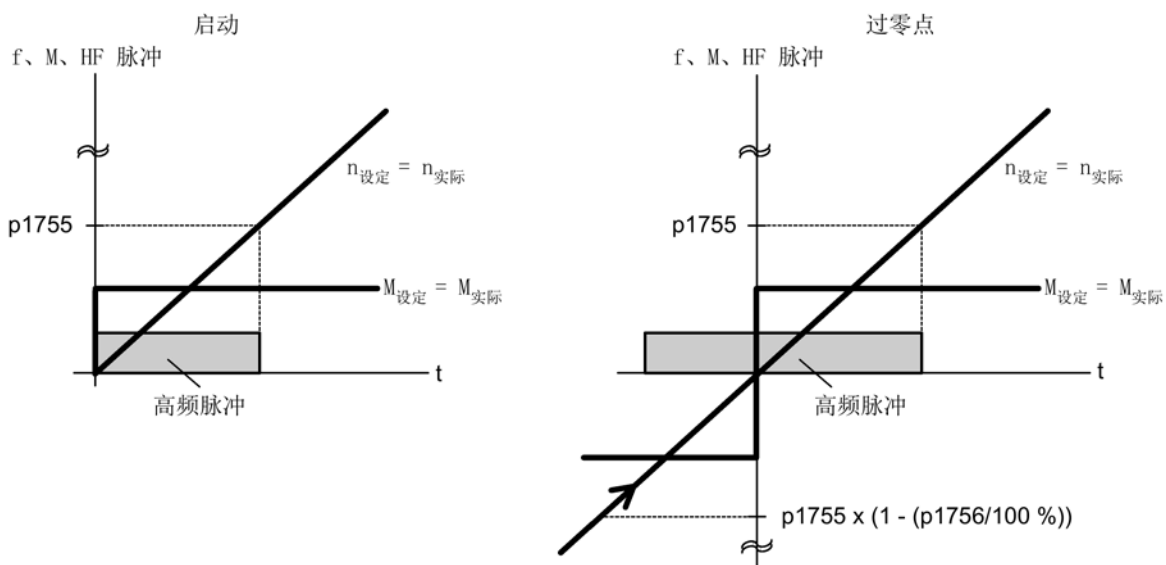
图 5-5 “零速前一直保持闭环控制”中的过零点
