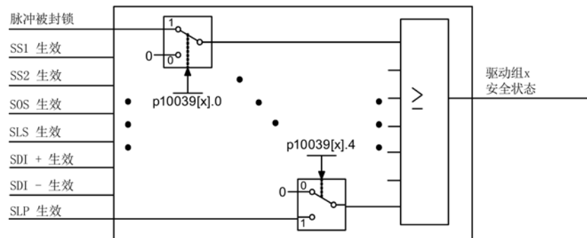
图 10-5 安全状态选择（扩展功能示例）
