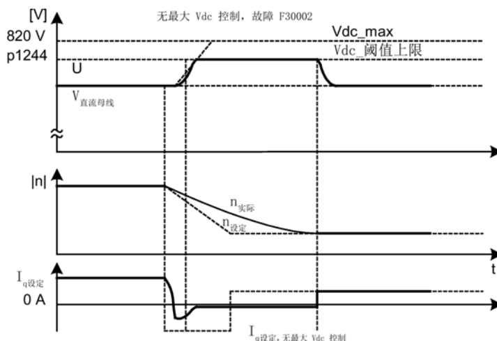
图 4-20 V dc_max 控制的激活/取消
