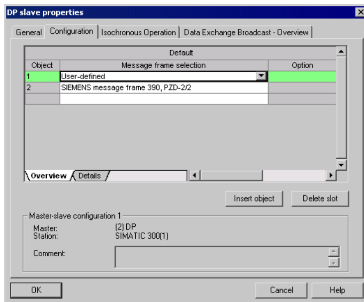
图 11-26 “从站-从站”通讯时的报文分配
