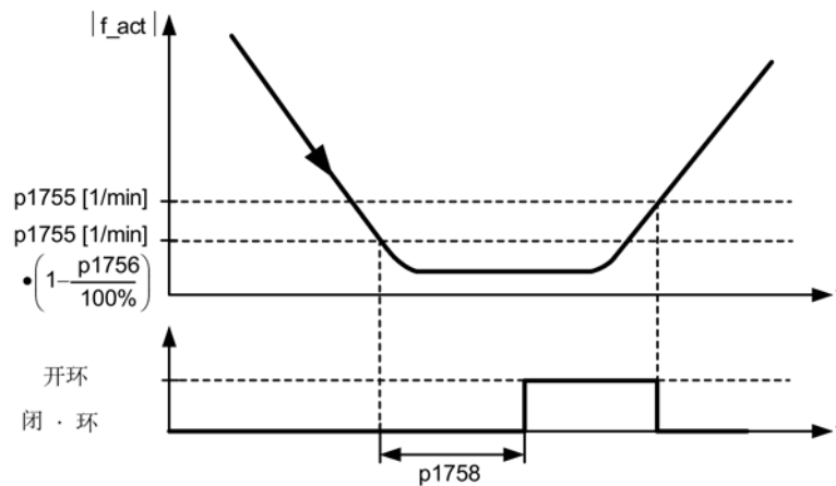
图 5-1 SLVC 的切换前提
