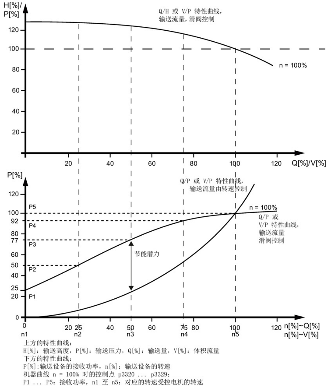
图 7-8 节能潜力
