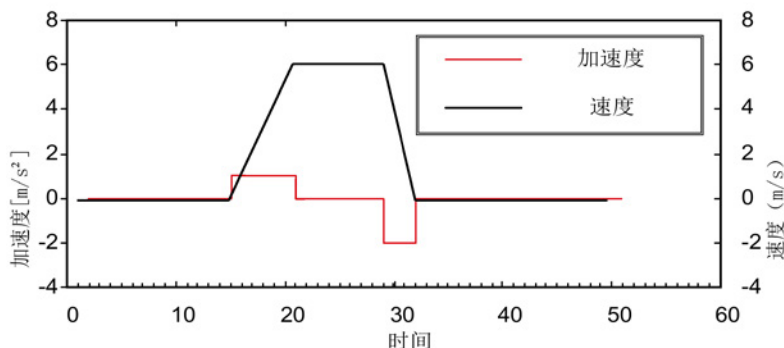
图 8-15 没有加加速度限制
