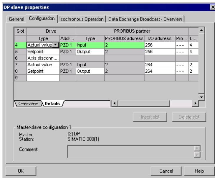
图 11-22 从站配置的信息视图
