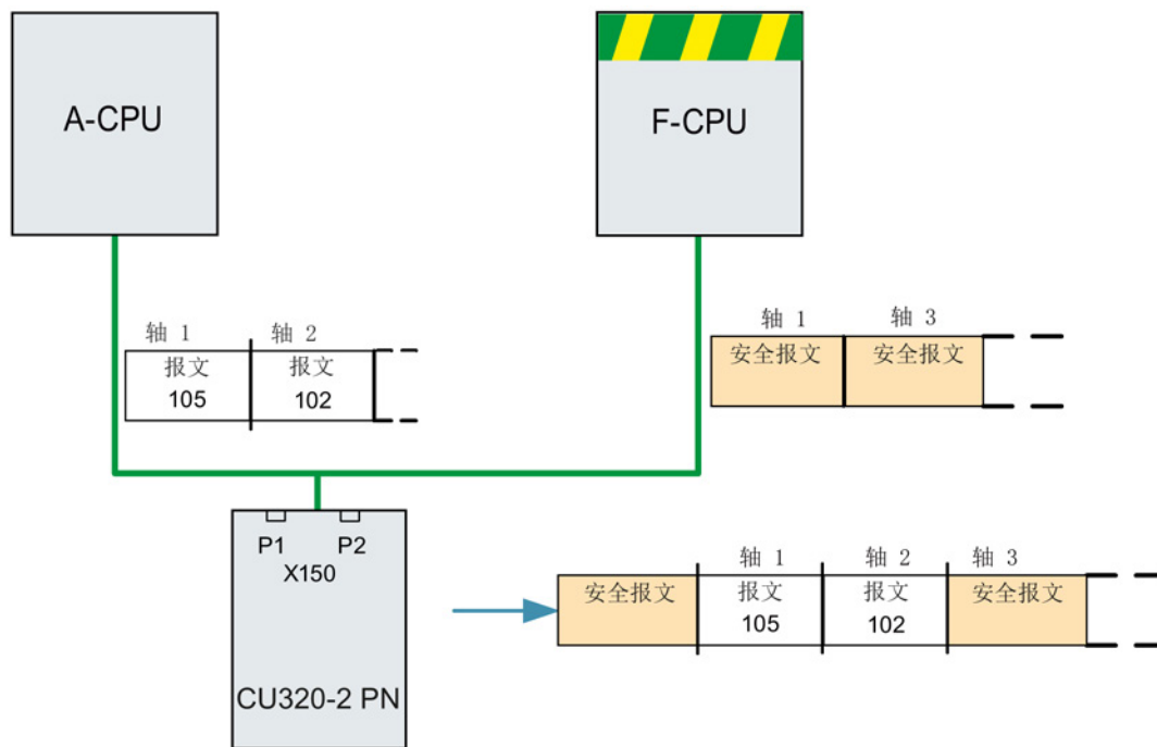
图 11-33 通讯流程示例
