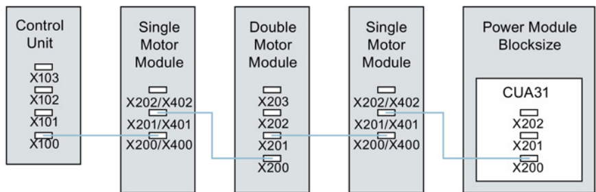
图 13-25 DRIVE-CLiQ 支路示例
