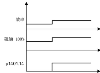
高级效率优化，增大磁通
