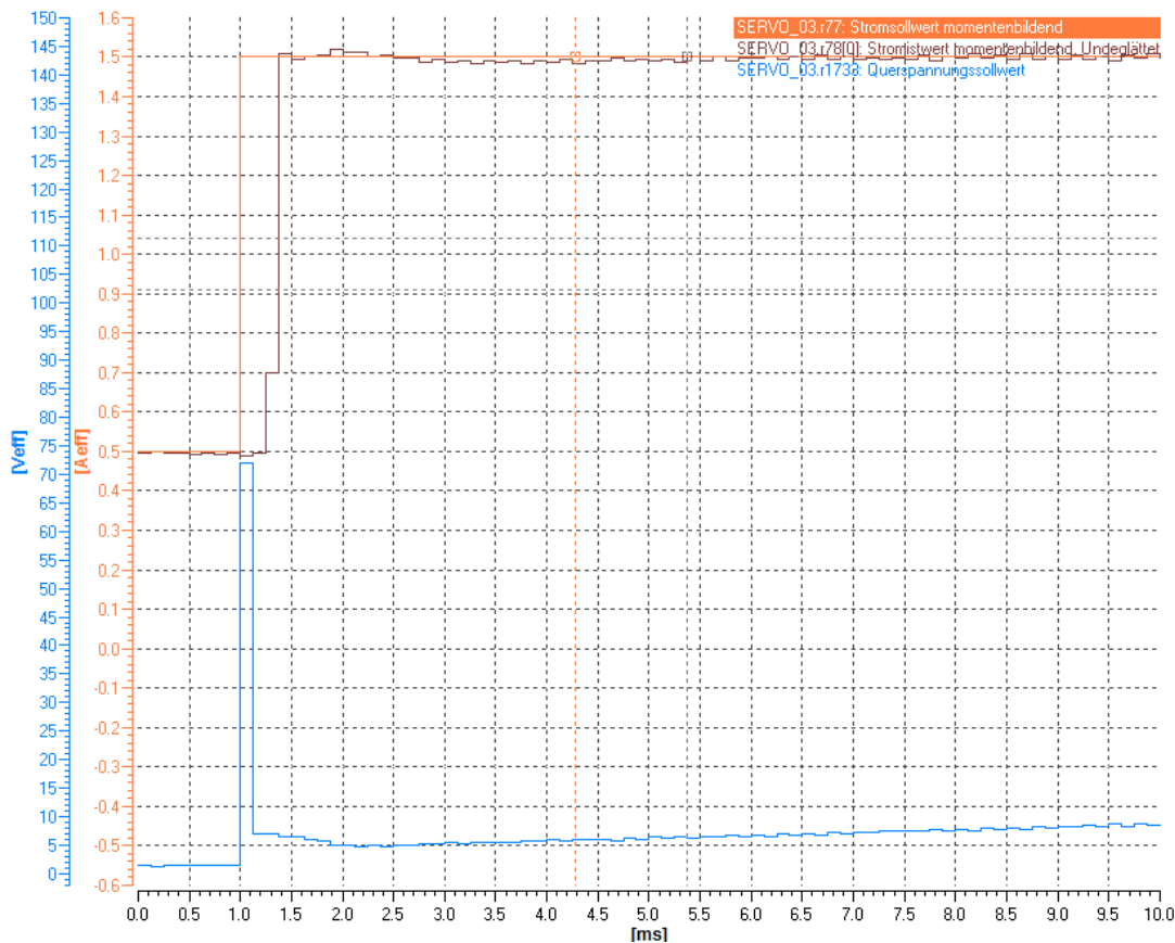
图 4-34 示例：优化之后
