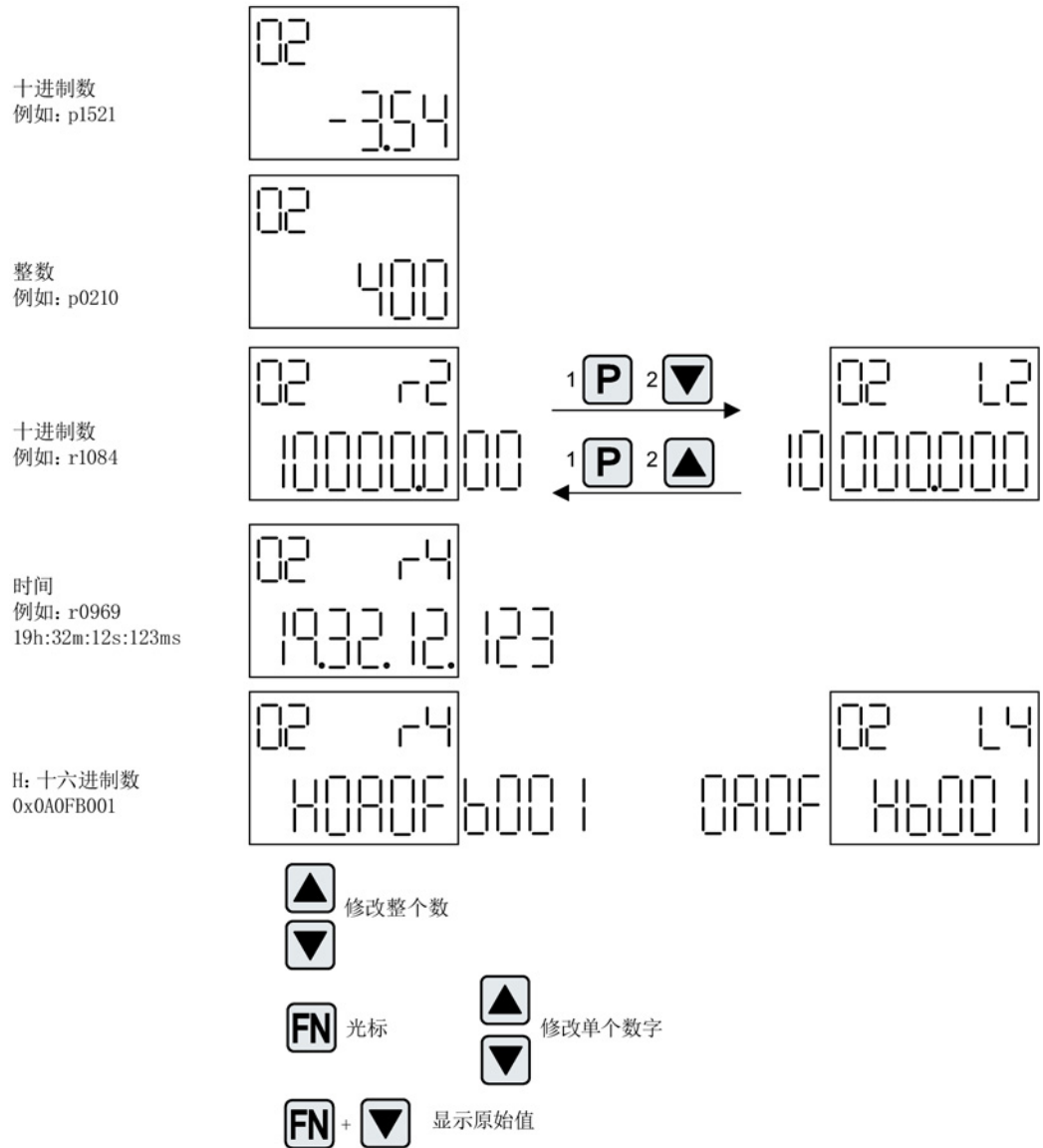
图 A-10 数值显示
