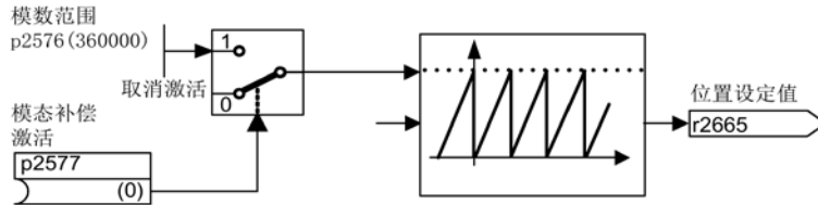
图 8-14 模态补偿
