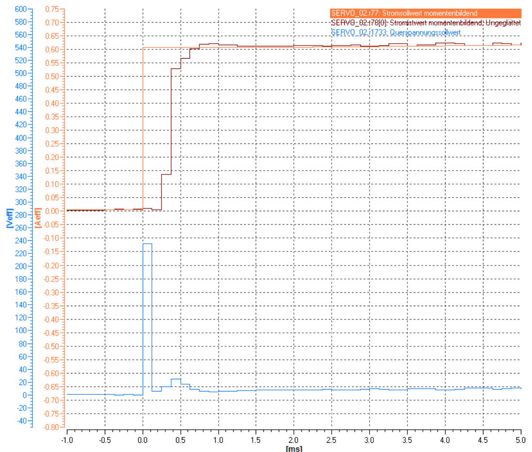
图 4-29 电压前馈控制 p1703 太小
