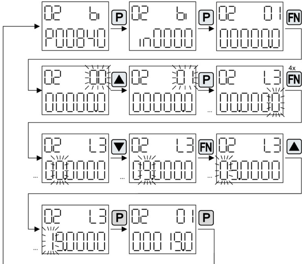
图 A-12 示例：修改带索引的二进制互联参数
