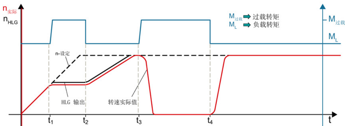
图 3-11 斜坡函数发生器跟踪标准
