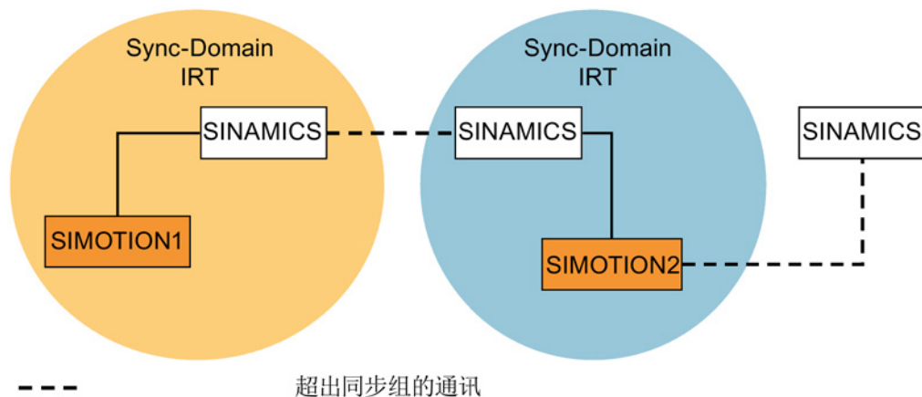
图 11-30 超出同步组极限实现实时同步
