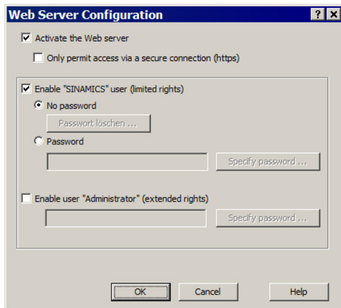
图 7-26 以缺省设置配置网络服务器
