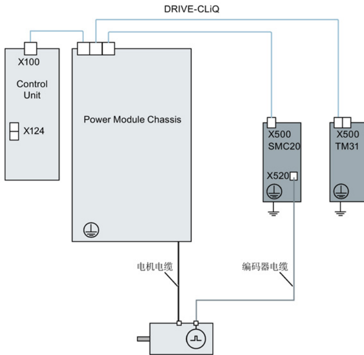
图 A-5 装机装柜型功率模块构成的驱动系统
