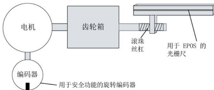
图 8-21 举例 2: EPOS和安全回参考点, 线性
