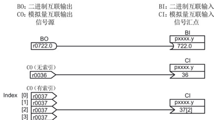
图 13-10 使用 BICO 技术互联信号
