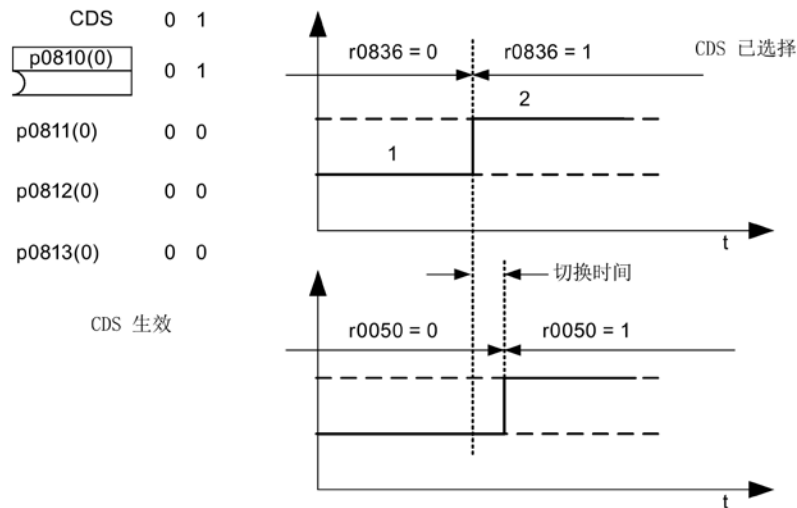
图 13-14 切换指令数据组（示例）
