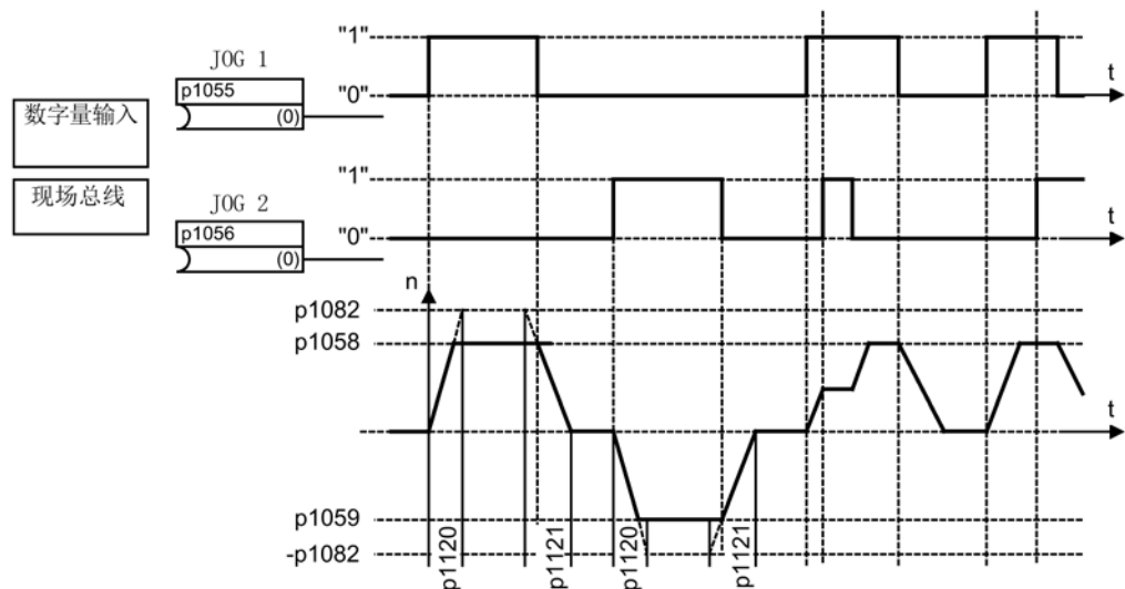
图 3-4 JOG 1 和 JOG 2 的流程图
