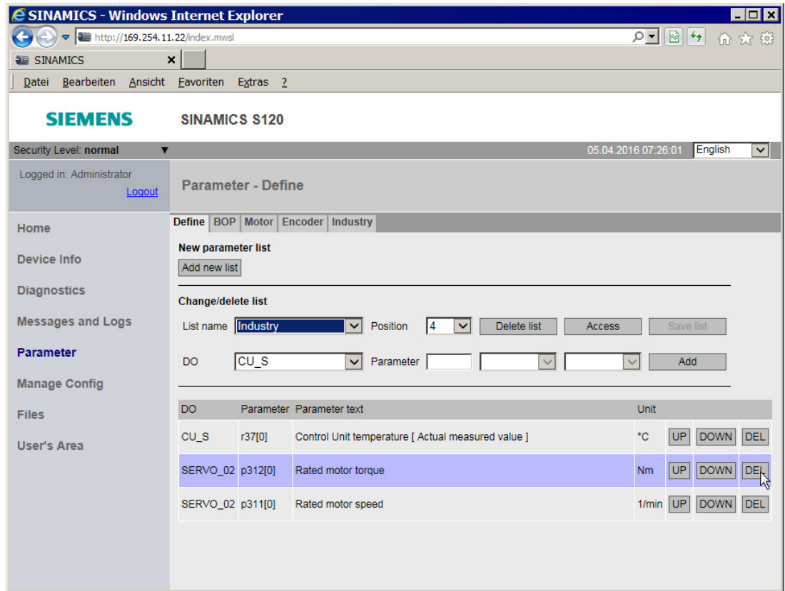
图 7-41 驱动参数 - 删除单个表
