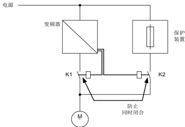
图 5-29 线路示例：不带同步的旁路
