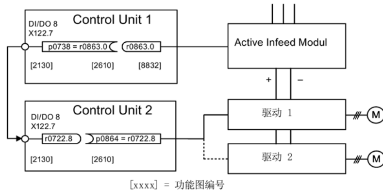
图 12-4 示例：多个控制单元的互联
