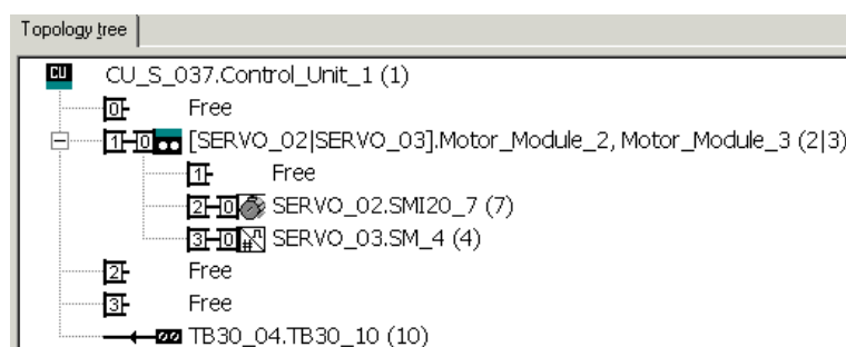
图 13-24 STARTER 中的拓扑结构视图
