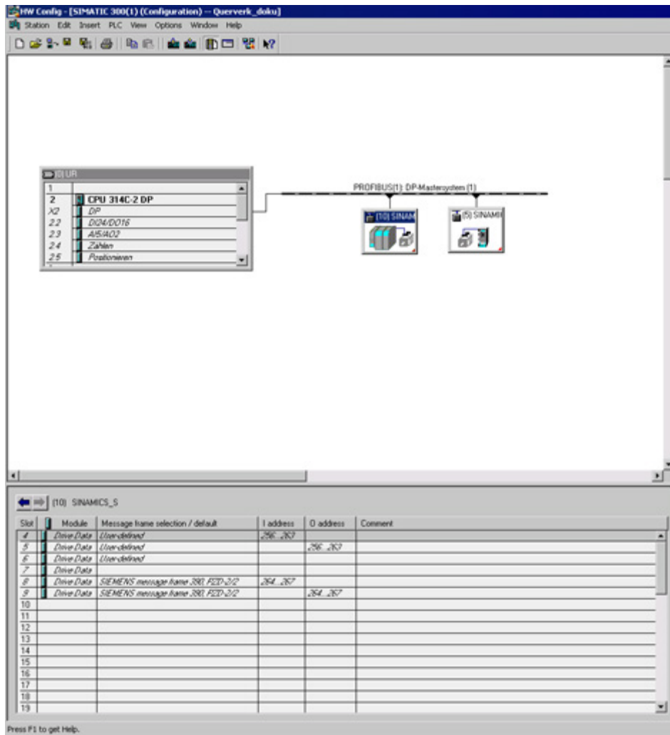
图 11-20 “HW-Config”中 PROFIBUS 网络的项目示例
