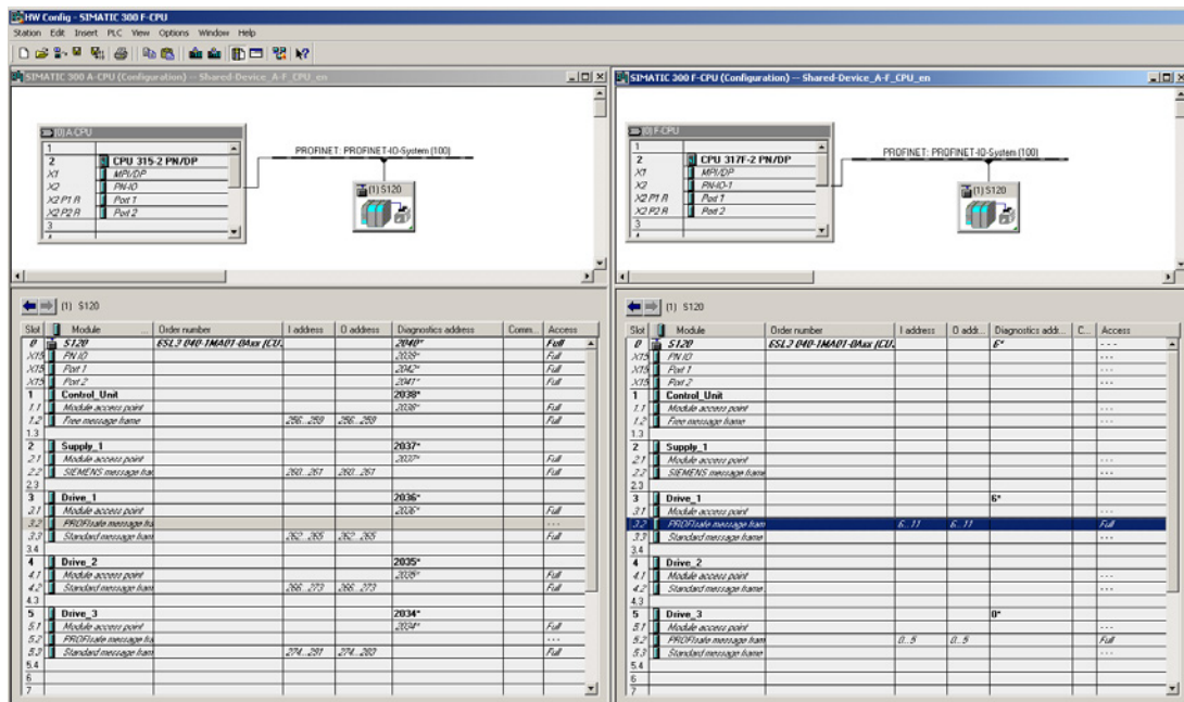
图 11-44 HW-Config 中完成配置的新项目
