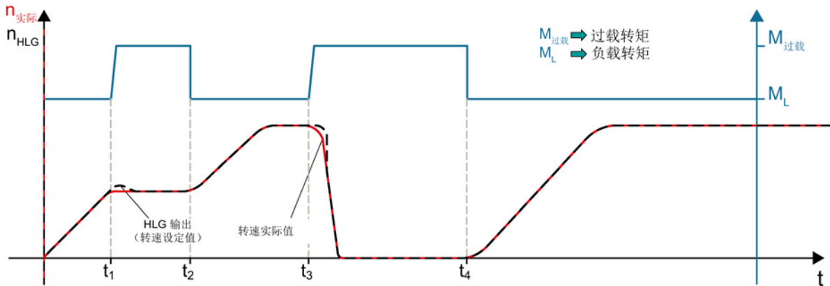
图 3-12 扩展斜坡函数发生器跟踪
