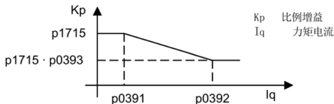
图 4-10 电流控制器适配
