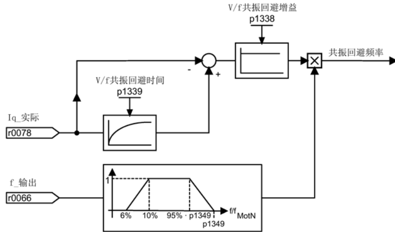
图 6-6 谐振抑制
