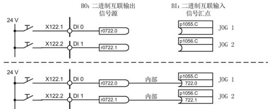
图 13-12 互联数字信号（示例）
