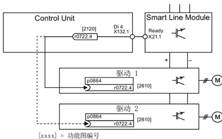
图 12-3 示例：没有 DRIVE-CLiQ 的调节型电源模块的互联
