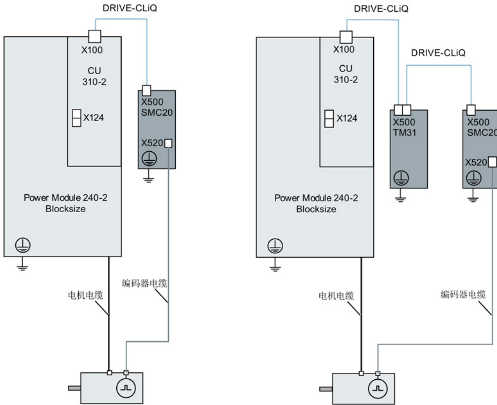
图 A-4 模块型功率模块构成的驱动系统
