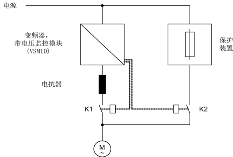
图 5-26 电路示例：带同步和重叠的旁路
