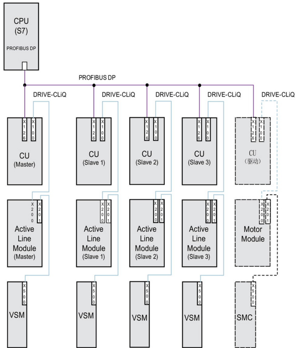
图 8-23 拓扑结构和 PROFIBUS 通讯网络：带冗余电源模块的主从运行，4 条电源支路
