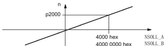
图 11-2 转速定标
