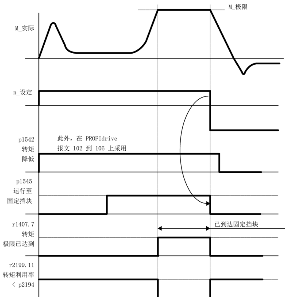
图 4-22 “运行到固定停止点”时的信号图
