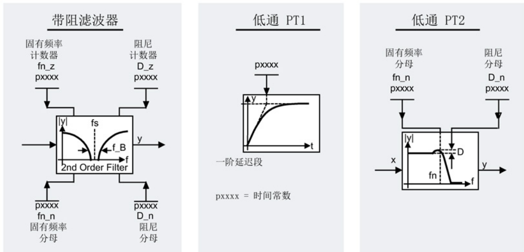
图 4-2 转速设定值滤波器概述
