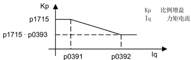
图 5-17 电流控制器适配： p0393 < 1 , p0391 < p0392
