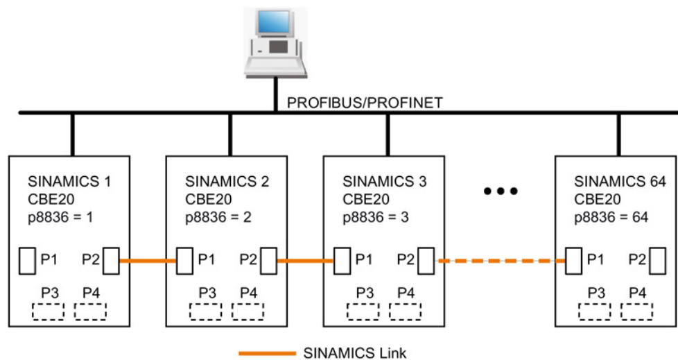
图 11-51 最大拓扑结构
