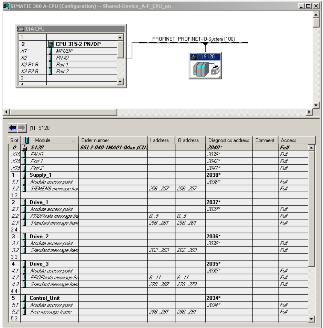
图 11-41 HW-Config 中更新过的项目
