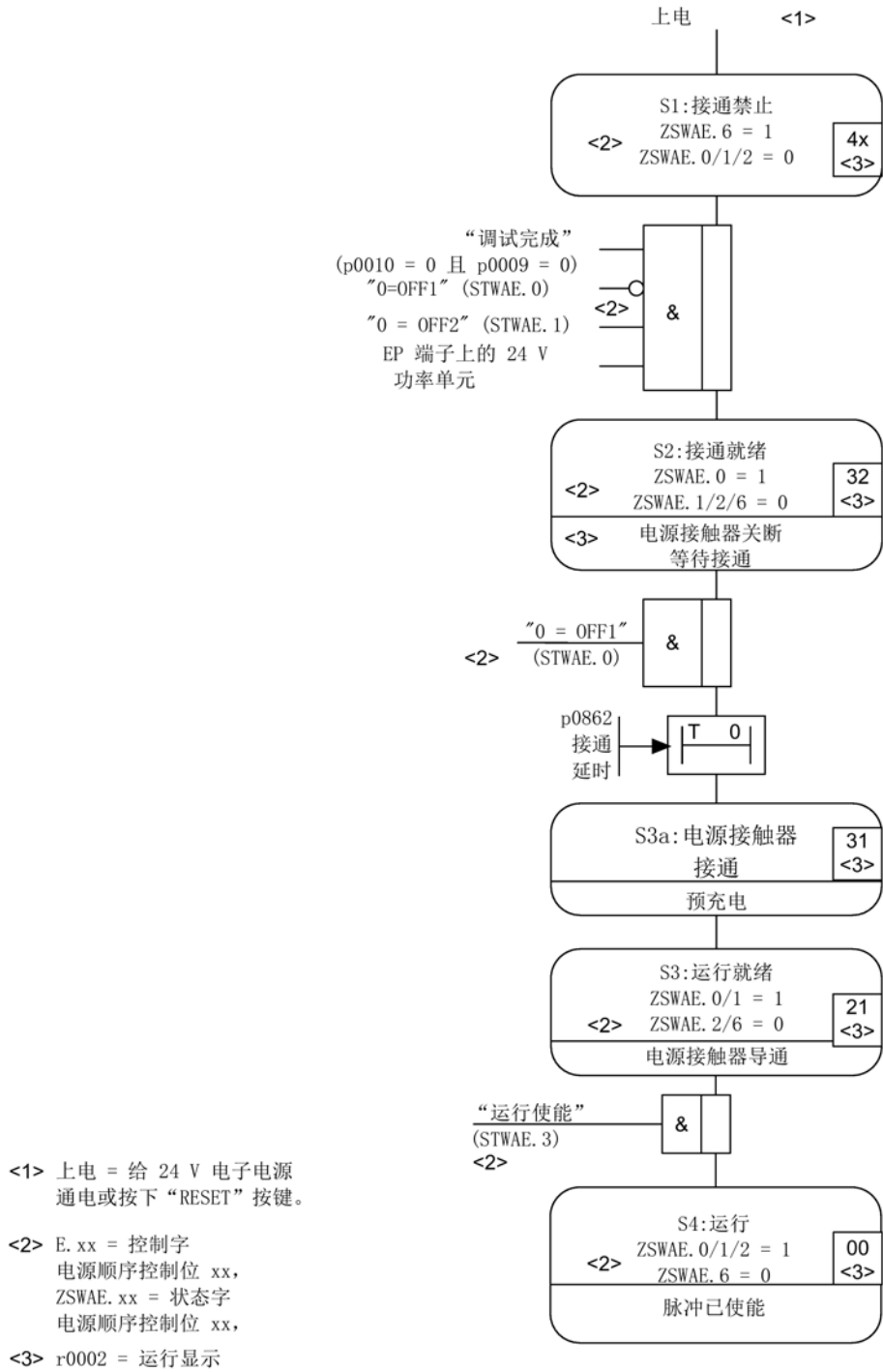
图 2-6 非调节型电源的启动过程
