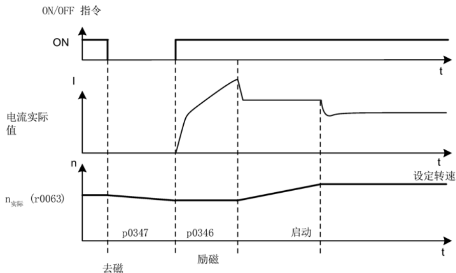
图 5-25 示例：捕捉重启，用于带编码器异步电机
