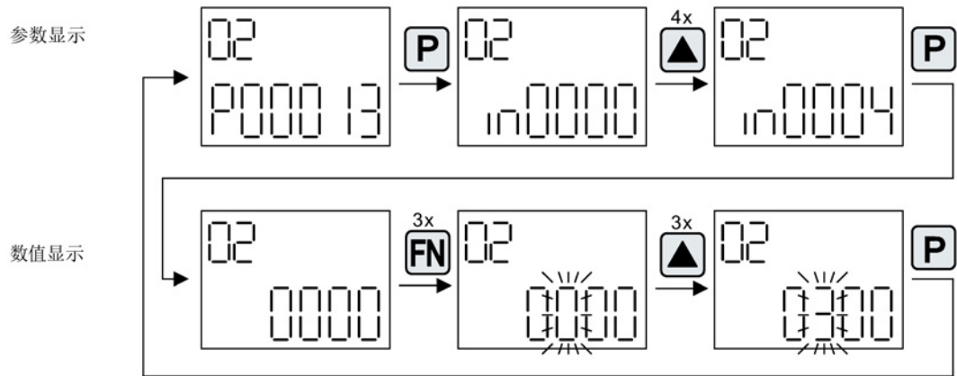
图 A-11 示例：将 p0013[4] 从 0 修改到 300
