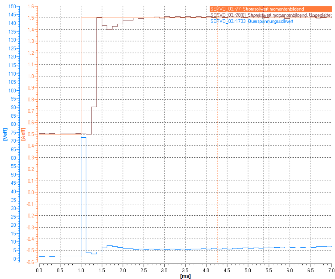
图 4-32 示例：优化前的电压前馈控制，有电压骤降现象
