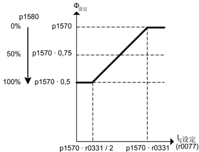
图 5-21 效率优化
