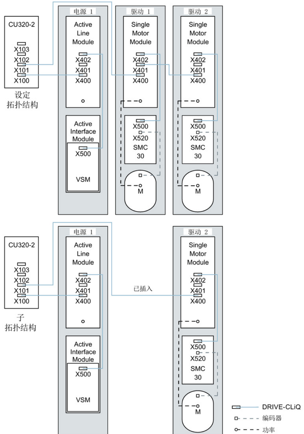
图 13-27 部分拓扑结构示例
