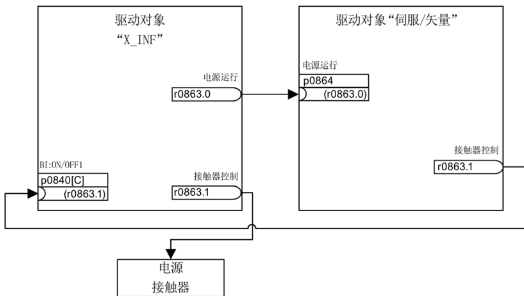
图 12-1 BICO 互联：通过驱动接通电源
