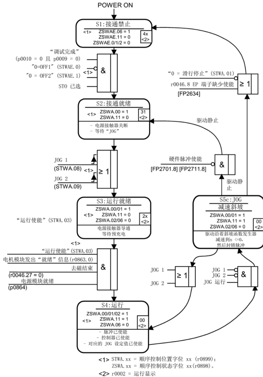
图 3-5 JOG 流程图
