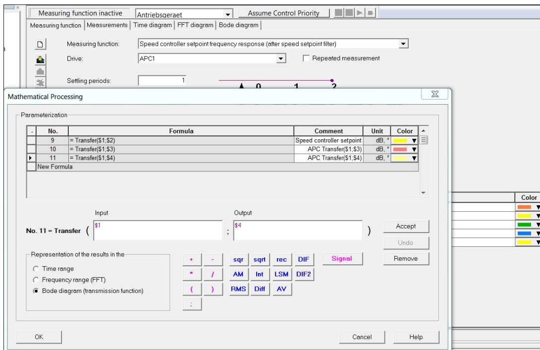
图 8-48 传递函数
