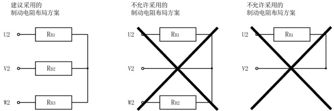
图 7-5 制动电阻
