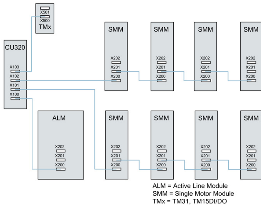
图 A-7 V/f 控制中矢量驱动系统的拓扑示例
