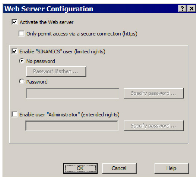
图 7-27 以缺省设置配置网络服务器
