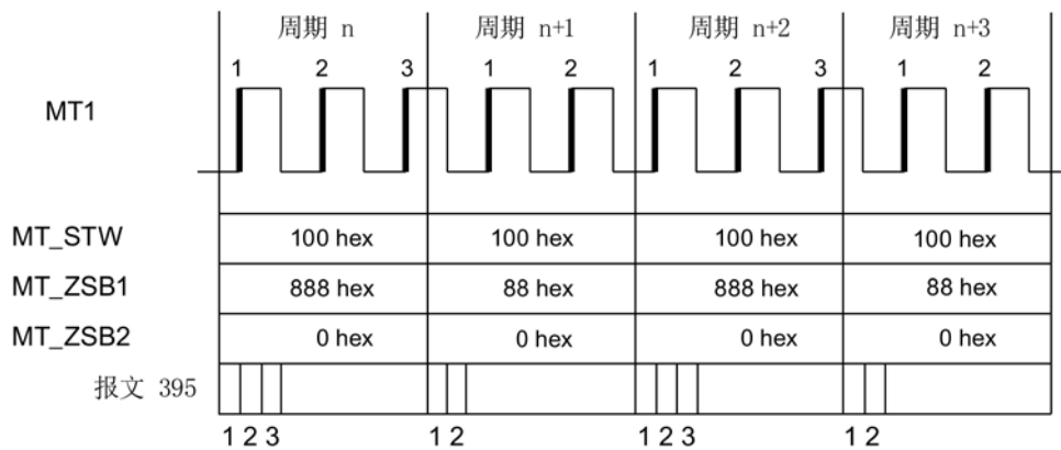
图 4-24 搜索测头 1 的上升沿
