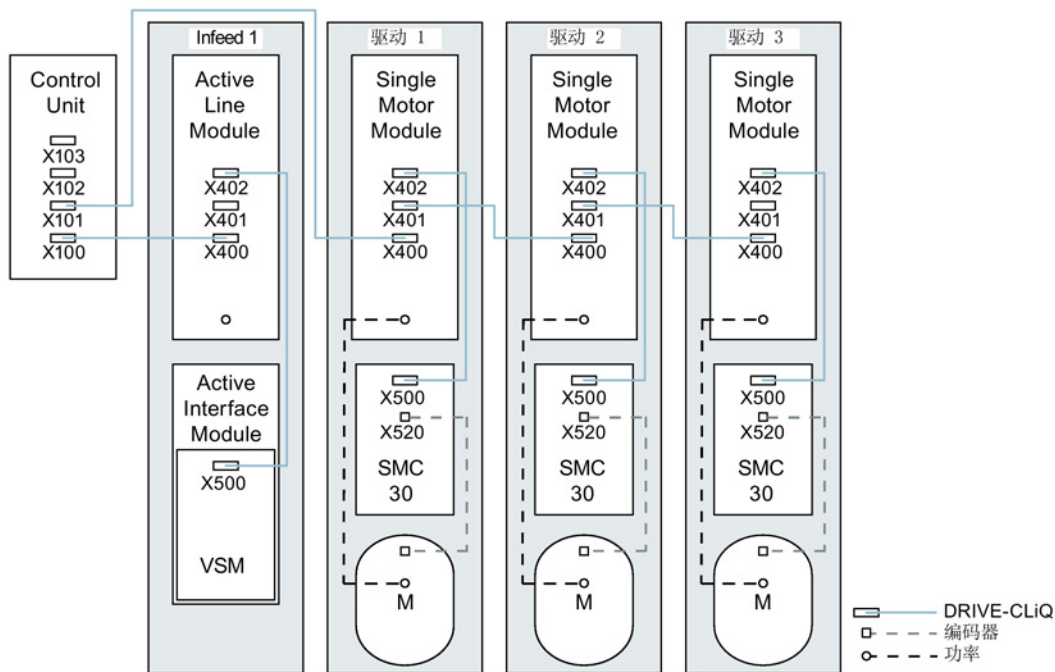
图 A-1 脉冲频率相同的驱动组（装机装柜型）
