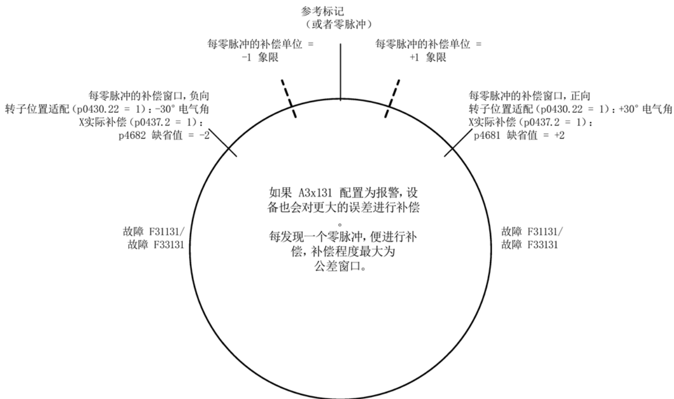
图 7-10 公差带和补偿
