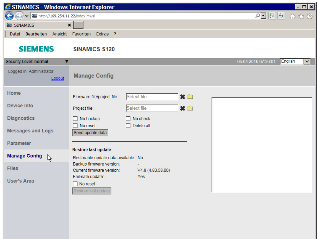
图 7-24 网络服务器显示区：Manage Config：只有在操作之后才会显示右侧状态
