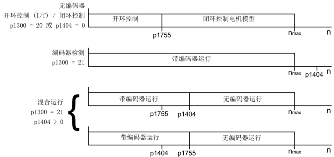
图 4-16 区域切换
