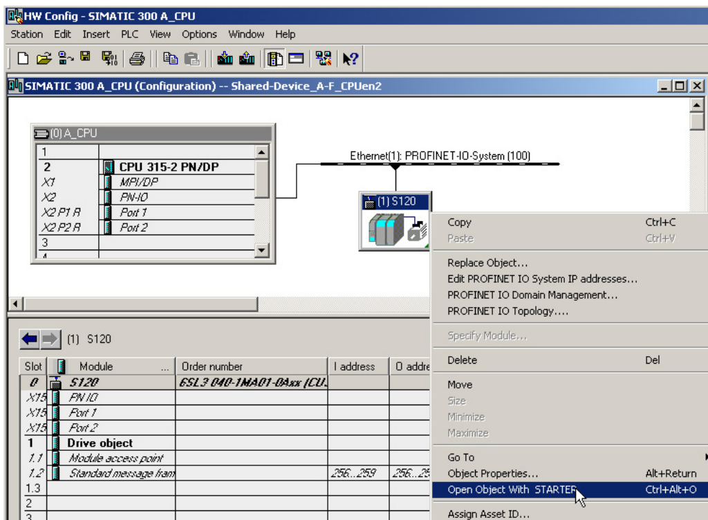
图 11-36 将新项目从 HW-Config 传输至 STARTER
