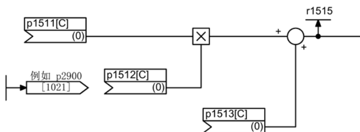
图 4-6 转矩设定值
