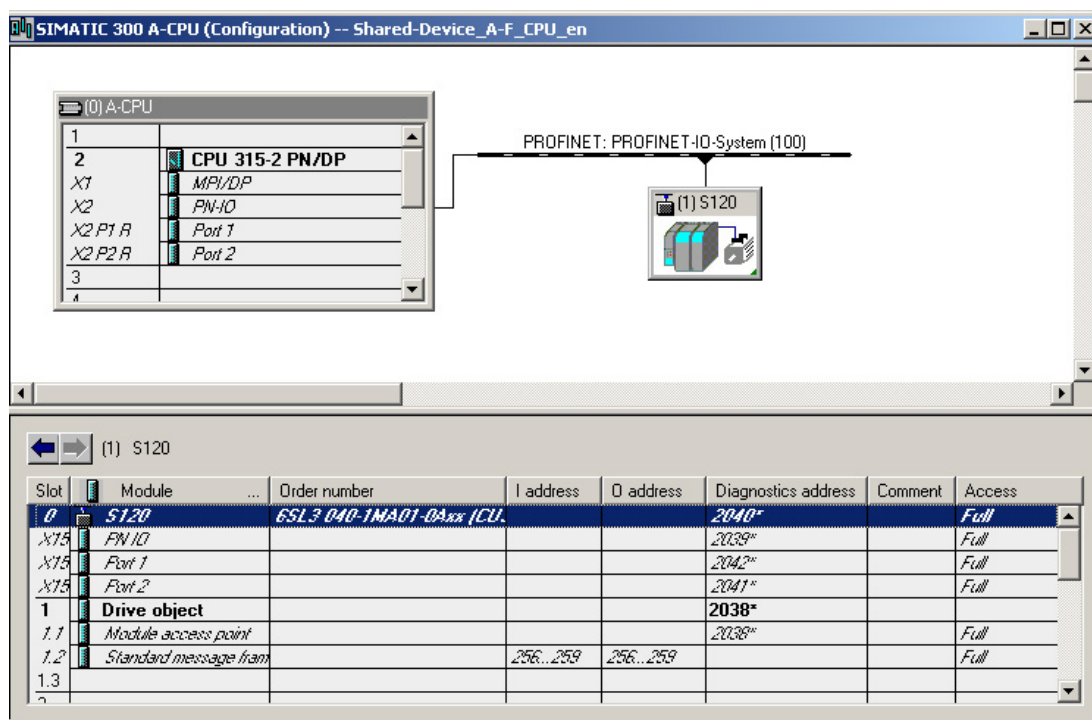
图 11-35 已在 HW-Config 中创建了自动化控制器
