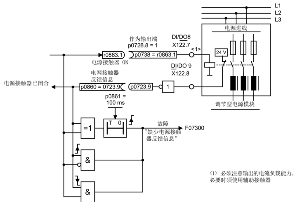
图 2-10 电源接触器控制
