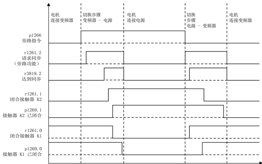
图 5-27 信号图：带同步和重叠的旁路
