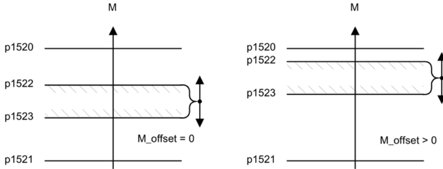
图 4-8 示例：带或不带偏移的转矩极限
