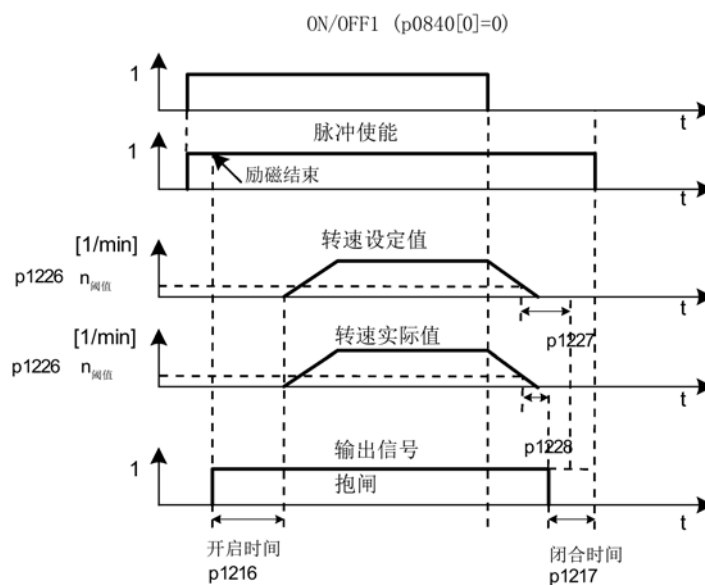
图 7-7 简单制动控制的时序图
