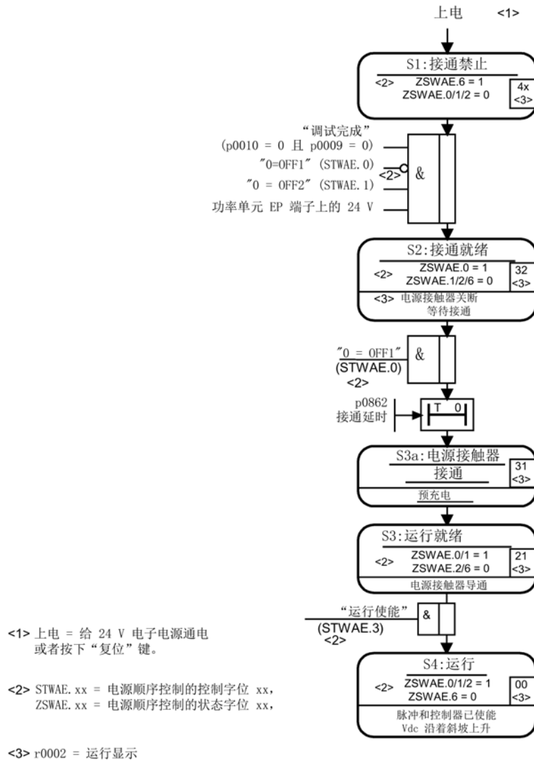
图 2-3 调节型电源的启动过程
