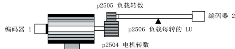
图 8-6 使用旋转编码器采集位置实际值
