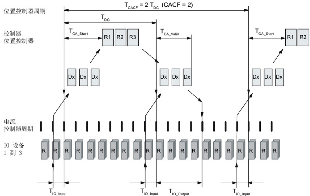
图 11-31 采用 PROFINET 的运动控制/等时同步驱动耦合，周期经过优化，CACF（Controller Application Cycle Factor，控制器应用循环系数）= 2
