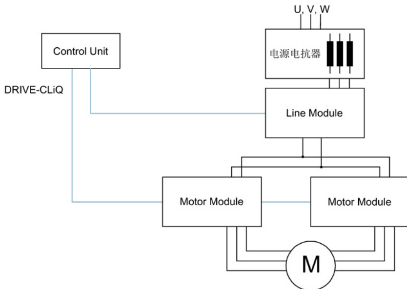
图 8-26 示例 1：并联
