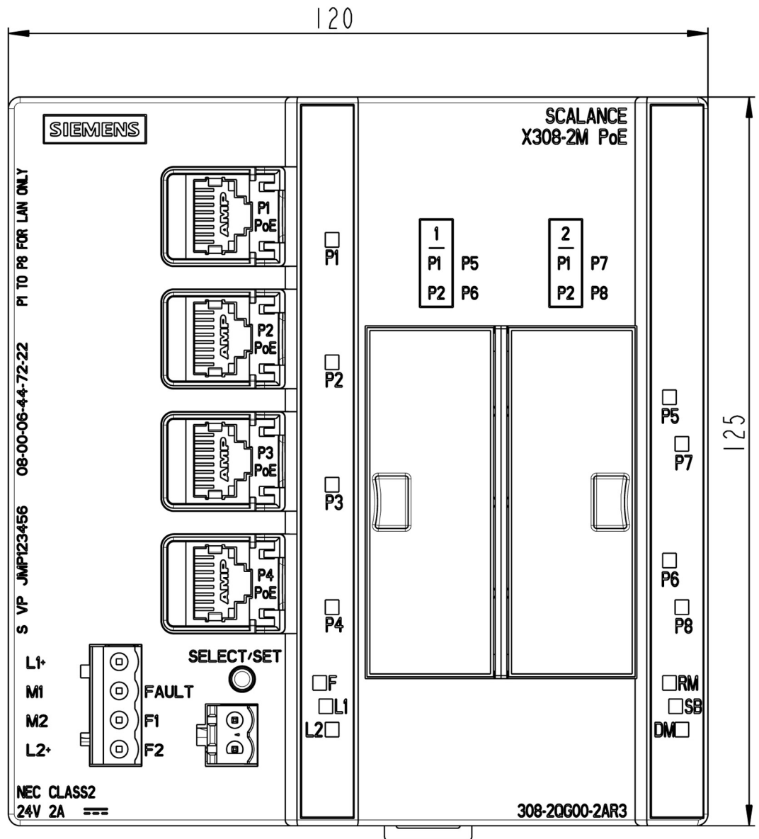
图 11-32 X308-2M PoE: 正视图
