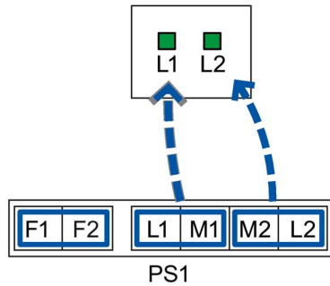
图 6-5 设备具有一个电源单元时 LED 指示灯与冗余电源引脚的分配
