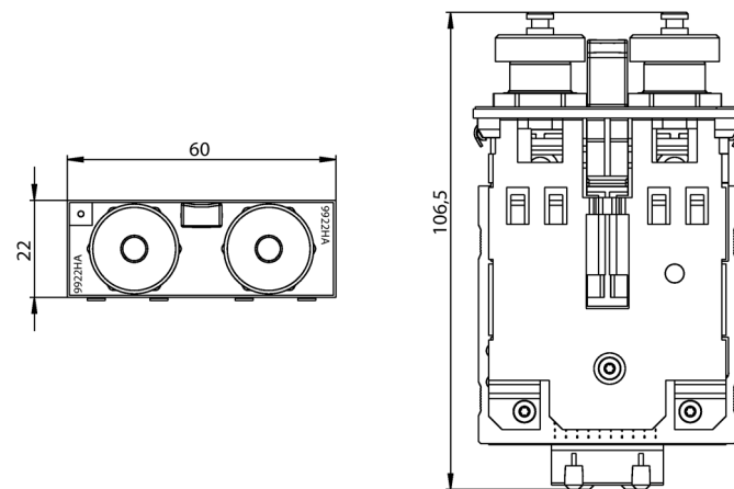
图 11-29 MM900 尺寸图 6: M12 电气端口
