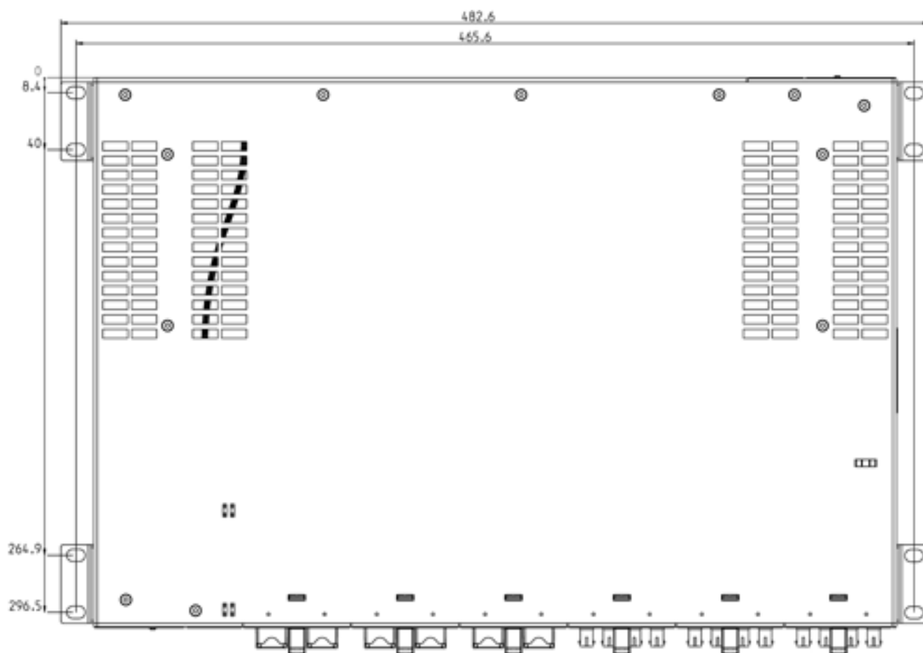
图 11-12 XR324-12M 的俯视图
