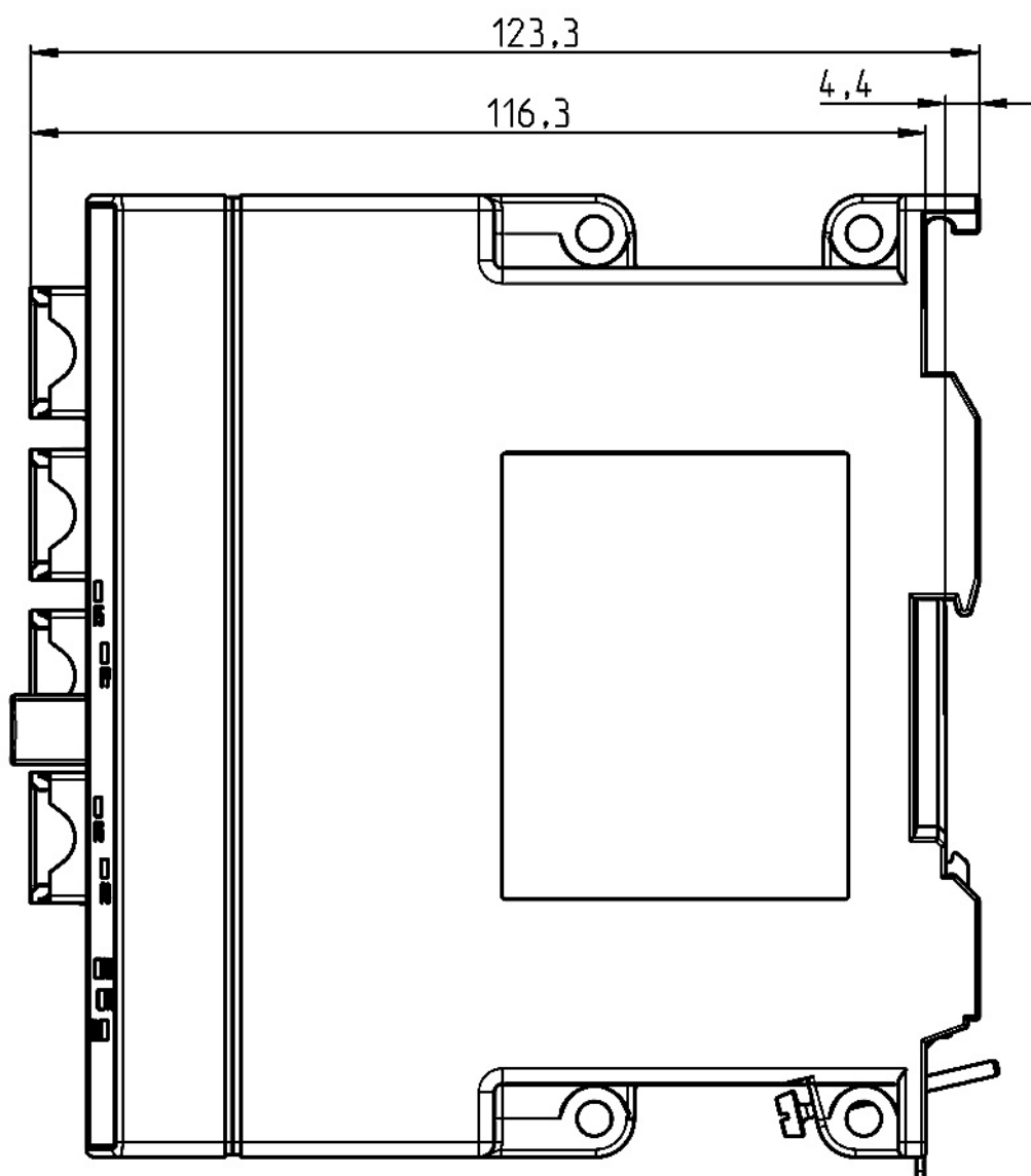
图 11-33 X308-2M PoE: 侧视图
