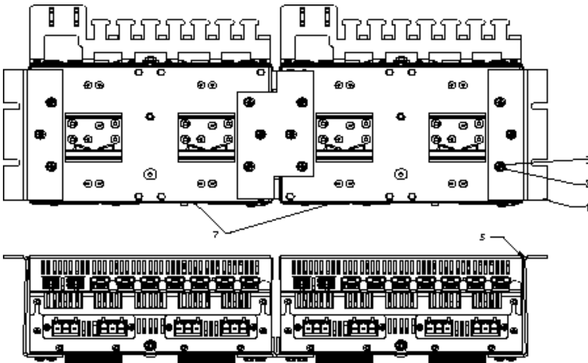
图 5-3 两个固定在一起的 IE Switch X-300EEC 的机架安装 上面的图：交换机的后面 下面的图：仰视图
