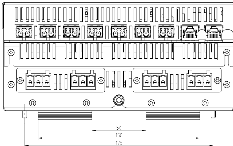
图 11-15 IE Switch X302-7EEC 尺寸图 - 俯视图
