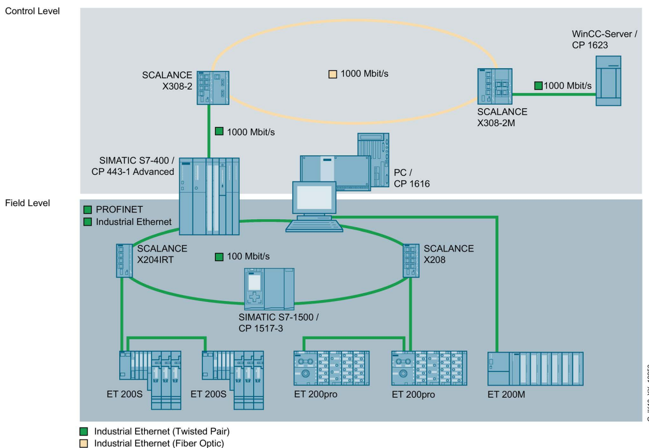
图 3-3 具有冗余管理器 (RM) 的环网
