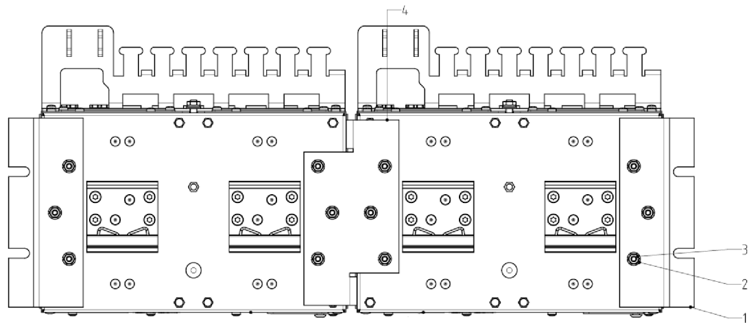
图 11-21 两个固定在一起的 X-300EEC 的机架安装（仰视图）
