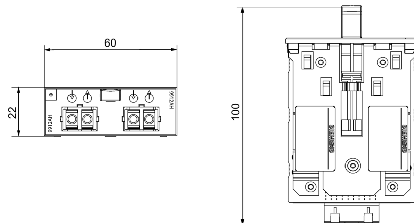
图 11-30 MM900 尺寸图 7: SC RJ 光学端口
