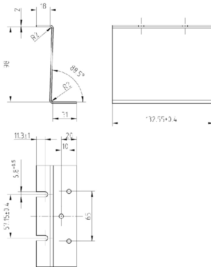
图 11-22 X-300EEC 的安装支架的侧面部分（尺寸以 mm 为单位）
