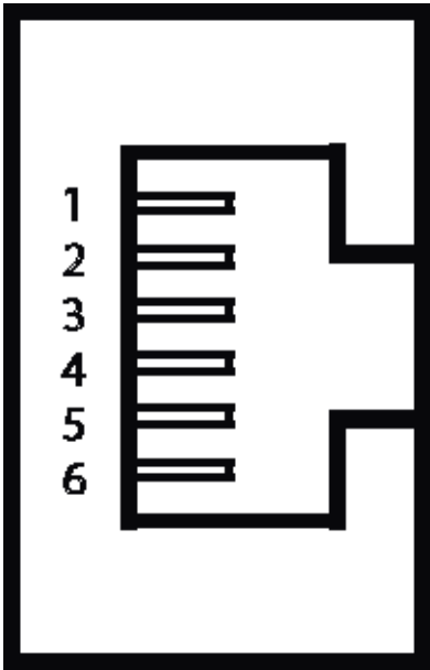
图 7-2 RJ-11 插孔（示意图）
