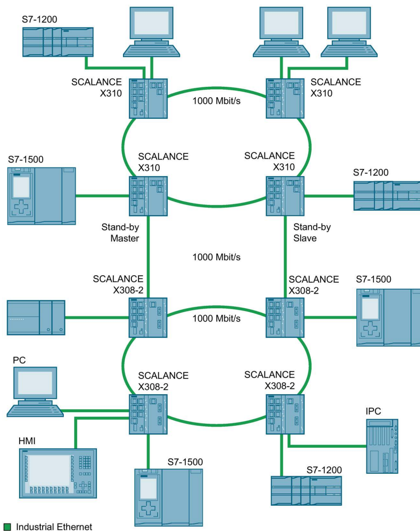
图 3-4 混合使用 SCALANCE X310 和 SCALANCE X308-2 对两个子网进行冗余连接
