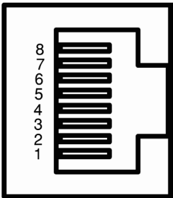
图 A-1 RJ-45 插孔
