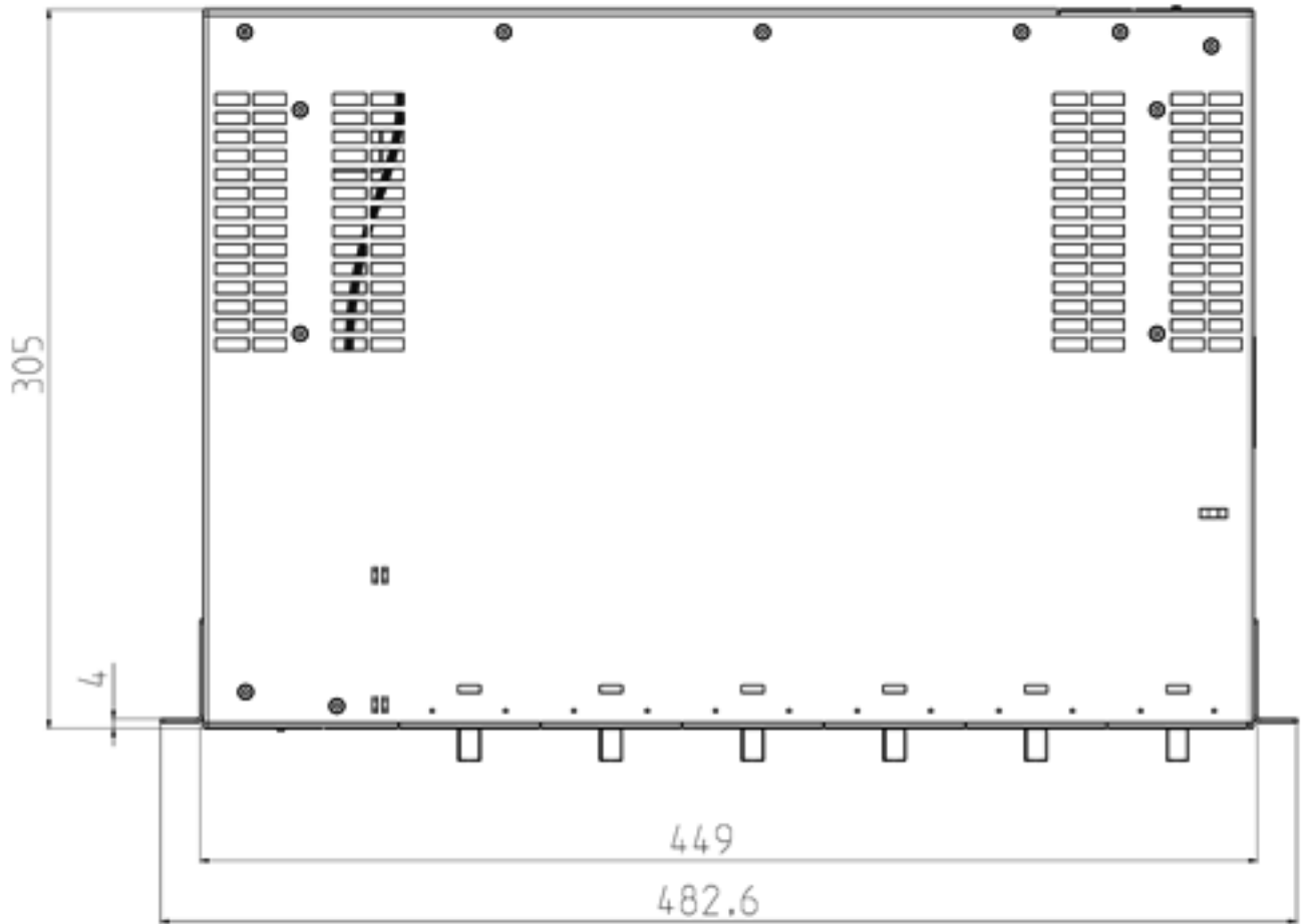
图 11-11 XR324-12M 的俯视图
