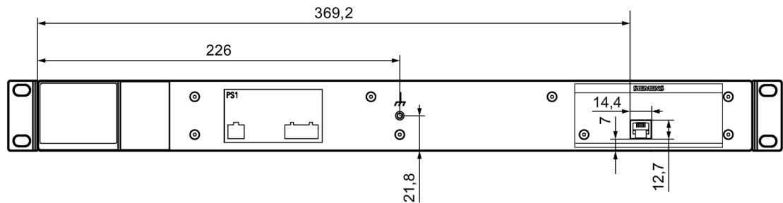
图 11-19 XR324-4M EEC 的示例（1 个 24 VDC，前置电缆出口）
