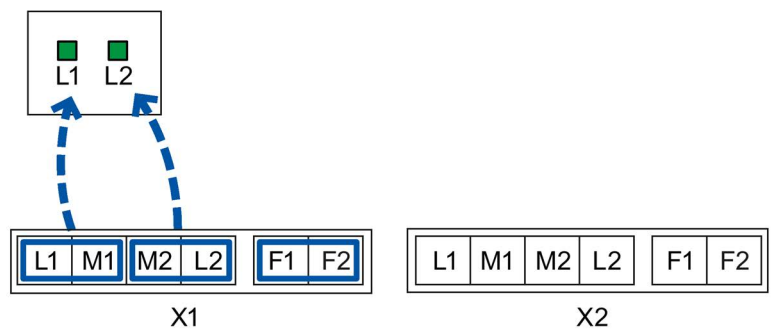
图 6-3 设备具有两个电源单元时 LED 指示灯与冗余电源引脚的分配
