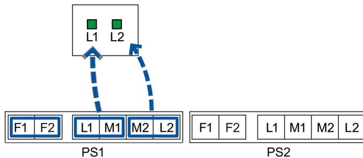
图 6-6 设备具有两个电源单元时 LED 指示灯与冗余电源引脚的分配
