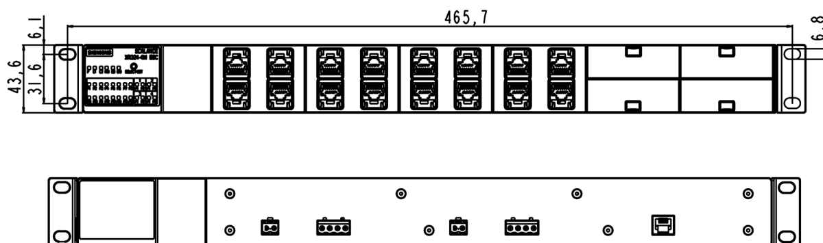
图 11-16 外壳前面和后面
