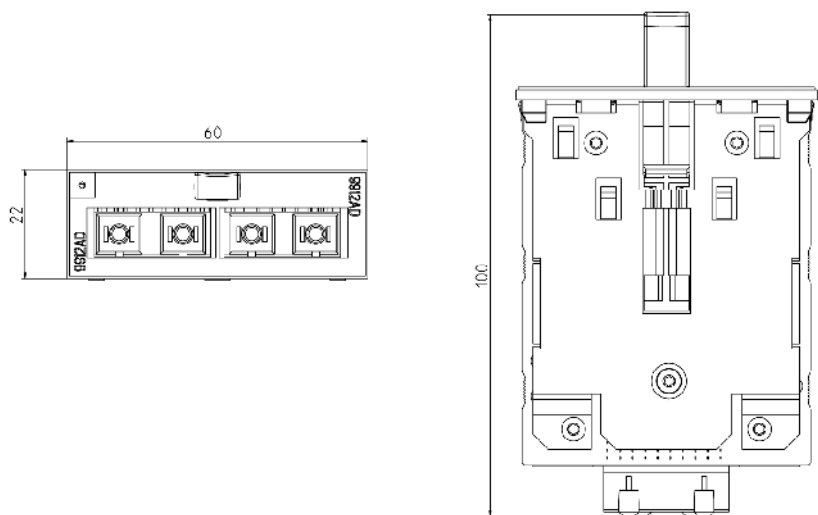
图 11-27 MM900 尺寸图 4: SC 光学端口
