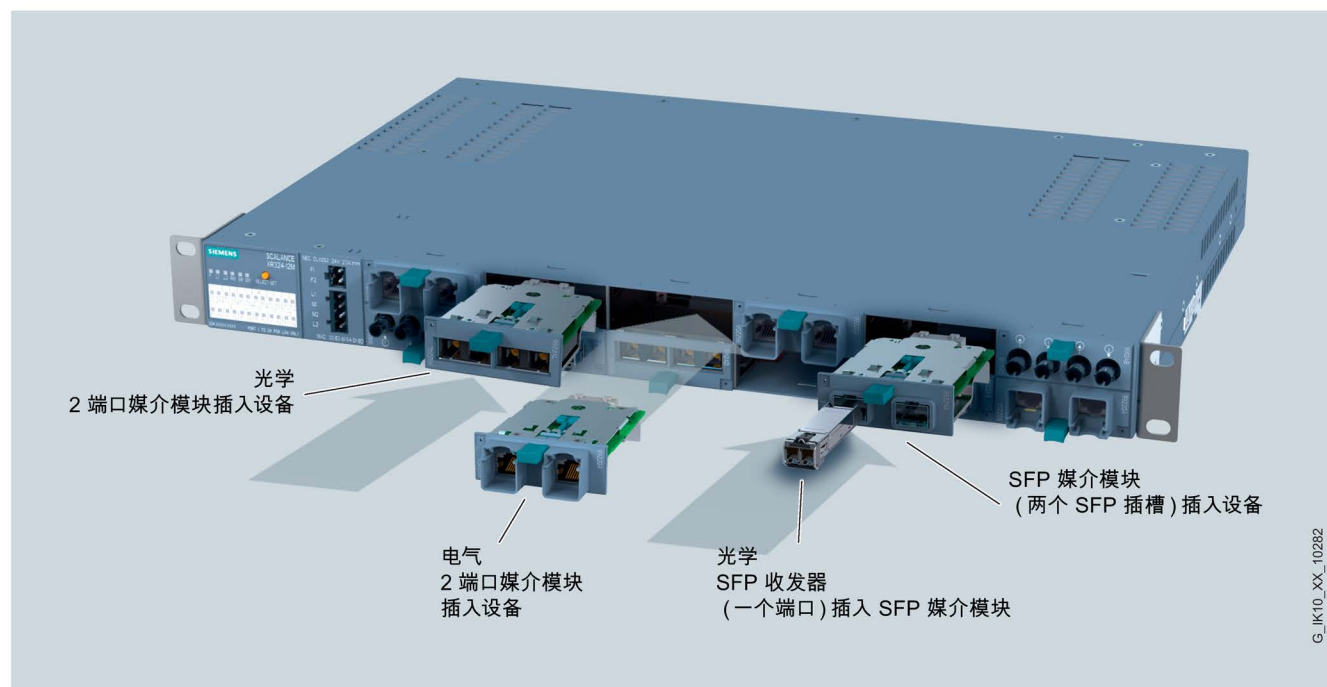
图 2-1 X-300 IE 交换机的设计，以媒介模块插入 XR324-12M 的媒介模块插槽为例
