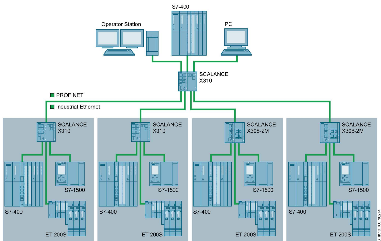
图 3-2 星型结构（电气）
