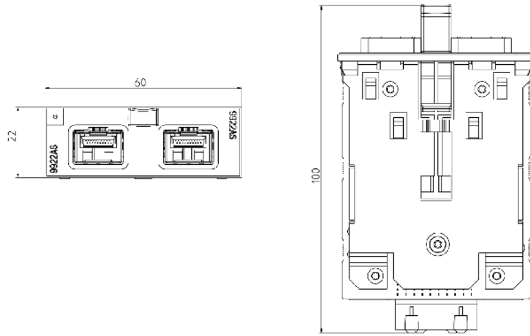
图 11-28 MM900 尺寸图 5: SFP 媒介模块
