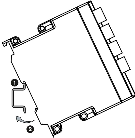
图 5-1 在 DIN 导轨 (35 mm) 上安装工业以太网交换机 X-300
