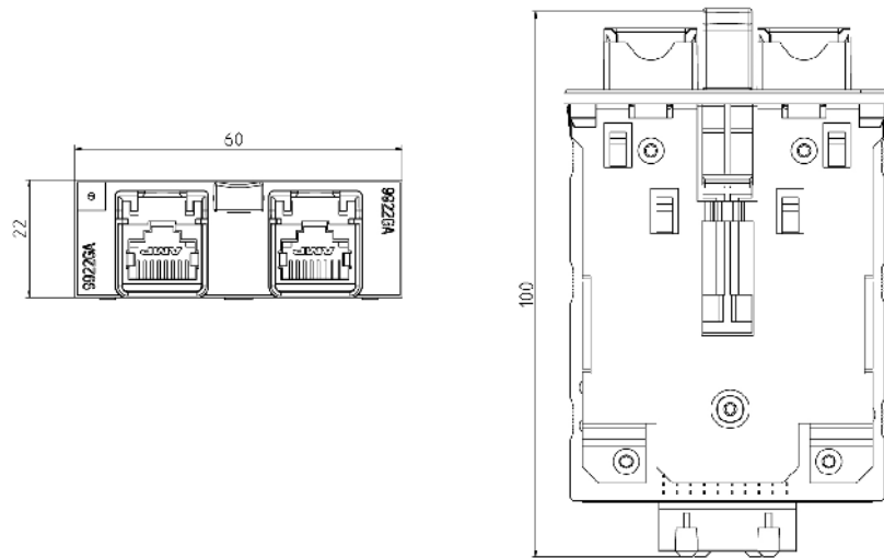
图 11-24 MM900 尺寸图 1: 带止动环的 RJ-45 电气端口
