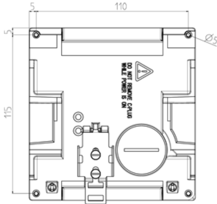
图 11-9 X308-2M 钻孔模板
