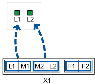
图 6-2 设备具有一个电源单元时 LED 指示灯与冗余电源引脚的分配
