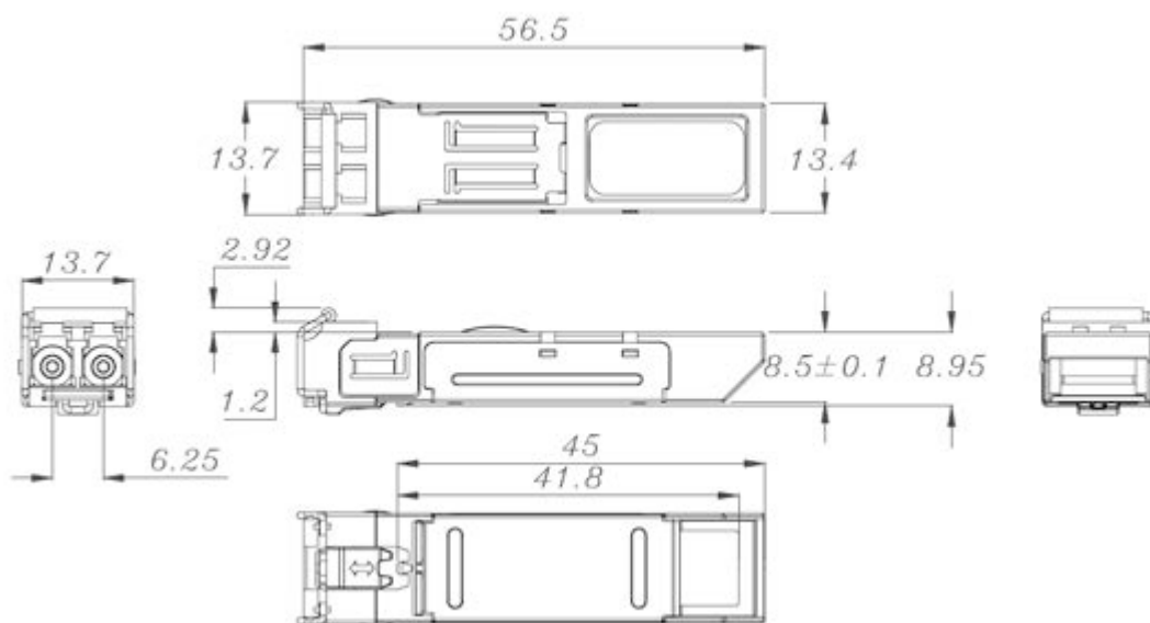
图 11-31 SFP 尺寸图
