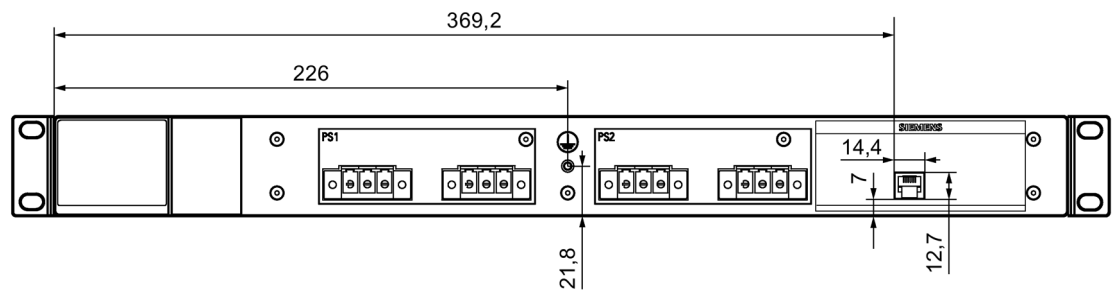
图 11-18 XR324-4M EEC 示例（2 个 100 到 240 VAC，前置电缆出口）
