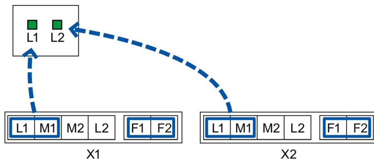
图 6-4 设备具有两个电源单元时 LED 指示灯与冗余电源引脚的分配
