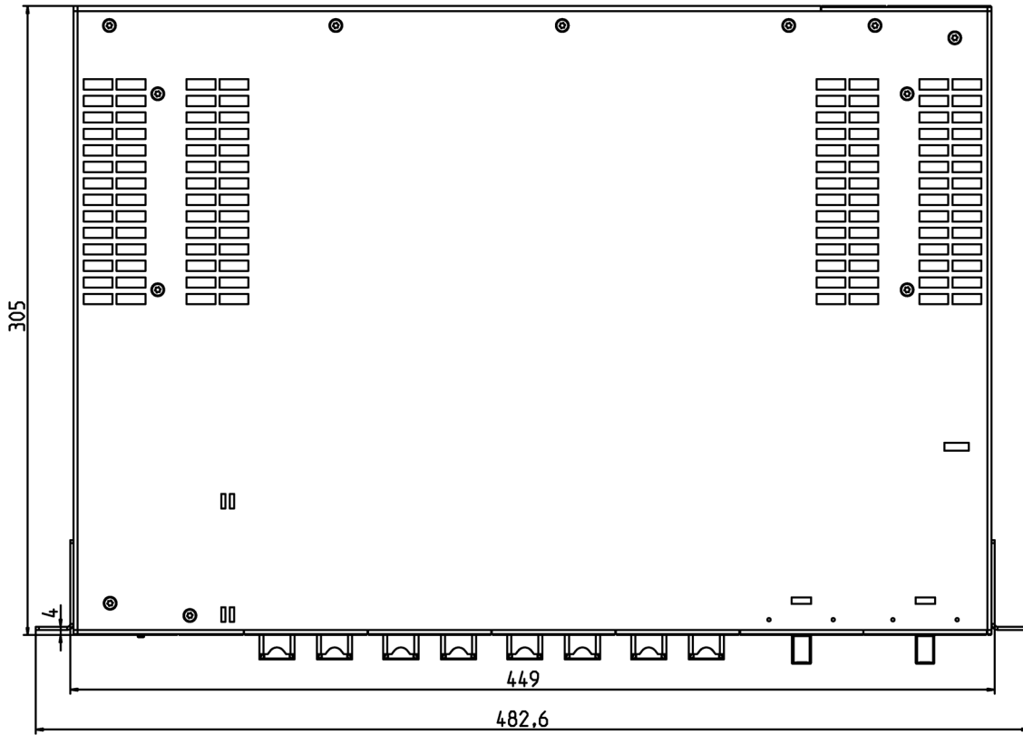
图 11-38 XR324-4M PoE 和 XR324-4M PoE TS: 俯视图
