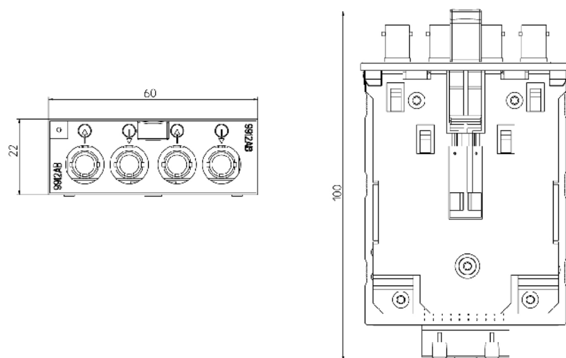
图 11-26 MM900 尺寸图 3: BFOC 端口
