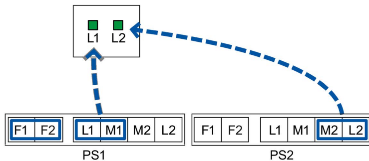
图 6-7 设备具有两个电源单元时 LED 指示灯与冗余电源针脚的分配。
