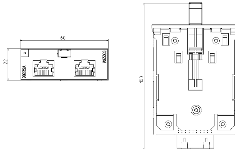
图 11-25 MM900 尺寸图 2: 不带止动环的 RJ-45 电气端口
