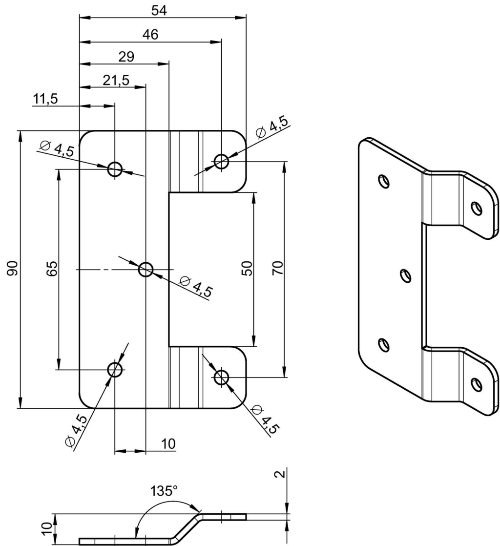
图 11-20 X-300EEC 墙式安装 (尺寸以 mm 为单位)
