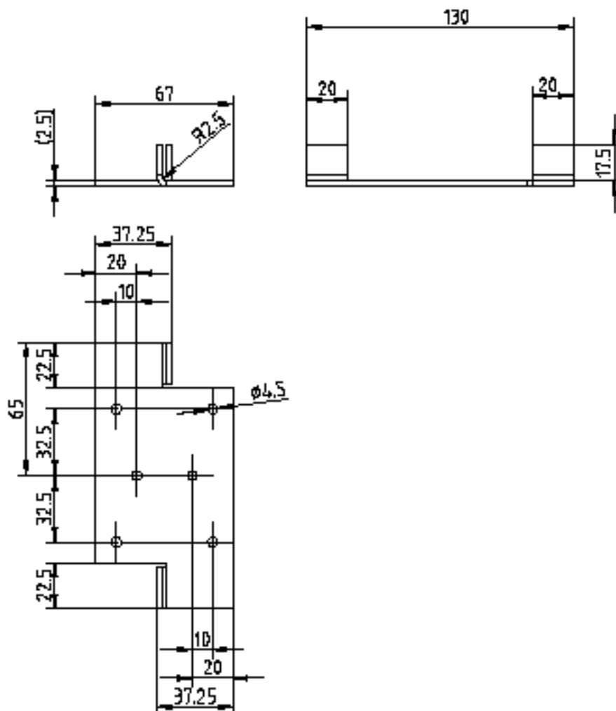
图 11-23 X-300EEC 的安装支架的中间部分（尺寸以 mm 为单位）
