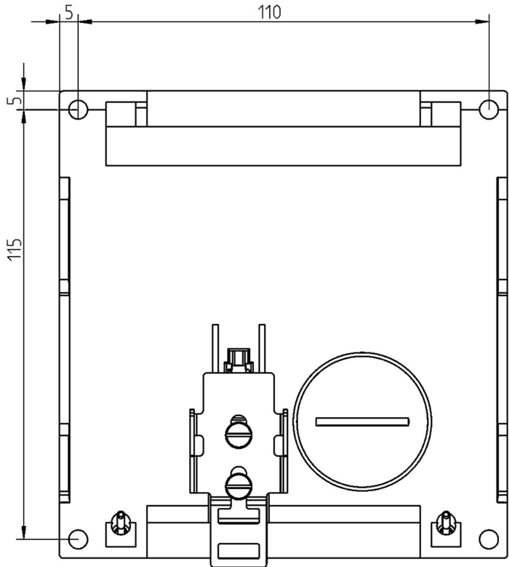
图 11-34 X308-2M PoE: 钻孔模板
