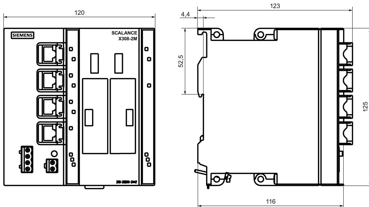
图 11-8 X308-2M 尺寸图
