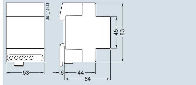
7LF5300-5 7LF5300-6 7LF5301-4 7LF5301-5 7LF5301-6 7LF5301-7
