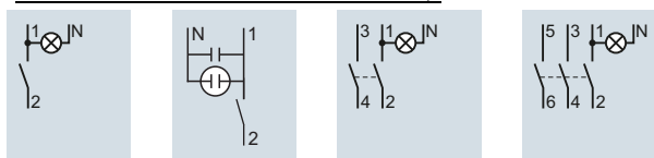
5TE8101 5TE8105 5TE8102 5TE8103 5TE8101-3
