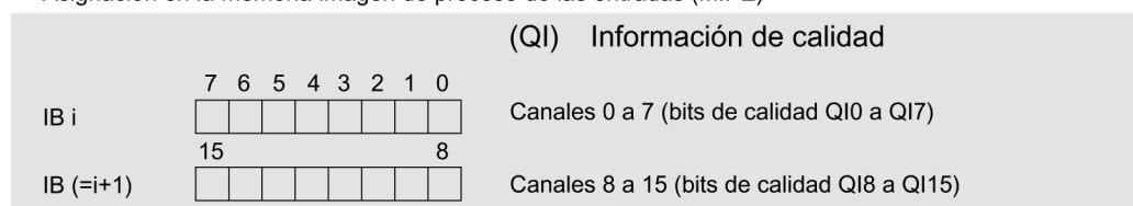
Figura 4-1 Área de direcciones en la configuración como DQ 16x24VDC/0.5A ST de 16 canales con información de calidad
