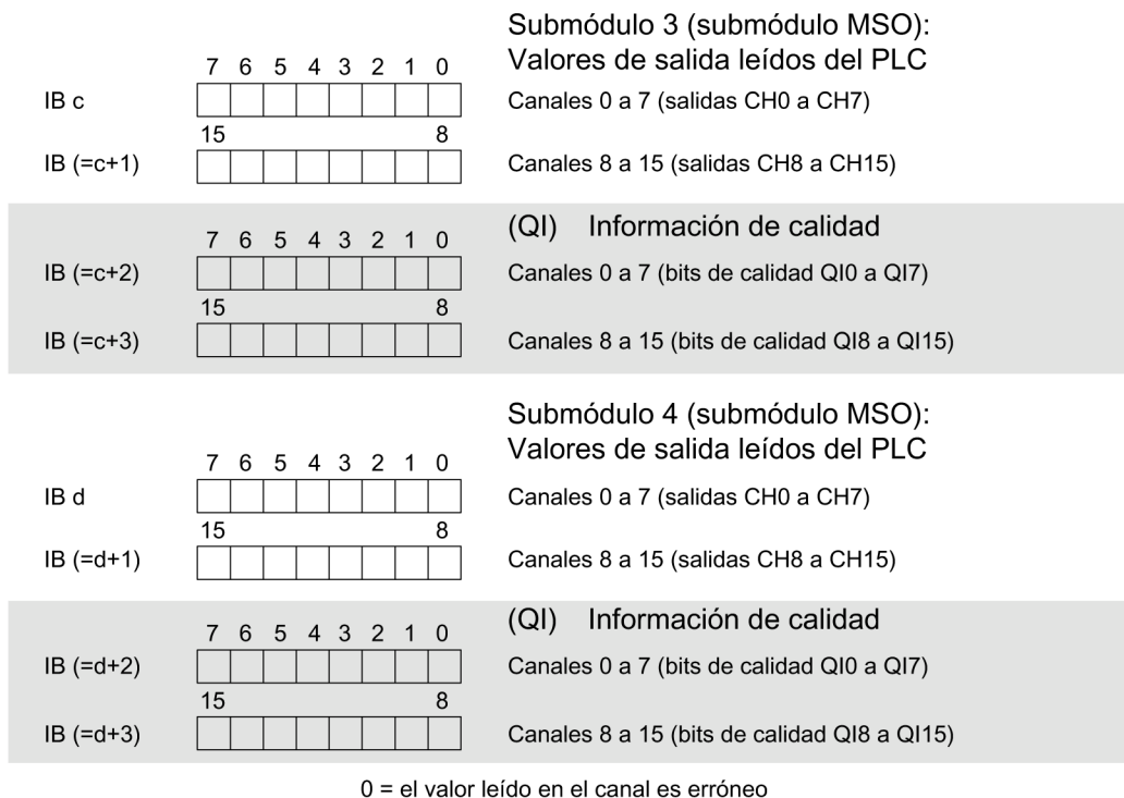
Figura 4-4 Área de direcciones en la configuración como DQ 16x24VDC/0.5A ST S MSO de 1 x 16 canales con información de calidad
