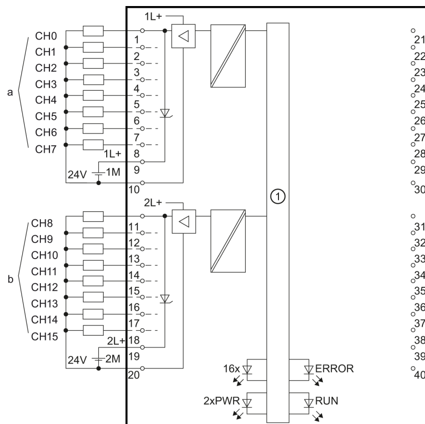
Figura 3-1 Esquema de principio y asignación de pines
