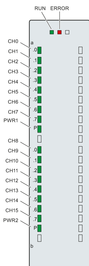
Figura 5-1 LED del módulo DQ 16x24VDC/0.5A ST
