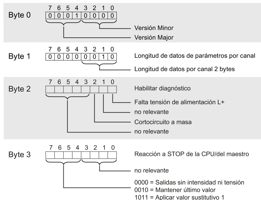
Figura B-1 Estructura del registro 64: bytes 0 a 3
