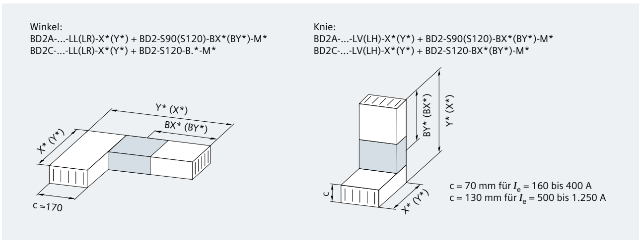
Abb. 4/22: Leiteranordnung für DC-Anwendungen des Schienenverteiler-Systems BD2 und Aufkleber zur Kennzeichnung von DC-Systemen (Maße in mm)
