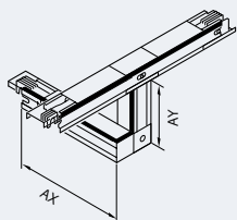
Abb. 5/5: Veranschaulichung von Richtungsänderungen mit Versatz und T-förmigen Schienenkästen (zu Tab. 5/4)
