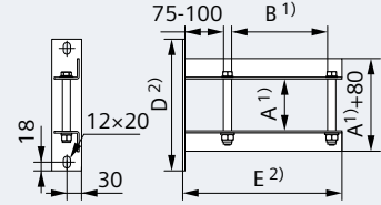
LR ... -BG
