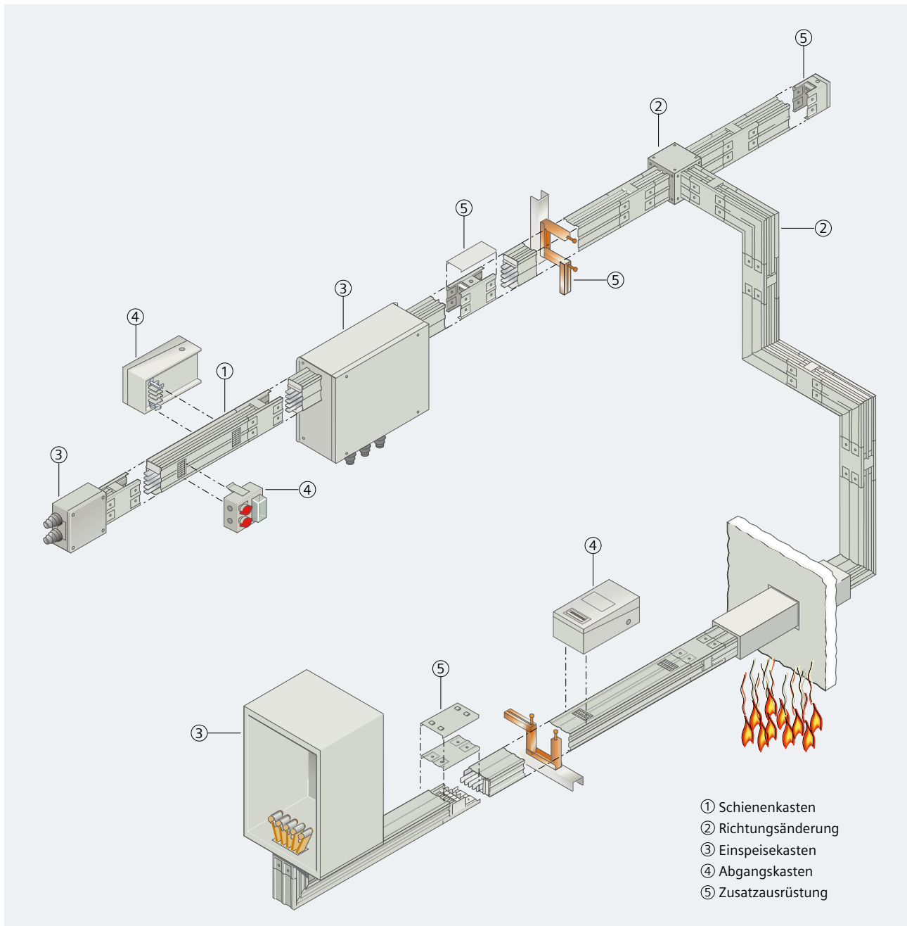
Abb. 4/1: Übersicht Schienenverteiler-System BD2
