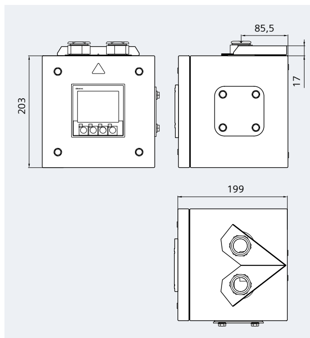
Abb. 6/21: Ansichten und Abmessungen der Messgerätebox (Maße in mm) für LI-Abgangskästen
