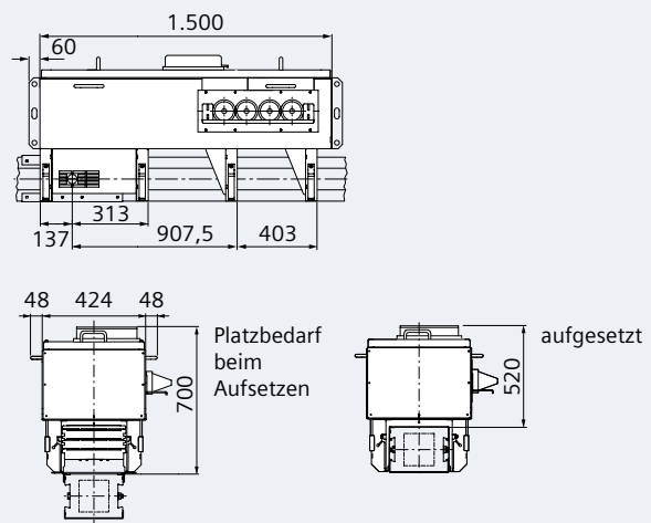
Abb. 5/15: Maße (in mm) und Ansichten für Abgangskästen mit Leistungsschalter 3VA bis 1.000 A und 3VL mit 1.250 A sowie Leerabgangskästen bis 400 A vorbereitet für den Einbau von Kompaktleistungsschaltern (Siemens, Schneider)
