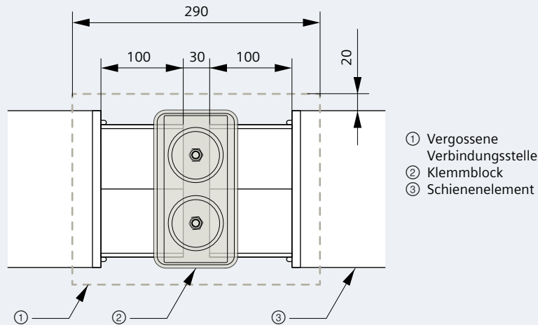
Abb. 7/9: Abmessungen für eine vergossene Verbindungsstelle (Maße in mm)
