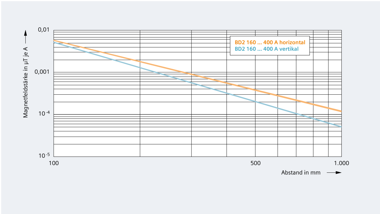
Abb. 8/7: Magnetfeldstärkenbänder für Schienenverteiler-Systeme BD2 160 ... 400 A in horizontaler und vertikaler Richtung (Abb. 2/4)
