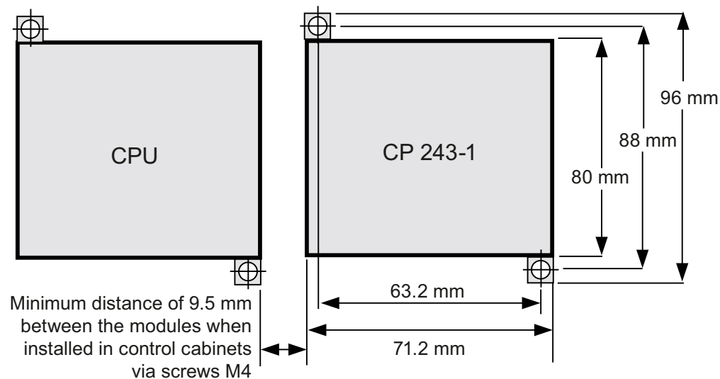
图 2-2 在控制面板中安装的尺寸
