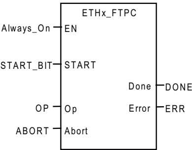
图 4-5 调用 ETHx_FTPC 子程序
