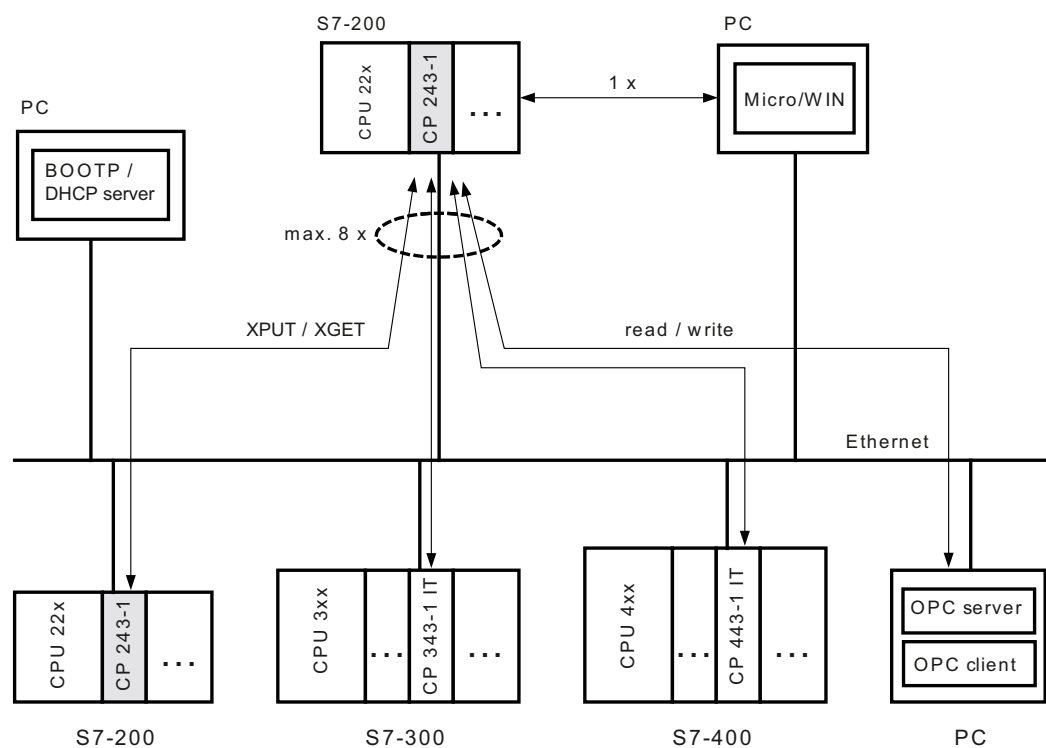
图 1-1 通信伙伴
