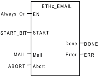
图 4-4 调用 ETHx_EMAIL 子程序
