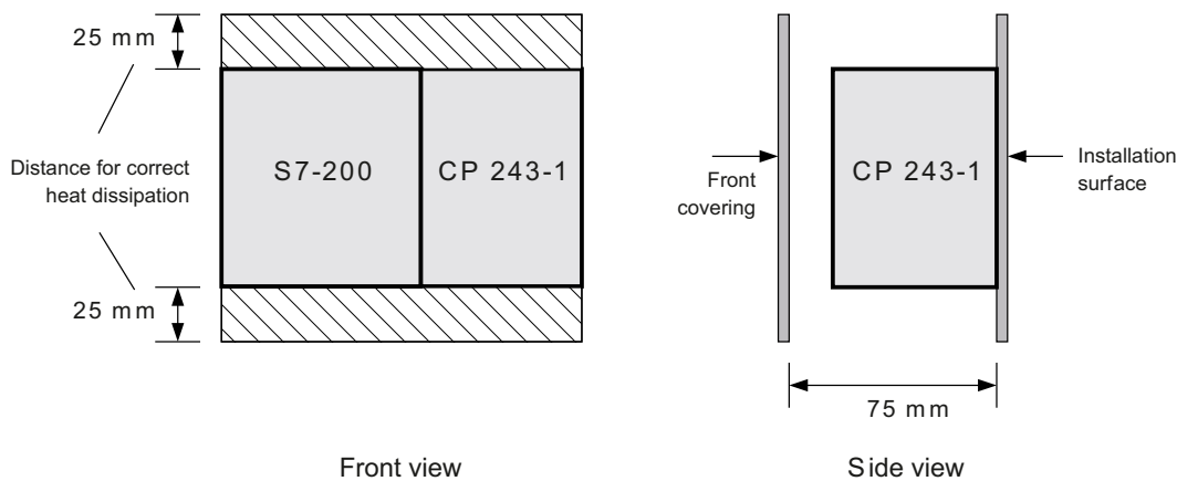
图 2-1 安装空间要求
