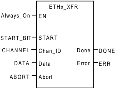
图 4-3 调用 ETHx_XFR 子程序
