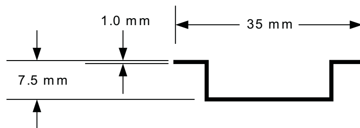
图 2-3 在 DIN 导轨上安装的尺寸
