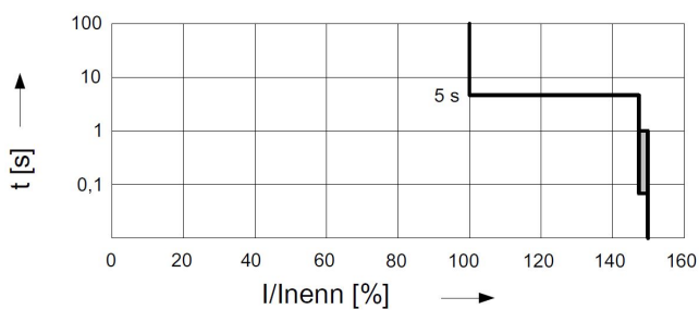
Abbildung 3: Abschaltcharakteristik (typisch) Figure 3: Disconnection characteristic (typical)
