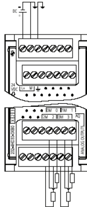
6ES7 232-4HD30-0XB0
