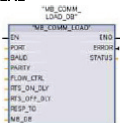
LAD
