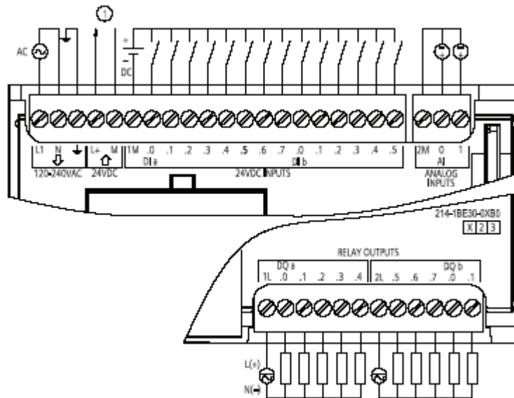
Рис. А-7. CPU 1214C AC/DC/Relay (6ES7 214-1BE30-0XB0)
