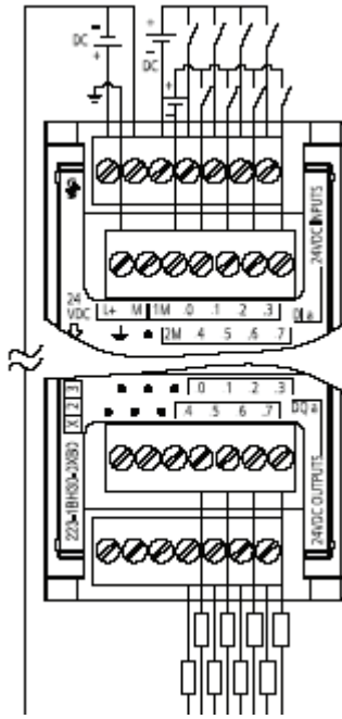
6ES7 223-1BH30-0XB0
