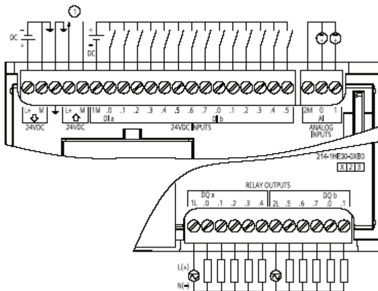
① Питание датчиков 24 В пост. тока Рис. А-8. CPU 1214C DC/DC/Relay (6ES7 214-1HE30-0XB0)
