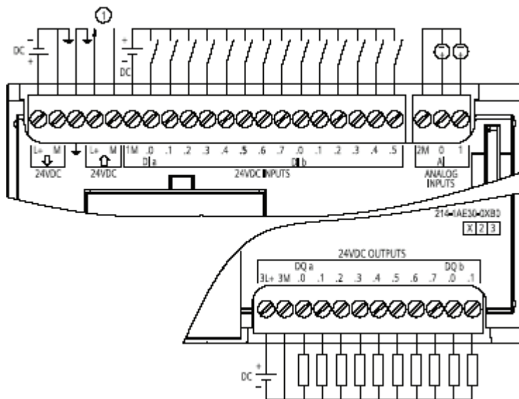
① Питание датчиков 24 В пост. тока Рис. А-9. CPU 1214C DC/DC/DC (6ES7 214-1AE30-0XB0)
