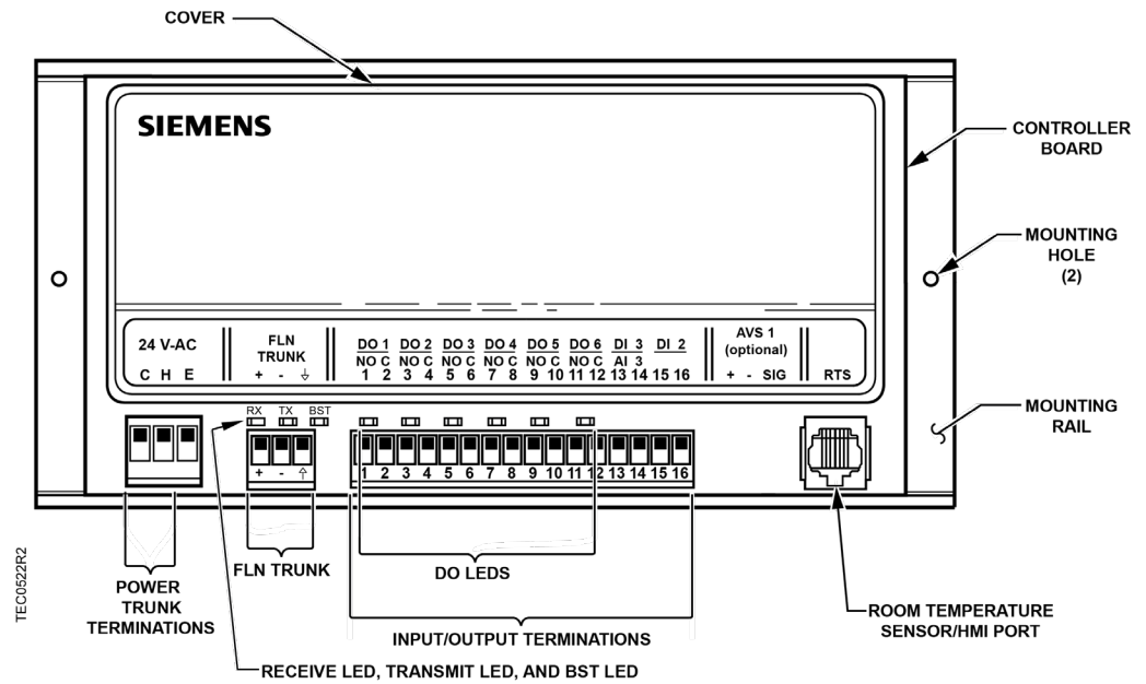
Fig. 176: 6 DO Controller.
