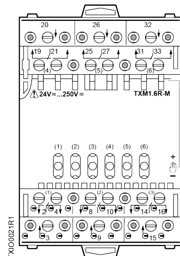
TXM1.6R-M
