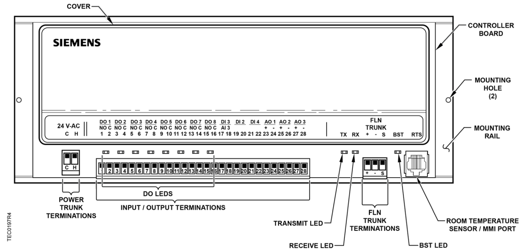
Fig. 173: 8 DO Controller.
