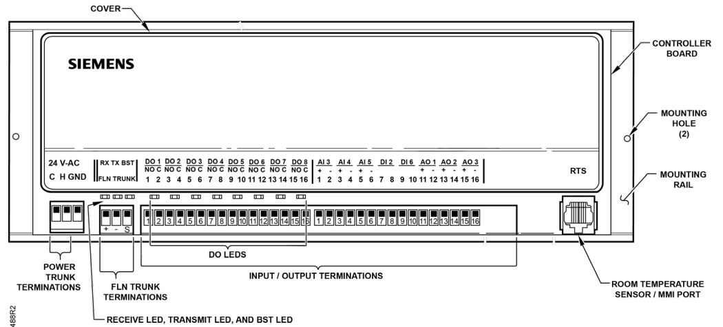
Fig. 178: 8 DO Controller.
