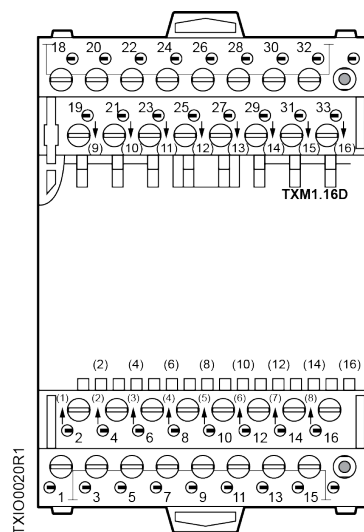
TXM1.16D
