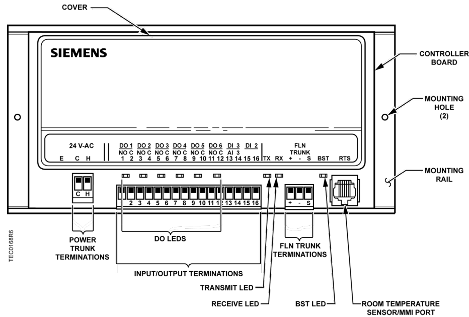
Fig. 171: 6 DO Controller.
