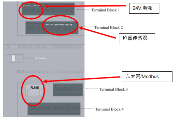
图 2-1 称重模块 WP231 接线
