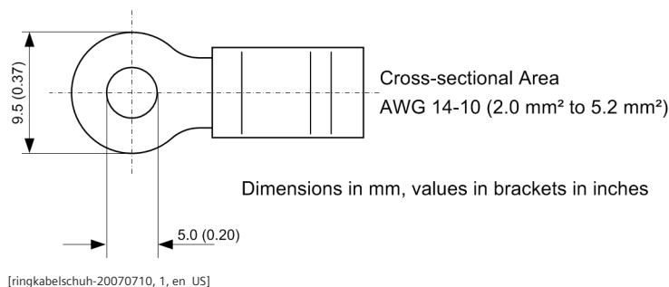
Figure 3-5 Ring lug
