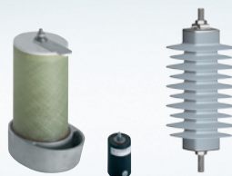
3EF surge limiter 3EJ, 3EK, 3EP-G, 3EQ0 surge arresters
