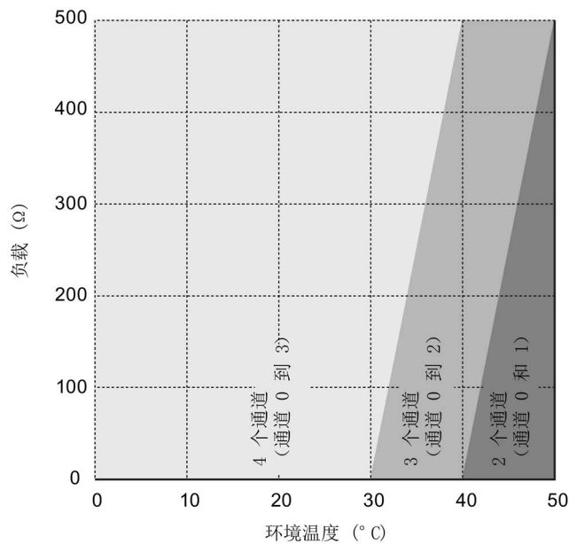
图 6-2 电流输出降低趋势（垂直安装）
