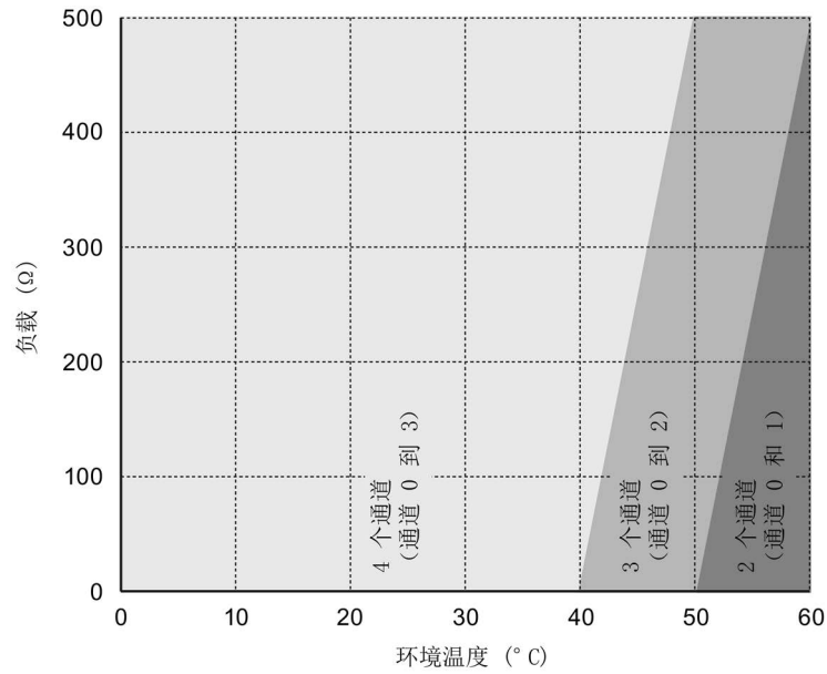
图 6-1 电流输出降低趋势（水平安装）
