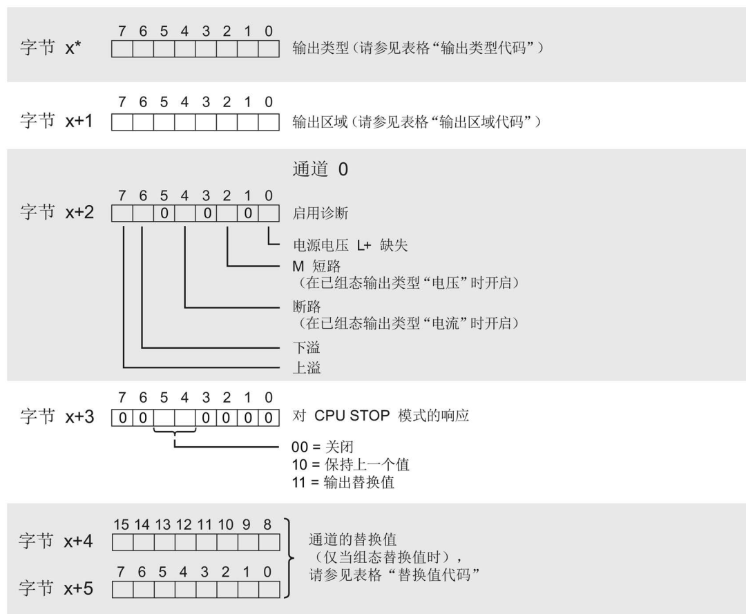
图 A-3 通道 0 到 3 中字节 x 到 x+5 的结构
