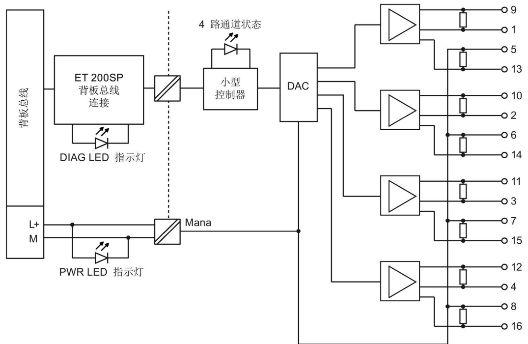
图 3-1 AQ 4xU/I ST 的电路示意图
