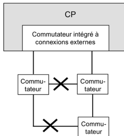
Figure 5-2 Connexion de commutateurs
