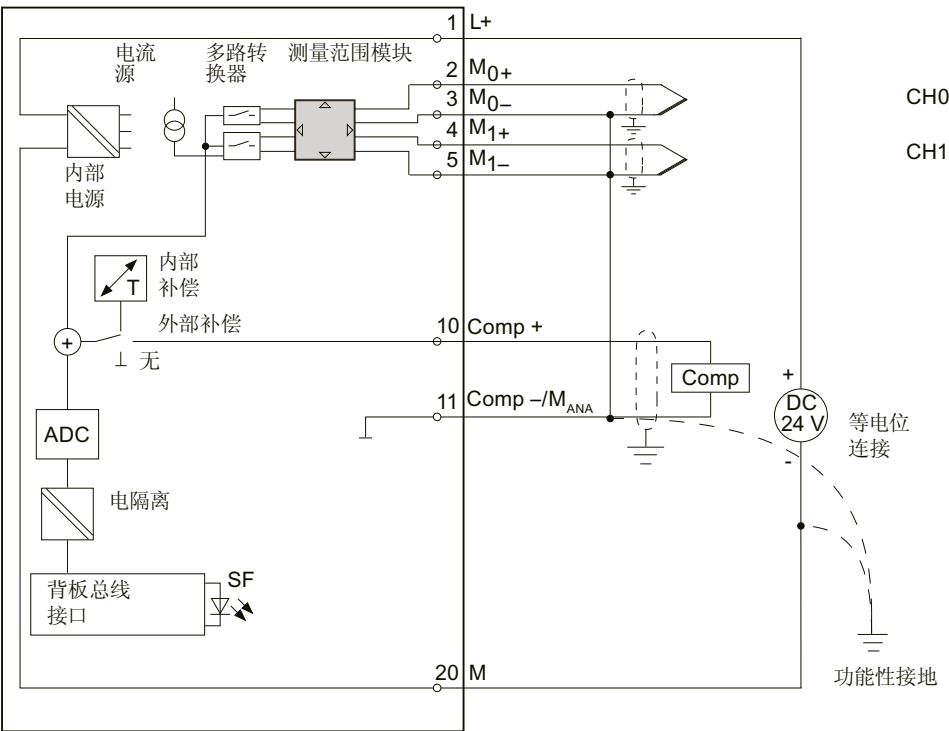
图 6-18 接线图与方框图
