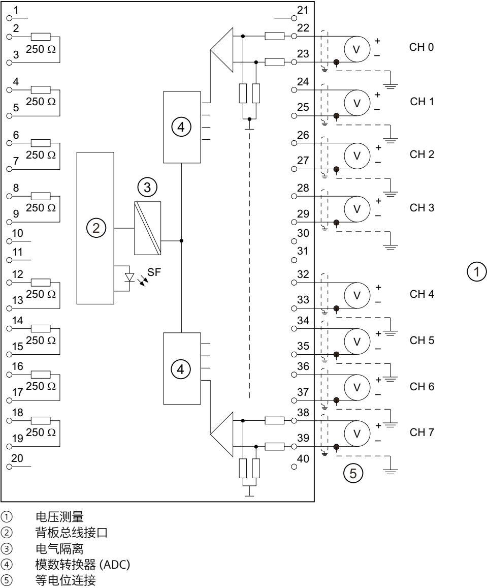
图 6-1 接线图与方框图
