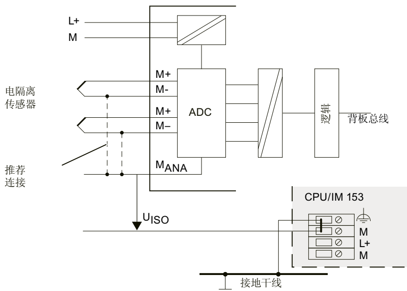
图 4-1 将电气隔离传感器接线, 并连接到电气隔离 AI
