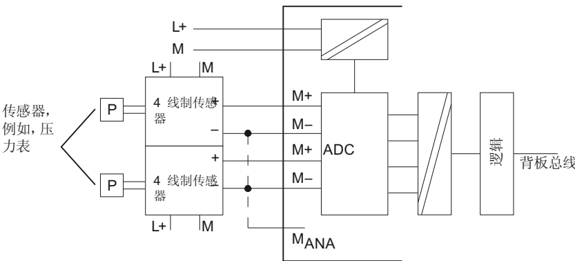
图 4-8 对 4 线传感器接线，并连接到电气隔离 AI
