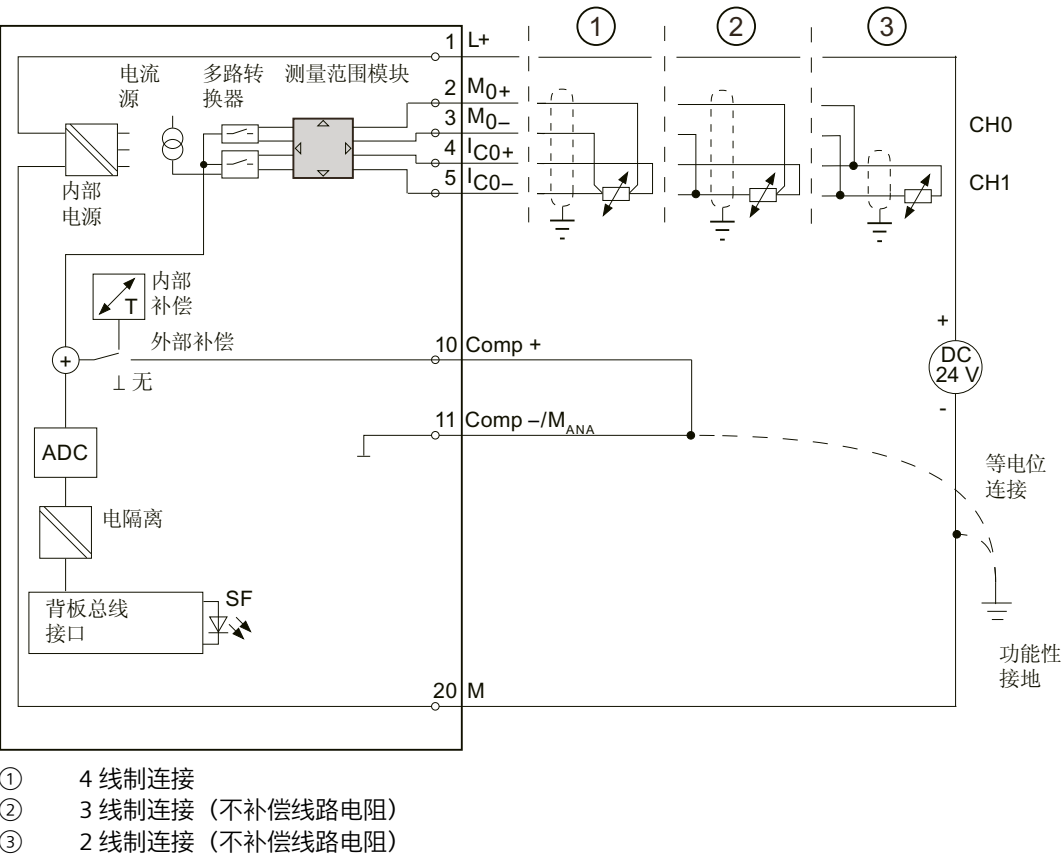
图 6-19 接线图与方框图
