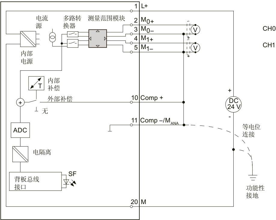
图 6-17 接线图与方框图
