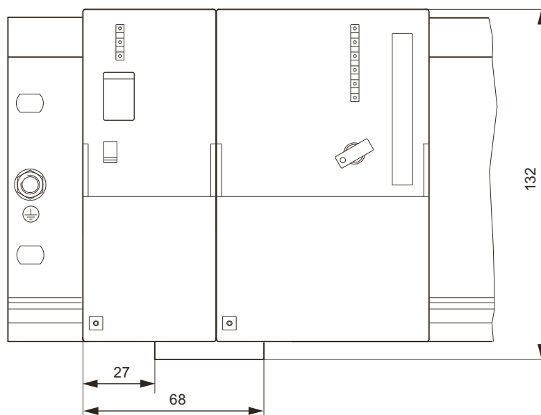
图 C-12 带有 CPU 313/314/315/315-2 DP 和电源模块 PS 307 ; 10 A 的尺寸图（正视图）
