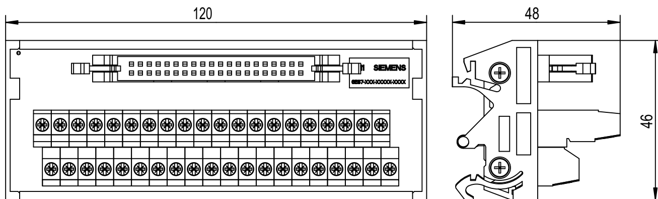
图 C-21 40 针端子块
