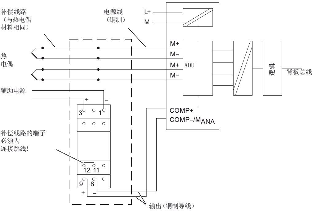
图 4-16 热电偶与基准结的连接
