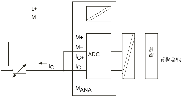
图 4-10 电阻温度计与电气隔离模拟量输入的 3 线制连接
