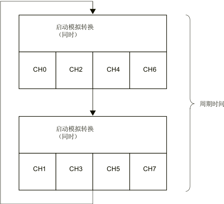
图 6-5 8 通道模式周期时间
