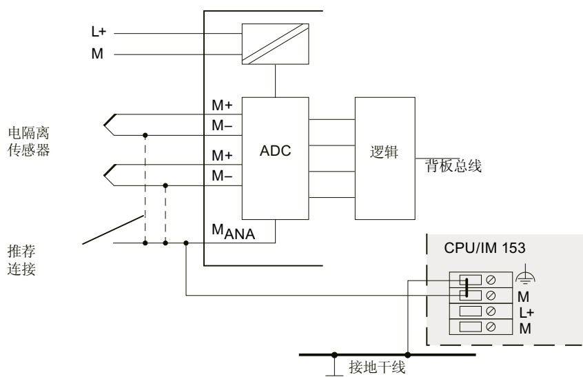
图 4-2 对电气隔离传感器接线并连接到非隔离 AI
