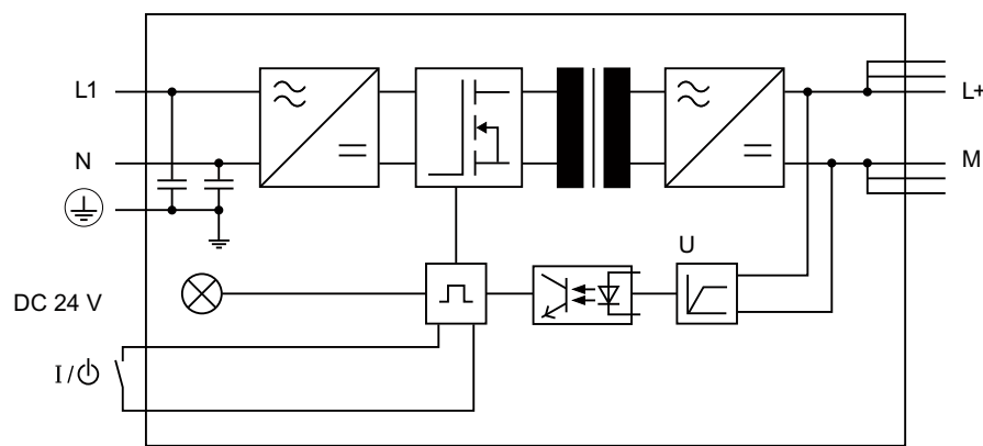
图 2-5 电源模块 PS 307; 5 A 的电路示意图
