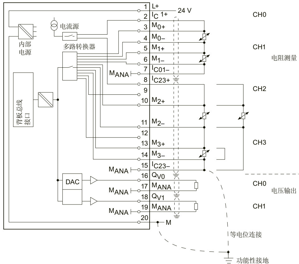
图 6-53 接线图与方框图
