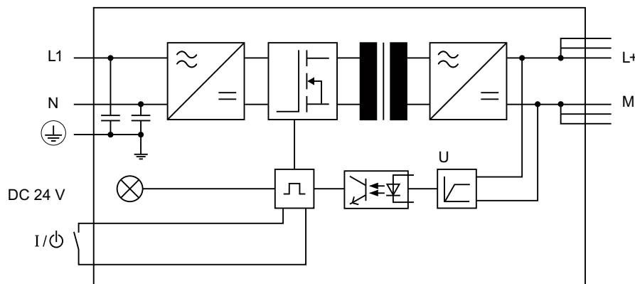
图 2-2 PS 307; 5 A 电源模块的方框图
