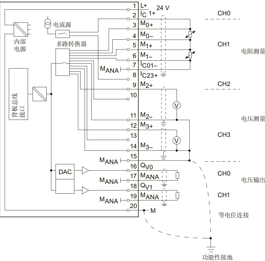
图 6-52 接线图与方框图
