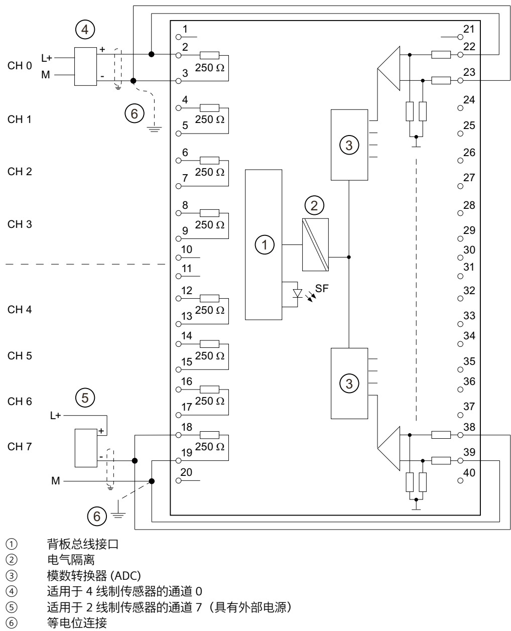
图 6-2 接线图与方框图
