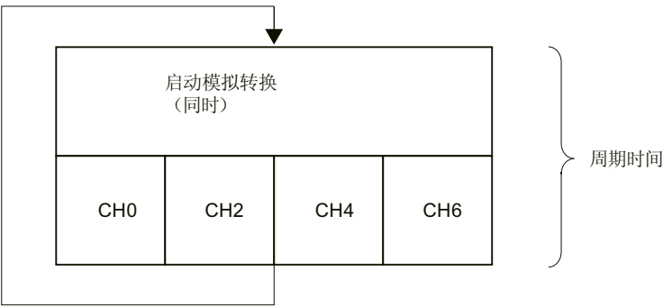
图 6-31 4 通道模式周期时间（硬件过滤器）
