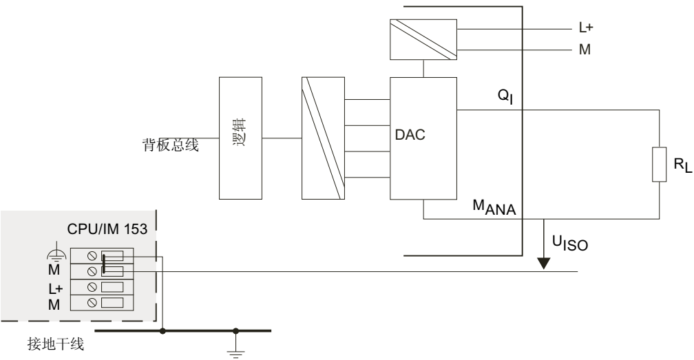
图 4-19 对负载进行接线，并连接到电气隔离模拟量输出模块的电流输出
