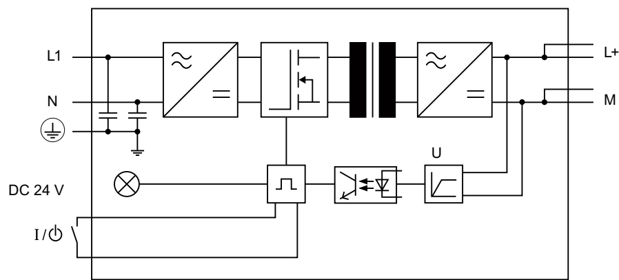
图 2-1 电源模块 PS 307; 2 A 的电路示意图
