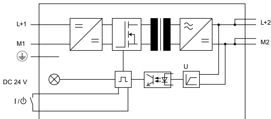
图 2-4 电源模块 PS 305; 2 A 的电路示意图
