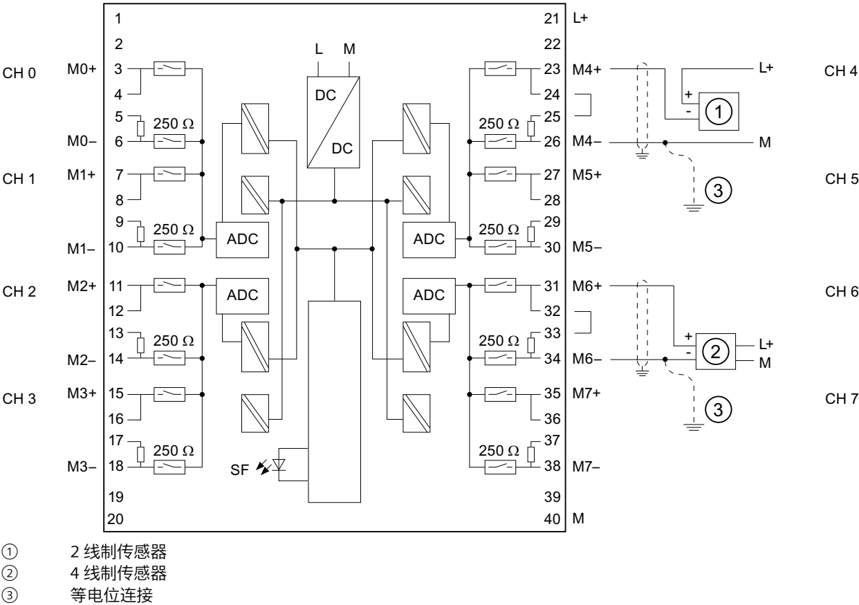
图 6-4 接线图与方框图
