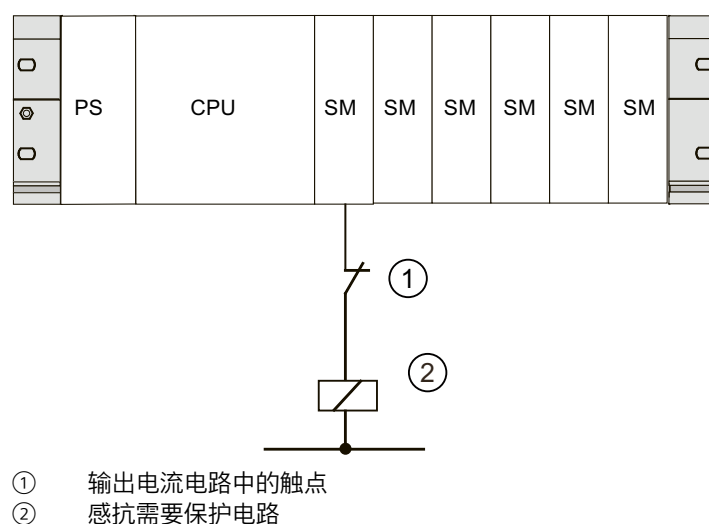
图 3-1 输出电流电路中用于急停的继电器触点
