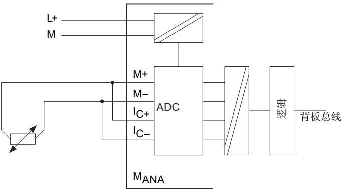
图 4-11 电阻温度计与电气隔离模拟量输入的 2 线制连接
