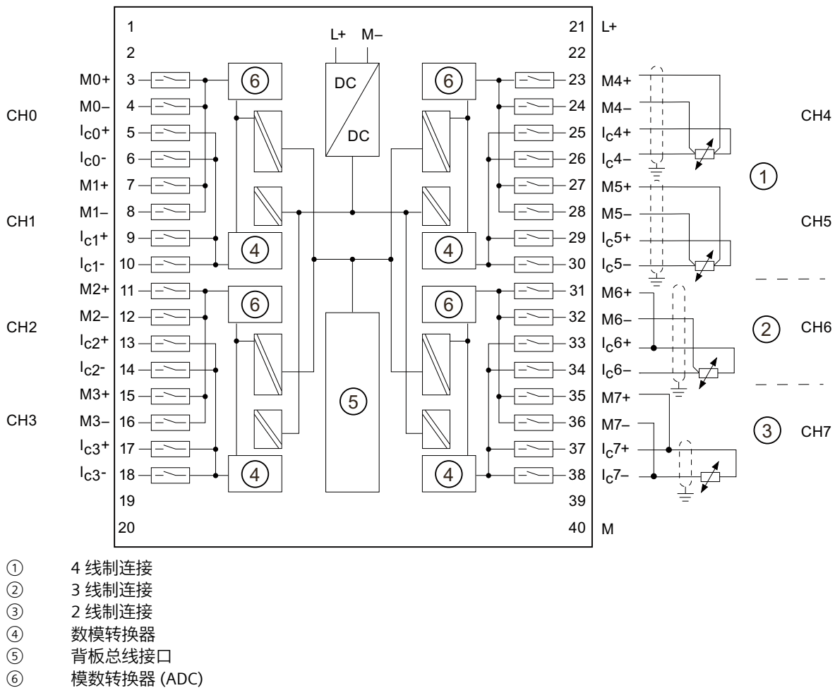
图 6-21 接线图与方框图
