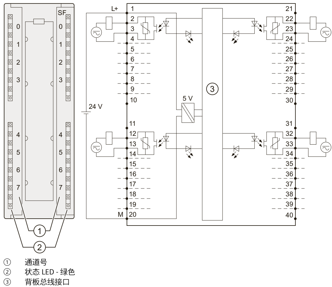
SM 322; DO 16 x UC 24/48 V 模块的接线图与方框图
