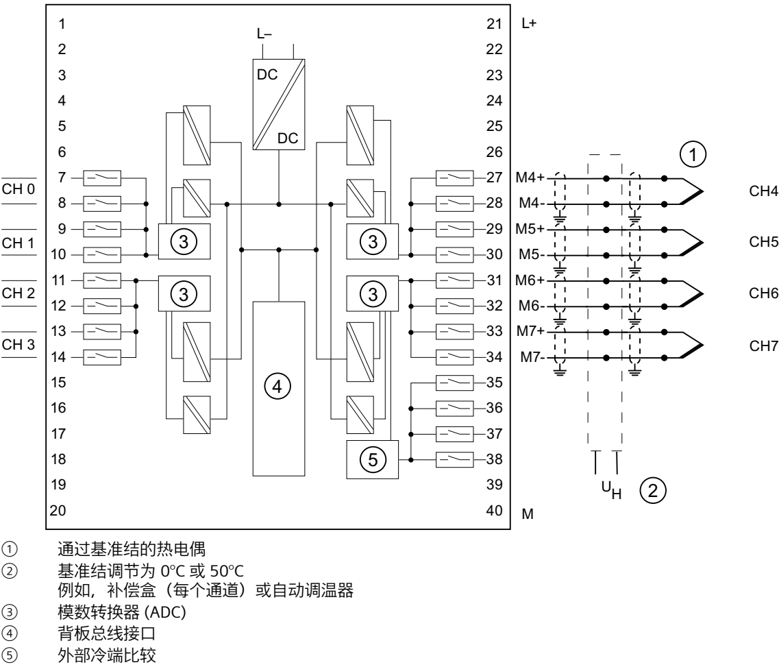
图 6-26 接线图与方框图
