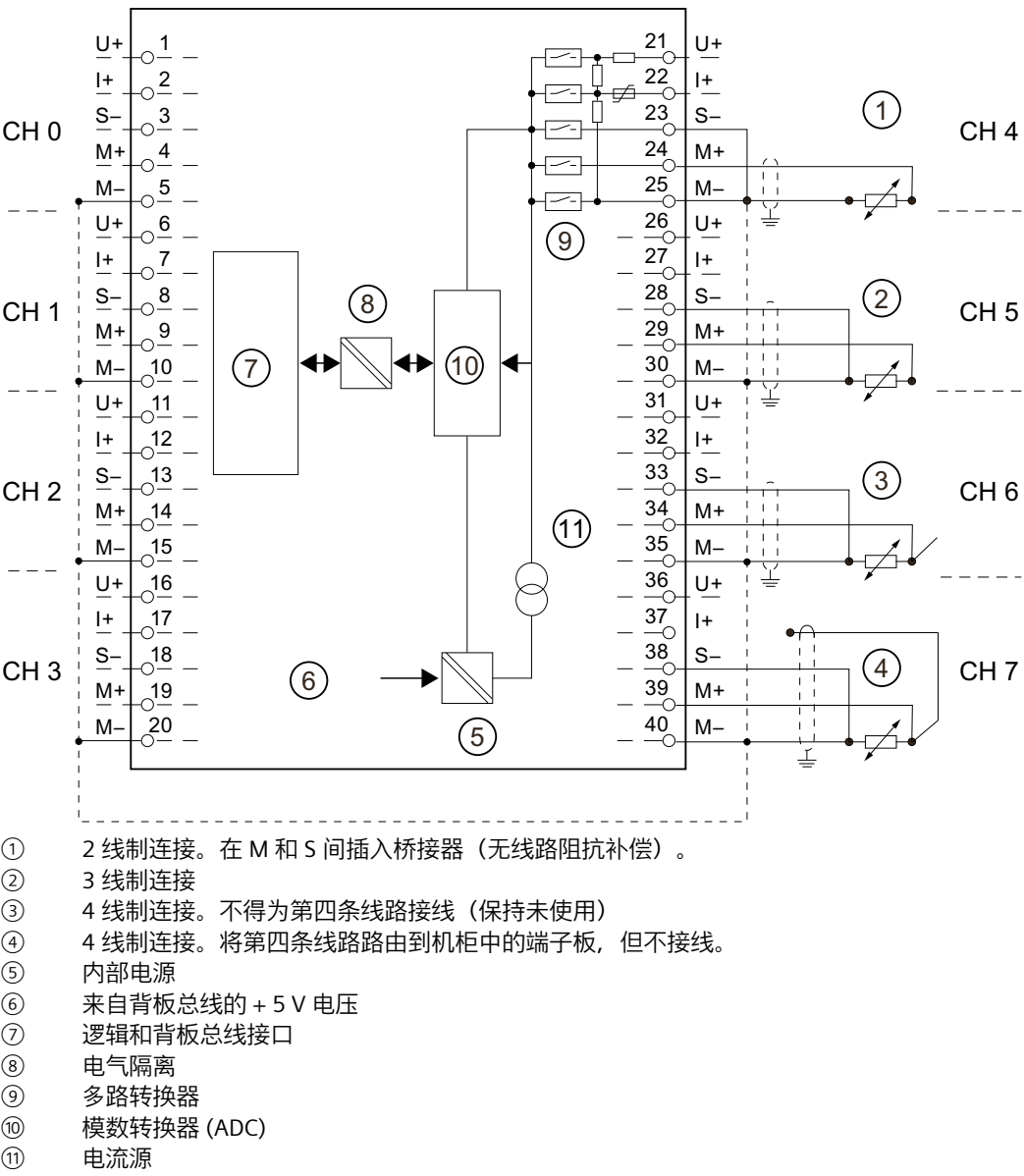
图 6-12 方框图和端子图
