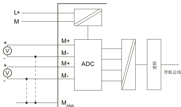
图 4-5 对电压传感器接线, 并连接到电气隔离 AI
