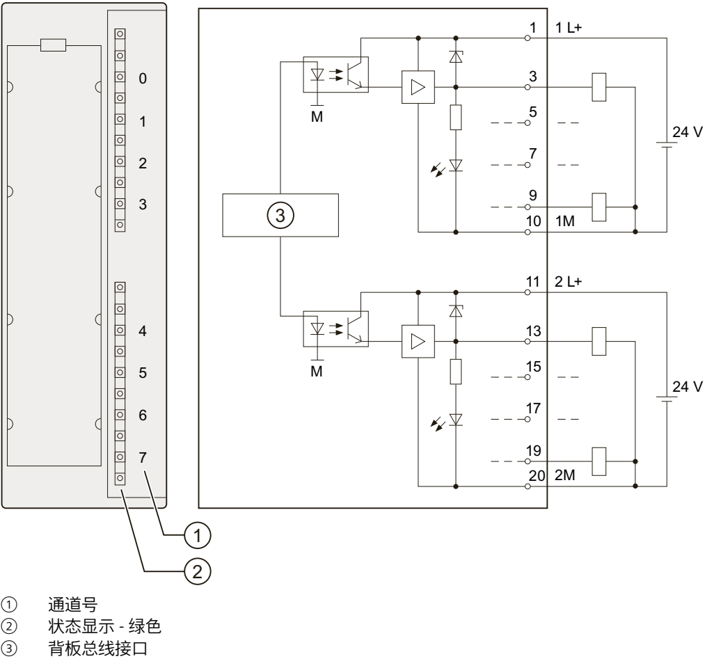
SM 322 ; DO 8 x DC 24 V/2 A 的接线图和方框图
