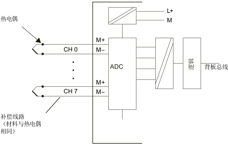
图 4-14 对带内部补偿的热电偶进行接线，并连接到电气隔离模拟量输入
