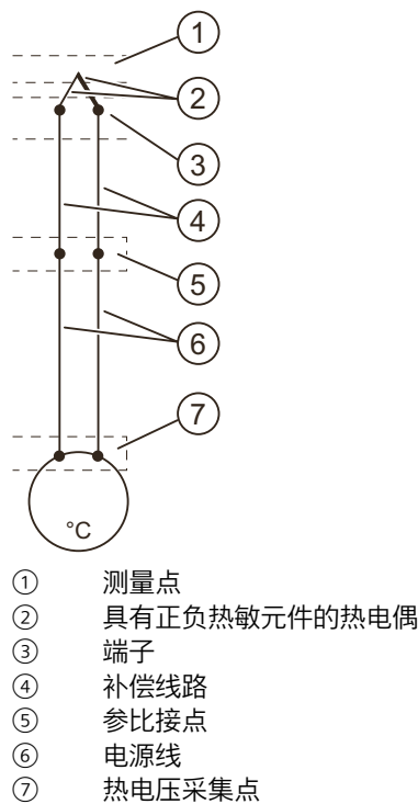
图 4-13 图 4-22 热电偶的结构
