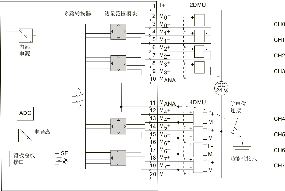
图 6-8 方框图和接线图
