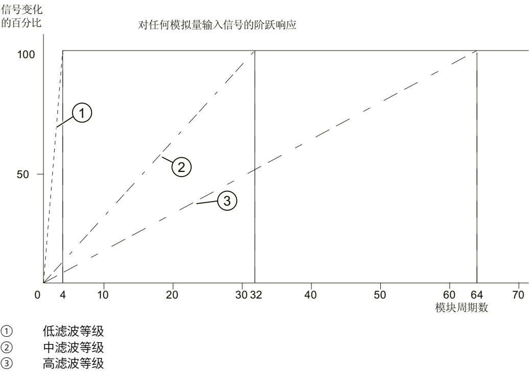
图 5-5 滤波对跳转响应的影响实例 (AI 8 x 14 位)
