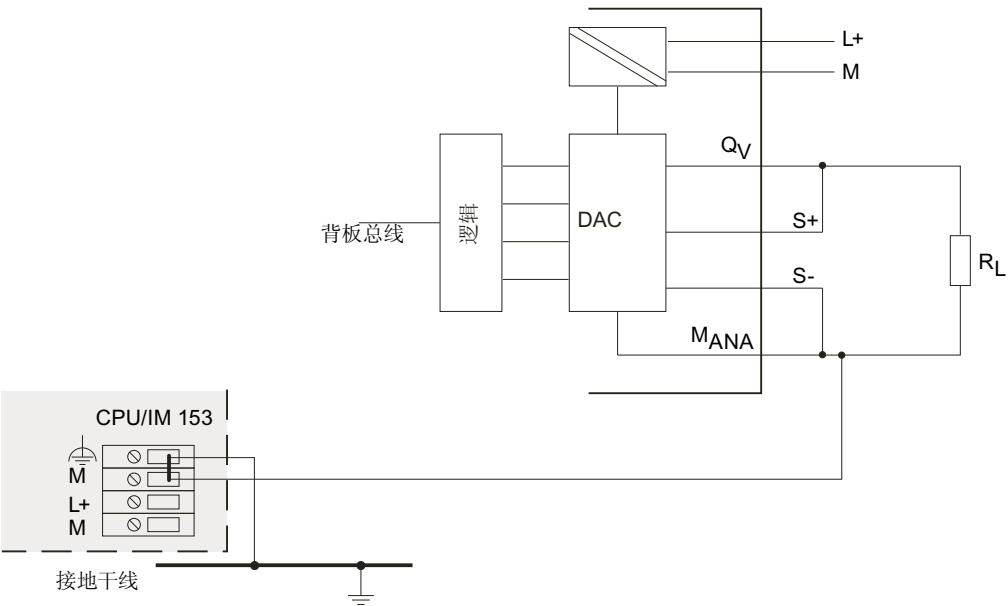
图 4-18 负载到非隔离模拟量模块电压输出的 2 线制连接
