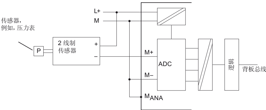
图 4-7 对从 L+ 供电的 2 线制传感器进行接线，并连接到电气隔离 AI
