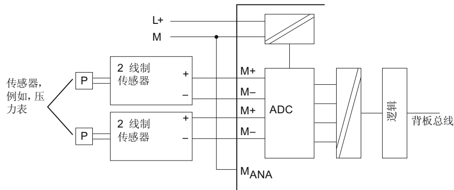
图 4-6 对 2 线传感器接线, 并连接到电气隔离 AI
