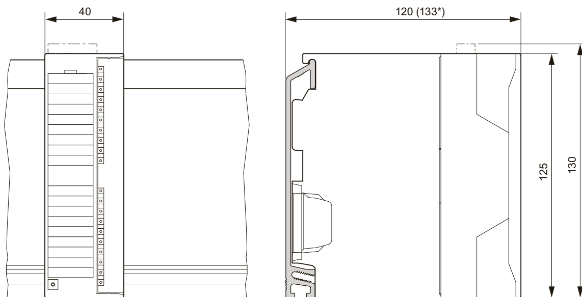
图 C-18 信号模块
