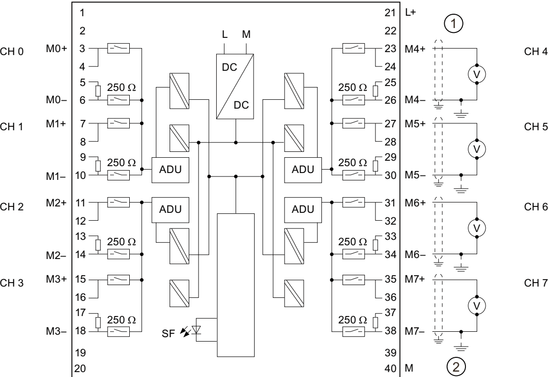
图 6-3 接线图与方框图
