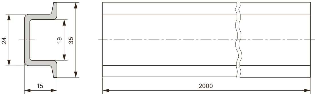
图 C-4 2000 mm 标准导轨的尺寸图
