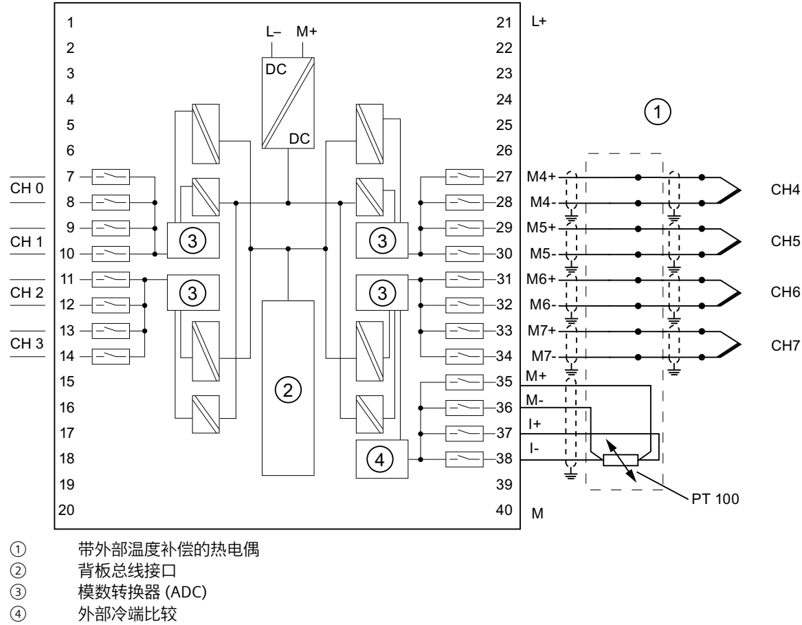
图 6-27 接线图与方框图
