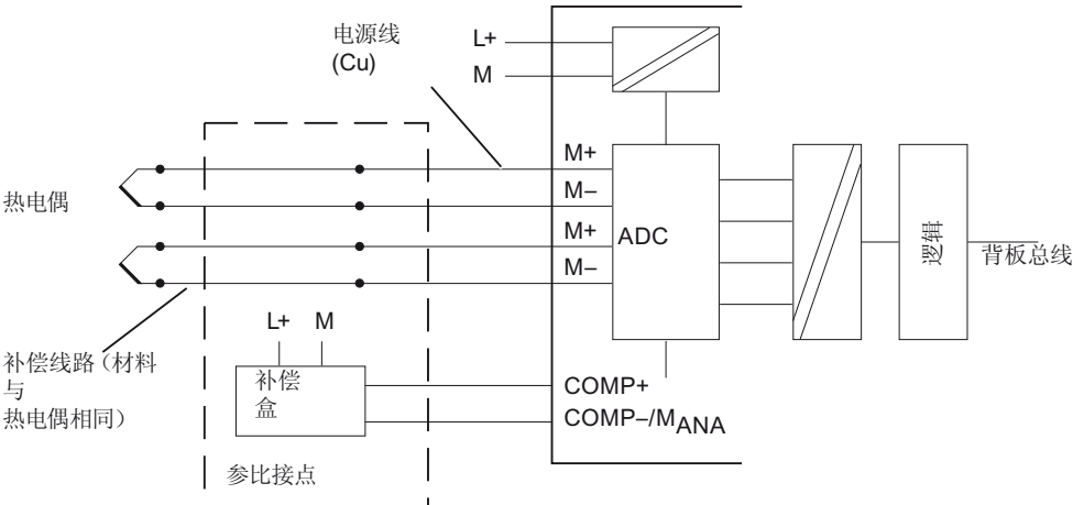
图 4-15 通过补偿盒对热电偶进行接线并连接到电气隔离模拟量输入
