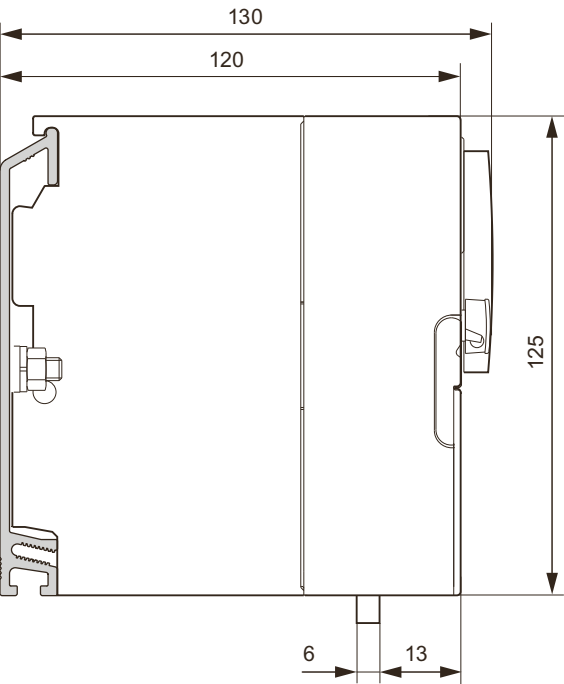
图 C-13 带 CPU 313/314/315/315-2 DP 的电源模块 PS 307 ; 10 A 的尺寸图（侧视图）
