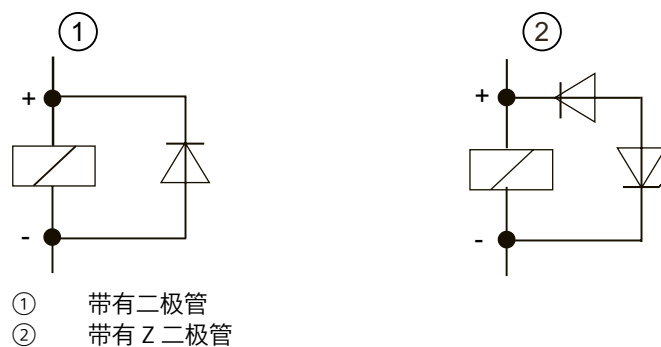
图 3-2 直流线圈的组态
