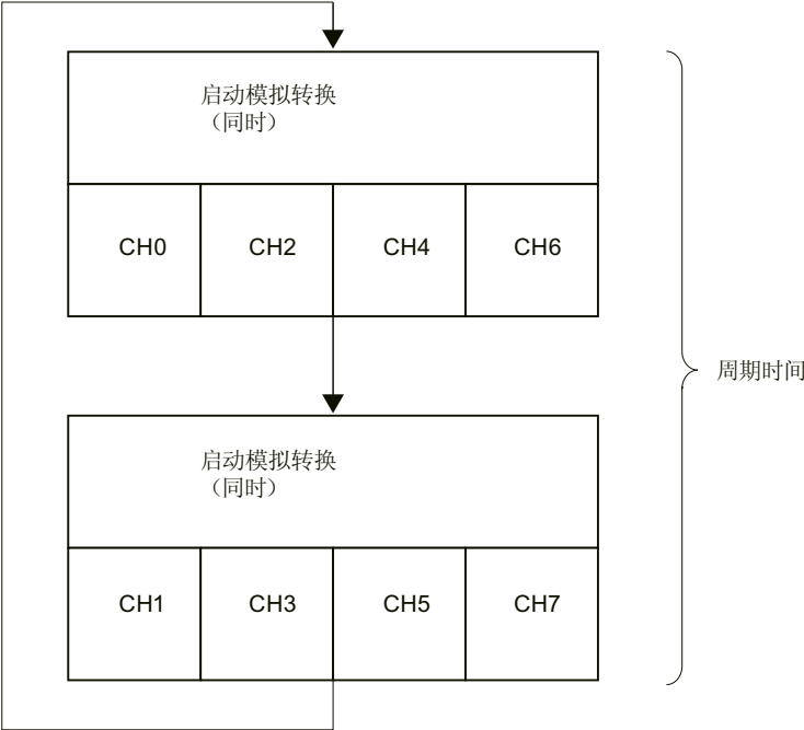
图 6-24 8 通道模式周期时间（软件过滤器）
