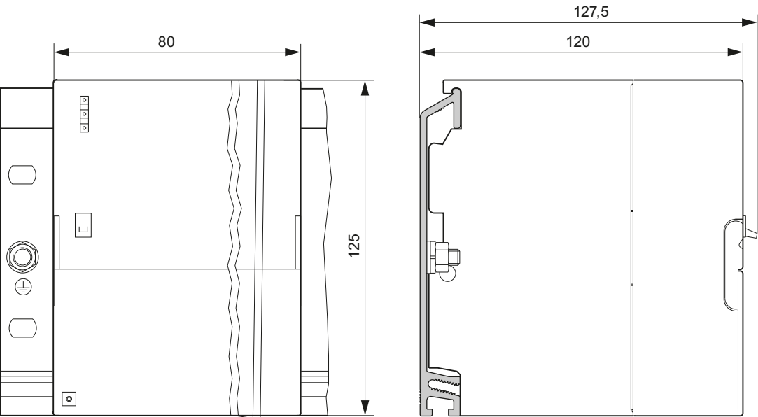
图 C-14 电源模块PS 307 ; 10 A
