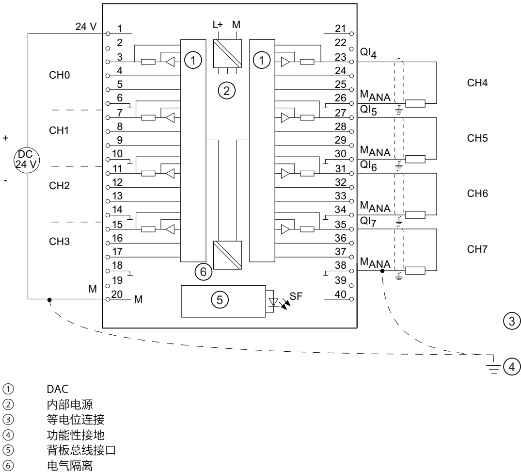
图 6-42 接线图与方框图
