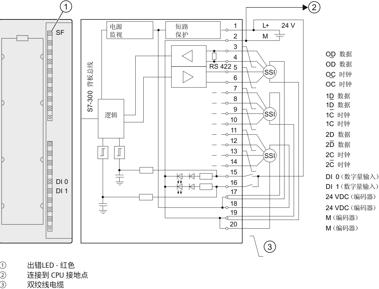
接线图和方框图
