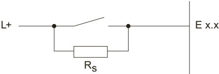
图 3-7 SM 321 ; DI 16 x DC 24 V/125 V 模块变送器并联电路的接线图
