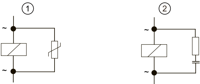
图 3-3 交流线圈的连接
