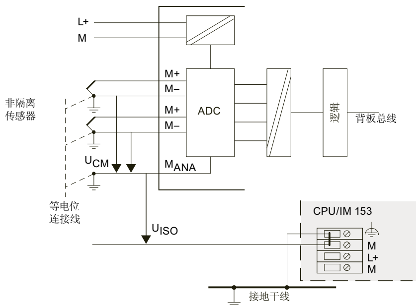
图 4-3 将非隔离传感器连接到电气隔离 AI
