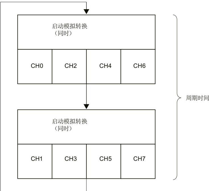
图 6-23 8 通道模式周期时间（硬件过滤器）
