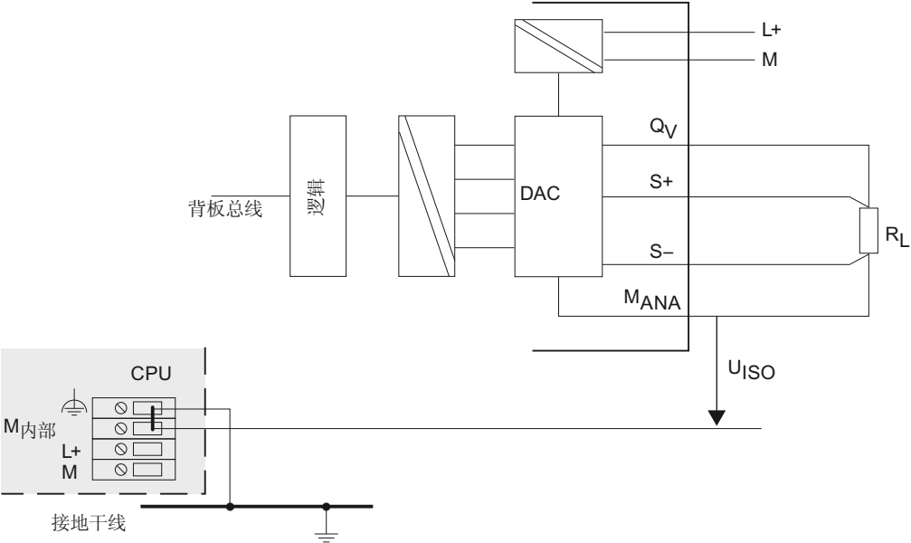
图 4-17 负载到电气隔离模拟量输出模块电压输出的 4 线制连接
