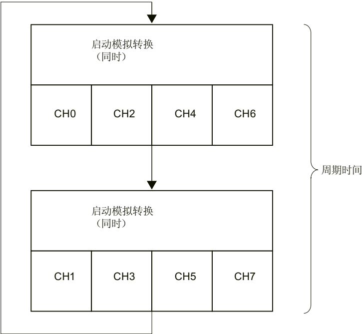
图 6-29 8 通道模式周期时间（硬件过滤器）
