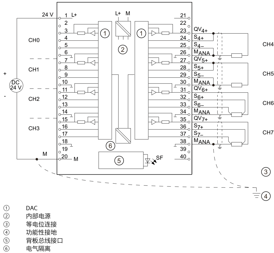
图 6-41 接线图与方框图
