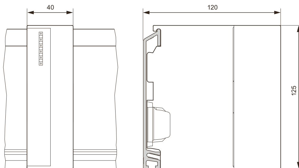
图 C-15 接口模块 IM 360
