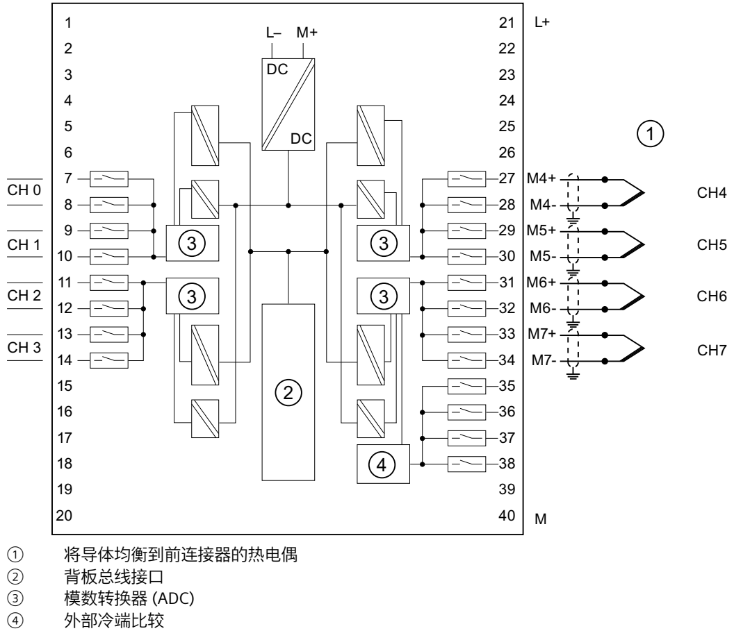
图 6-28 接线图与方框图
