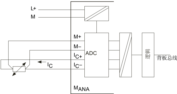
图 4-9 电阻温度计与电气隔离模拟量输入的 4 线制连接
