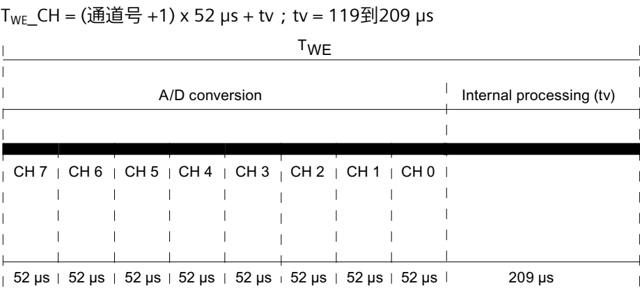
图 6-9 过滤和处理时间计算
