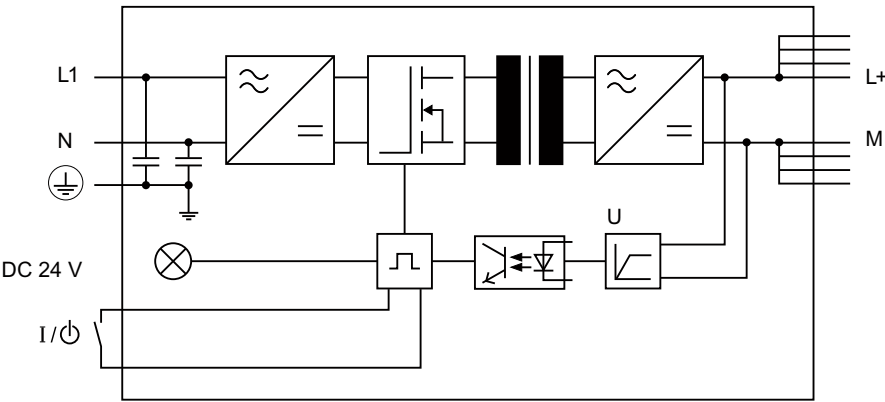
图 2-3 PS 307; 10 A 电源模块的方框图
