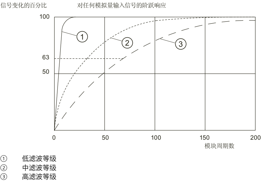
图 5-6 使用 AI 6 x TC 时滤波对阶跃响应的影响示例
