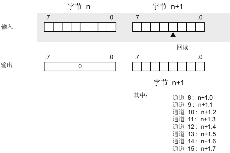
图 3-11 SM 327 ; DI 8/DO 8 x DC 24 V/0.5 A 的输出回读
