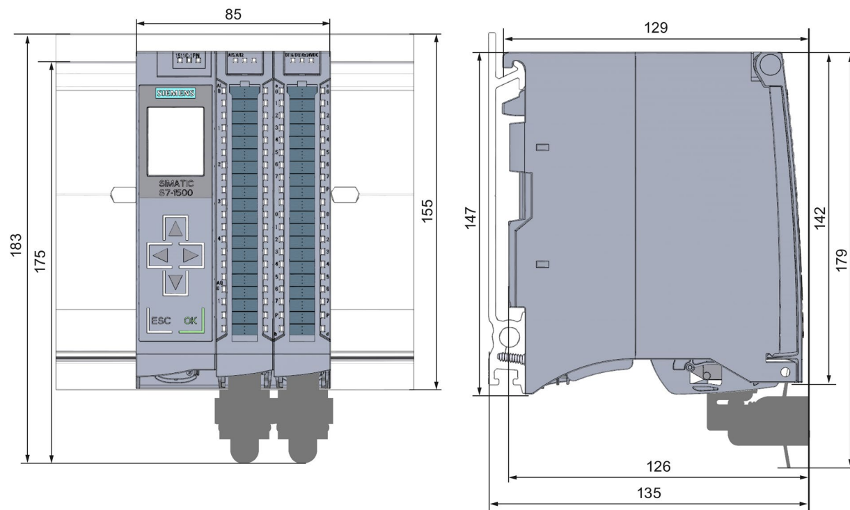
图 A-1 CPU 1511C-1 PN 的尺寸图，正视图和侧视图
