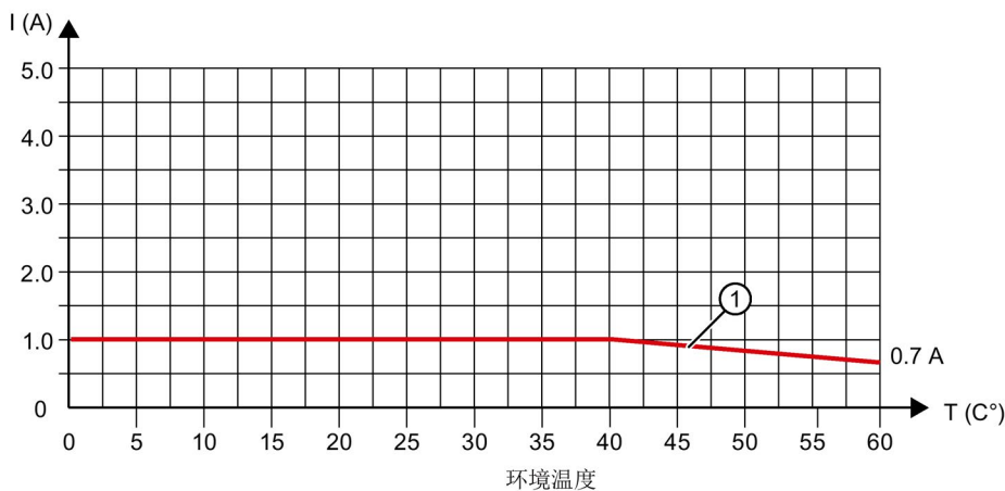
图 7-3 使用工艺功能时，编码器为数字量输入提供的额定负载电流
