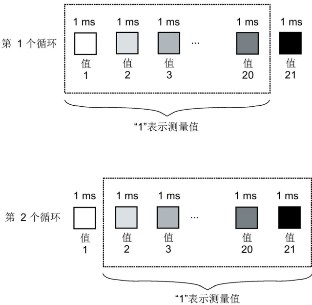
图 C-3 干扰频率抑制 50 Hz
