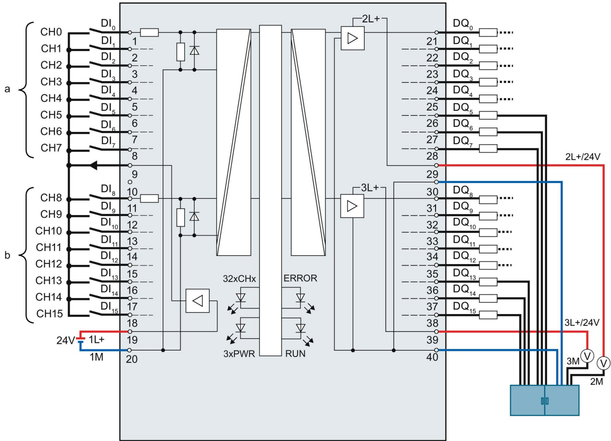
图 4-12 正确接线
