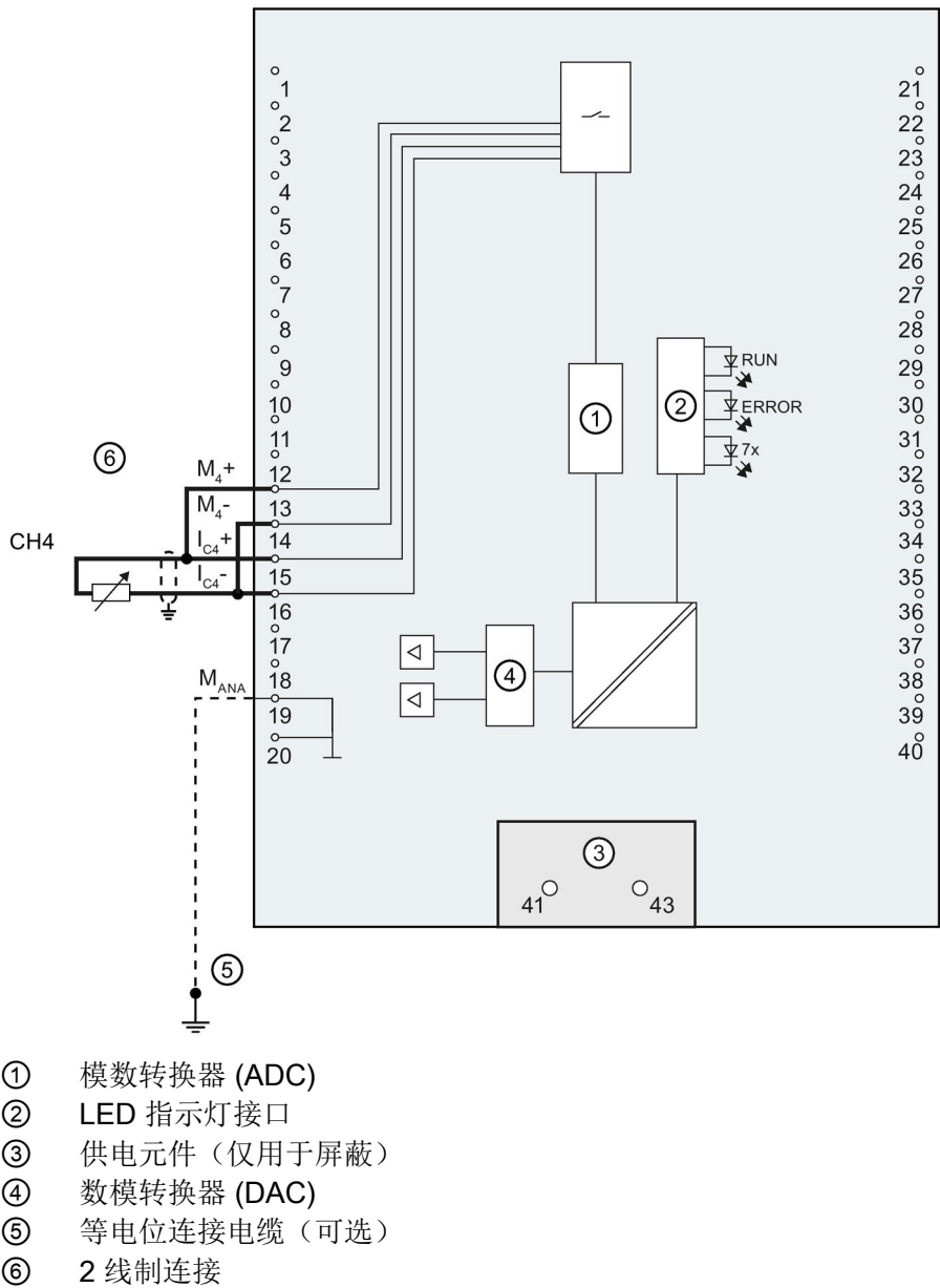
图 4-8 2 线制连接的方框图和端子分配
