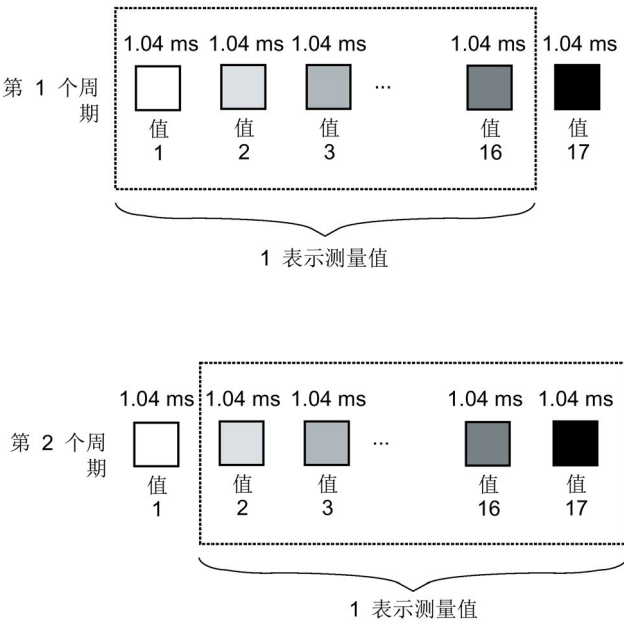
图 C-2 60 Hz 时的干扰频率抑制
