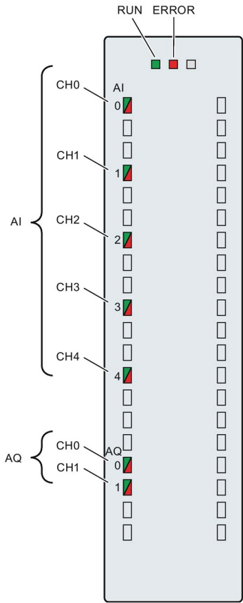
图 6-2 LED 指示灯
