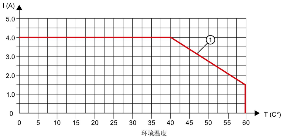
图 7-2 使用工艺功能时，数字量输出的负载额定值
