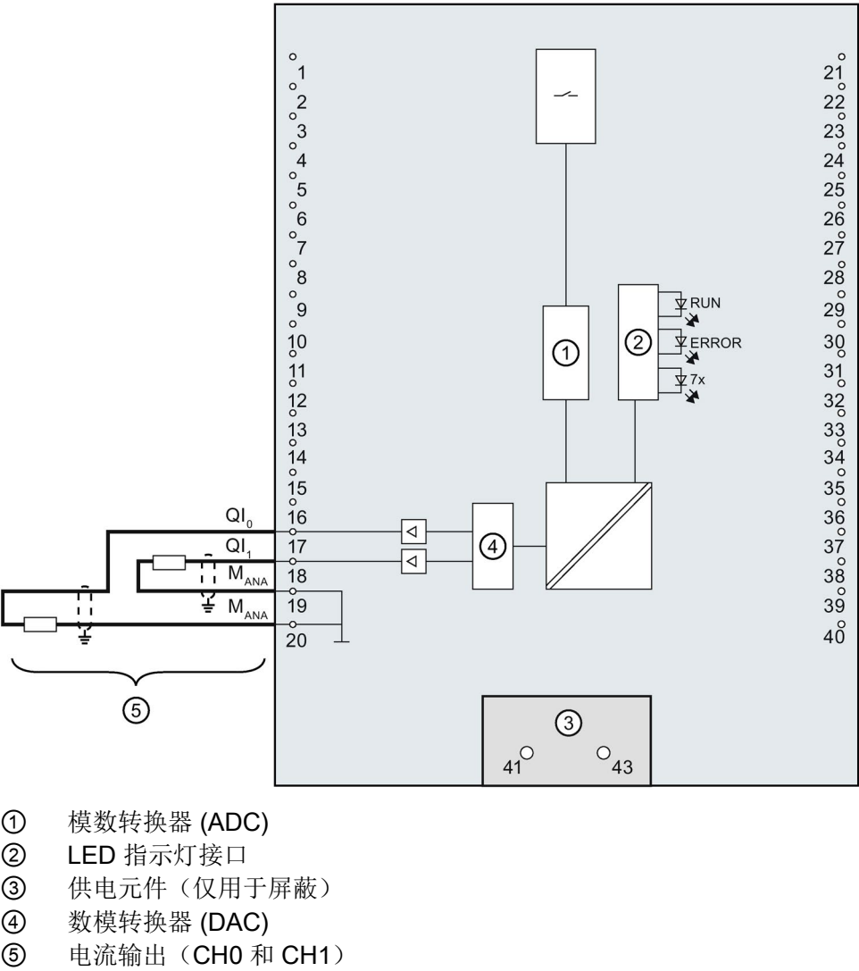
图 4-10 电流输出的方框图和端子分配
