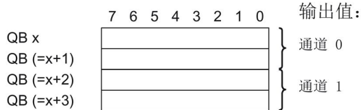
图 5-1 7 通道板载 I/O 的地址空间（带值状态）
