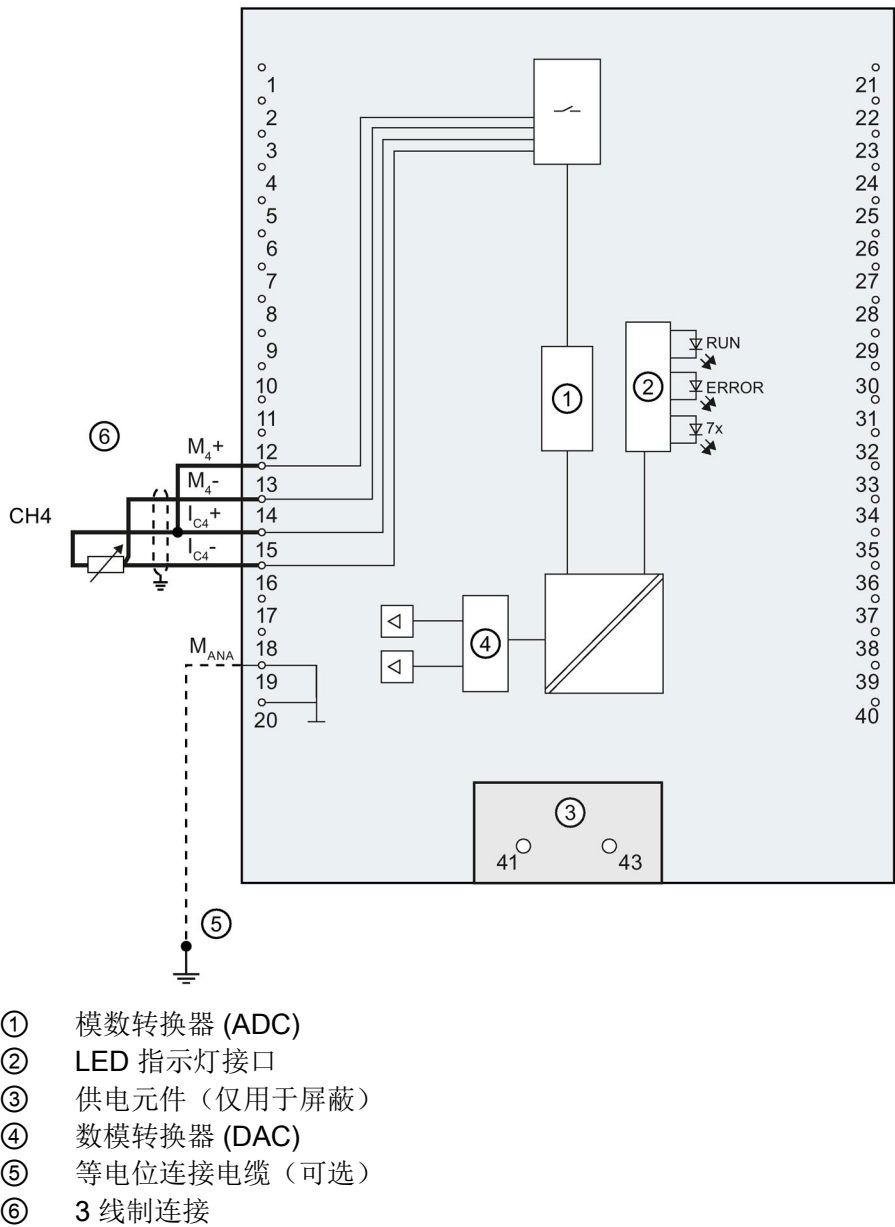
图 4-7 3 线制连接的方框图和端子分配
