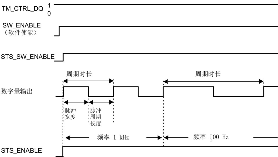
图 3-3 脉冲示意图
