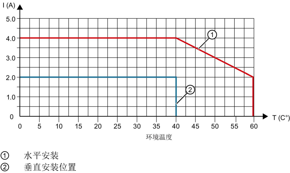
图 7-1 不同安装位置处，数字量输出的负载能力
