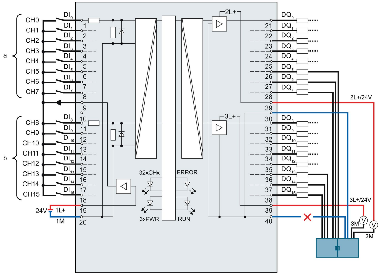
图 4-15 第二根接地电缆断路
