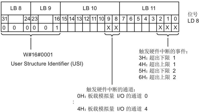
图 6-4 组织块的启动信息
