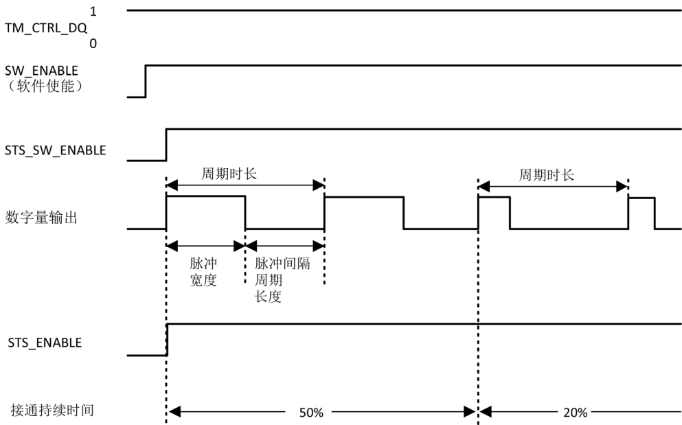
图 3-1 脉冲示意图
