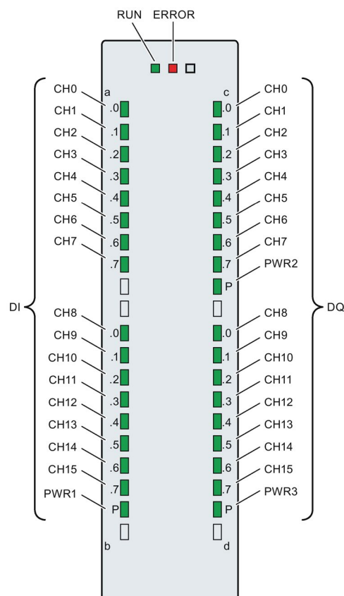
图 6-3 LED 指示灯
