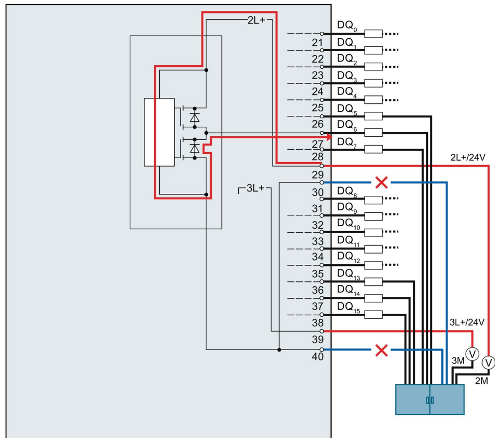
图 4-16 两根接地电缆同时断路时的电流。
