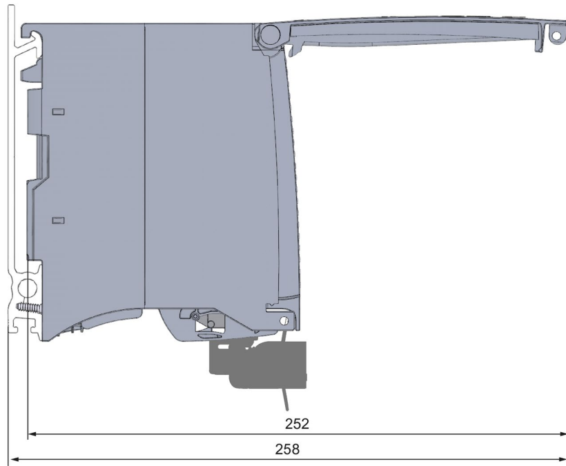
图 A-2 CPU 1511C-1 PN 的尺寸图，前面板打开时的侧视图
