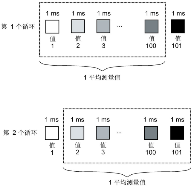
图 C-4 10 Hz 时的干扰频率抑制
