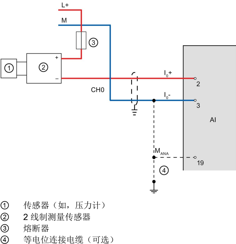
图 4-5 通道 0 处的 2 线制测量传感器
