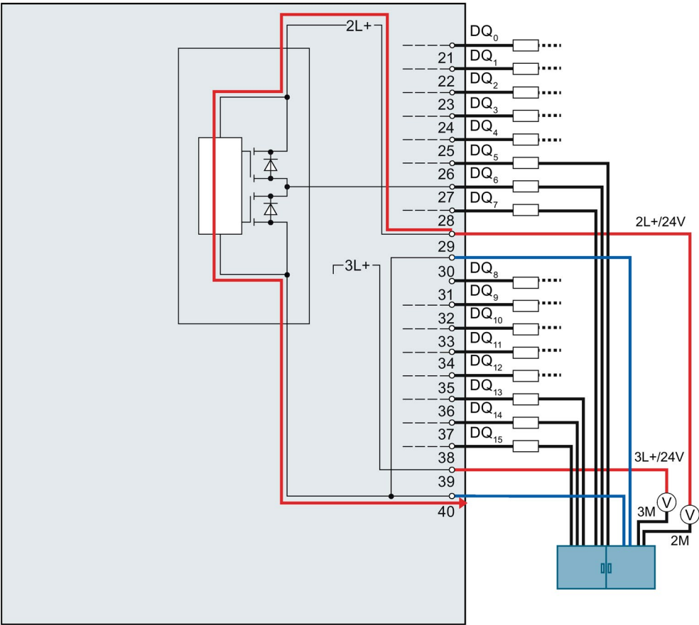
图 4-13 下图为正确接线时的电流。
