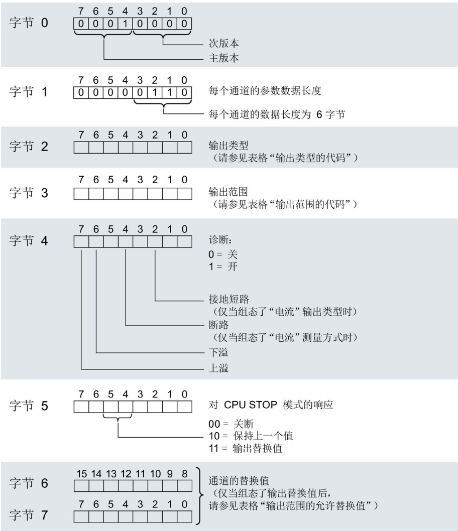
图 B-3 数据记录 64 的结构：字节 0 到 7
