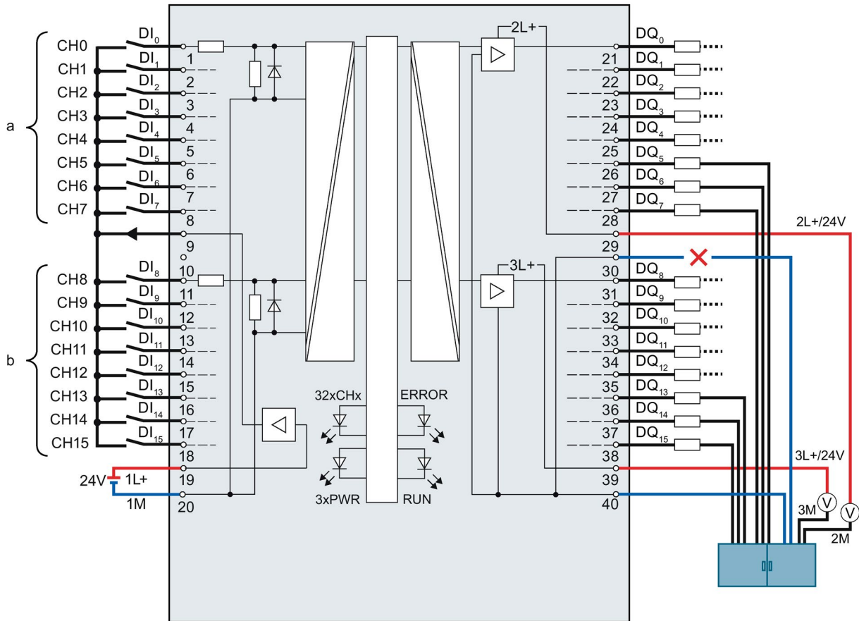
图 4-14 第一根接地电缆断路
