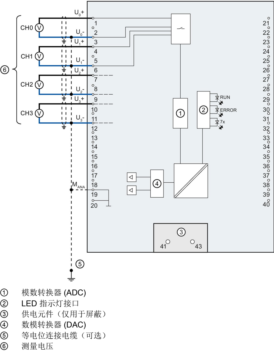
图 4-3 电压测量的方框图和端子分配
