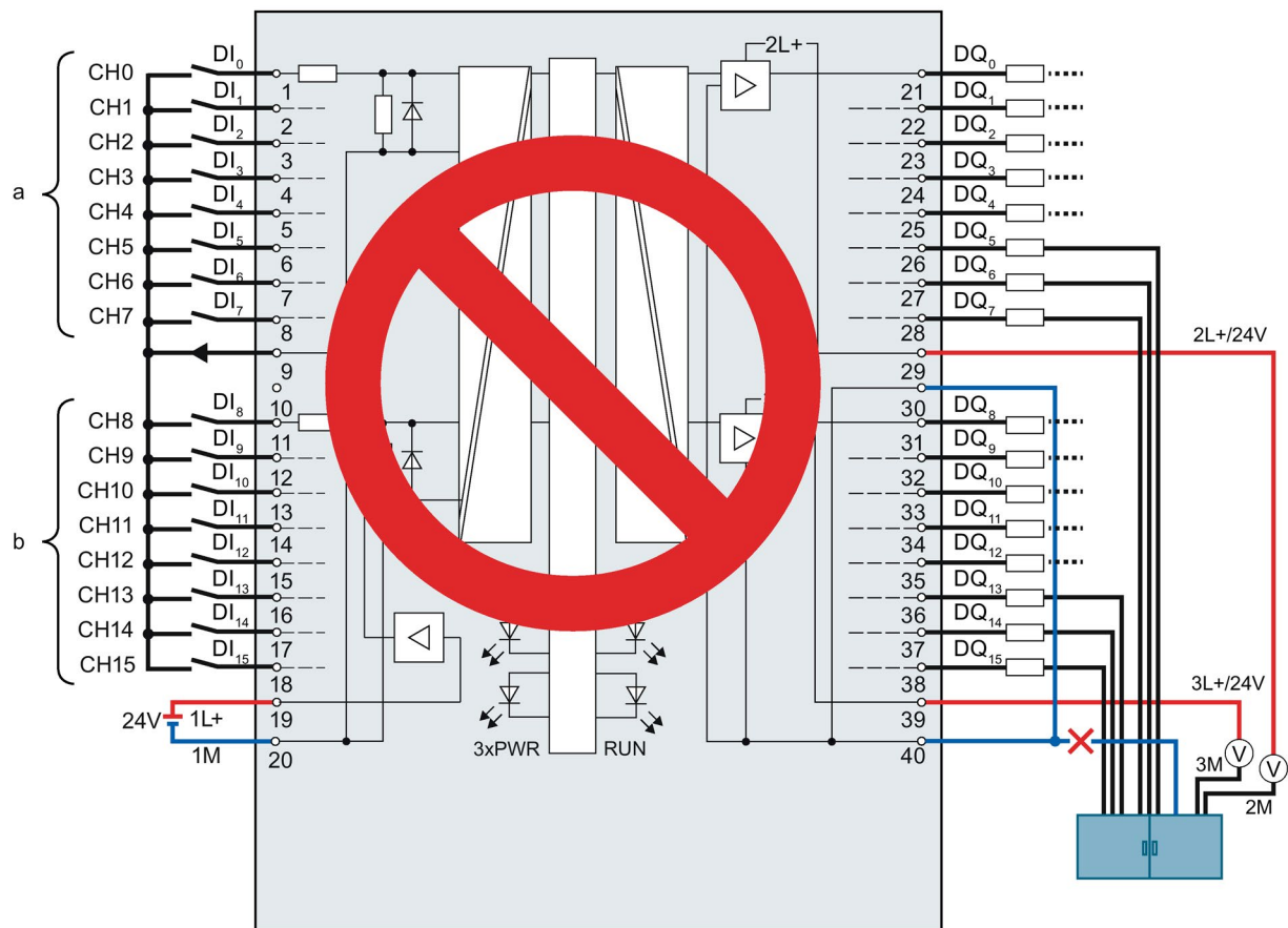
图 4-17 错误接线：电路桥
