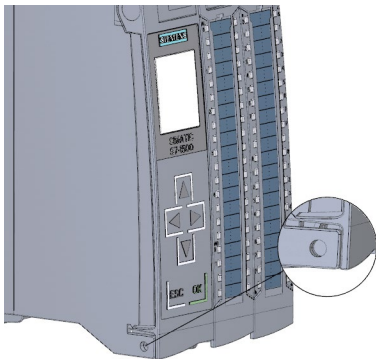
图 2-5 CPU 上的锁扣装置
