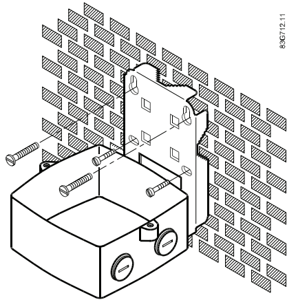
图 4-5 墙式安装
