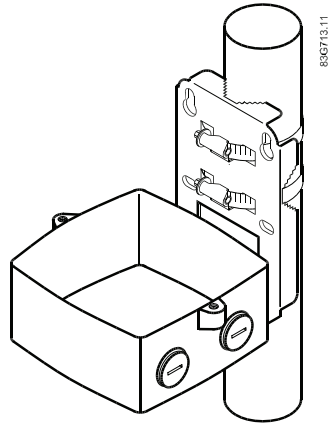
图 4-6 管道安装 - 垂直
