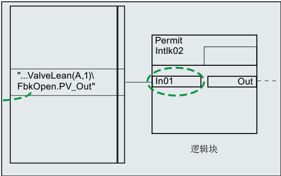
控制模块“ValveLean1”的 CFC
