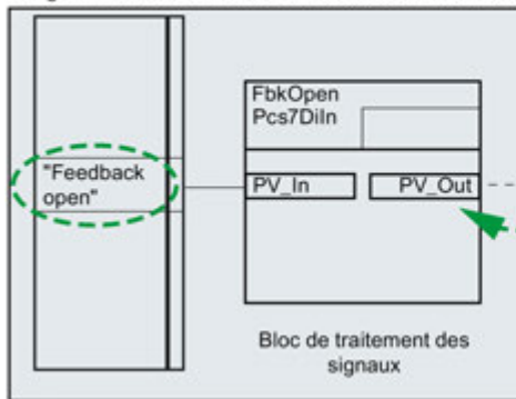
Diagramme CFC du module de commande "ValveLean"
