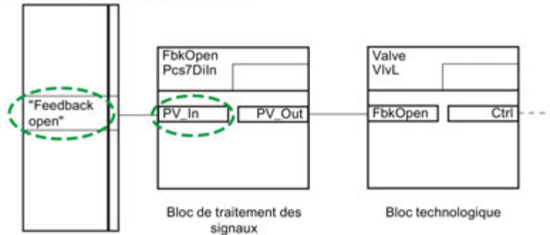
Diagramme CFC du module de commande
