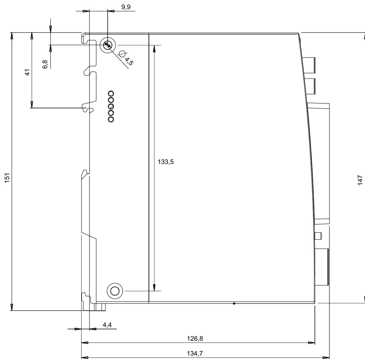
Bild 10-2 Seitenansicht
