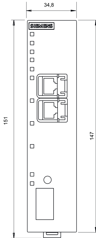
Bild 10-1 Vorderansicht
