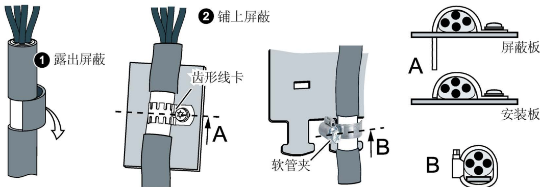
图 4-4 符合 EMC 规定的屏蔽层敷设示例
