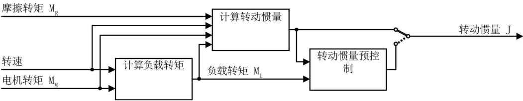
图 6-54 转动惯量测定器的功能一览
