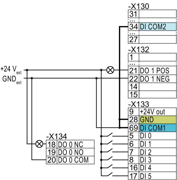
连接源型触点和外部电源
