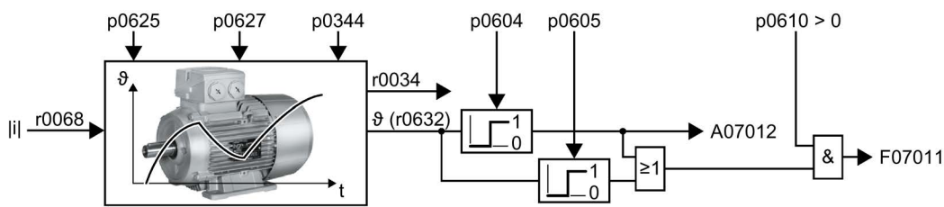
图 6-58 感应电机的热模型 2
