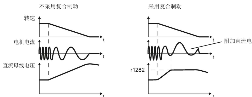
图 6-55 电机制动：无复合制动，有复合制动
