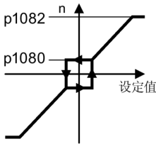
图 5-9 电机的最大转速和最小转速
