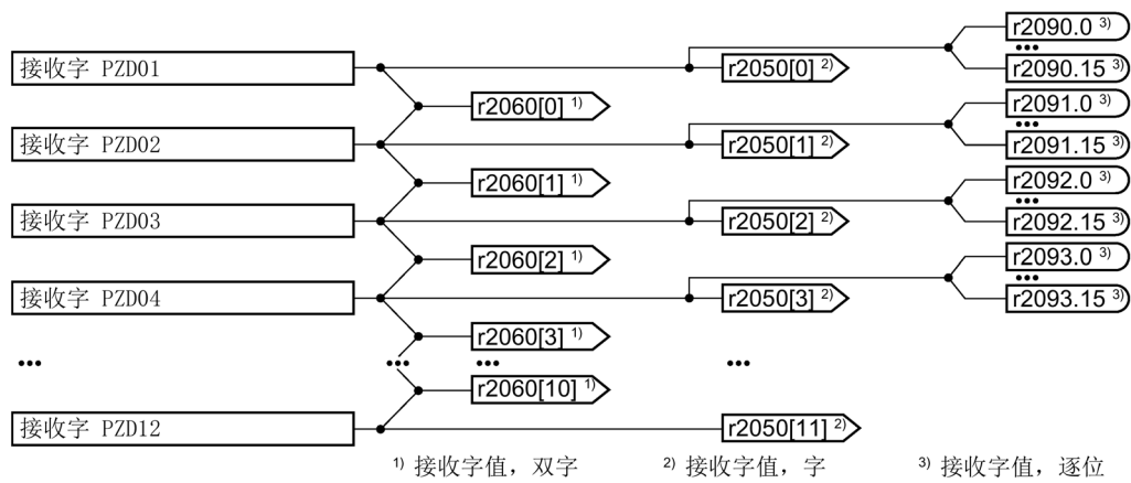
图 6-11 接收字的互联
