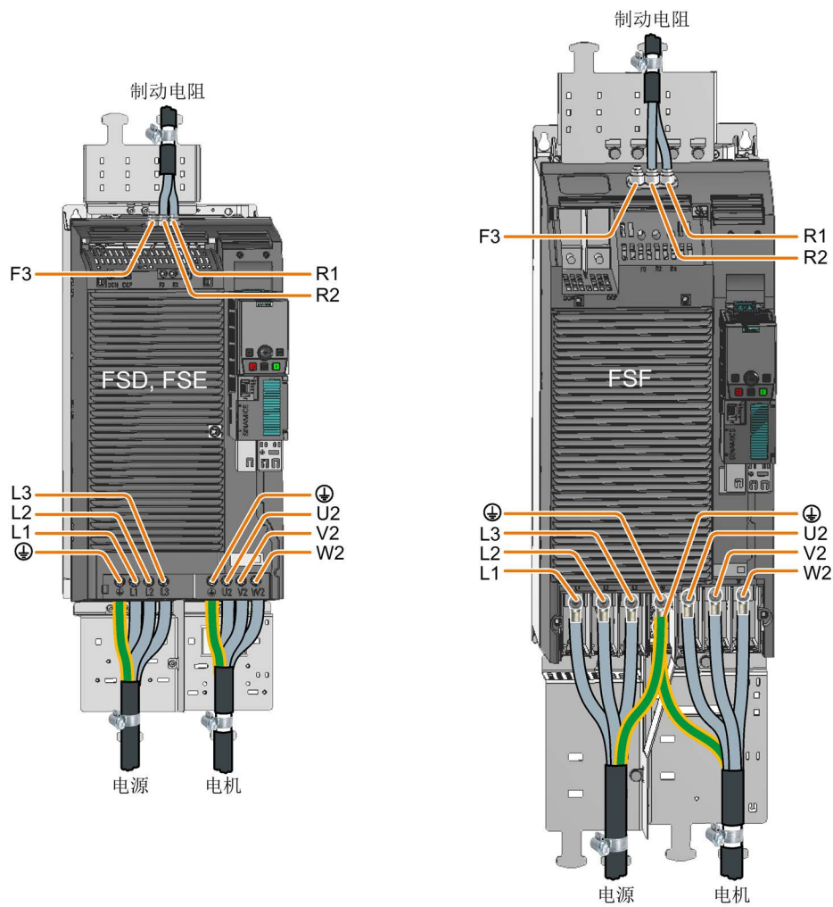
图 4-18 电源、电机和制动电阻的连接器
