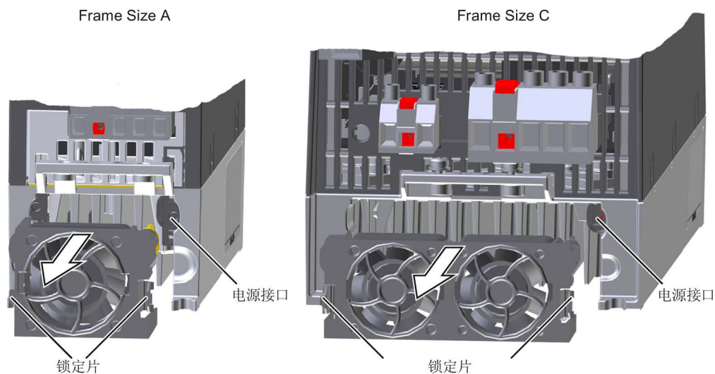
图 9-1 拆卸散热器的风扇单元
