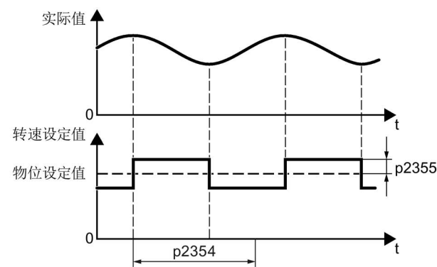
图 6-42 自动优化时的转速设定值和过程实际值示例
