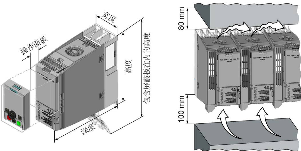
图 4-7 尺寸和与其他设备之间的最小间距，FSAA ... FSC
