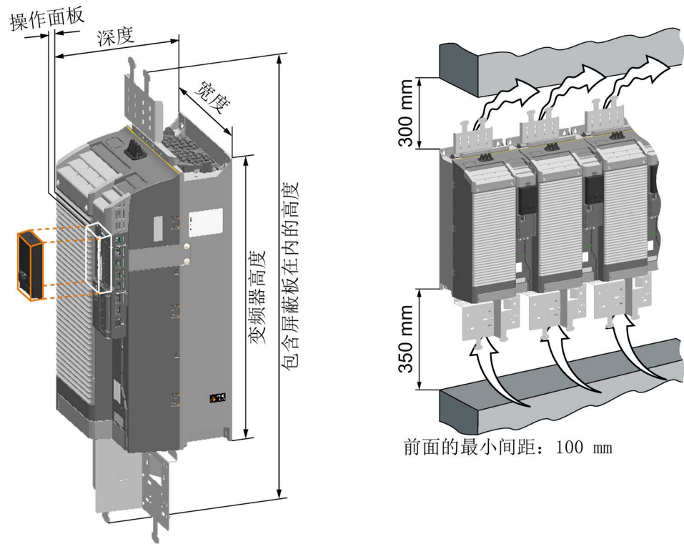
图 4-8 尺寸和与其他设备之间的最小间距，FSD ... FSF
