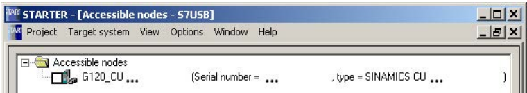
图 5-13 在 STARTER 中找到的变频器
