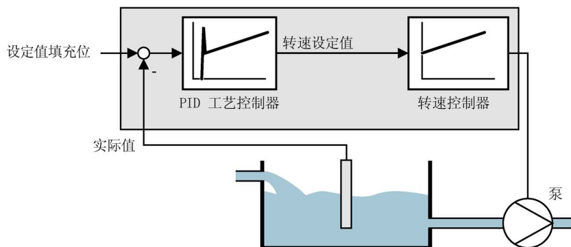
图 6-39 示例：工艺控制器用作流量控制器
