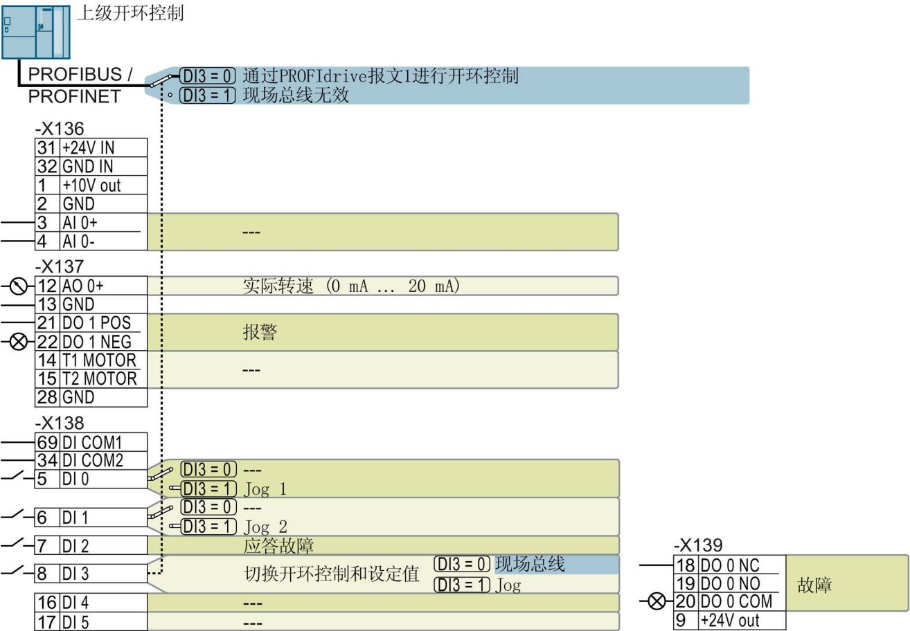
图 4-23 G120C DP 和 G120C PN 的 FSAA ... FSC 出厂设置
