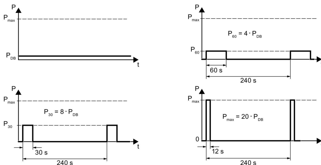
图 10-8 制动电阻接通持续时间的脉冲功率 P_{\text{max}} 、额定功率 P_{\text{DB}} 和示例
