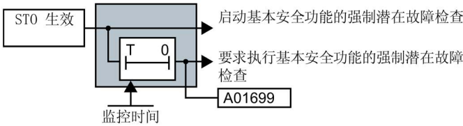
图 6-27 强制潜在故障检查的启动和监控 (Teststopp)
