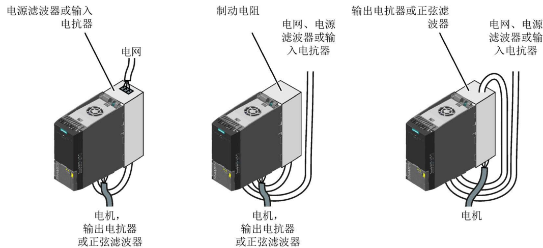
图 4-5 可用的底座型部件
