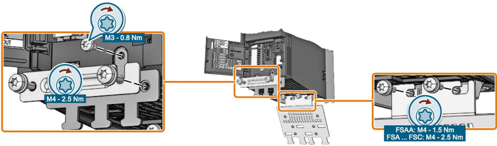
图 4-9 安装屏蔽板，FSAA ... FSC
