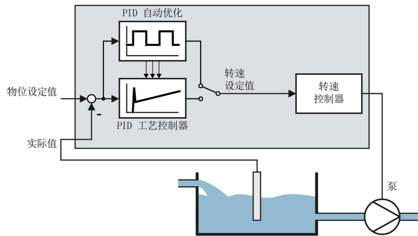
图 6-41 PID 控制器的自动优化示例（物位调节）
