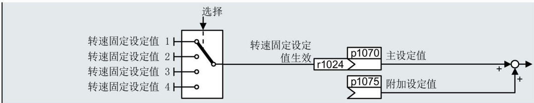
图 6-34 转速固定设定值设为设定值源
