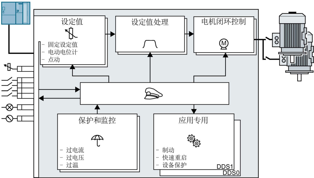
图 6-69 在变频器内切换传动数据组
