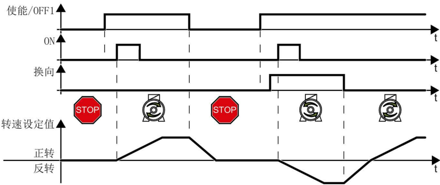
图 6-9 三线制控制，方法 2
