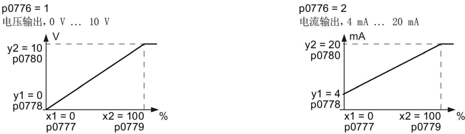
图 6-4 定标特性曲线示例
