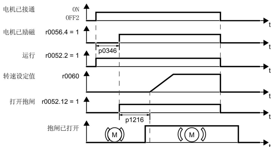
图 6-20 发出 OFF2 指令后电机抱闸的控制方式
