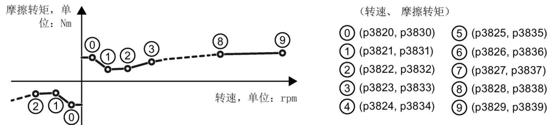
图 6-51 摩擦特性曲线
