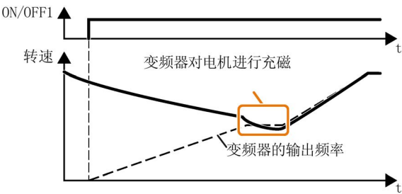
图 6-61 捕捉重启的基本工作方式
