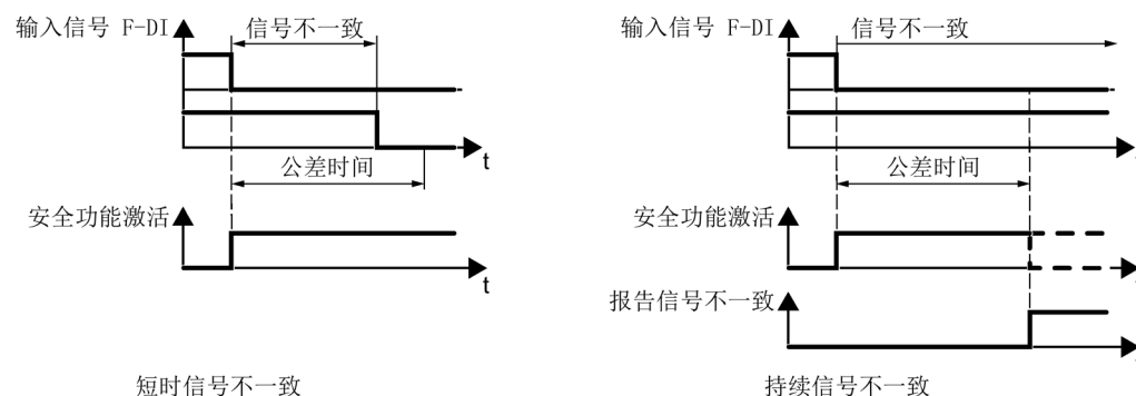
图 6-24 差异时间一致性监控
