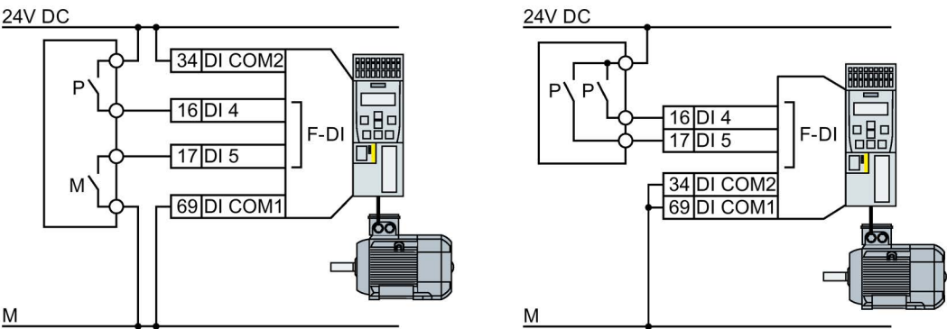
图 A-9 源型和漏型故障安全数字量输出的接线
