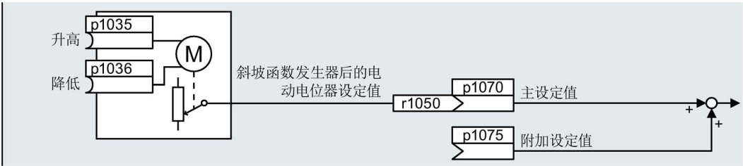
图 6-32 电动电位器设为设定值源
