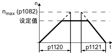
图 5-6 电机的升降时间
