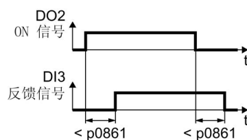
图 6-66 通过 DO 2 的电源接触器控制，带通过 DI 3 的反馈信息
