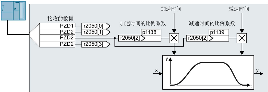
图 6-38 运行中修改斜坡函数发生器时间的示例
