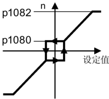
图 5-5 电机的最小转速和最大转速
