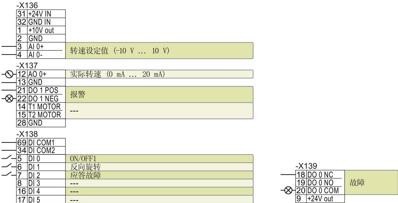
图 4-22 G120C USS 的 FSAA ... FSC 出厂设置
