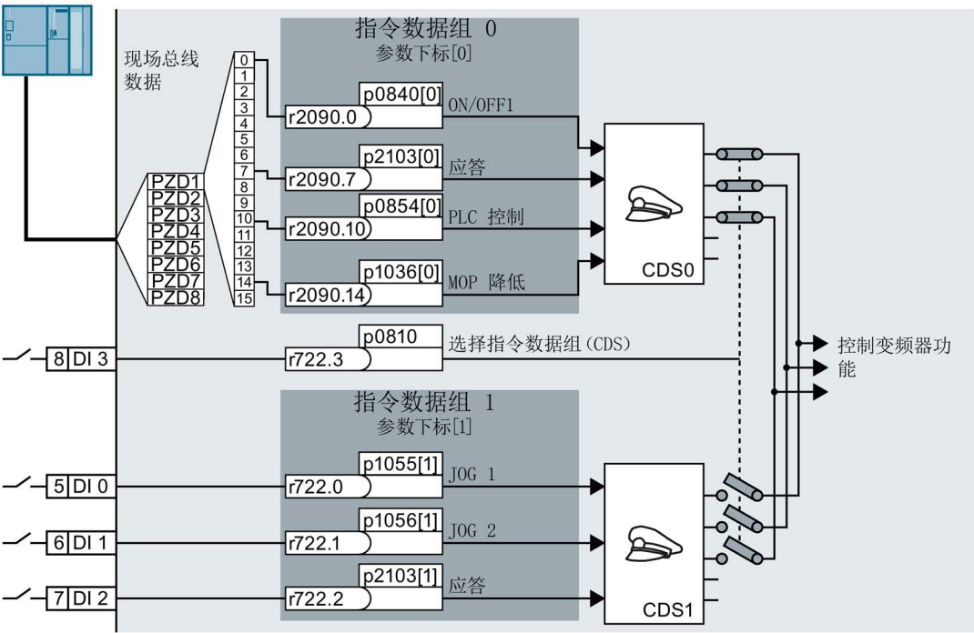
图 6-16 示例：控制方式从端子排切换到 PROFIBUS 或 PROFINET
