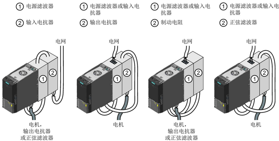
图 4-6 允许的底座型部件组合
