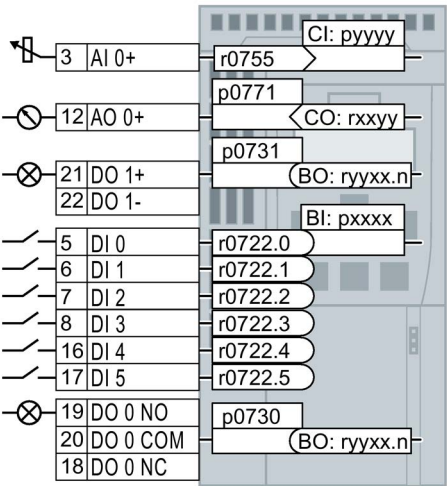
图 6-2 变频器中输入和输出的互联
