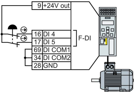
图 A-10 传感器（如：急停蘑菇按钮、限位开关）的接线
