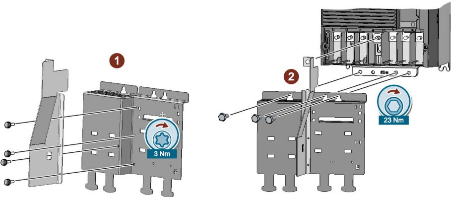
图 4-11 安装下方屏蔽板，FSF
