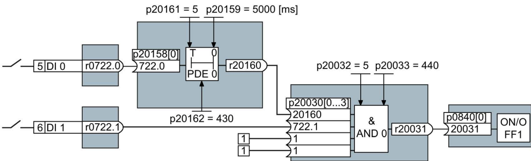
图 A-7 示例：控制逻辑信号互联
