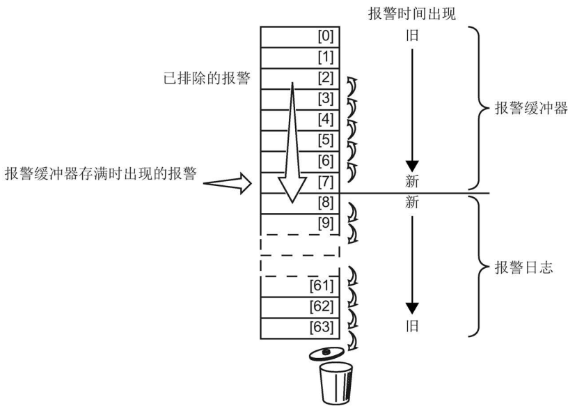
图 8-2 已排除的报警转移到报警日志中
