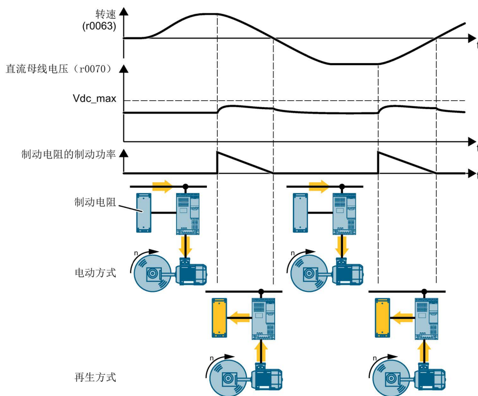
图 6-56 电阻制动的简单时序图
