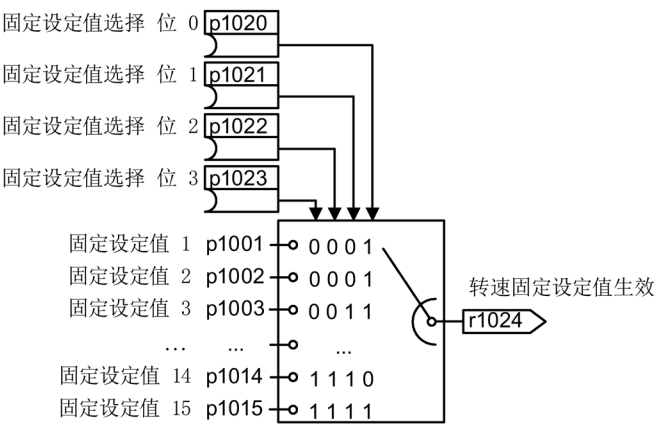
图 6-36 二进制选择转速固定设定值的简易功能图
