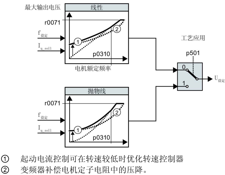
图 6-46 选择应用等级Standard Drive Control后的特性曲线
