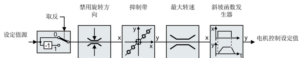
图 6-37 变频器内的设定值处理
