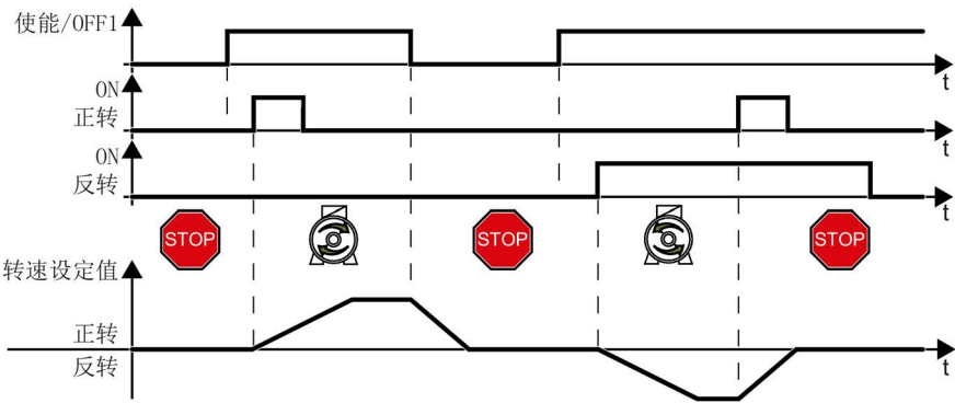
图 6-8 三线制控制，方法 1
