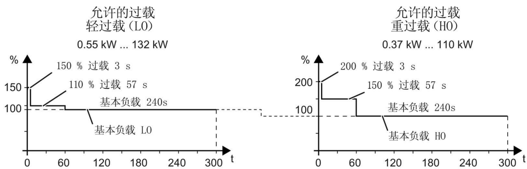
图 10-1 重过载和轻过载的工作周期
