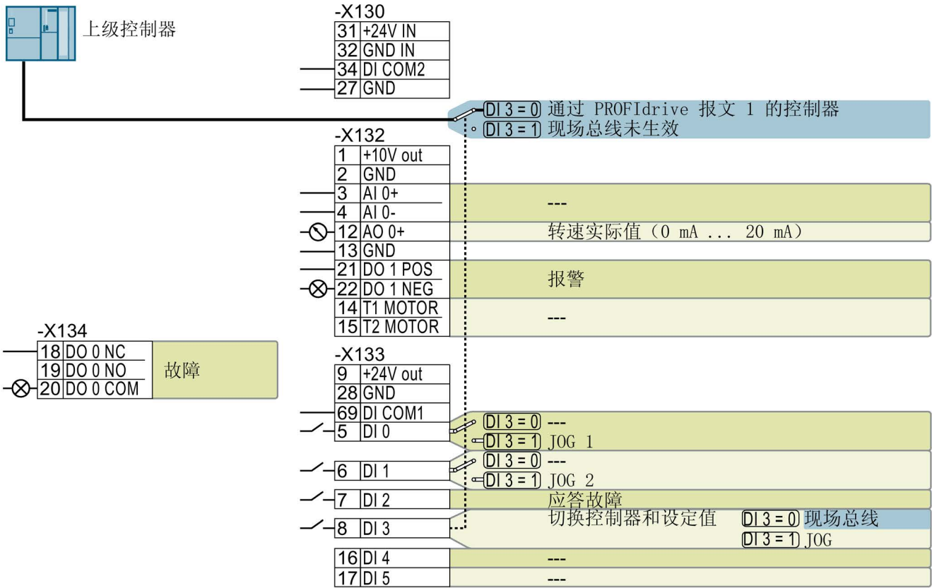
图 4-24 G120C PN 的 FSD ... FSF 出厂设置
