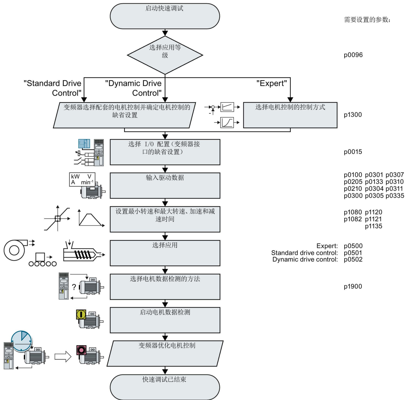
图 5-15 使用 PC 进行快速调试
