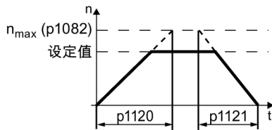
图 5-10 电机的升降时间
