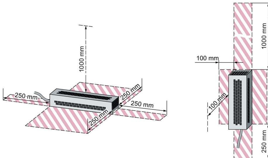
图 4-15 地面安装或墙面安装时制动电阻的最小间距
