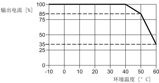
图 10-5 允许的输出电流和环境温度的函数关系，FSAA ... FSC
