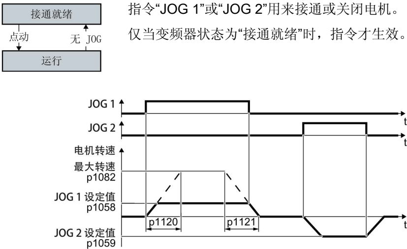
图 6-15 JOG时电机的工作时序
