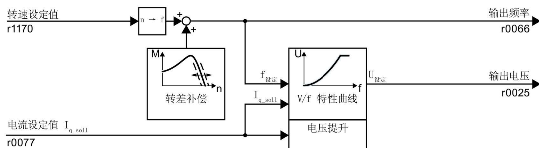
图 6-44 选择Standard Drive Control后的 V/f 控制的预设置
