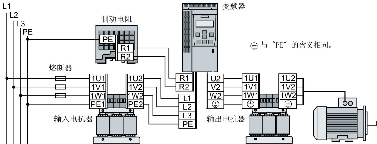
图 4-17 变频器及其可选组件的连接
