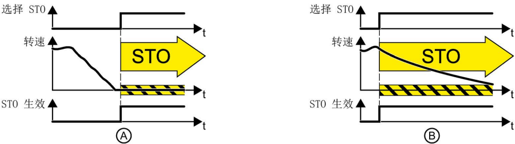
图 6-21 静态电机 (A) 和旋转电机 (B) 上的 STO 功能的工作原理
