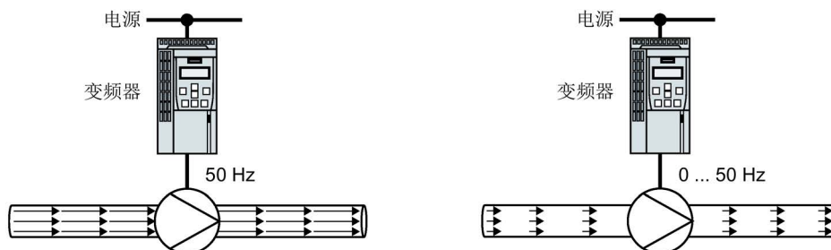
图 6-68 使用泵和变频器的流体控制
