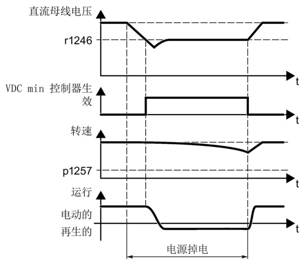
图 6-64 动能缓冲的工作原理
