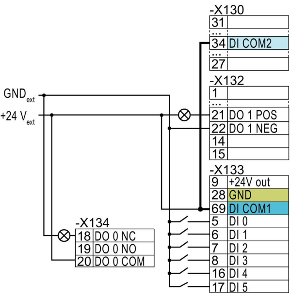
连接漏型触点和外部电源
