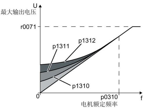
图 6-47 线性特性曲线上的升压降低示例
