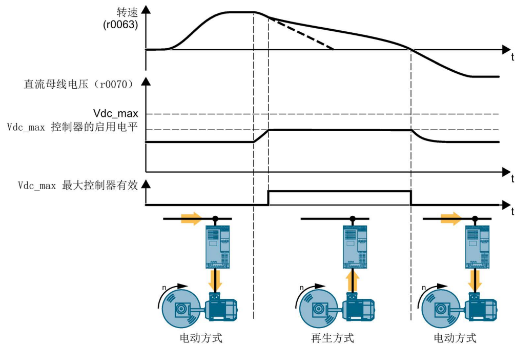
图 6-60 V dc_max 控制器的简化示意图
