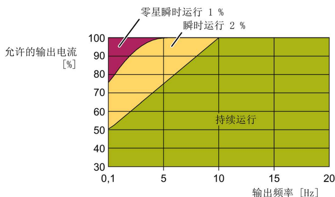
图 10-4 变频器允许的运行范围
