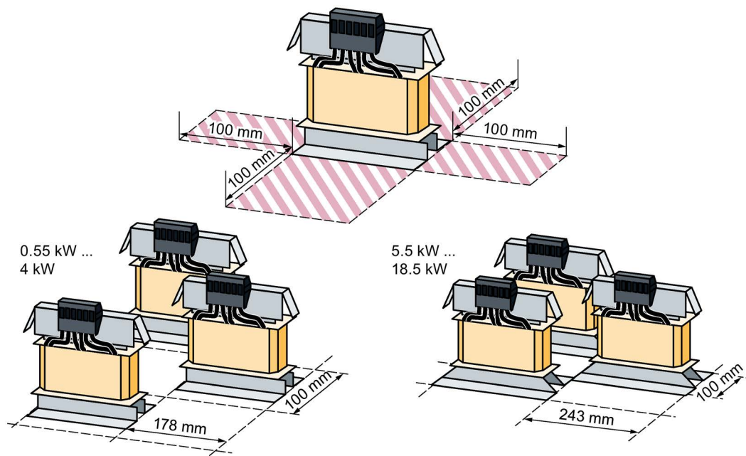
图 4-14 输出电抗器和其它设备之间的最小间距 - 节省空间的安装示例
