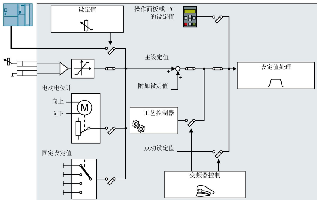
图 6-29 变频器的设定值源
