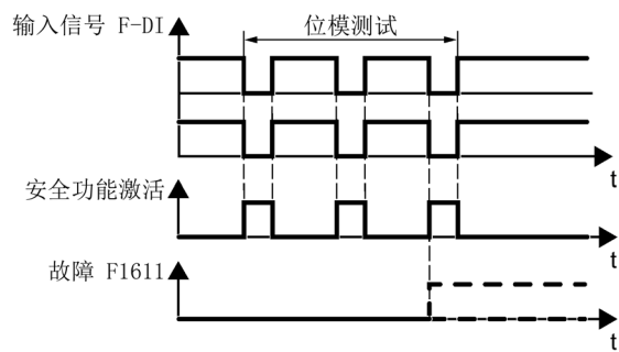
图 6-25 变频器对位模测试作出响应
