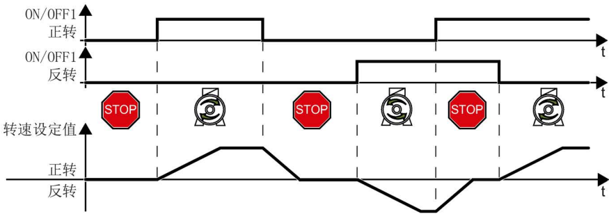
图 6-7 双线制控制，方法 3
