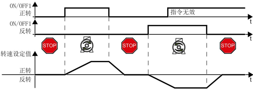
图 6-6 双线制控制，方法 2
