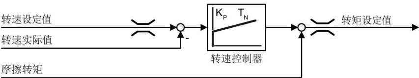
图 6-50 带摩擦转矩的转速控制器前馈控制
