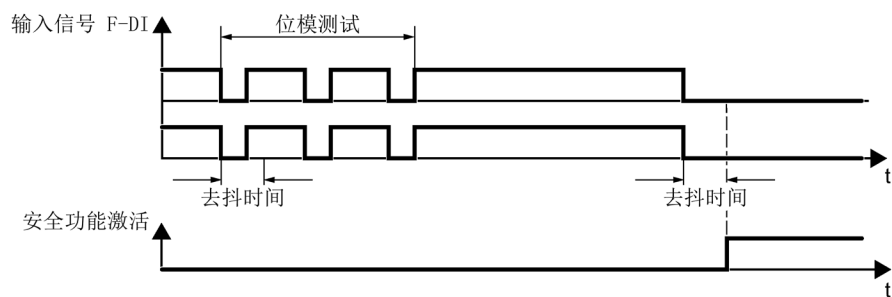
图 6-26 对短暂出现的信号进行滤波
