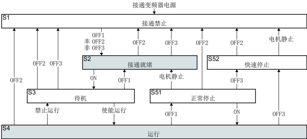
图 6-1 电机接通和关闭时变频器的内部顺序控制
