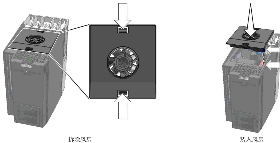
图 9-2 拆卸及安装内部风扇
