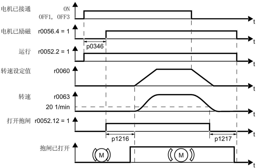
图 6-19 电机接通/关闭时电机抱闸的控制
