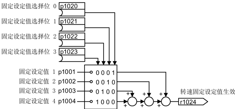
图 6-35 直接选择转速固定设定值的简易功能图
