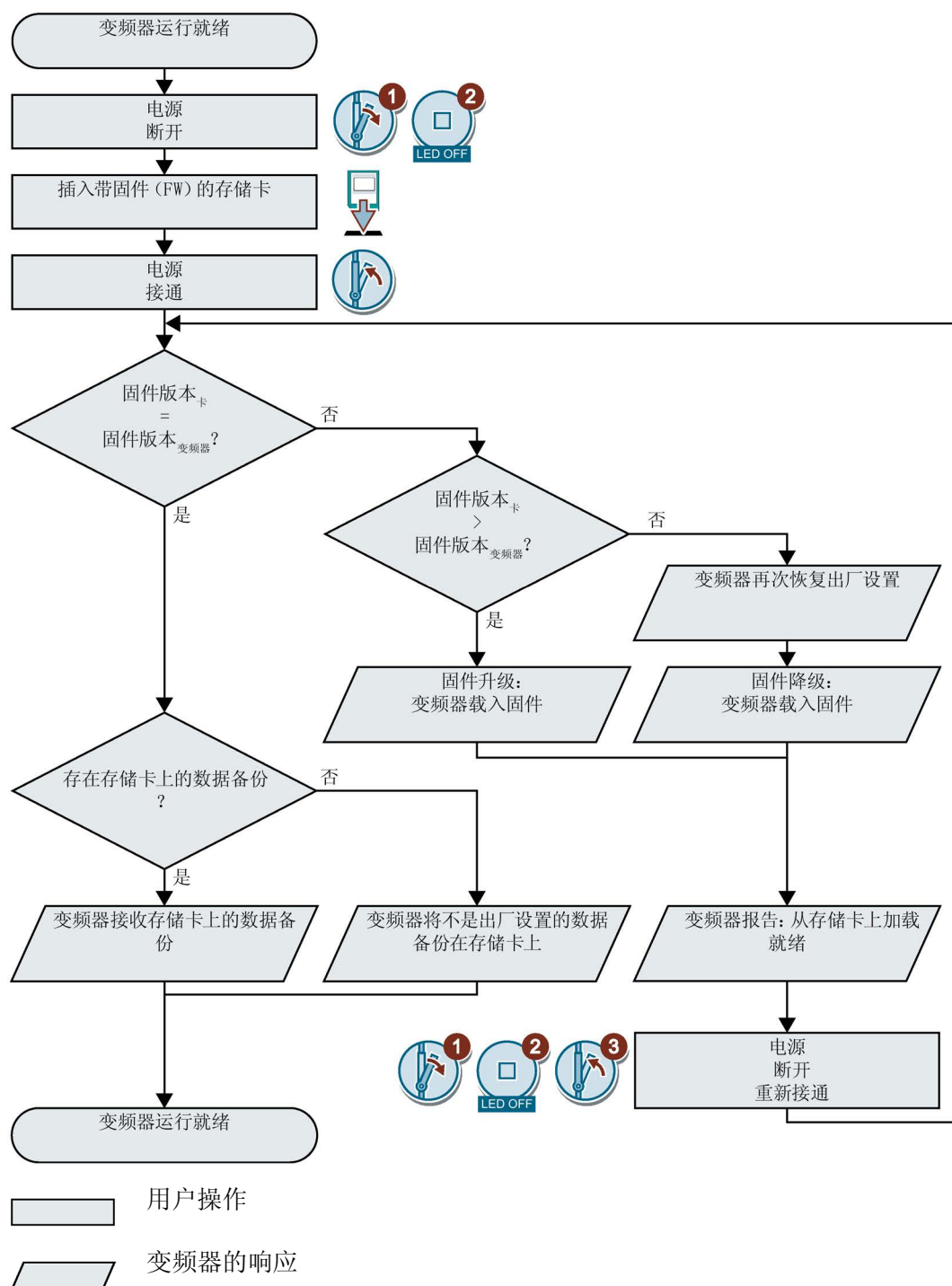
图 9-4 固件升级和降级一览
