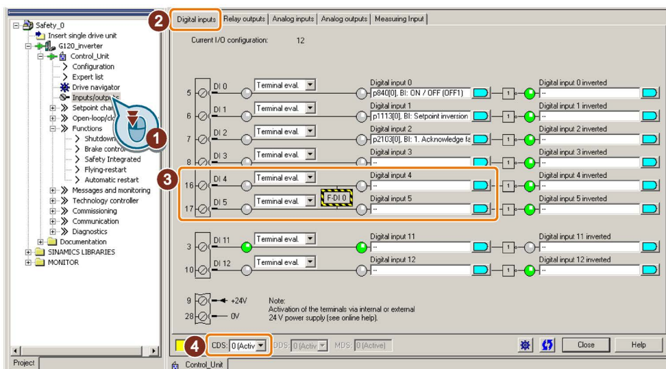
图 6-28 断开 DI 4 和 DI 5 的互联
