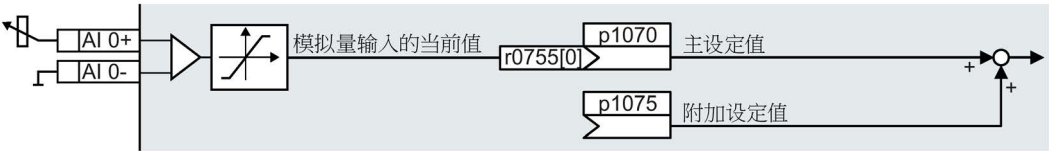
图 6-30 示例：模拟量输入 0 设为设定值源
