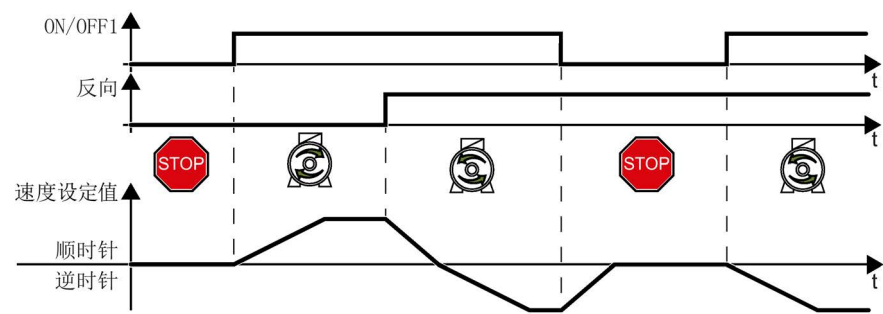
图 6-5 双线制控制：方法 1
