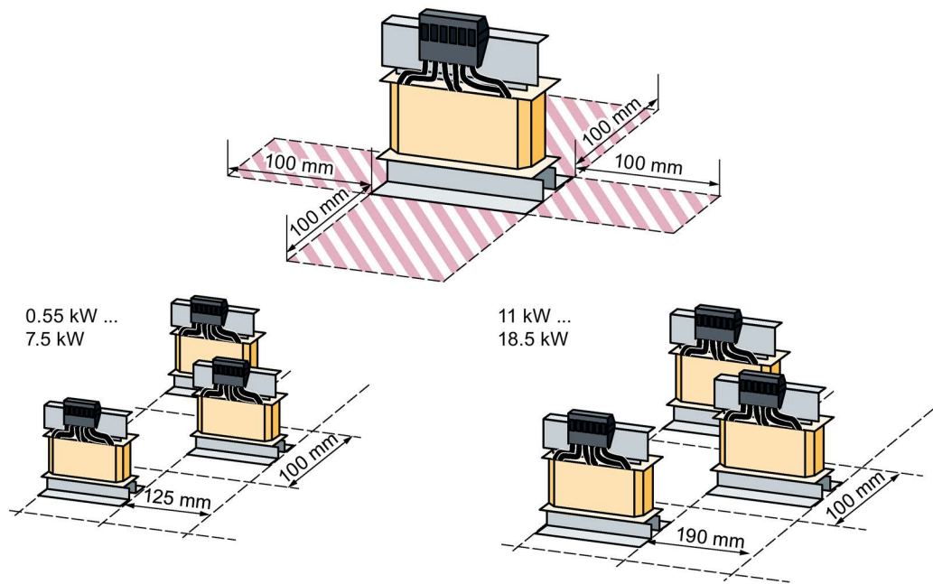
图 4-13 输入电抗器和其它设备之间的间距 - 节省空间的安装示例
