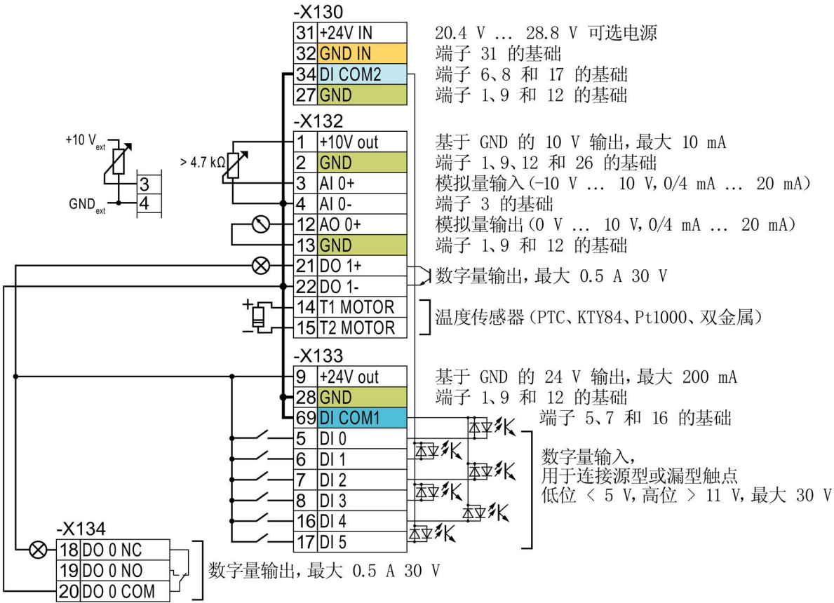
图 4-21 使用变频器内部 24 V 电源的数字量输入的布线示例
