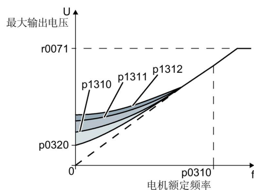
图 6-48 线性特性曲线上的升压降低示例
