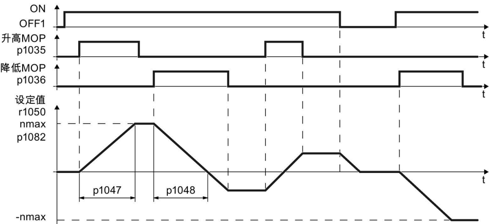
图 6-33 电动电位器的功能图
