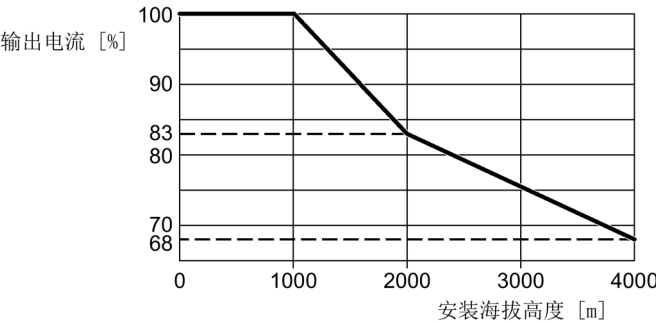
图 10-3 FSD ... FSF 的特性曲线
