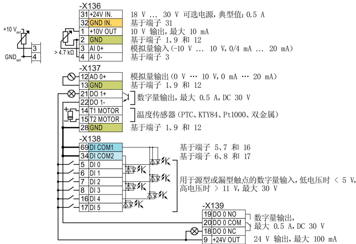
图 4-20 使用变频器内部 24 V 电源的数字量输入的布线示例
