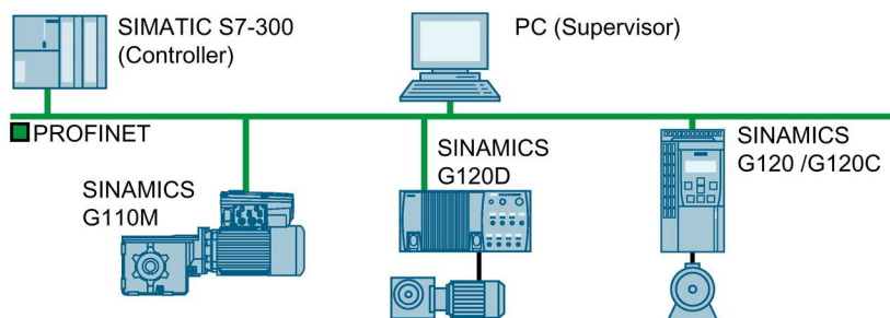
图 4-28 变频器在 PROFINET IO 模式中
