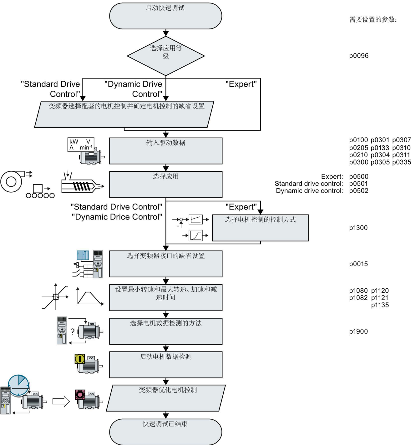
图 5-4 使用操作面板 BOP-2 进行快速调试
