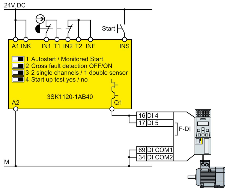
图 A-11 安全开关设备（如 SIRIUS 3SK11）的接线
