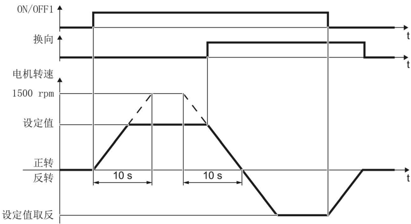
图 5-2 出厂设置中电机的接通、关闭和换向
