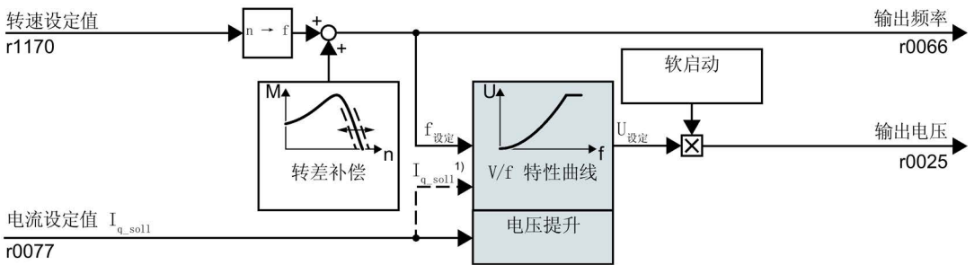
图 6-43 V/f 控制的简易功能图
