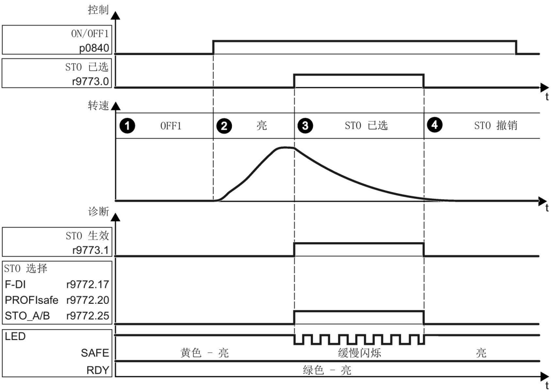
图 A-13 基本安全功能 STO 的验收测试
