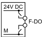
漏型数字量输出
