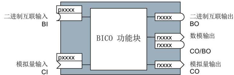
图 A-6 二进制输入/输出和模拟量输入/输出的符号
