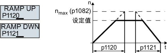
图 5-8 电机的升降时间
