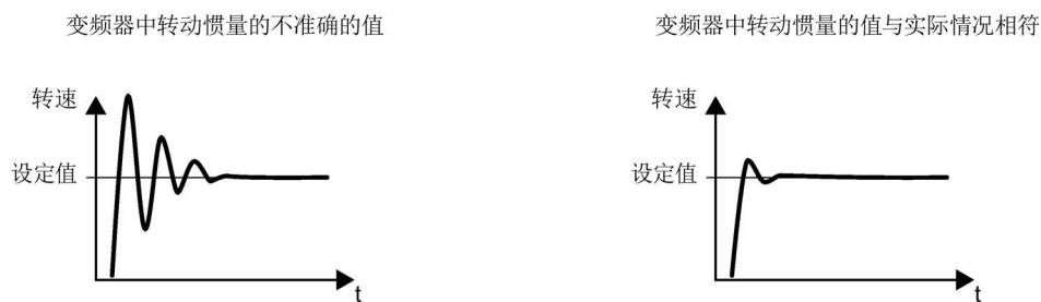
图 6-53 转动惯量对转速的影响
