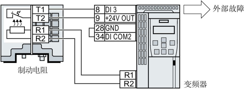
图 4-27 示例：通过控制单元的数字量输入 DI 3 进行制动电阻的温度监控
