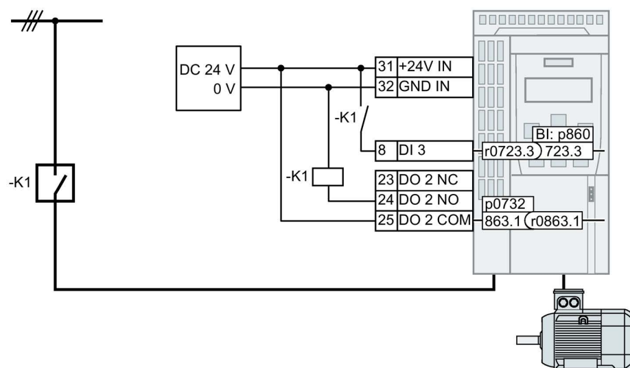
图 6-65 通过 DO 2 的电源接触器控制，带通过 DI 3 的反馈信息
