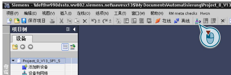
图 5-12 Startdrive 中的“Accessible nodes”
