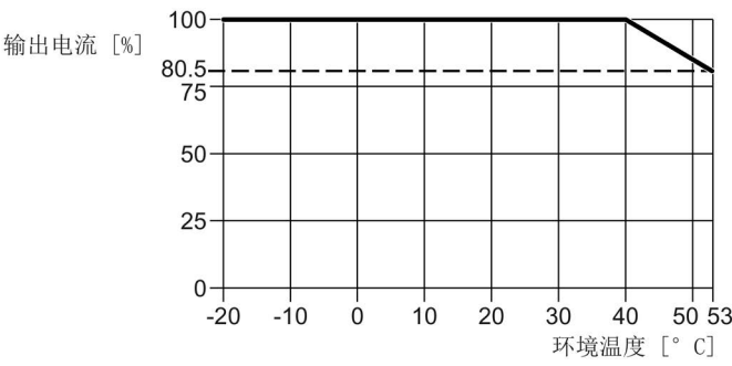
图 10-6 允许的输出电流和环境温度的函数关系，FSD ... FSF
