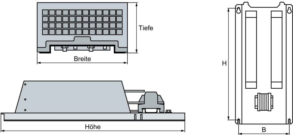
图 4-16 制动电阻的尺寸
