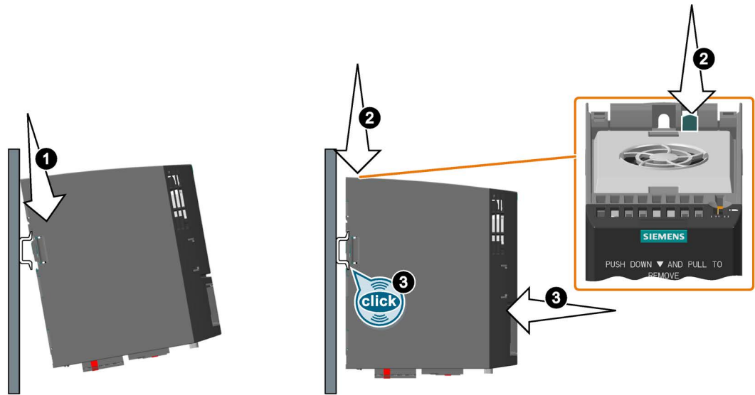
图 4-12 在导轨上固定
