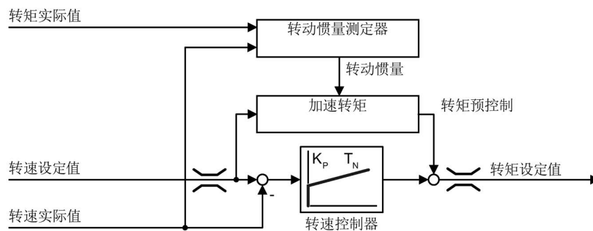
图 6-52 转动惯量测定器对转速控制的影响
