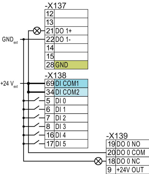
将漏型触点与外部电源连接
