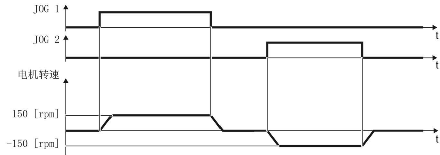
图 5-3 出厂设置中电机的JOG模式
