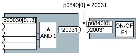
图 A-8 设置 p0840[0] = 20031，连接功能块
