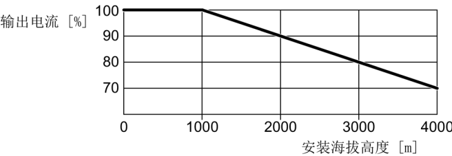
图 10-2 FSAA ... FSC 的特性曲线
