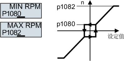
图 5-7 电机的最小转速和最大转速
