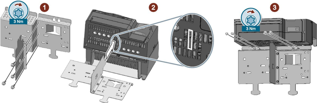
图 4-10 安装下方屏蔽板，FSD 和 FSE
