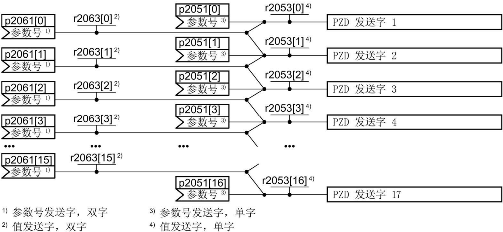
图 6-10 发送字的互联
