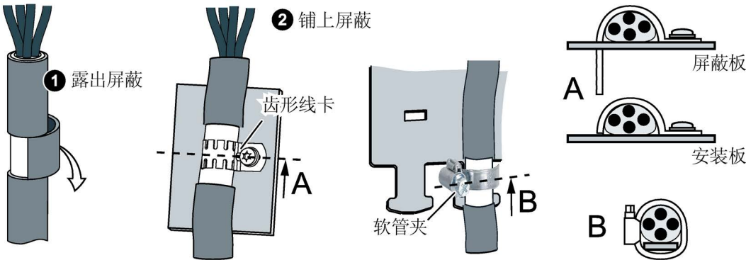
图 4-26 电磁兼容屏蔽层
