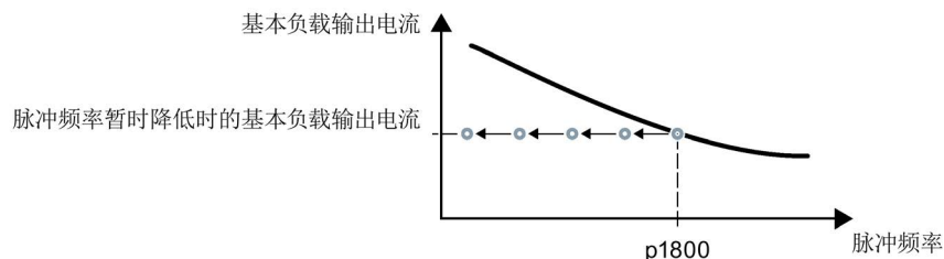
图 6-57 过载时的降容特性曲线和基本负载输出电流
