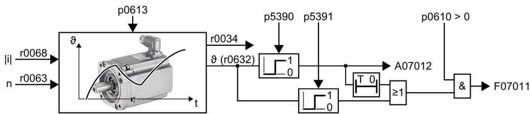
图 6-59 用于无编码器同步电机 1FK7 的电机热模型 3
