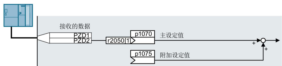
图 6-31 现场总线设为设定值源
