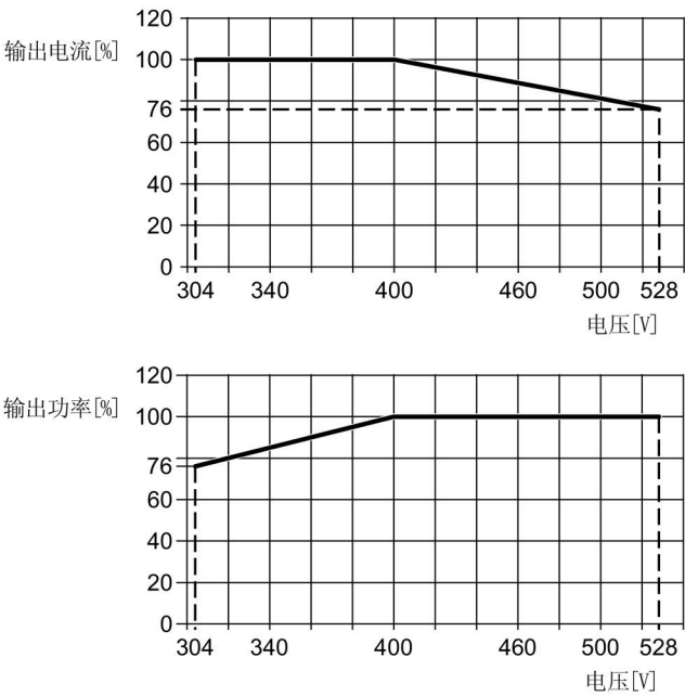
图 10-7 电流和电压降容与输入电压的函数关系
