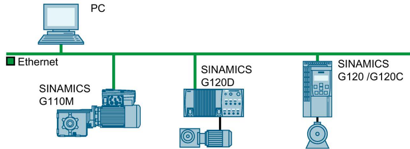
图 4-29 变频器作为以太网节点
