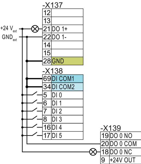
将源型触点与外部电源连接
