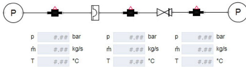
Bild 8-73 Verschaltungsmöglichkeit des Komponententyps RuptureDisc
