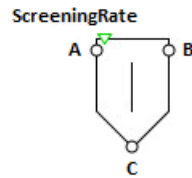
Bild 8-52 Symbol des Komponententyps Separator
