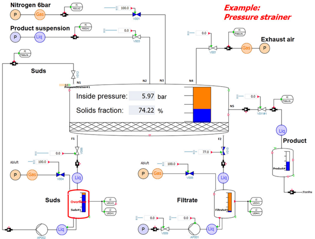
Bild 8-49 Beispielverschaltung des Komponententyps PressureStrainer
