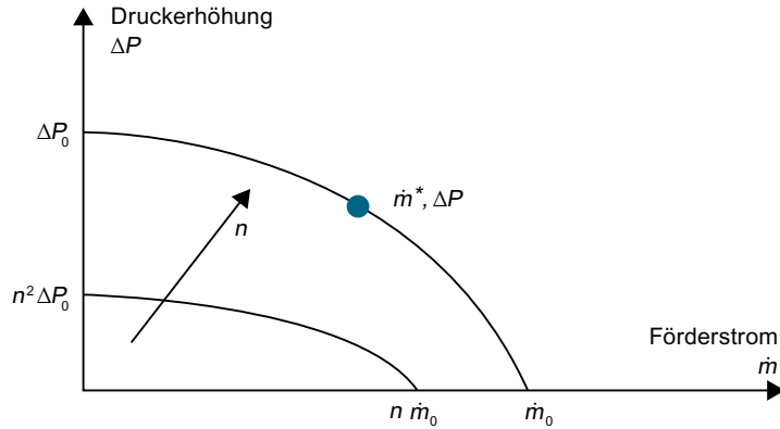
Bild 8-40 Pumpenkennlinie qualitativ
