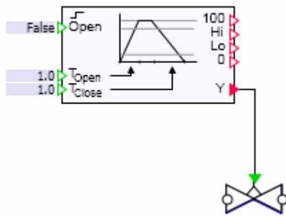
Bild 8-2 Kopplung des Komponententyps Valve mit einem Antrieb
