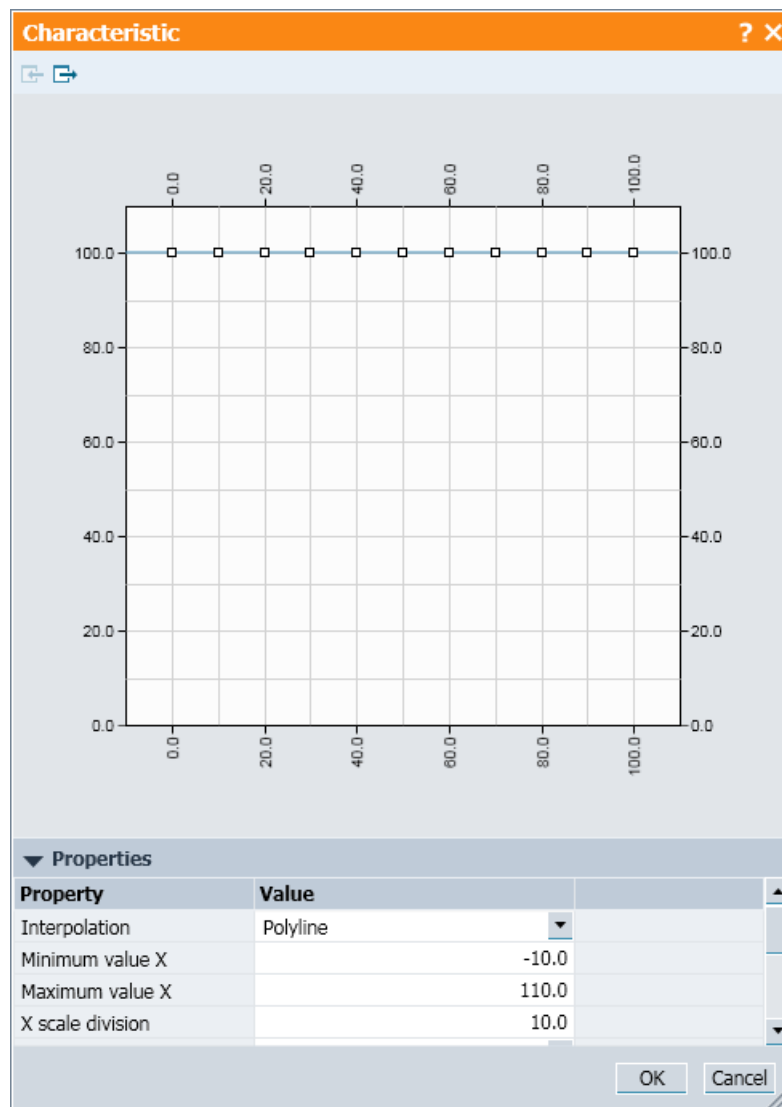
Bild 8-66 Parameter AgitatorInfluence des Komponententyps HeatingJacket
