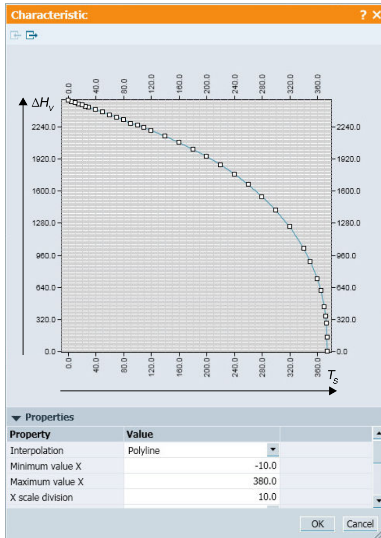
Bild 8-14 Verdampfungsenthalpie Komponententyp Condenser
