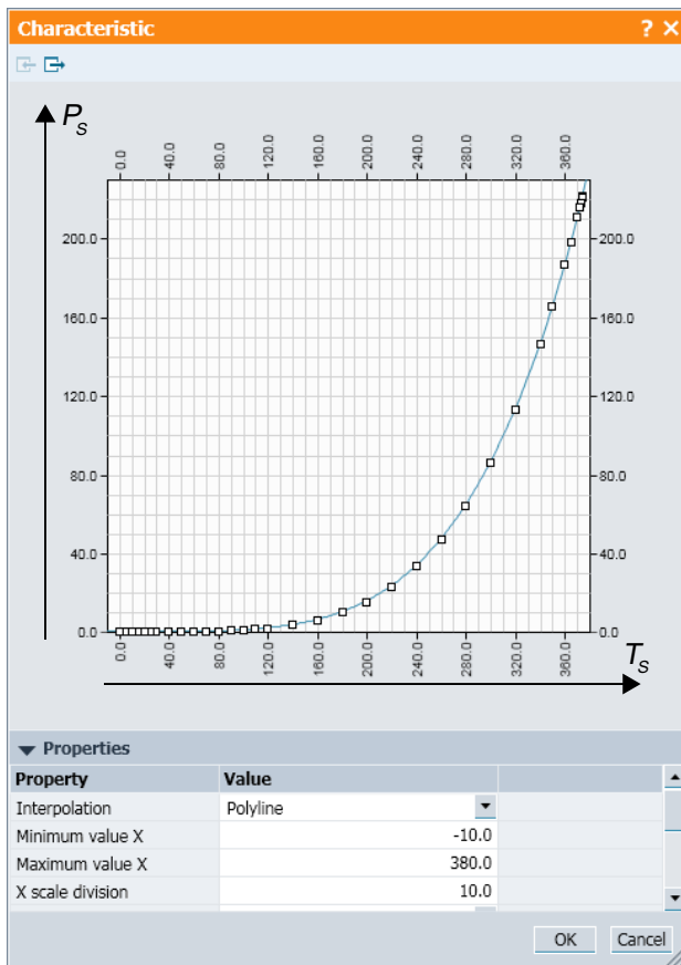
Bild 8-68 Beispiel für Verdampfungsenthalpie und Dampfdruckkurve
