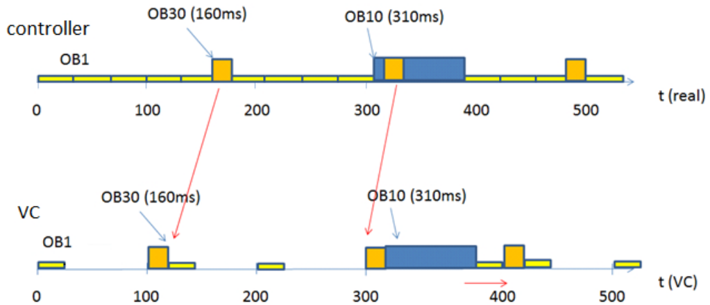
Bild 2-1 Ablaufsteuerung
