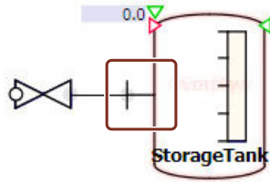
Bild 8-8 Beispielverschaltung Komponententyp Nozzle mit StorageTankLiquid
