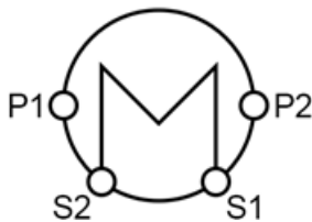
Bild 8-16 Symbol des Komponententyps HeatExchangerGeneral
