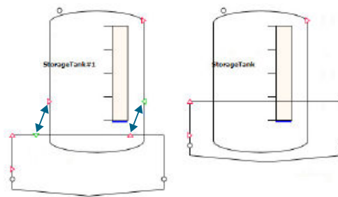
Bild 8-65 Symbol des Komponententyps HeatingJacket in Verbindung mit der Komponente StorageTankLiquid, Darstellung der zu verbindenden Anschlüsse
