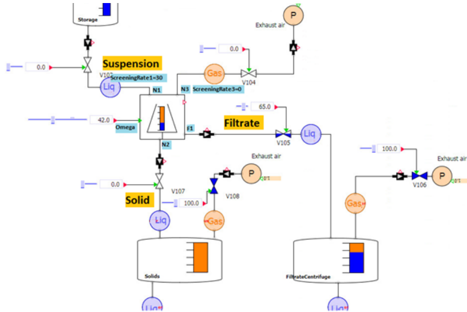
Bild 8-44 Beispielverschaltung des Komponententyps Zentrifuge
