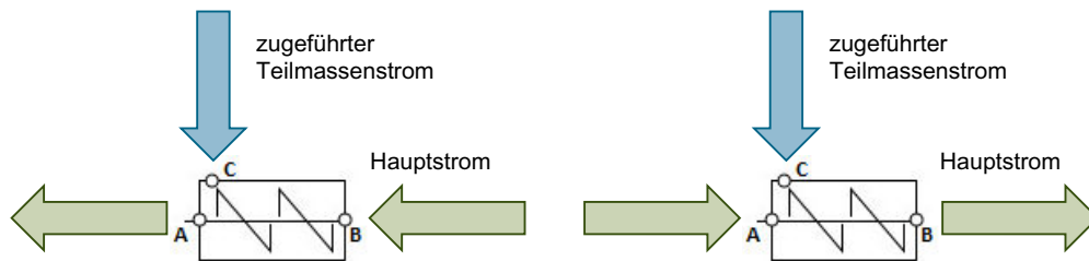
Bild 8-38 Strömungsmöglichkeiten im Komponententyp Mixer
