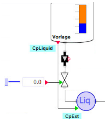
Bild 8-57 Beispiel für die Verschaltung des Eingangs CpExt
