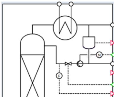
Darstellung: Pumpe im Rücklauf
