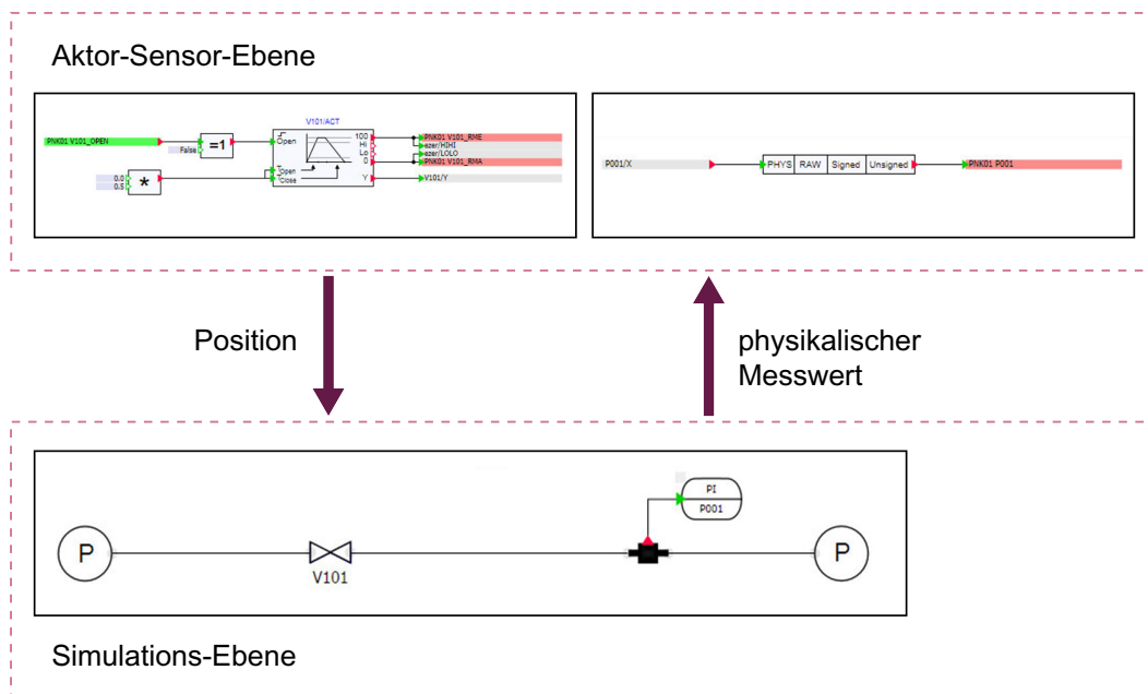
Bild 8-1 Schematische Kopplung der Aktor-Sensor-Ebene mit der Simulationsebene
