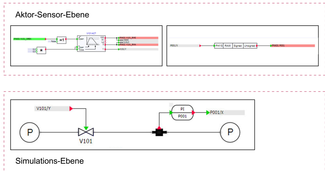
Bild 8-3 Kopplung der Aktor-Sensor-Ebene mit der Simulationsebene mittels Signallinien und Konnektoren
