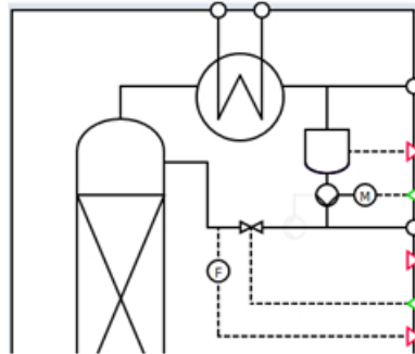
Pumpe für Rücklauf und Destillat
