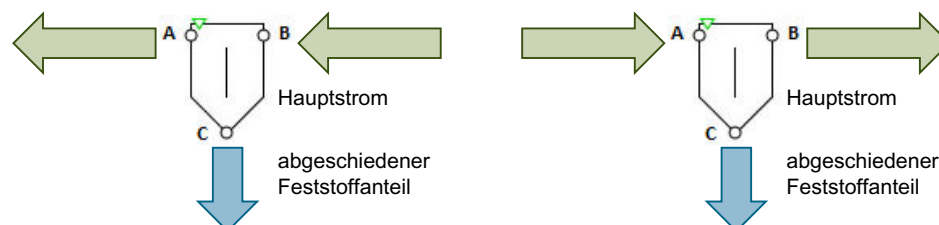
Bild 8-53 Strömungsmöglichkeiten des Komponententyps Separator
