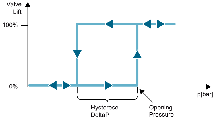
Bild 8-76 Öffnungs- und Schließverhalten des Sicherheitsventils
