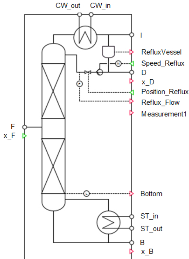
Symbol des Komponententyps Column
