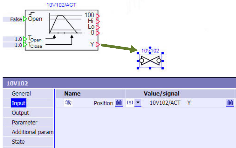
Bild 8-4 Implizite Kopplung des Komponententyps Valve mit einem Antrieb
