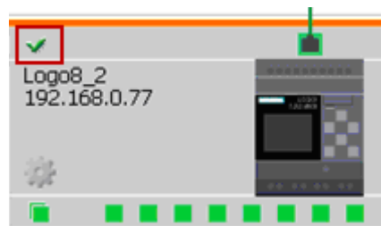
Dispositivo LOGO!
