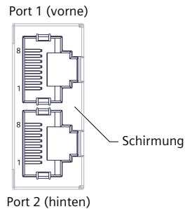
Bild 4-1 PROFINET Ports
