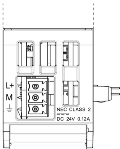
Figura 6-1 Connettore femmina per l'alimentazione esterna di CC 24 V (vista da sopra)
