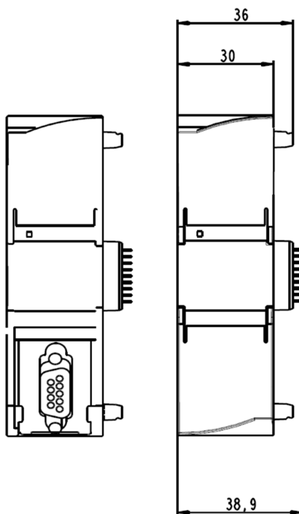
Figura A-1 CM 1243-5 - Vista anteriore
