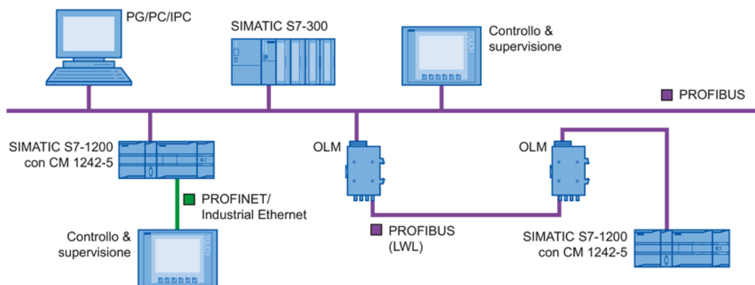
Figura 1-1 Esempio di configurazione con CM 1242-5 come slave PROFIBUS
